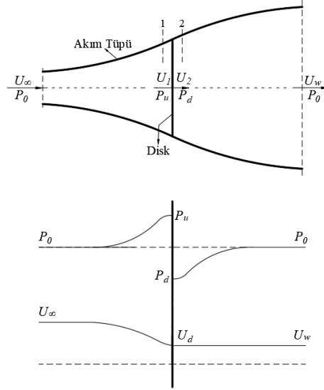
Şekil 20. Aktüatör disk metodu (Daniel ve Nicklas, 2013; Muratoğlu, 2014)
