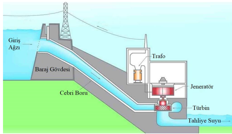
Şekil 5. Hidrostatik türbinlerin uygulama alanının genel görünümü (Mallı, 2017)
