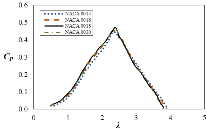
Şekil 33. Kanat kesiti-Güç katsayısı grafiği
