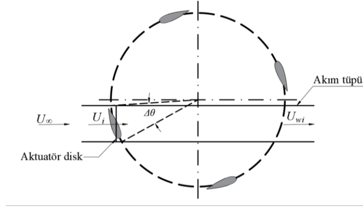
Şekil 22. Çoklu akım tüpü modeli (Daniel ve Nicklas, 2013)
