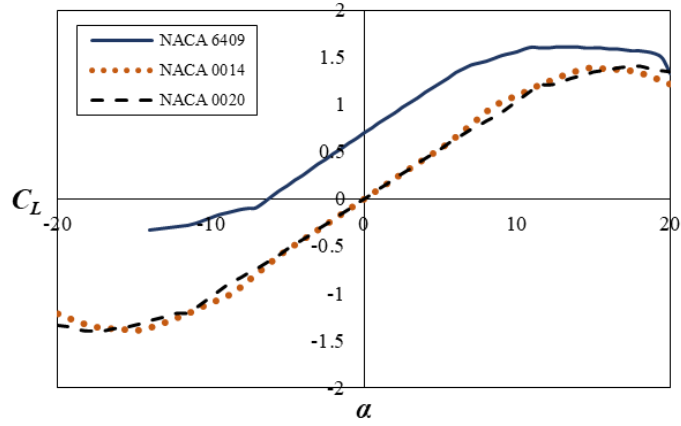
Şekil 32. Simetrik ve asimetrik kesitlerin performans karşılaştırması
