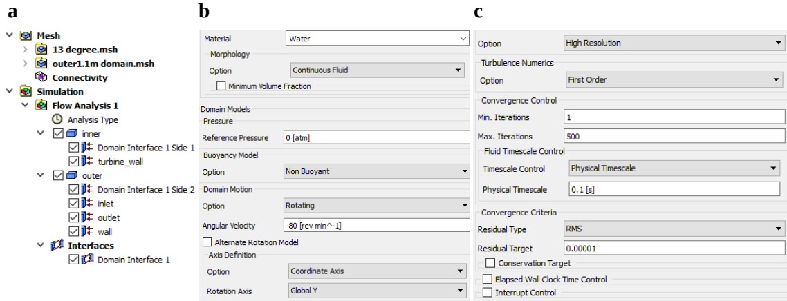
Şekil 31. CFX çözüm bölümünün oluşturulması
