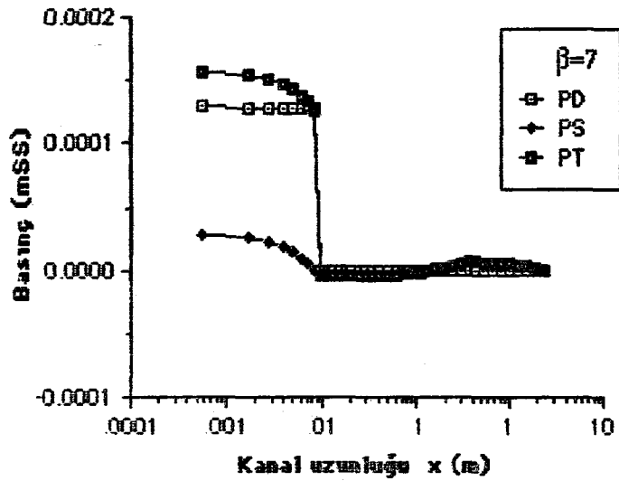
Şekil 6.2.70. \beta=7 çap oranı için toplam baskı P_T , dinamik baskı P_D , statik baskı P_S 'nin x eksenini boyunca değişimi ( Re_d=100 , Silindirik koordinat).
