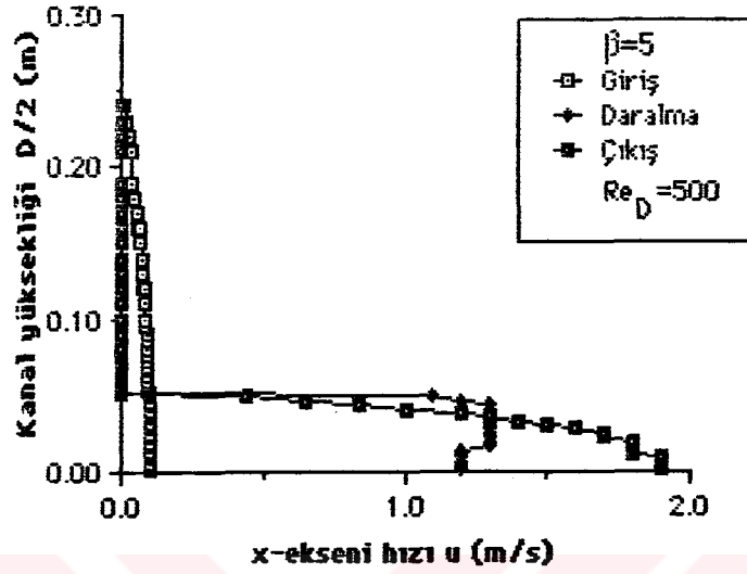
Şekil 6.3.19. Çap oran \beta=5 için eksenel hız u 'nun kanal boyunca değişik x mesafelerindeki hız profilinin değişimi ( Re_D=500 , Silindirik koordinat).
