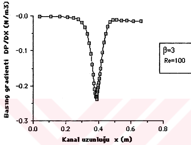
Şekil 6.3.33 \beta=3 çap oranı için basınç gradienti'nin x eksenı boyunca değışimi ( Re_D=100 , Kartezyen koordinat)
