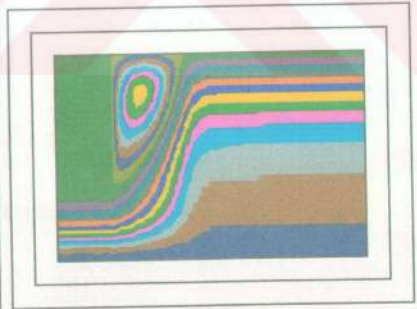
Şekil 6.2.83 Ani genişleme için akım çizgileri ( \beta=4 Re=50 )
