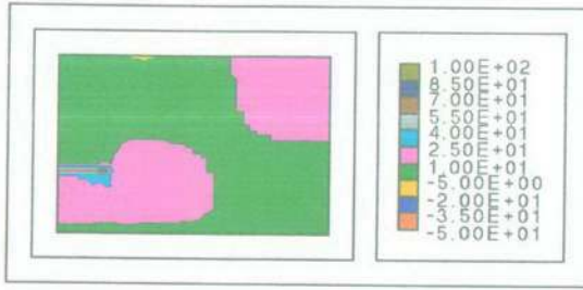
Şekil 6.2.102 Ani genişleme için girdap konturları ( \beta=2 , Re=100 )
