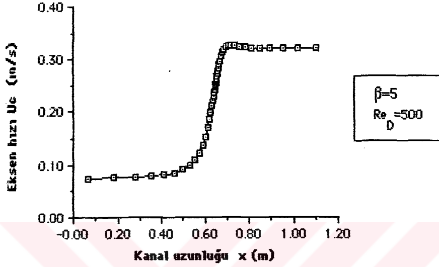
Şekil 6.3.25. \beta=5 çap oranı için simetri eksenindeki U_c hızının x eksenı boyunca değişimi ( Re_D=500 , Kartezyen koordinat)
