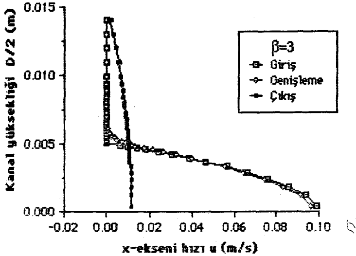
Şekil 6.2.48. \beta=3 çap oranı için kanal boyunca değişik x mesafelerindeki eksenel hız profilleri ( Re_d=100 , Silindirik koordinat).
