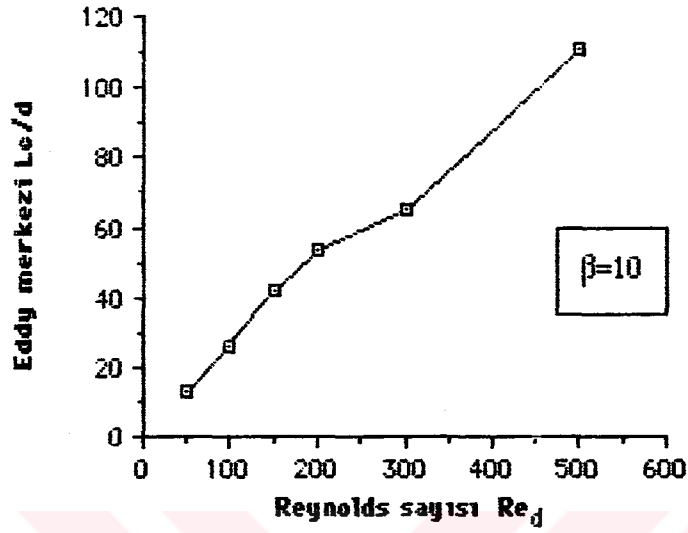
Şekil 6.2.29. \beta=10 çap oranı için değişik Reynolds sayılarında eddy merkezinin yeri L_e 'nin değişimi (Kartezyen Koordinat).
