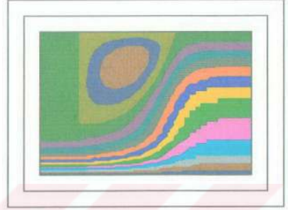
Şekil 6.2.95. Ani genişleme için akım çizgileri ( \beta=4 , Re=200 , S.K.)
