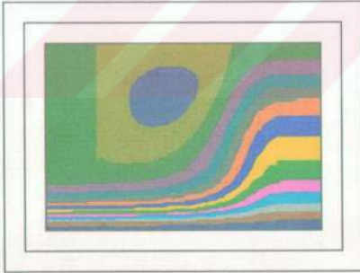
Şekil 6.2.93 Ani genişleme için akım çizgileri( \beta=2 Re=200 S.K)
