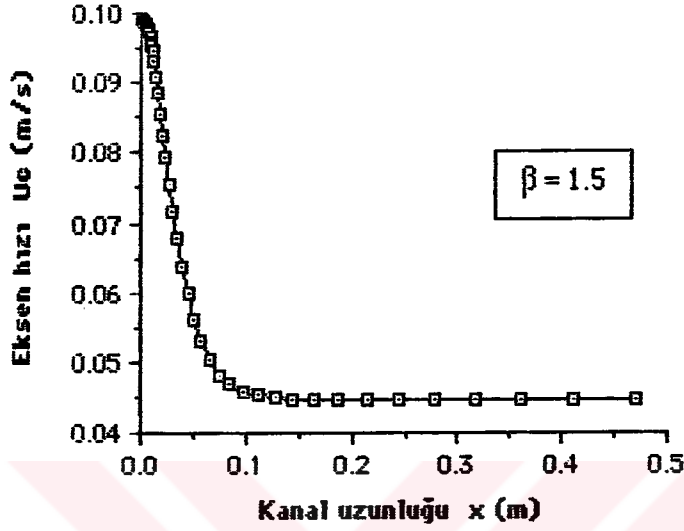
Şekil 6.2.55. \beta=1.5 çap oranı için kanal boyunca ekseneki u_c hızı'nın değişimi ( Re_d=100 , Silindirik koordinat).
