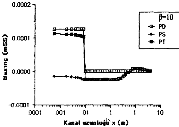
Şekil 6.2.74. \beta=10 çap oranı için toplam basınç P_T , dinamik basınç P_D , statik basınç P_S 'nin x eksenı boyunca değışimi ( Re_d=100 , Silindirik koordinat).
