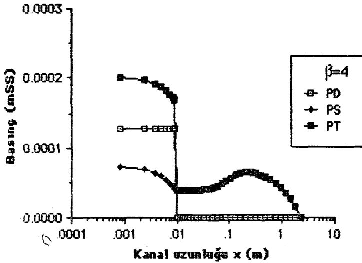
Şekil 6.2.68. \beta=4 çap oranı için toplam baskı P_T , dinamik baskı P_D , statik baskı P_S 'nin x eksenı boyunca değışimi ( Re_d=100 , Silindirik koordinat).
