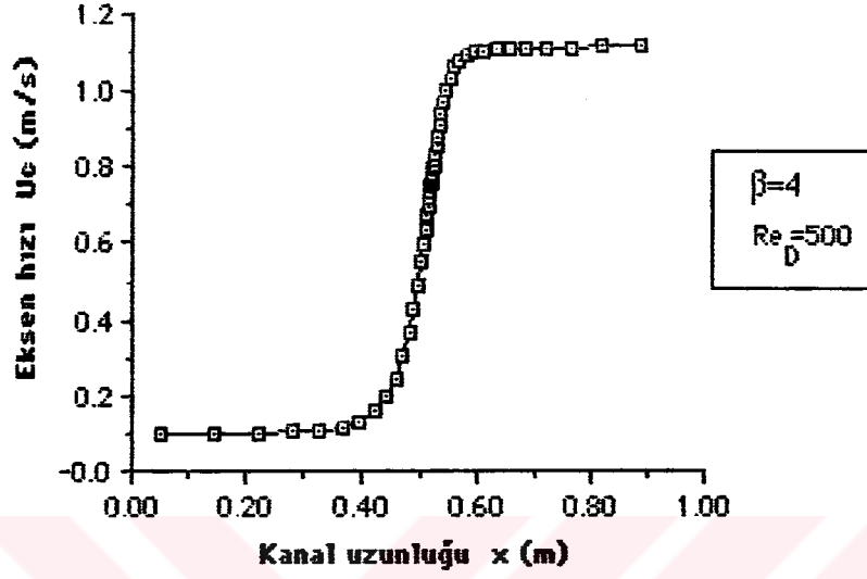
Şekil 6.3.23. \beta=4 çap oranı için simetri eksenindeki U_c hızının x ekseni boyunca değişimi ( Re_D=500 , Silindirik koordinat)
