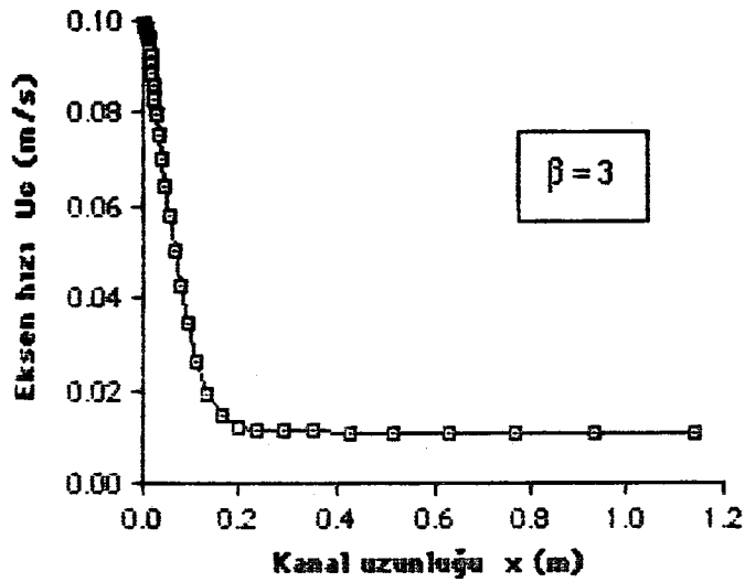
Şekil 6.2.56. \beta=3 çap oranı için kanal boyunca ekseneki u_c hızı'nın değişimi ( Re_d=100 , Silindirik koordinat).
