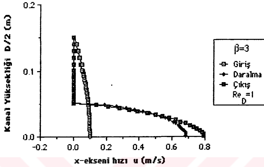
Şekil 6.3.17. \beta=3 çap oranı için eksenel hız u 'nun kanal boyunca değişik x mesafelerindeki hız profilinin değişimi ( Re_D=1 , Silindirik koordinat).
