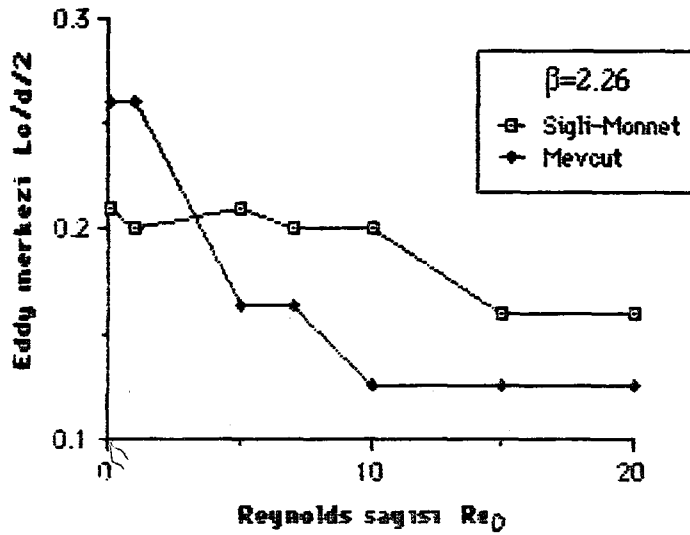
Şekil 6.3.2. \beta=2.26 çap oranı için eddy merkezinin daralma başlangıcına olan mesafesi L_o 'nin farklı Re_D sayılarına göre değişiminin Sigli-Monnet'in deneysel çalışmalarıyla karşılaştırılması (creeping flow-Silindirik koordinat).
