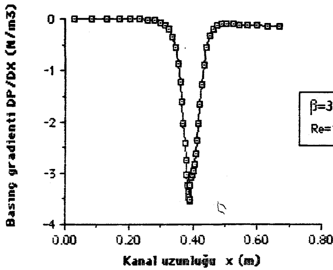
Şekil 6.3.32. \beta=3 çap oranı için basınç gradienti'nin x eksenı boyunca değışimi ( Re_D=100 , Silindirik koordinat)
