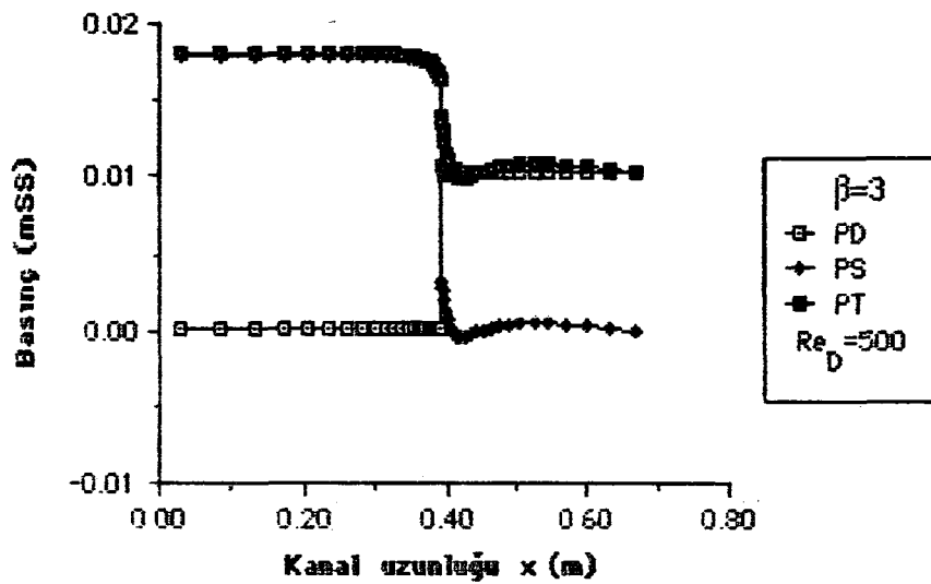
Şekil 6.3.28. \beta=3 çap oranı için dinamik basınç P_D , statik basınç P_S ve toplam basınç P_T 'nin x eksenı boyunca değışimi ( Re_D=500 , Silindirik koordinat)
