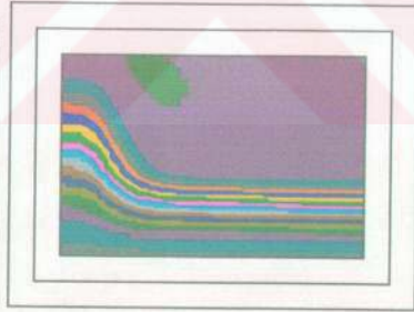
Şekil 6.3.37. \beta=2.26 çap oranı için anı daralma akım çizgileri ( Re=10 , S.K)
