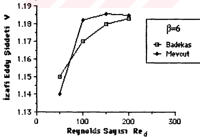
Şekil 6.2.38. \beta=6 çap oranı için değişik Reynolds sayılarında izafi eddy şiddeti Y'nin Badekas'ın sayısal sonuçları ile karşılaştırılması (Silindirik Koordinat).
