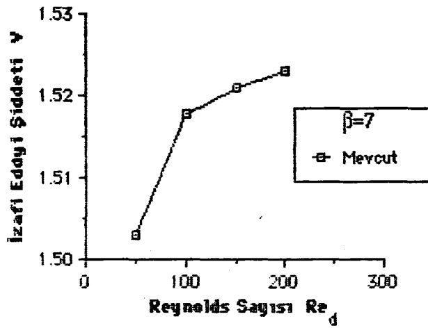
Şekil 6.2.40. \beta=7 çap oranı için değişik Reynolds sayılarında izafi eddy şiddeti Y 'nin değişimi (Silindirik Koordinat).
