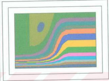
Şekil 6.2.81 Ani genişleme için akım çizgileri ( \beta=2 Re=50 )
