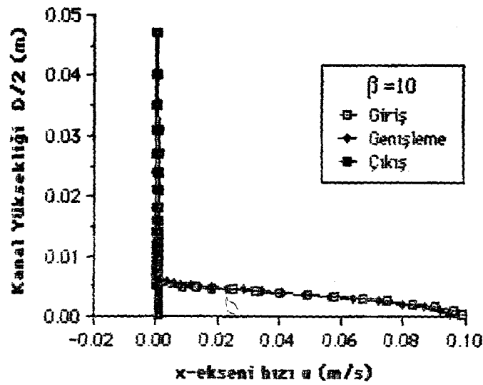
Şekil 6.2.52. \beta=10 çap oram için kanal boyunca değişik x mesafelerindeki eksenel hız profilleri ( Re_d=100 , Silindirik koordinat).
