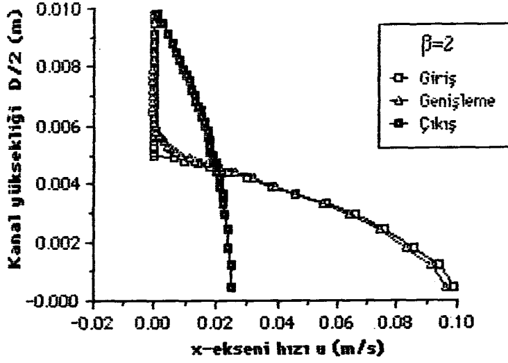
Şekil 6.2.47. \beta=2 çap oranı için kanal boyunca değişik x mesafelerindeki eksenel hız profilleri ( Re_d=100 , Silindirik koordinat).
