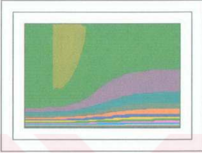
Şekil 6.2.95 Ani genişleme için akım çizgileri ( \beta=1.5 , Re=200 , S.K.)
