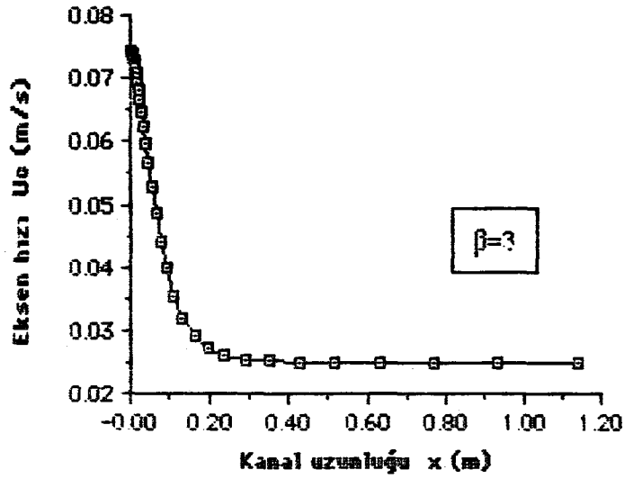
Şekil 6.2.60. \beta=3 çap oranı için kanal boyunca eksendeki u_c hızı'nın değişimi ( Re_d=100 , Kartezyen koordinat).
