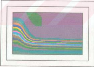
Şekil 6.3.36. \beta=2.26 çap oranı için anı daralma akım çizgileri ( Re=0.1 , S.K)
