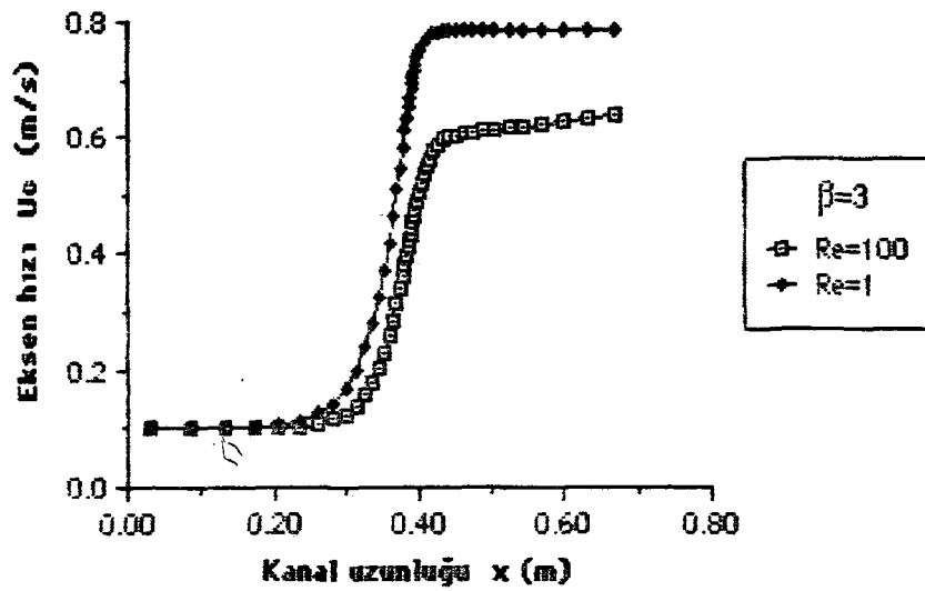
Şekil 6.3.26. \beta=3 çap oranı için simetri eksenindeki U_c hızının iki farklı Reynolds sayısı için x eksenı boyunca değişimi (Silindirik koordinat)
