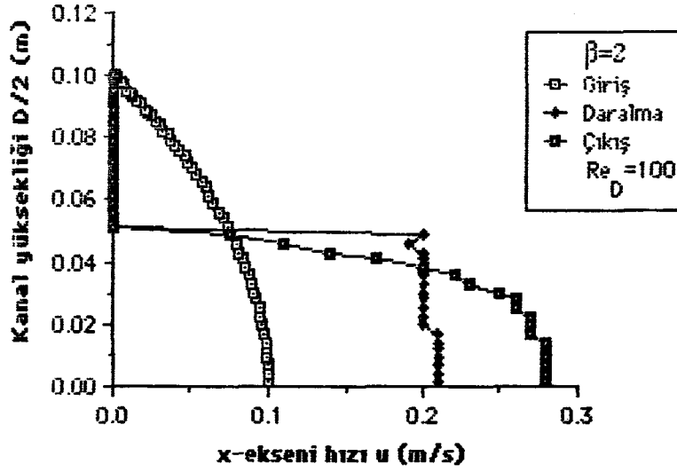
Şekil 6.3.15. \beta=2 çap oranı için aksenal hız u 'nun kanal boyunca değişik x mesafelerindeki hız profilinin değişimi ( Re_D=100 , Silindirik koordinat).
