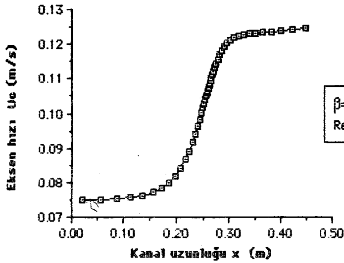
Şekil 6.3.24. \beta=2 çap oranı için simetri eksenindeki U_c hızının x ekseni boyunca değişimi ( Re_D=100 , Kartezyen koordinat)
