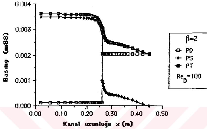
Şekil 6.3.27. \beta=2 çap oranı için dinamik basınç P_D , statik basınç P_S ve toplam basınç P_T 'nin x eksenı boyunca değışimi ( Re_D=100 , Silindirik koordinat)
