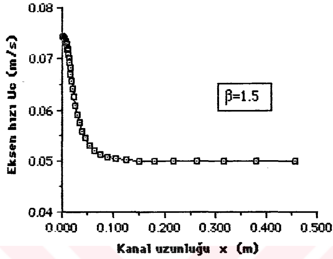
Şekil 6.2.59. \beta=1.5 çap oranı için kanal boyunca eksendeki u_c hızı'nın değişimi ( Re_d=100 , Kartezyen koordinat).
