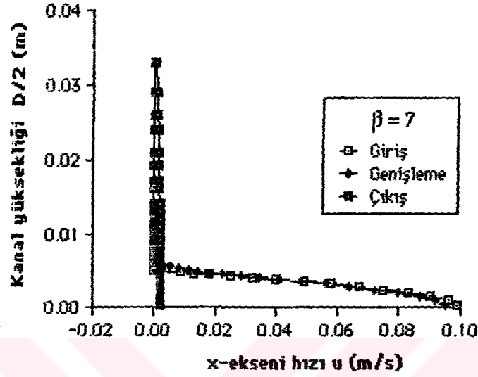
Şekil 6.2.51. \beta=7 çap oram için kanal boyunca değişik x mesafelerindeki eksenel hız profilleri ( Re_d=100 , Silindirik koordinat).
