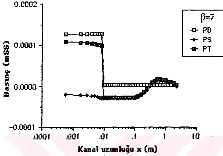
Şekil 6.2.73. \beta=7 çap oranı için toplam basınç P_T , dinamik basınç P_D , statik basınç P_S 'nin x eksenı boyunca değışimi ( Re_d=100 , Kartezyen koordinat).
