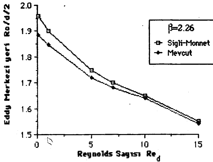
Şekil 6.2.2. \beta=2.26 çap oranı için değişik Reynolds sayılarında eddy merkezi'nin eksen'e olan mesafesi R_c 'nin Sigli-Monnet'in deneysel sonuçları ile karşılaştırılması (Silindirik koordinat).
