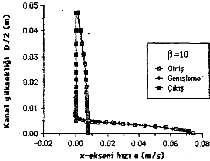
Şekil 6.2.54. \beta=10 çap oranı için kanal boyunca değişik x mesafelerindeki eksenel hız profilleri ( Re_d=100 , Kartezyen koordinat).
