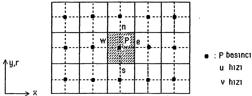
Şekil.3.2. Şaşırtmasız grid sistemi şeması
