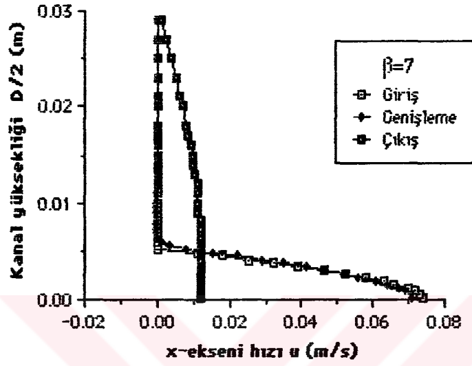
Şekil 6.2.53. \beta=7 çap oranı için kanal boyunca değişik x mesafelerindeki eksenel hız profilleri ( Re_d=100 , Kartezyen koordinat).
