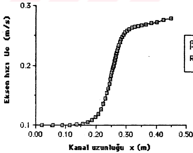
Şekil 6.3.22. \beta=2 çap oranı için simetri eksenindeki U_c hızının x eksenı boyunca değişimi ( Re_D=100 , Silindirik koordinat)
