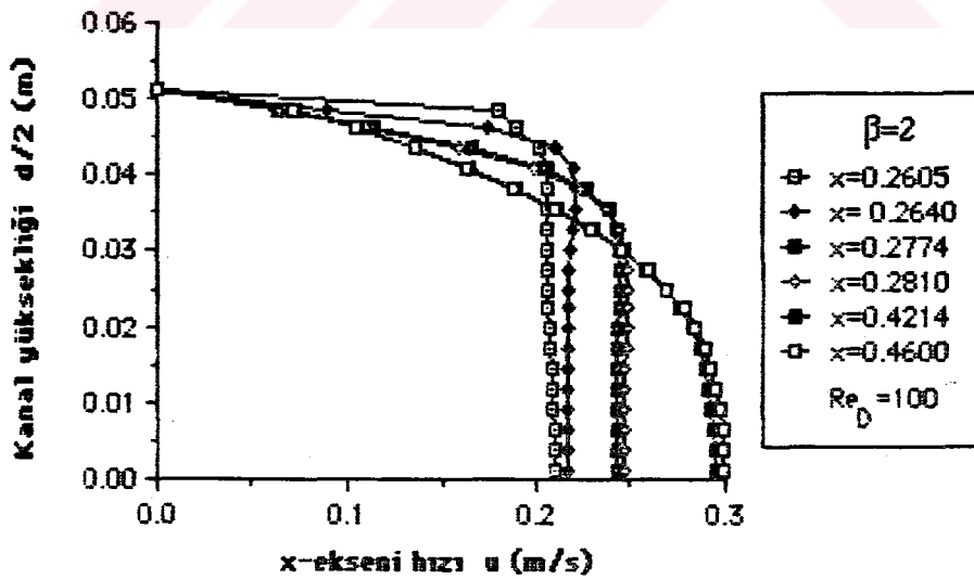
Şekil 6.3.16. \beta=2 çap oranı için aksenal hız u 'nun daralan kanal boyunca değişik x mesafelerindeki hız profilinin değişimi ( Re_D=100 , Silindirik koordinat).
