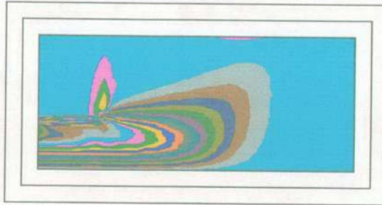
Şekil 6.2.104 Ani genişleme için girdap konturları ( \beta=6 , Re=100 )
