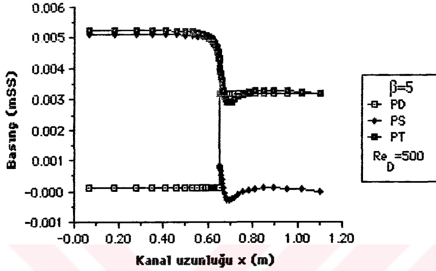
Şekil 6.3.31. \beta=5 çap oranı için dinamik basınç P_D , statik basınç P_S ve toplam basınç P_T 'nin x eksenı boyunca değışimi ( Re_D=500 , Kartezyen koordinat)
