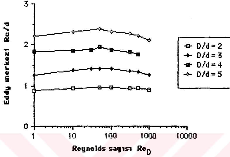
Şekil 6.3.13. Değişik çap oranları için eddy merkezinin simetri eksenine olan mesafe Re/d 'nin farklı Re_D sayılarına göre değişimi (Kartezyen koordinat).
