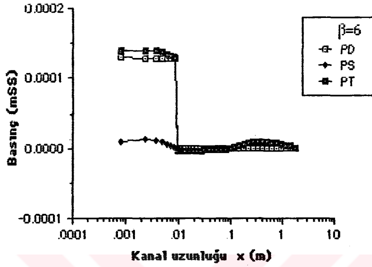
Şekil 6.2.69. \beta=6 çap oranı için toplam baskı P_T , dinamik baskı P_D , statik baskı P_S 'nin x eksenini boyunca değişimi ( Re_d=100 , Silindirik koordinat).
