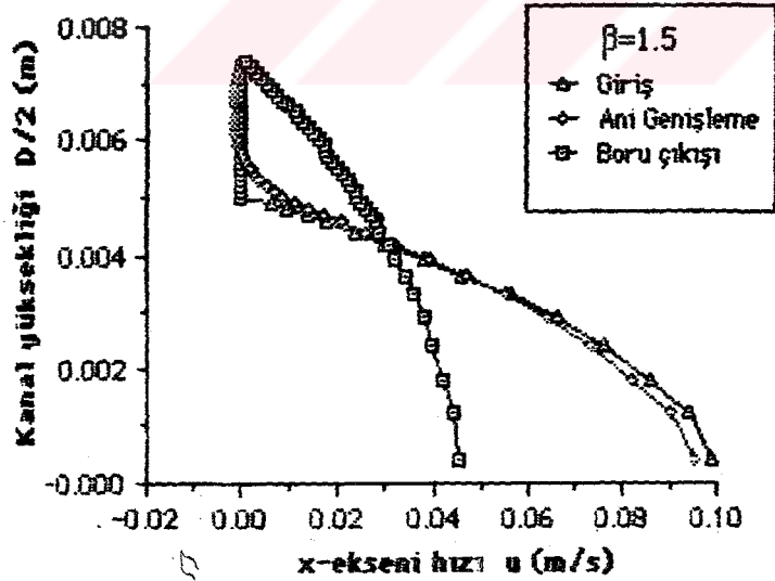
Şekil 6.2.46. \beta=1.5 çap oranı için kanal boyunca değişik x mesafelerindeki aksenal hız profilleri ( Re_d=100 , Silindirik koordinat).
