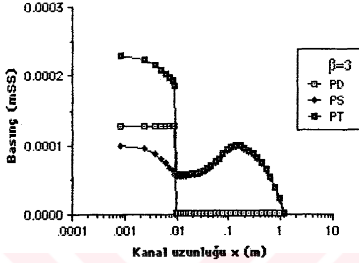
Şekil 6.2.67. \beta=3 çap oranı için toplam baskı P_T , dinamik baskı P_D , statik baskı P_S 'nin x eksenı boyunca değışimi ( Re_d=100 , Silindirik koordinat).
