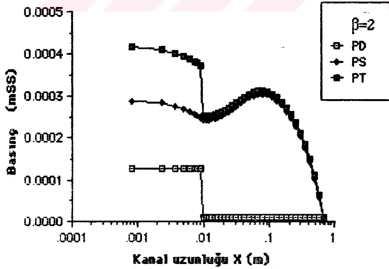
Şekil 6.2.66. \beta=2 çap oranı için toplam basınç P_T , dinamik basınç P_D , statik basınç P_S 'nin x eksenı boyunca değişimi ( Re_d=100 , Silindirik koordinat).
