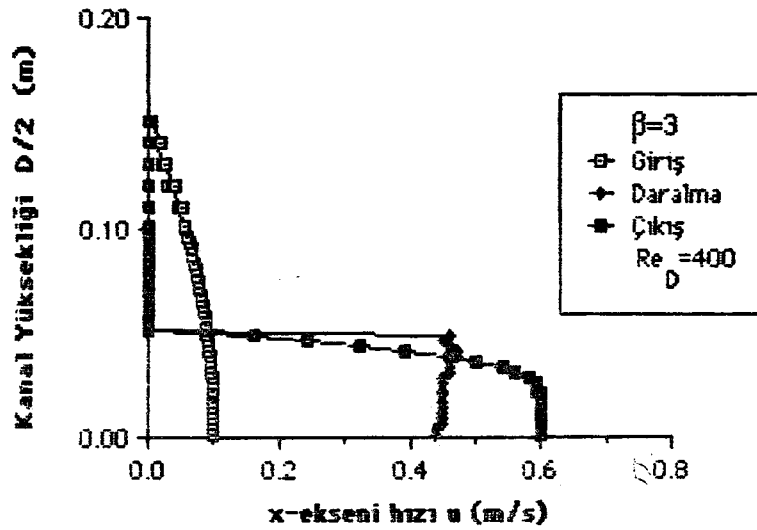
Şekil 6.3.18. \beta=3 çap oranı için eksenel hız u 'nun kanal boyunca değişik x mesafelerindeki hız profilinin değişimi ( Re_D=400 , Silindirik koordinat).
