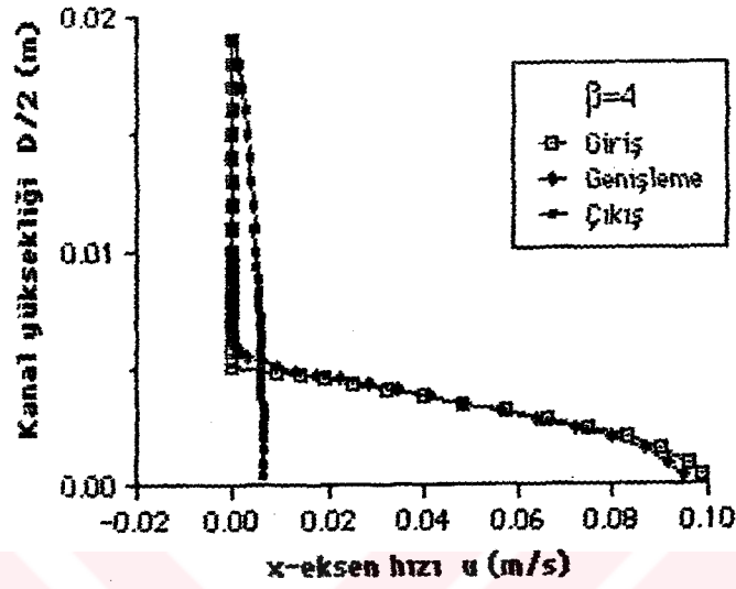
Şekil 6.2.49. \beta=4 çap oranı için kanal boyunca değişik x mesafelerindeki eksenel hız profilleri ( Re_D=100 , Silindirik koordinat).
