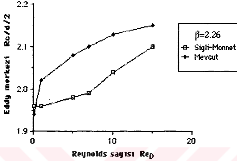
Şekil 6.3.3. \beta=2.26 çap oranı için eddy merkezinin simetri eksenine olan mesafesi R_0 'nin farklı Re_D sayılarına göre değişiminin Sigli-Monnet'in deneysel çalışmalarıyla karşılaştırılması (creeping flow, Silindirik koordinat).
