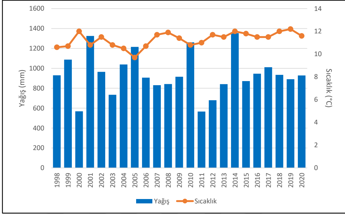
Grafik 6: 1998-2020 Yıl Aralığında Tuzla'nın Yıllara Göre Ortalama Sıcaklık ve Yağış Değerleri
