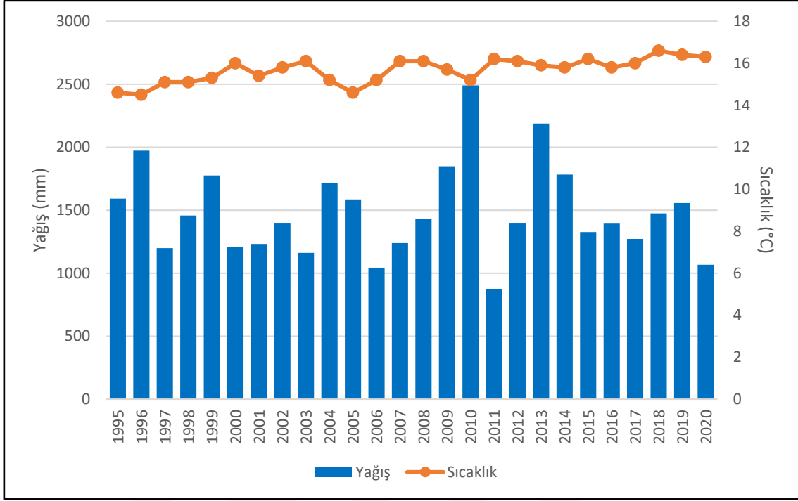
Grafik 4: 1995-2020 Yıl Aralığında Mostar'ın Yıllara Göre Ortalama Sıcaklık ve Yağış Değerleri
