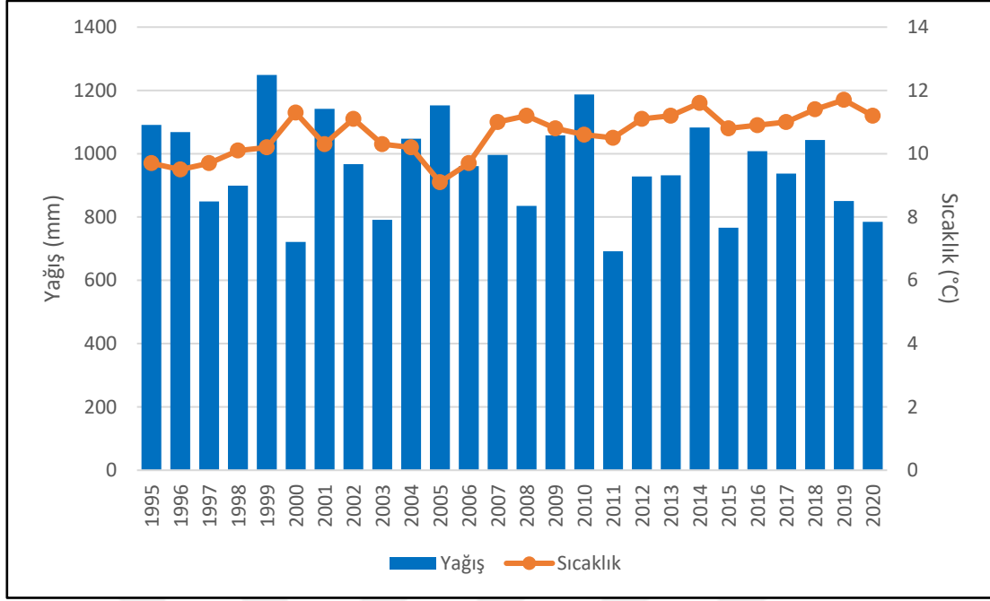
Grafik 2: 1995-2020 Yıl Aralığında Saraybosna'nın Yıllara Göre Ortalama Sıcaklık ve Yağış Değerleri
