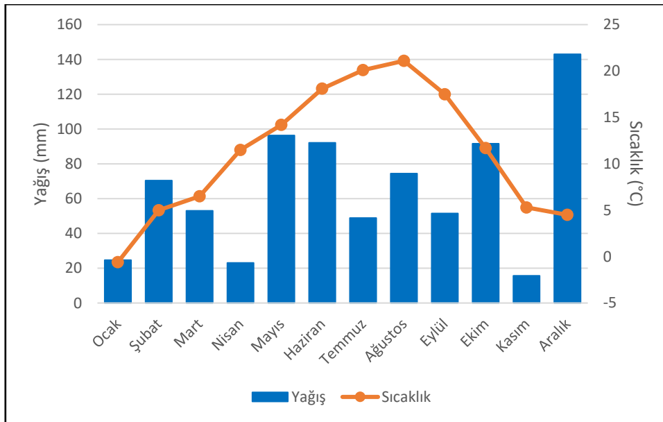
Grafik 1: Saraybosna'da 2020 Yılında Görülen Aylık Yağış ve Sıcaklık Değerleri
