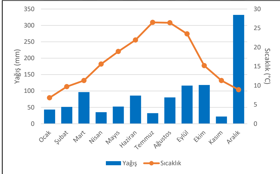
Grafik 3: Mostar'da 2020 Yılında Görülen Aylık Yağış ve Sıcaklık Değerleri
