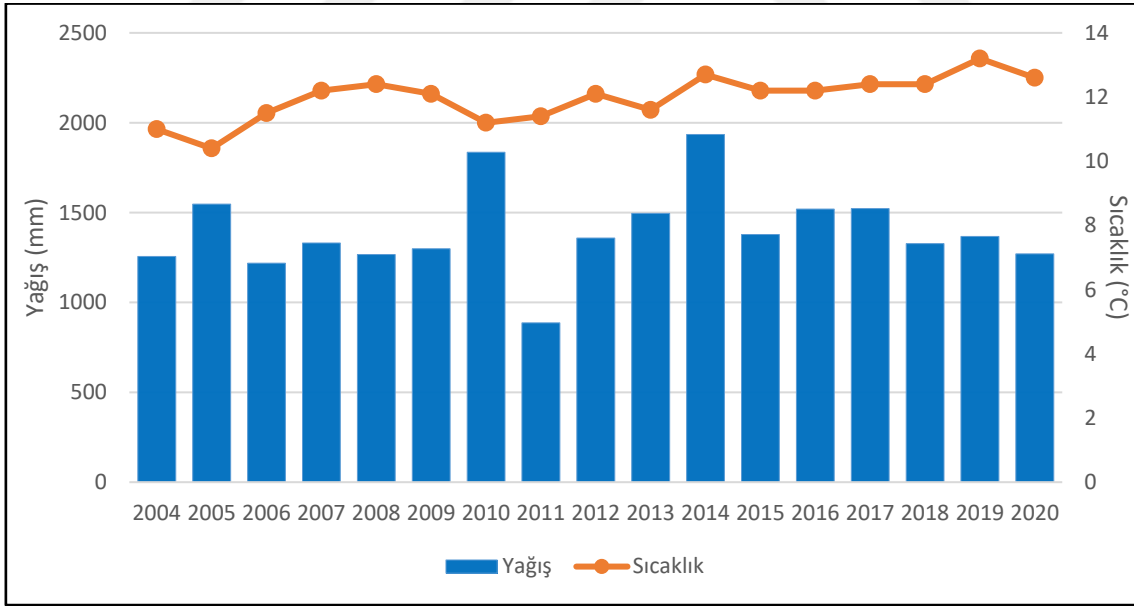
Grafik 5: 2004-2020 Yıl Aralığında Bihaç'ın Yıllara Göre Ortalama Sıcaklık ve Yağış Değerleri
