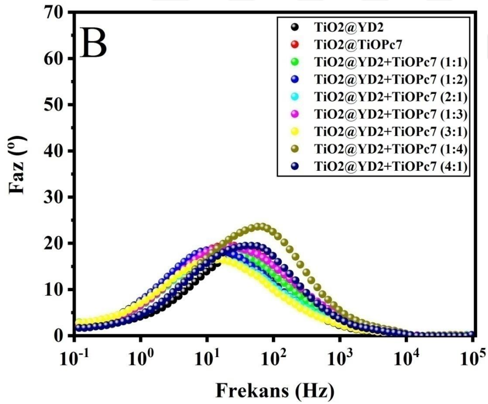
Şekil 4.38. \text{TiO}_2@\text{YD2} , \text{TiO}_2@\text{TiOPc7} ve \text{TiO}_2@\text{YD2}+\text{TiOPc7} fotoanotlarına ait A)Nyquist B)Bode eğrileri
