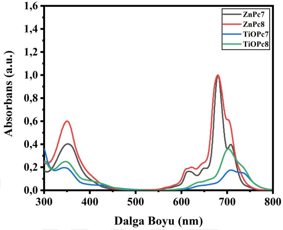
Şekil 4.19. ZnPc7-8 ve TiOPc7-8 boyaların UV-Vis spekturumları
