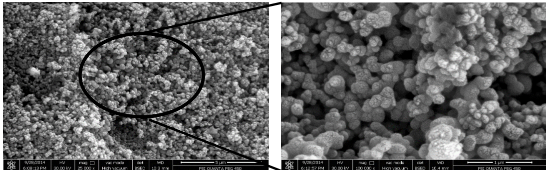
Şekil 4.9. \text{FTO@TiO}_2 fotoanoduna ait FE-SEM yüzey görüntüleri
