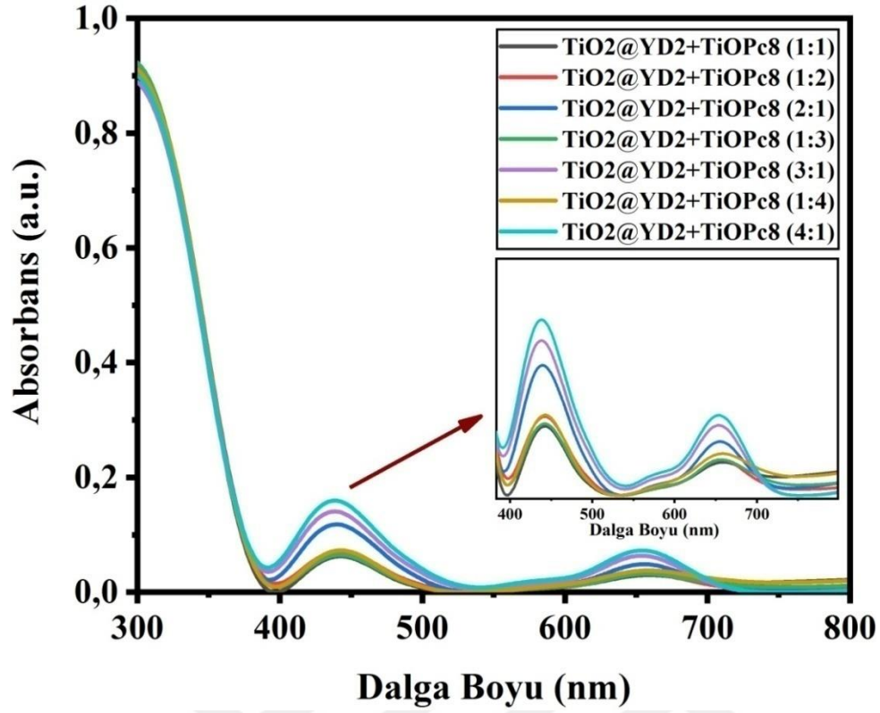
Şekil 4.29. \text{TiO}_2@\text{YD2}+\text{TiOPc8} fotoanotlarına ait UV-Vis spekturumları
