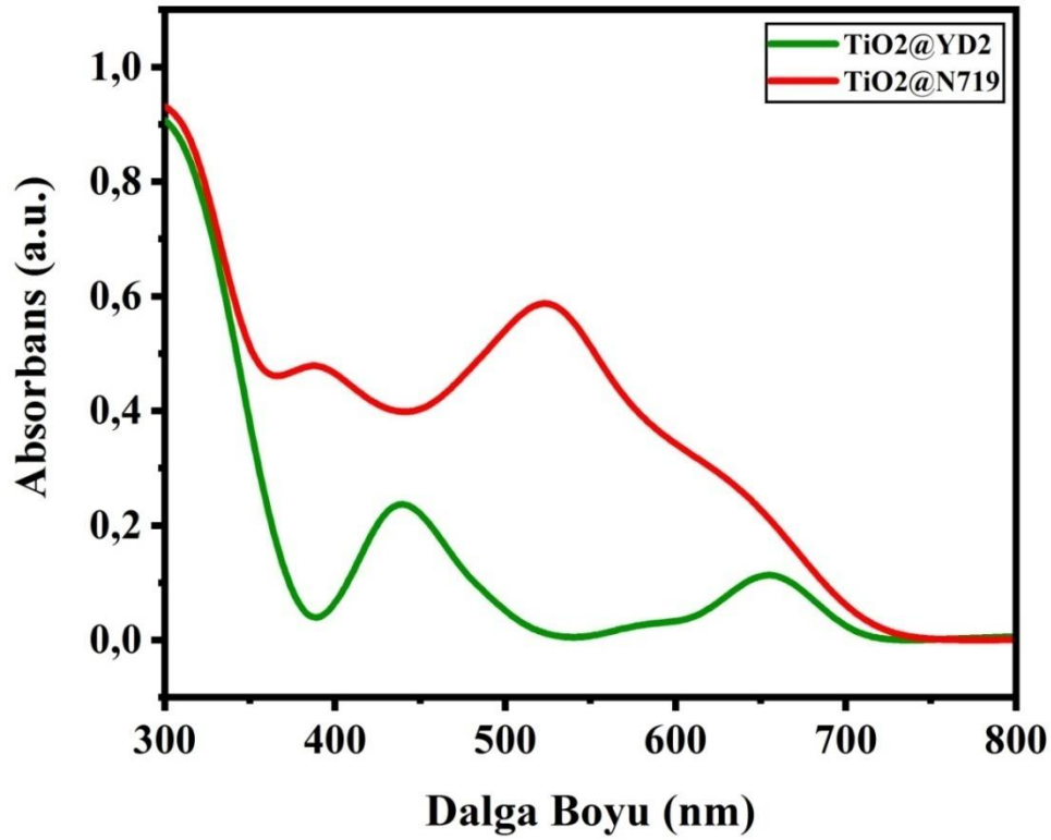
Şekil 4.30. \text{TiO}_2@\text{YD2} ve \text{TiO}_2@\text{N719} fotoanotlarına ait UV-Vis spekturumları
