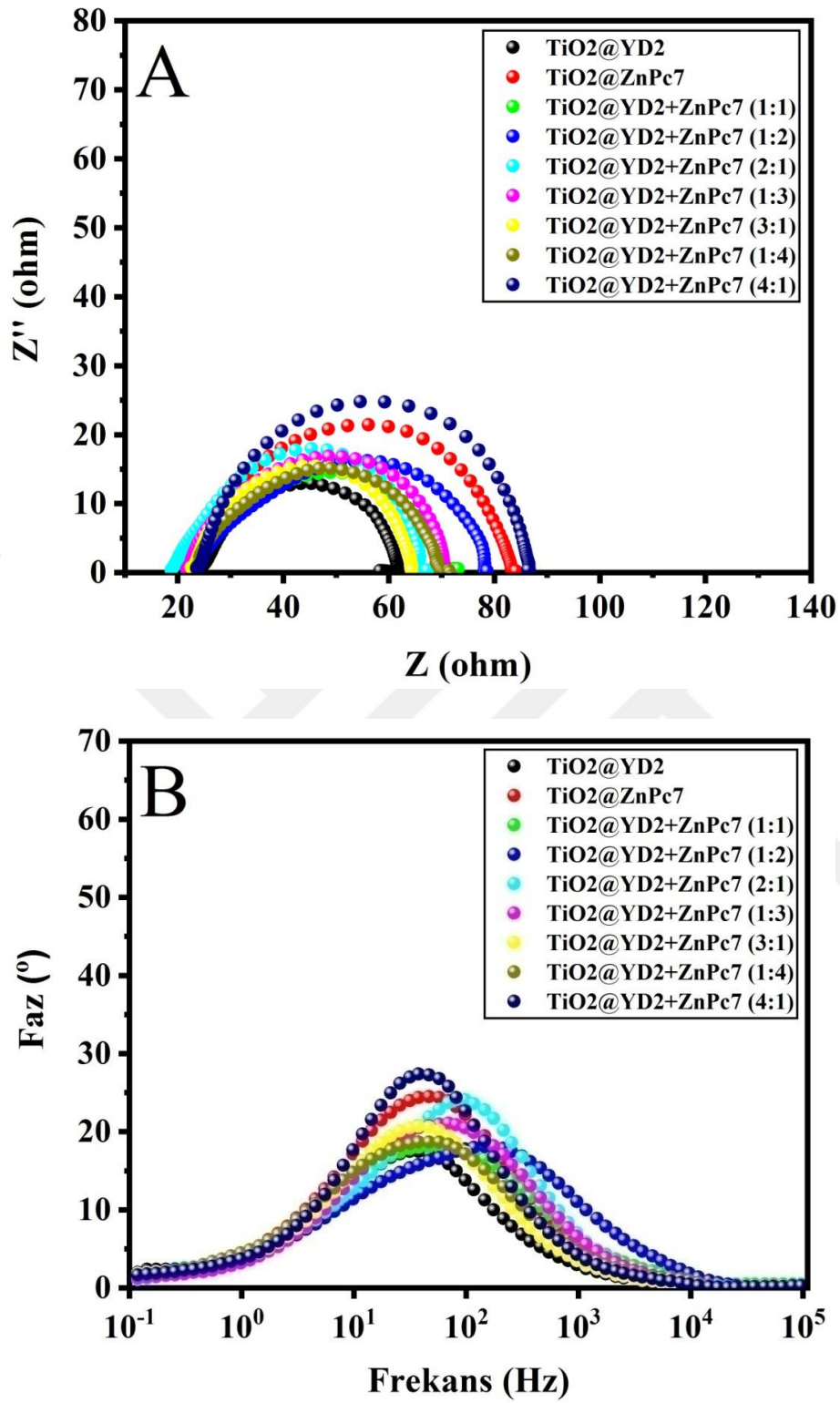
Şekil 4.36. TiO 2 @YD 2 , TiO 2 @ZnPc 7 ve TiO 2 @YD 2 +ZnPc 7 fotoanotlarına ait A)Nyquist B)Bode eğrileri
