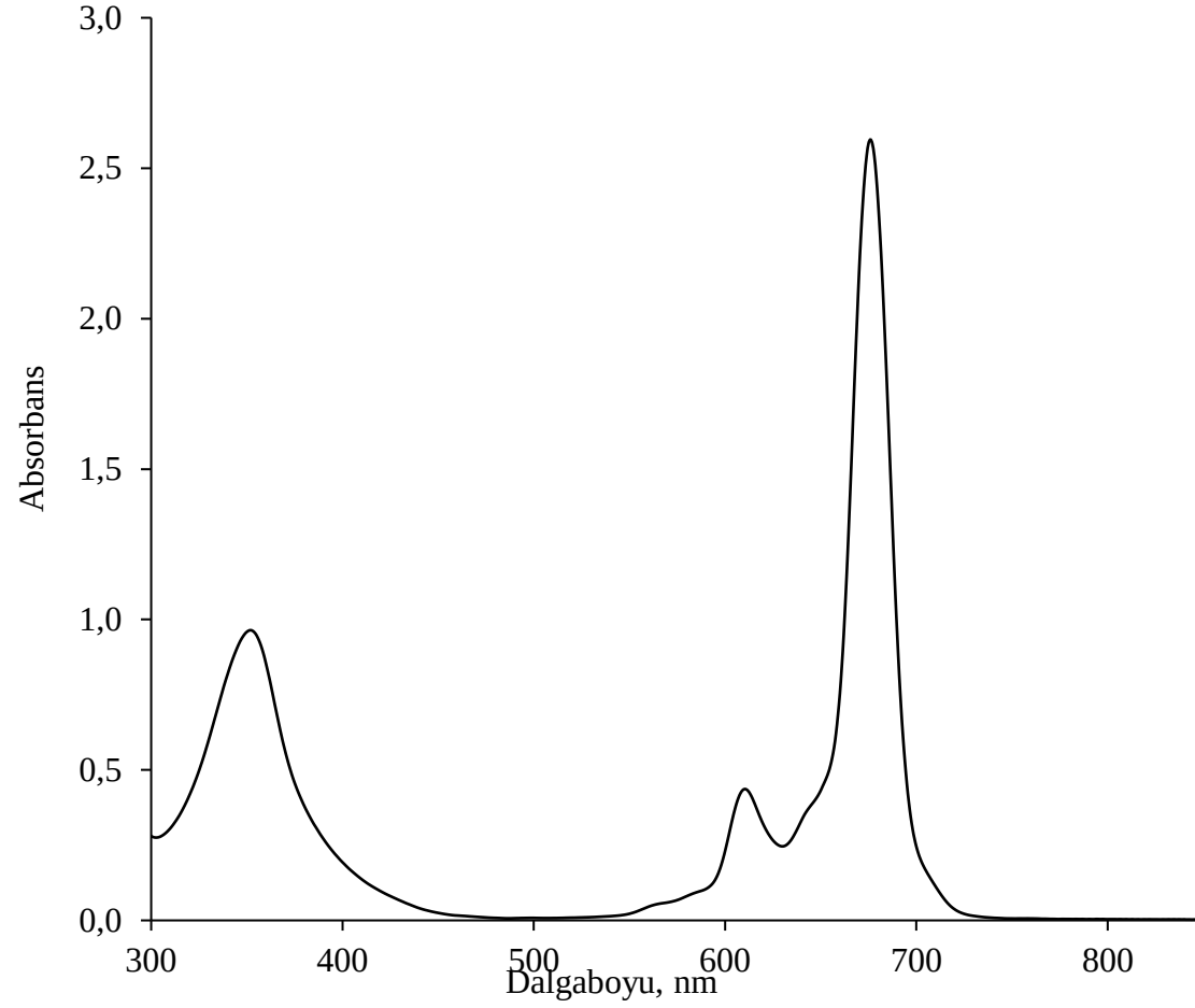
Şekil A.22. ZnPc8 bileşiğine ait THF çözücüsünde alınan UV-Vis spektrumu
