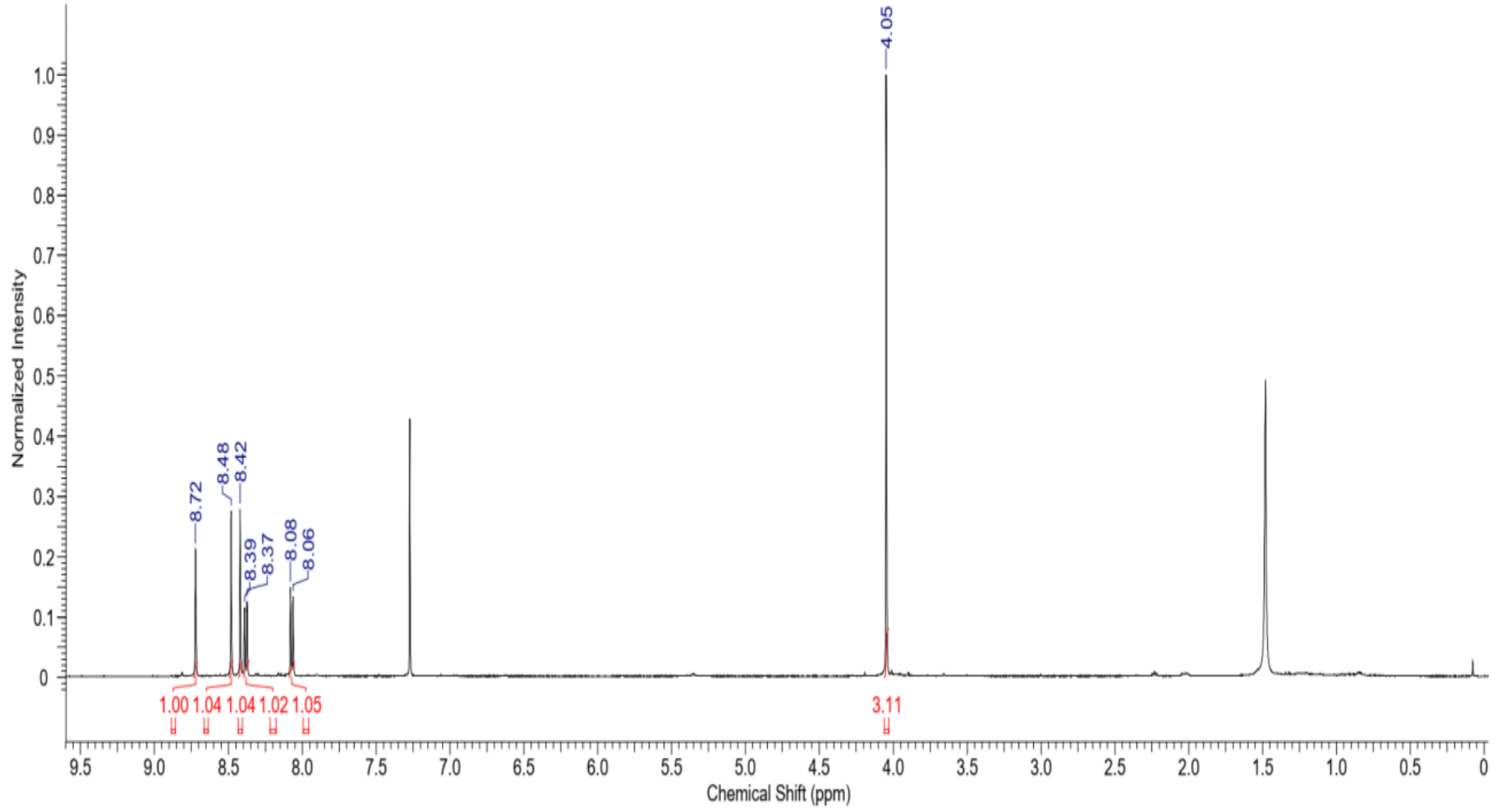
Şekil A.14. 6-Karboximetil-2,3-disiyanonaftalen (N3) bileşiğine ait \text{CDCl}_3 içinde alınmış ^1\text{H} -NMR spektrumu
