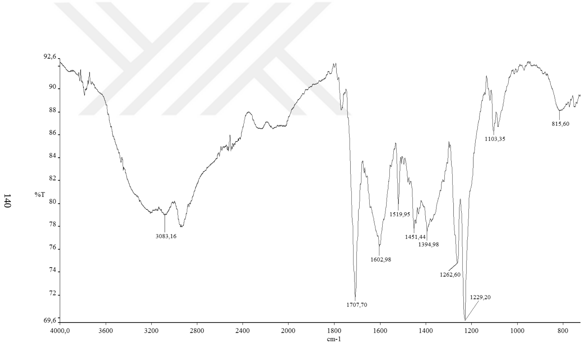
Şekil A.25. TiOPc7 bileşiğine ait FTIR spektrumu
