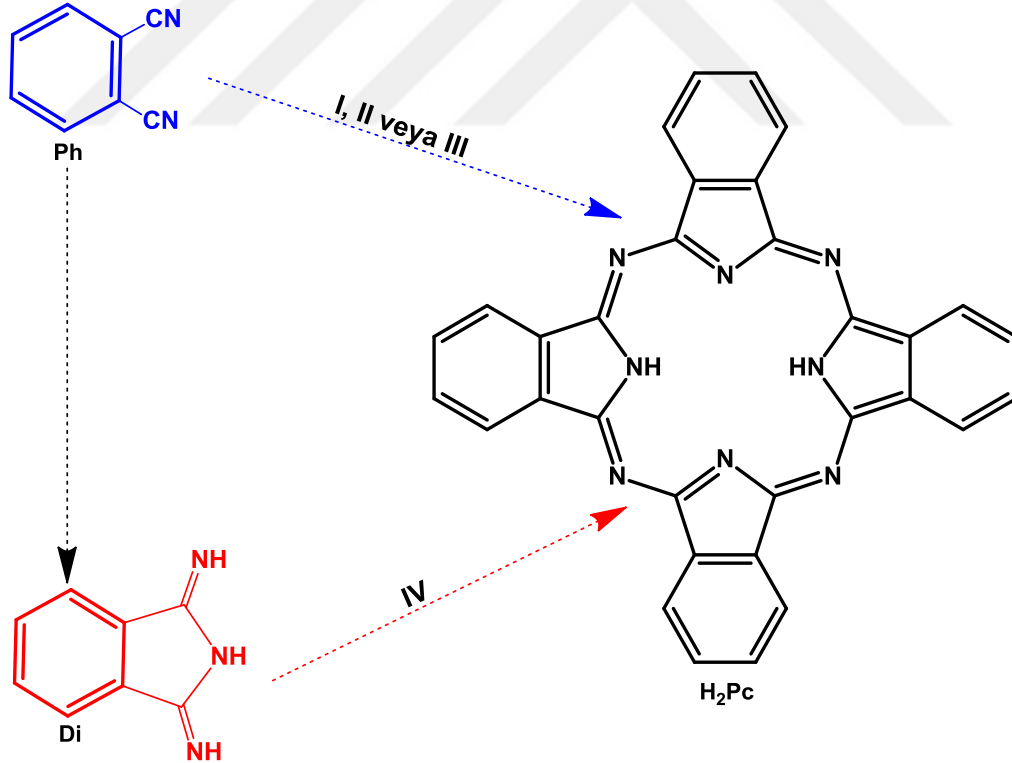
Şekil 2.2. Metallsız ftalosiyanınların ( H_2Pc ) sentez metotları
