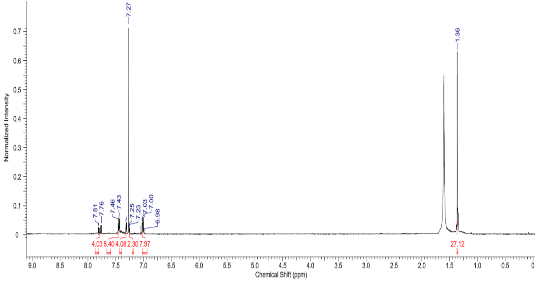
Şekil A.30. TiOPc8 bileşiğine ait CDCl 3 içinde alınmış 1 H-NMR spektrumu
