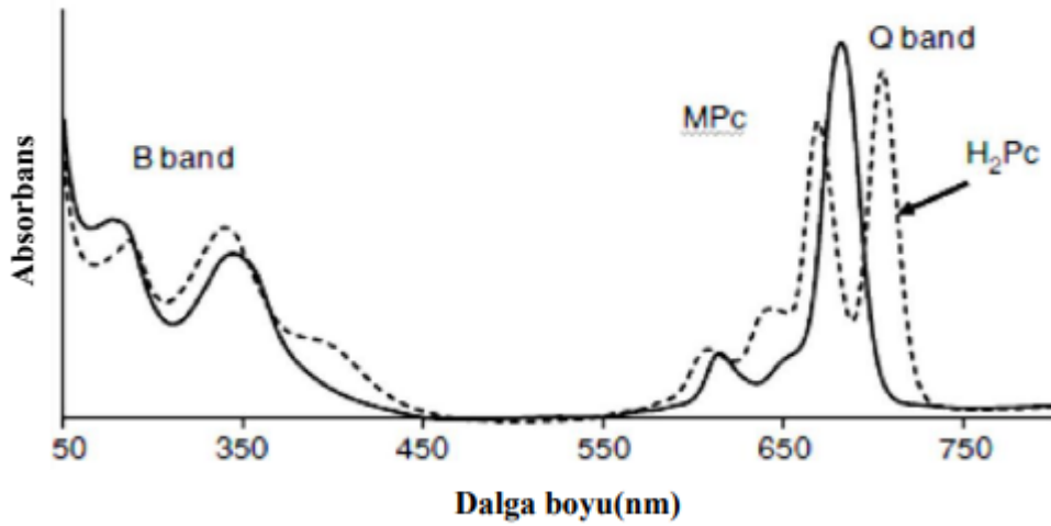
Şekil 2.4. MPc ve H 2 Pc bileşiklerine ait UV-Vis spektrumları [50]
