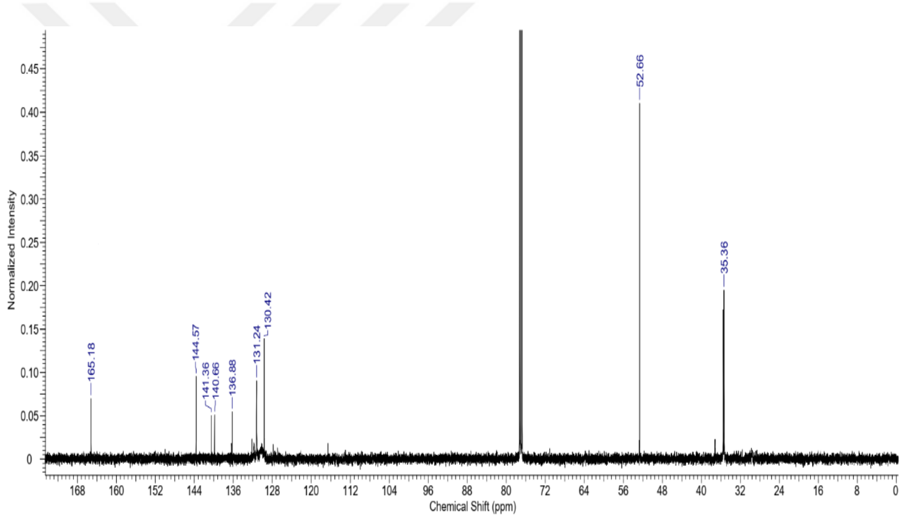
Şekil A.12. Metil 3,4-dibromobenzoat (N2) bileşiğine ait \text{CDCl}_3 içinde alınmış ^{13}\text{C} -NMR spektrumu
