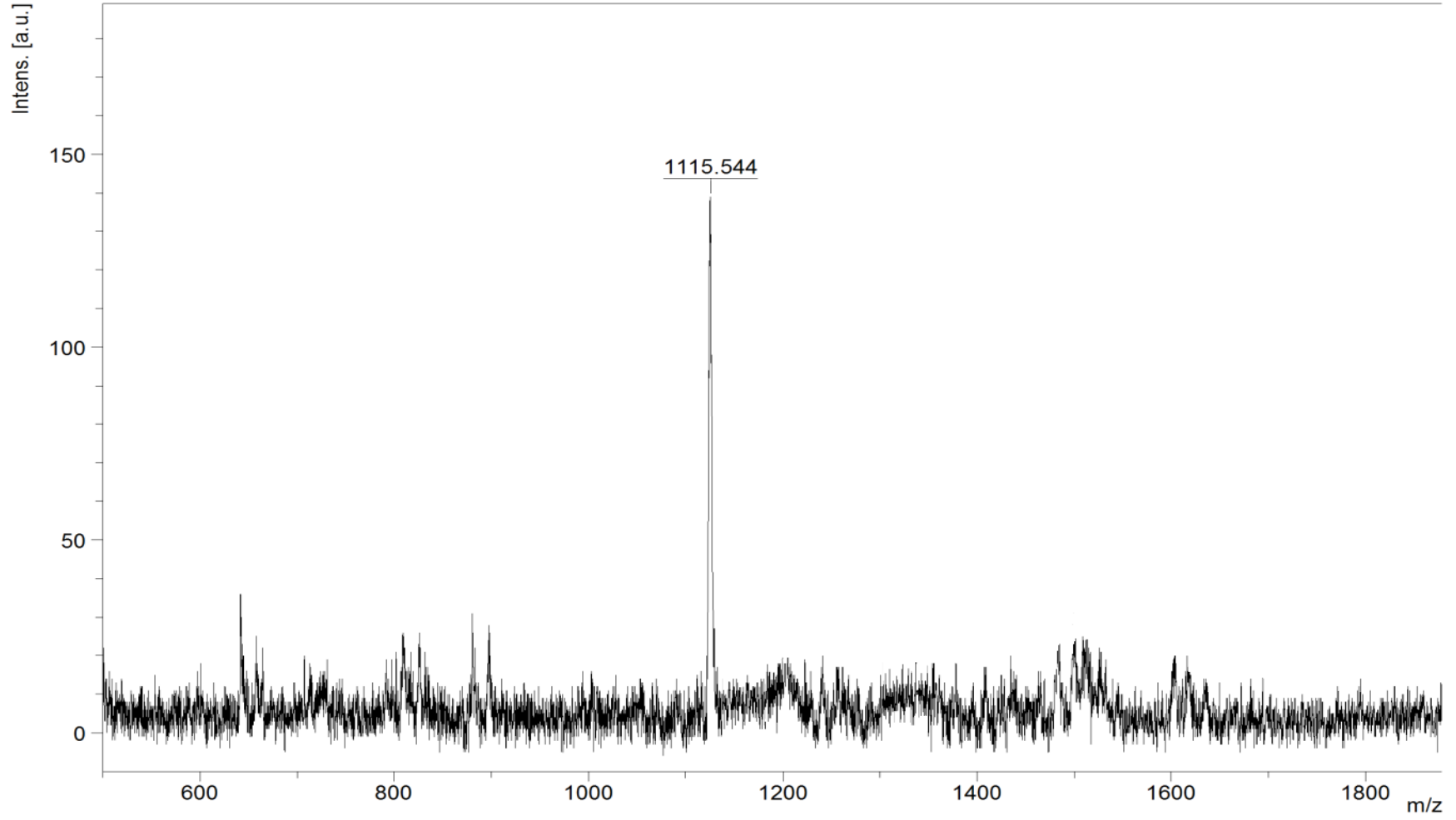
Şekil A.32. TiOPc8 bileşiğine ait MALDI-TOF kütle spektrumu (Matrix: DIT).
