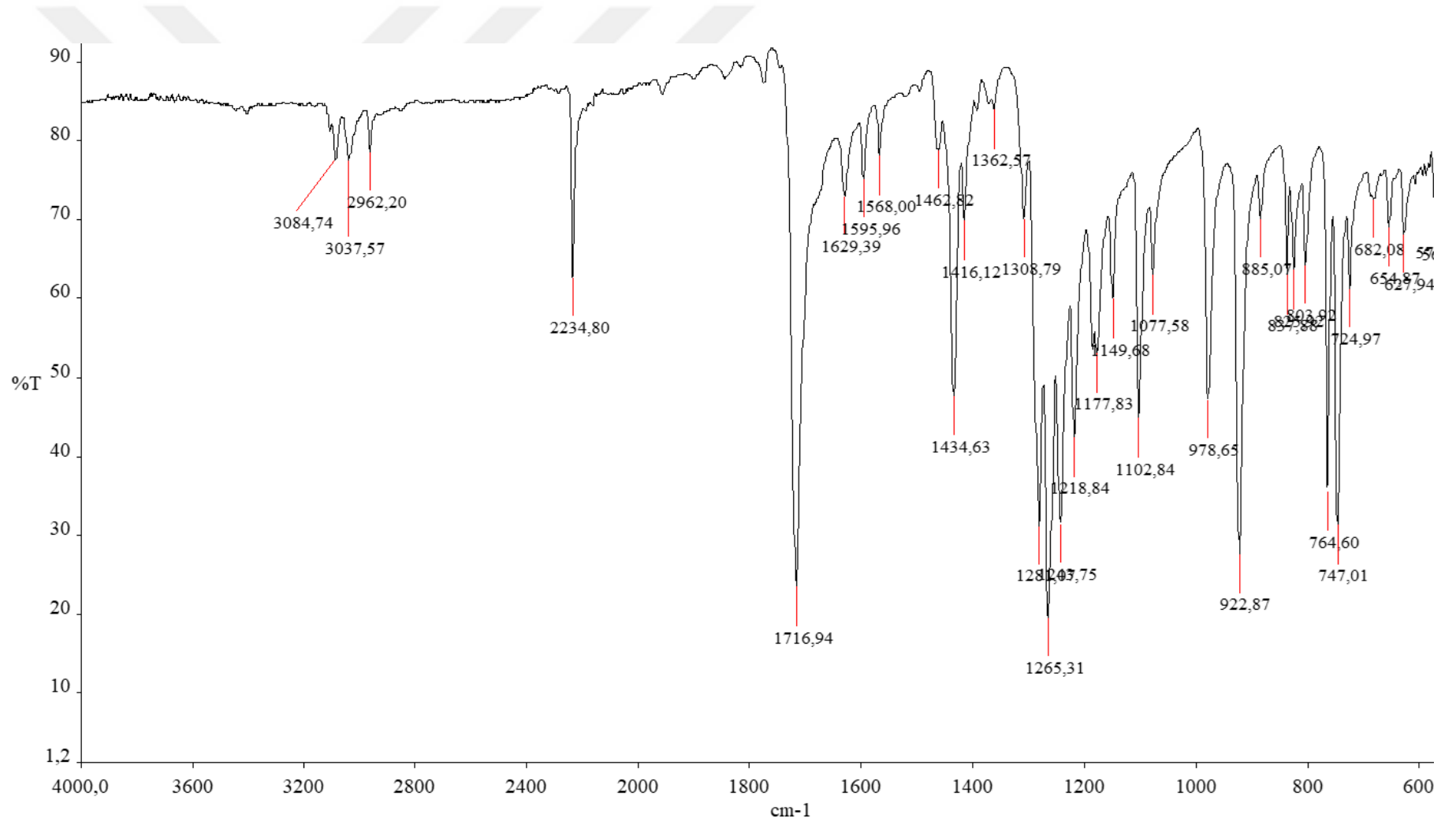
Şekil A.13. 6-Karboksimetil-2,3-disiyanonaftalen ( N3 ) bileşiğine ait FTIR spektrumu
