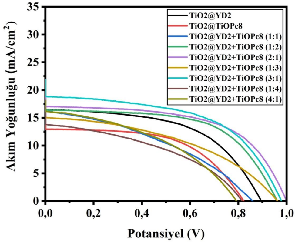
Şekil 4.34. \text{TiO}_2@\text{YD2} , \text{TiO}_2@\text{TiOPc8} ve \text{TiO}_2@\text{YD2}+\text{TiOPc8} fotoanotlarına ait J-V eğrileri
