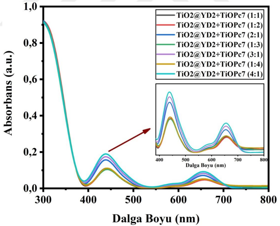
Şekil 4.28. \text{TiO}_2@\text{YD2}+\text{TiOPc7} fotoanotlarına ait UV-Vis spektrumları
