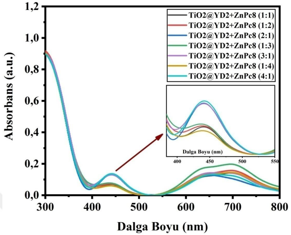
Şekil 4.27. \text{TiO}_2@\text{YD2}+\text{ZnPc8} fotoanotlarına ait UV-Vis spektrumları
