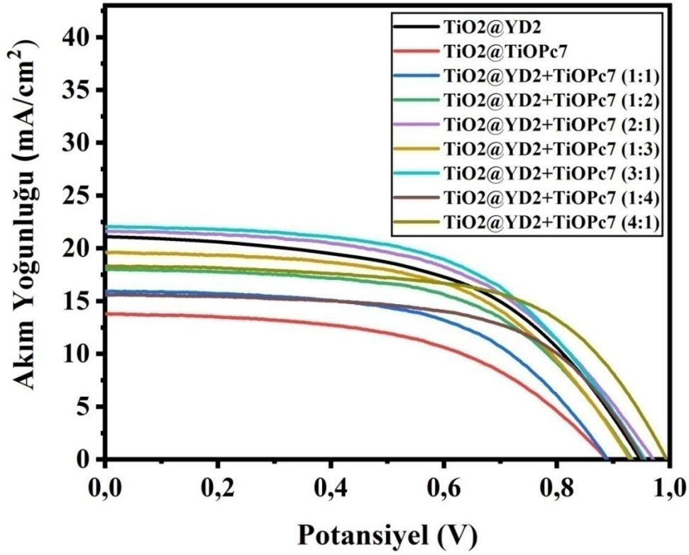
Şekil 4.33. \text{TiO}_2@\text{YD2} , \text{TiO}_2@\text{TiOPc7} ve \text{TiO}_2@\text{YD2}+\text{TiOPc7} fotoanotlarına ait J-V eğrileri
