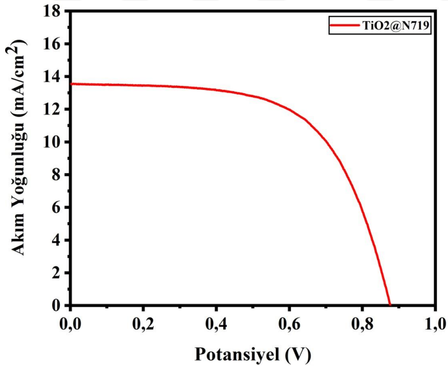
Şekil 4.35. \text{TiO}_2@\text{N719} fotoanotuna ait J-V eğrileri
