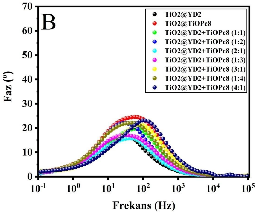
Şekil 4.39. \text{TiO}_2@\text{YD}_2 , \text{TiO}_2@\text{TiOPc8} ve \text{TiO}_2@\text{YD}_2+\text{TiOPc8} fotoanotlarına ait A)Nyquist B)Bode eğrileri
