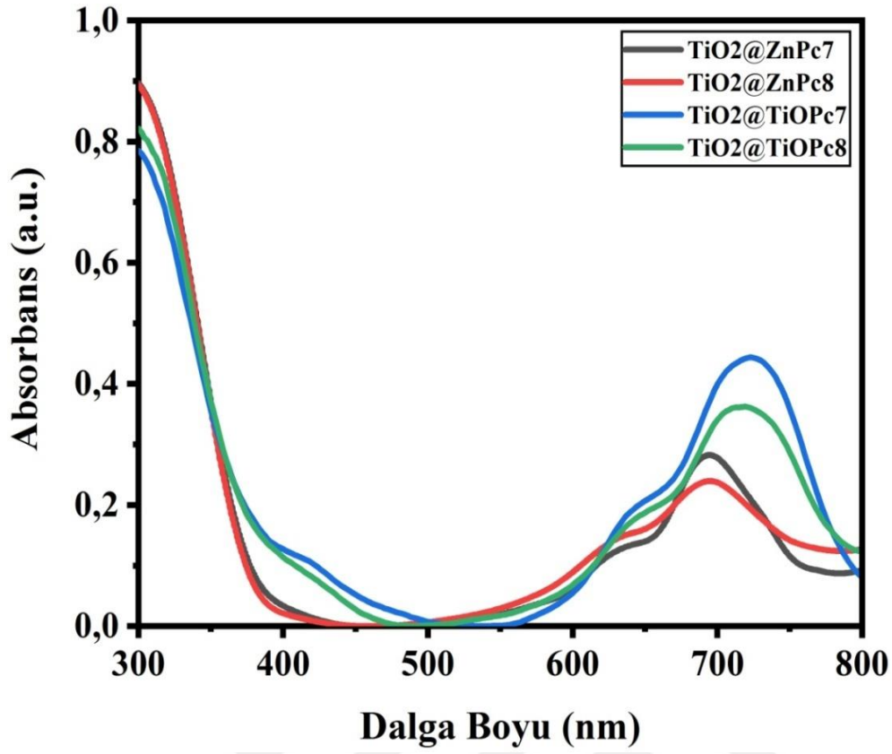
Şekil 4.25. \text{TiO}_2@\text{ZnPc7-8} ve \text{TiO}_2@\text{TiOPc7-8} fotoanotlarına ait UV-Vis spekturumları
