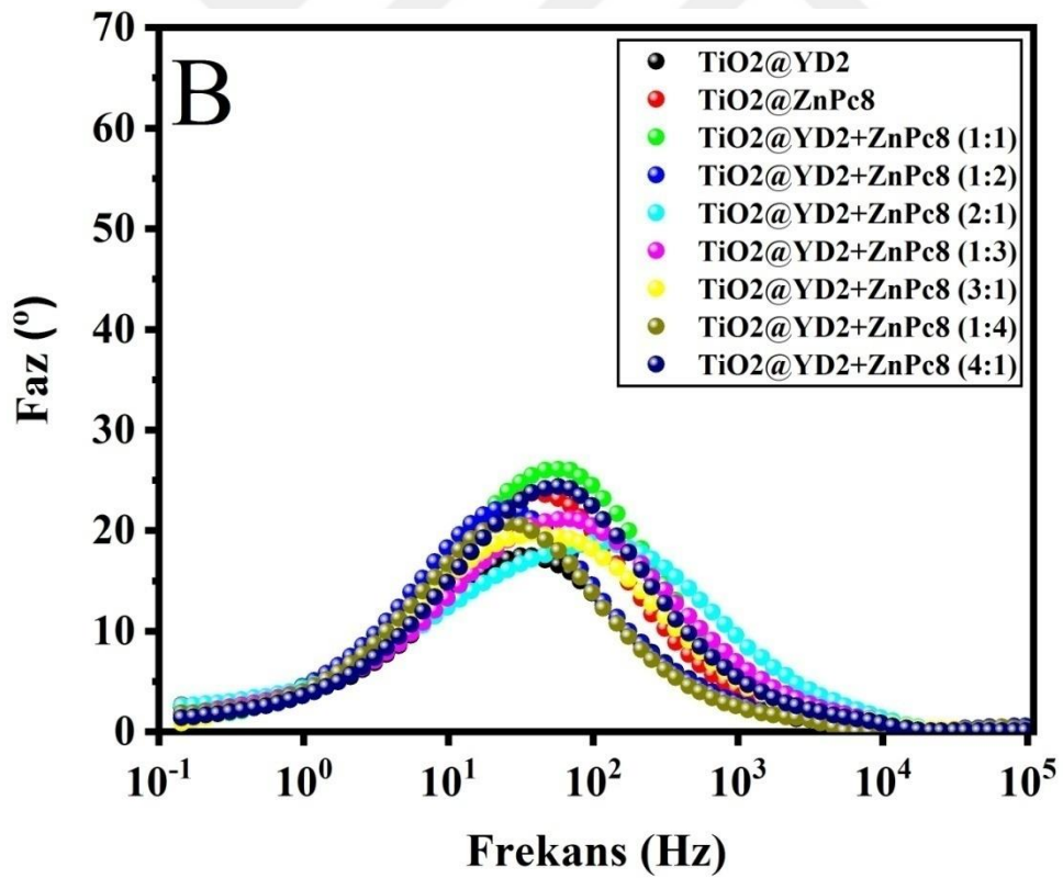
Şekil 4.37. \text{TiO}_2@\text{YD}_2 , \text{TiO}_2@\text{ZnPc}8 ve \text{TiO}_2@\text{YD}_2+\text{ZnPc}8 fotoanotlarına ait A)Nyquist B)Bode eğrileri
