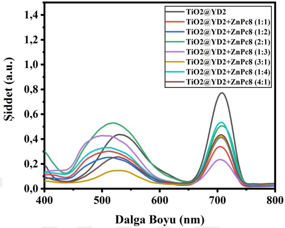
Şekil 4.16. TiO 2 @YD 2 , TiO 2 @ZnPc 8 fotoanotlarına ait PL emisyon spektrumları
