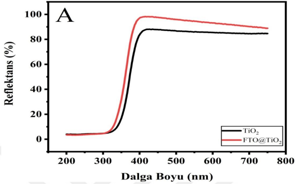
Şekil 4.11. Sentezlenen \text{TiO}_2 nanopartiküllerinin ve \text{FTO@TiO}_2 fotoanotunun DRS spekturumları
