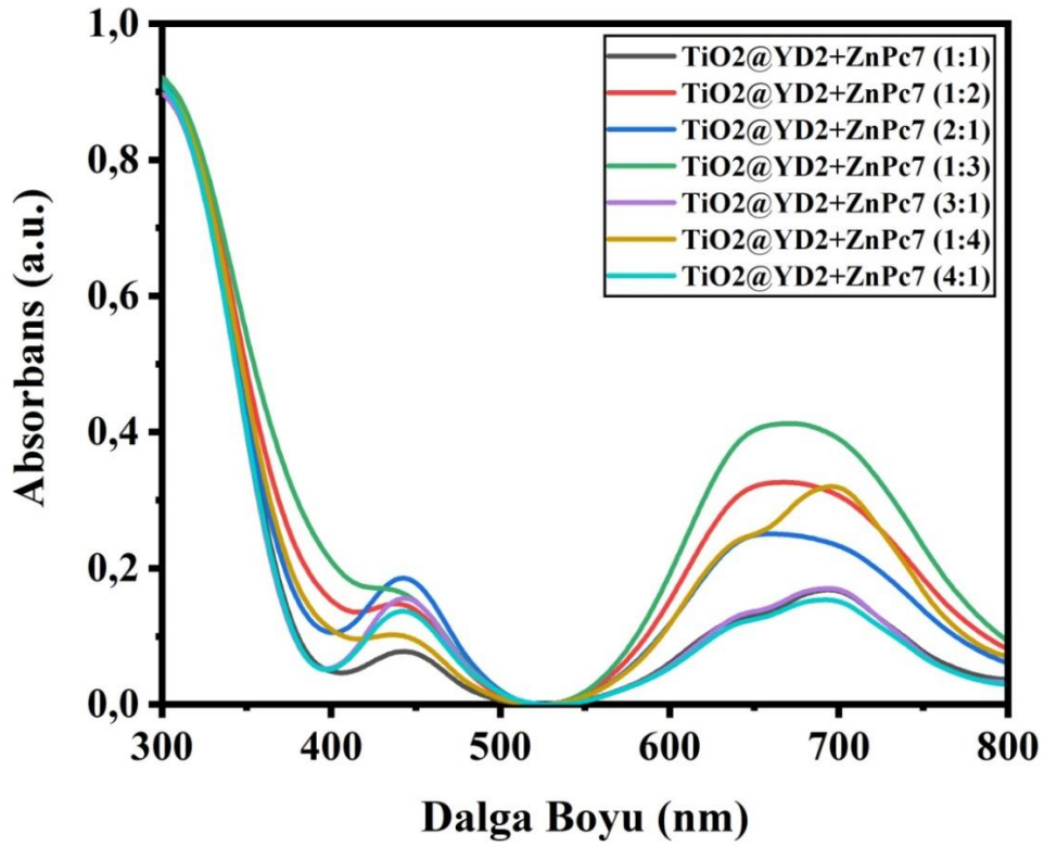
Şekil 4.26. \text{TiO}_2@\text{YD2+ZnPc7} fotoanotlarına ait UV-Vis spekturumları
