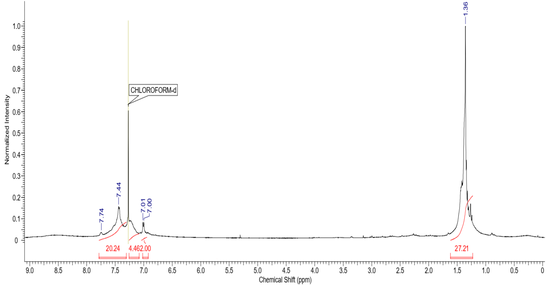
Şekil A.21. ZnPc8 bileşiğine ait CDCl 3 içinde alınmış 1 H-NMR spektrumu.
