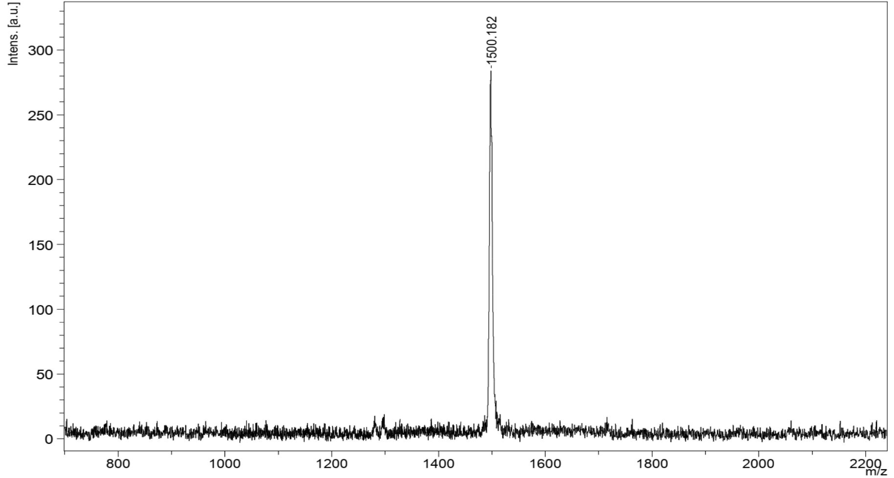
Şekil A.19. ZnPc7 bileşiğine ait MALDI-TOF kütle spektrumu (Matrix: DIT)
