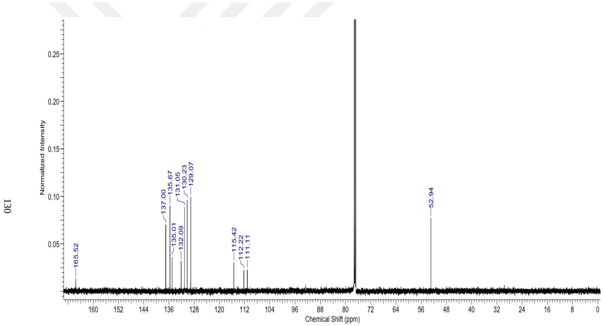
Şekil A.15. 6-Karboksimetil-2,3-disiyanonaftalen (N3) bileşiğine ait CDCl 3 içinde alınmış 13 C-NMR spektrumu
