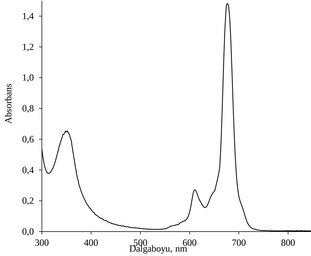
Şekil A.18. ZnPc7 bileşiğine ait THF çözücüsünde alınan UV-Vis spektrumu
