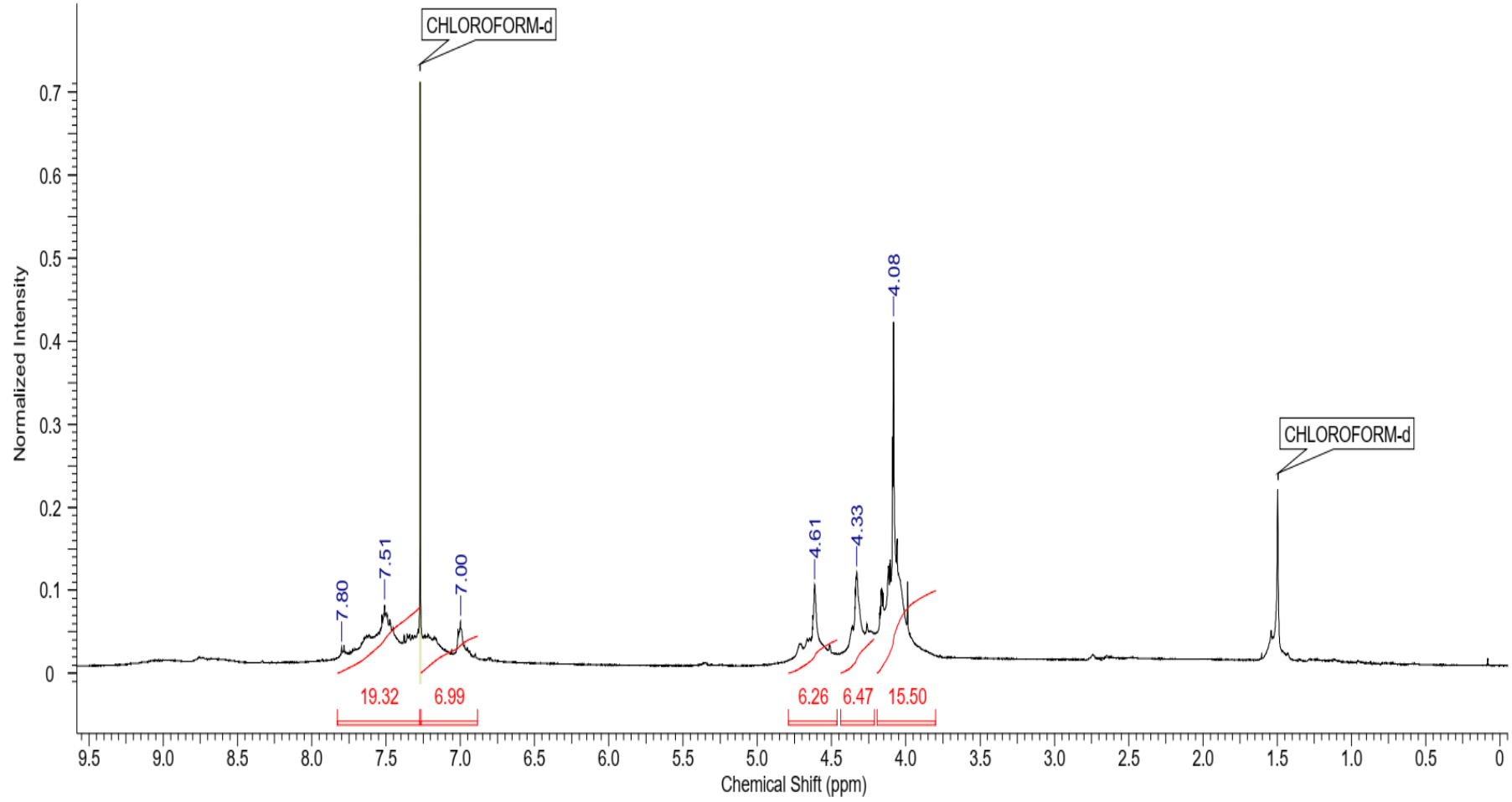
Şekil A.17. ZnPc7 bileşiğine ait CDCl 3 içinde alınmış 1 H-NMR spektrumu
