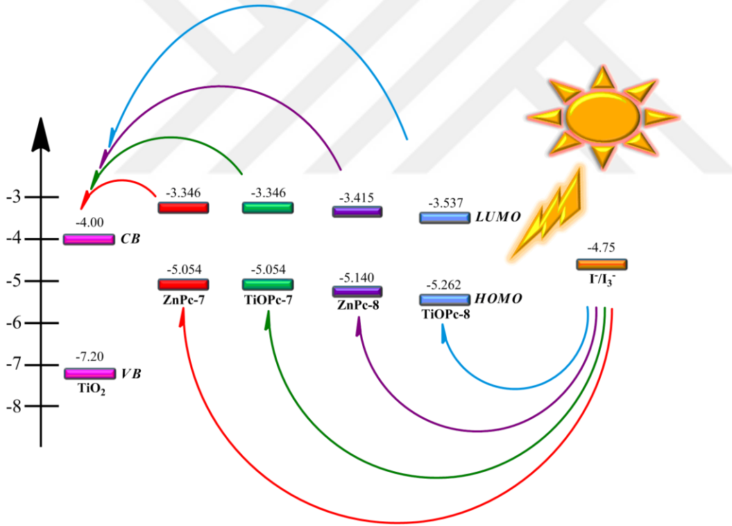
Şekil 4.2. ZnPc7-8 ile TiOPc7-8 boyaların HOMO-LUMO enerji düzeyleri
