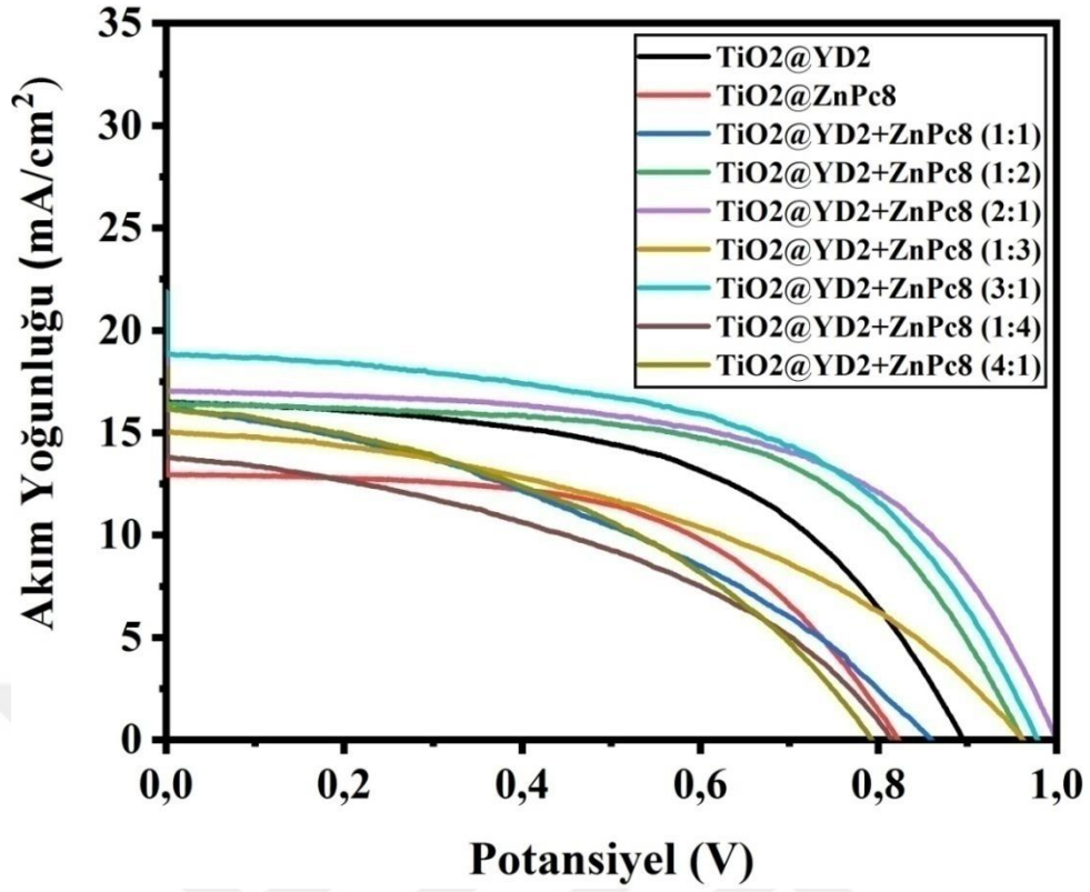
Şekil 4.32. \text{TiO}_2@\text{YD2} , \text{TiO}_2@\text{ZnPc8} ve \text{TiO}_2@\text{YD2}+\text{ZnPc8} fotoanotlarına ait J-V eğrileri
