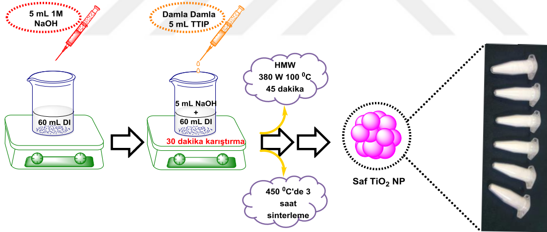
Şekil 3.2. Güneş pillerinde kullanılan \text{TiO}_2 nanopartiküllerin sentez aşamaları.
