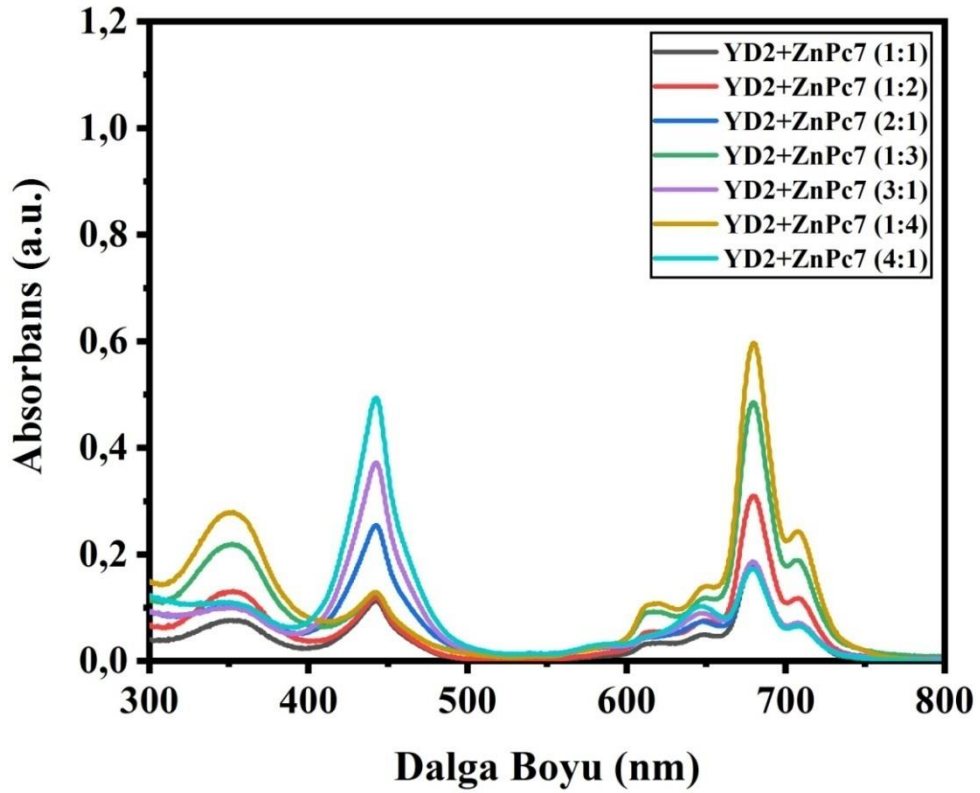
Şekil 4.20. YD2+ZnPc7 kokteyl boyaların UV-Vis spekturumları
