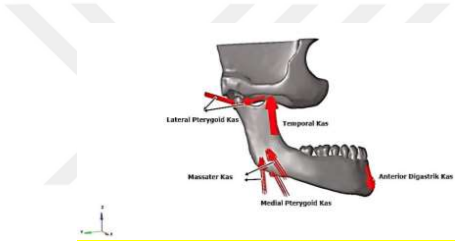
Şekil 5. Yükleme Senaryosu: Modelimizde kasların uygulanma doğrultuları
