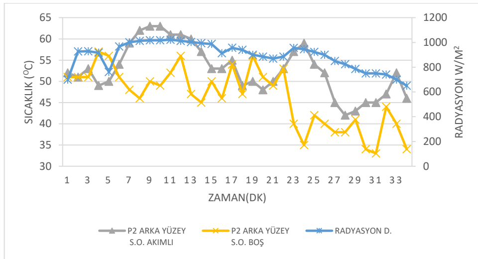
Şekil 7.5. Modül-2 sıcaklık karşılaştırılması
