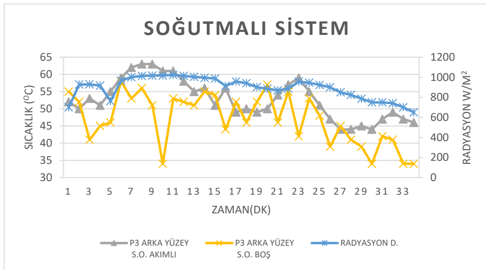
Şekil 7.6. Modül-3 sıcaklık karşılaştırılması
