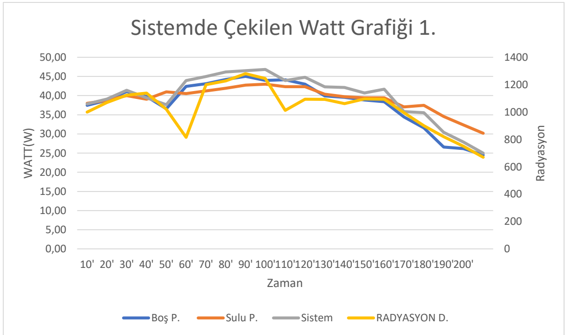
Şekil 10.7. Soğutma sistemin güç grafiği 2. gün
