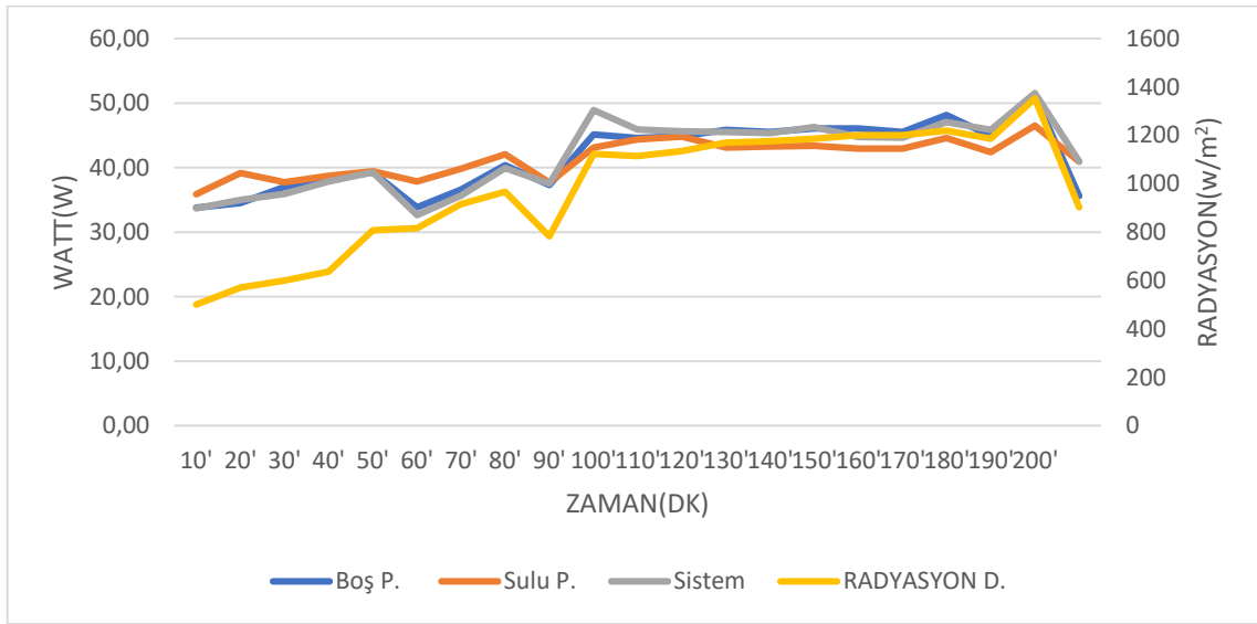
Şekil 7.11. Panellerden çekilen watt grafiği
