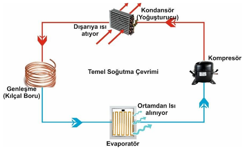
Şekil 4.22. Temel soğutma çevrimi ve deney sisteminde kullanımı
