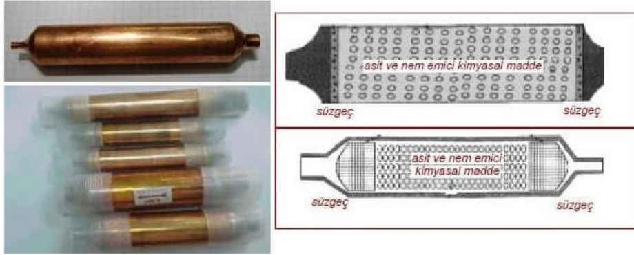
Şekil 4.10. Filtre görünümü ve kesiti ( https://www.thesisat.org/drayer-filtre-montaji.html )
