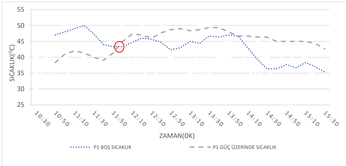
Şekil 7.17.Modül-1(P1) sıcaklık karşılaştırılması
