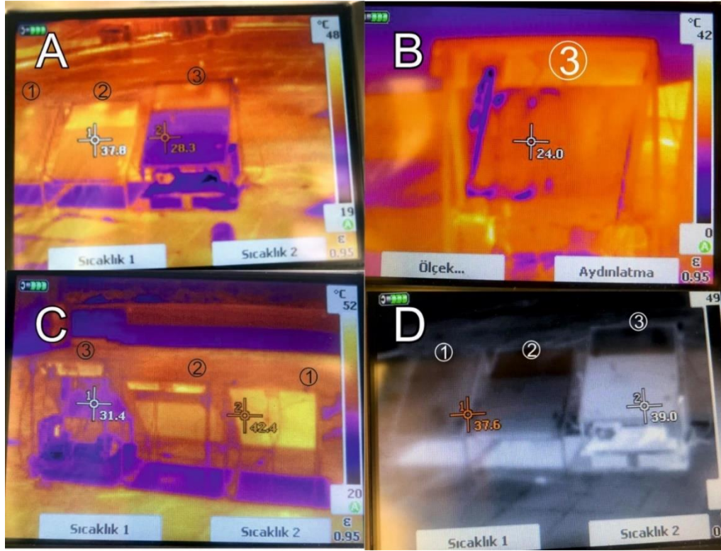
Şekil 7.16. Termal kamera ile soğutulan panellerin görüntüsü
