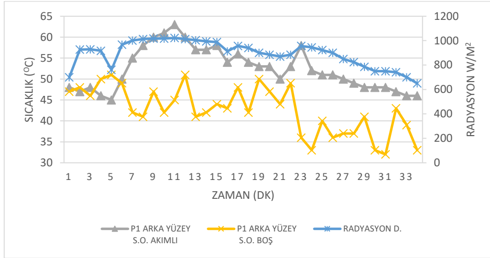
Şekil 7.4. Modül-1 sıcaklık karşılaştırılması
