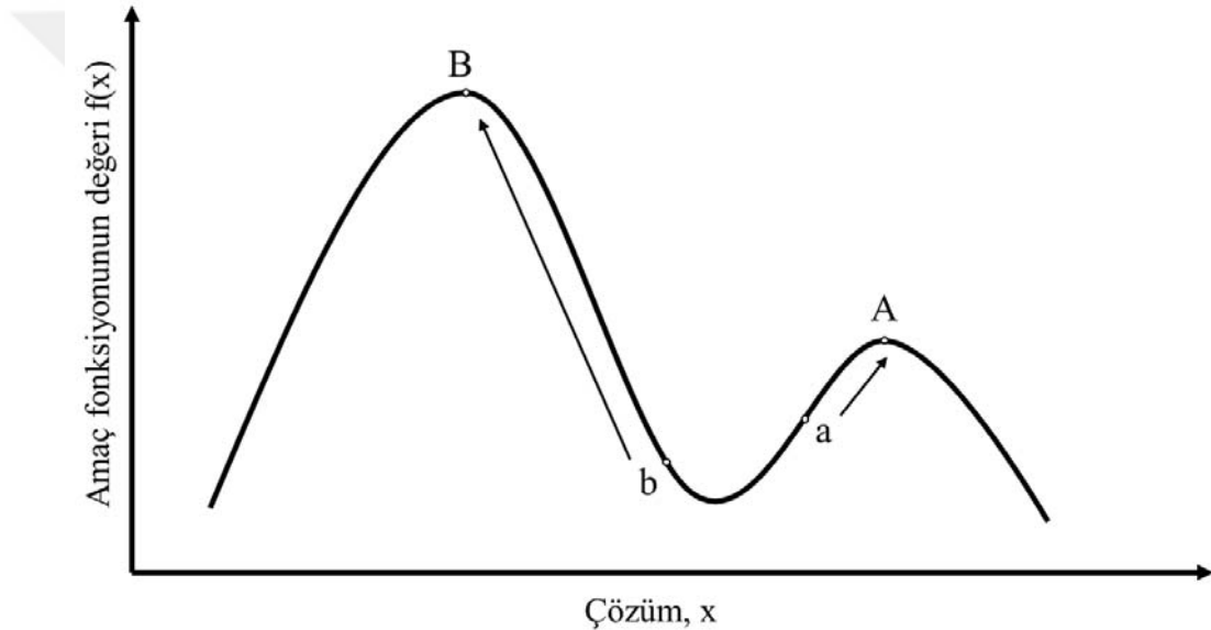
Şekil 3.3. Global optimum ve yerel optimum noktalar.
