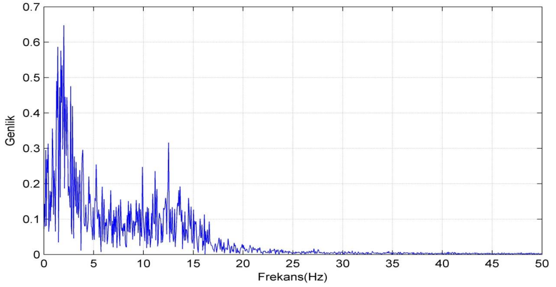
Şekil 3.27. Sprott sisteminin frekans spektrumu
