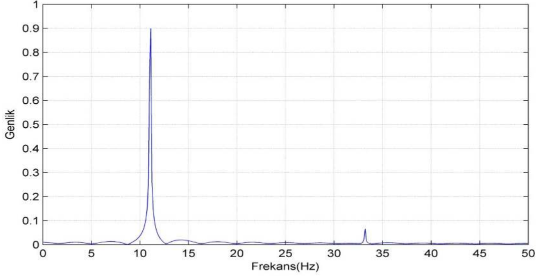
Şekil 3.10. q = 0.7 için kesir dereceli Van der Pol osilatörünün frekans spektrumu
