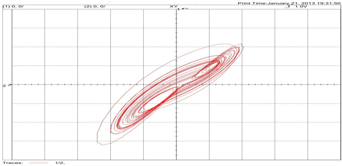
Şekil 3.24. KD Lorenz kaotik çekisi (yatay eksen: x :500mV/kare, düşey eksen y :500mV/kare)
