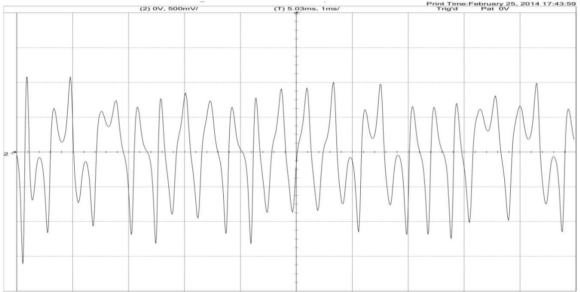
Şekil 3.22. y' 'in değişim eğrisi (yatay eksen:Zaman:1 ms/kare düşey eksen y :500mV/kare)
