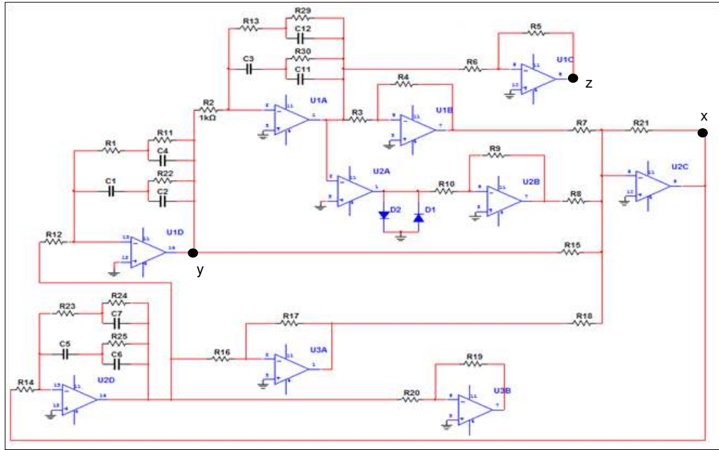
Şekil 3.28. KD Sprott kaotik sisteminin elektronik devre modeli
