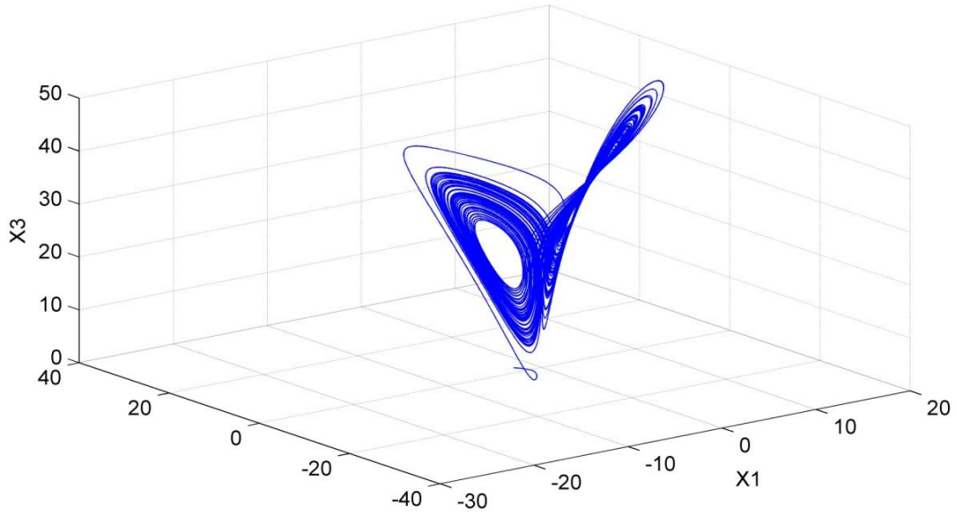
Şekil 3.4. q=0.9 için oluşan kaotik çeki
