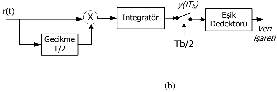
Şekil 5.10. (a) CDSK modülatör, (b) demodülatör
