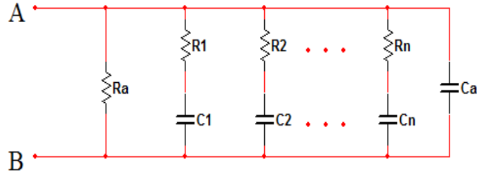
Şekil 2.5. Ľubomír Dorčák v.d. tarafından oluşturulan devre modeli
