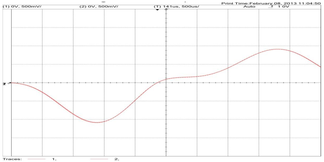
Şekil 3.47. KDPID devre simülasyonundan elde edilen çıkış değişimleri (yatay eksen:Zaman 500 \mu s/kare, düşey eksenler x_1 ve x_2 500mV/kare)
