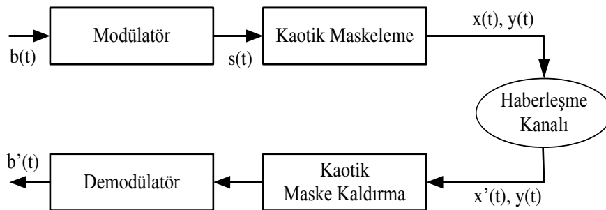
Şekil 5.2. K-PSK yöntemine ait blok diyagramı
