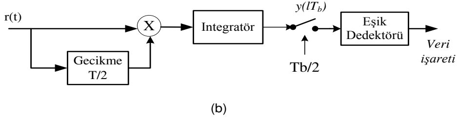
Şekil 5.9. (a) DCSK Modülatör ve (b) demodülatör
