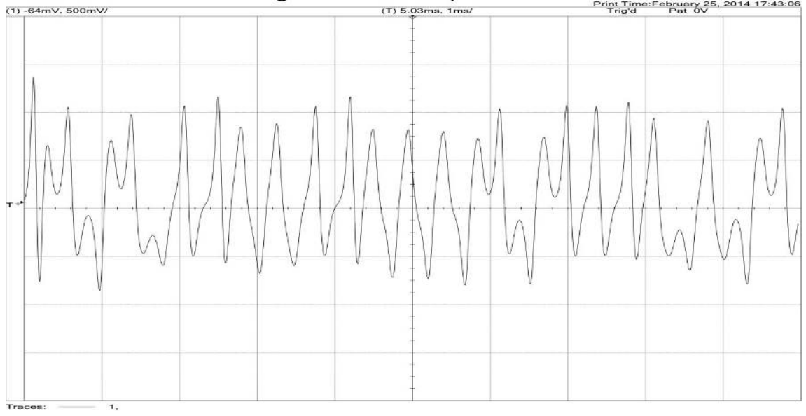
Şekil 3.21. x' 'in değişim eğrisi (yatay eksen:Zaman:1 ms/kare, düşey eksen x :500mV/kare)
