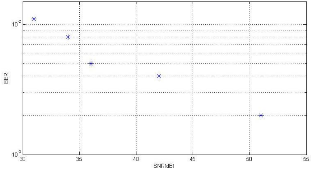
Şekil 5.31. BER grafiği
