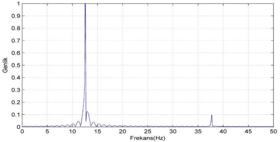
Şekil 3.11. q = 0.8 için kesir dereceli Van der Pol osilatörünün frekans spektrumu
