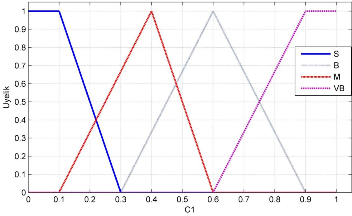
Şekil 4.3. C_1 'ye ait üyelik fonksiyonu
