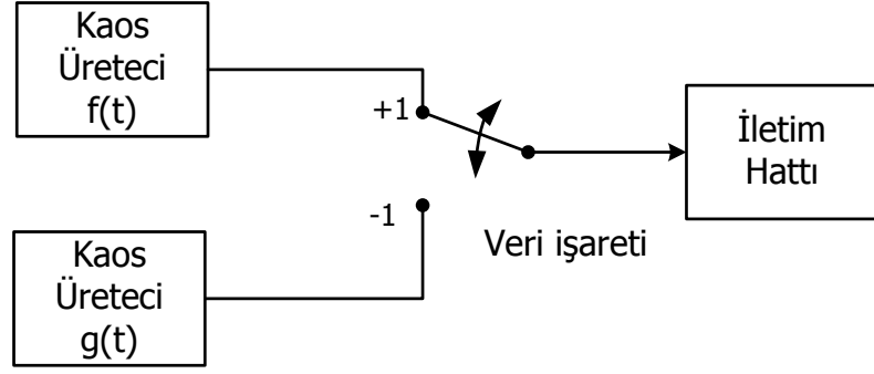
Şekil 5.7. CSK Modülatörüne ait blok diyagramı
