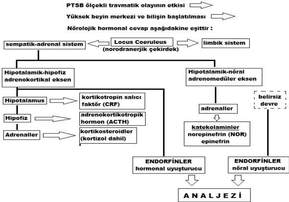
Şekil 3.1 PTSD Stres Tepkisine Dâhil Bazı Kimyasal Maddeler 751
