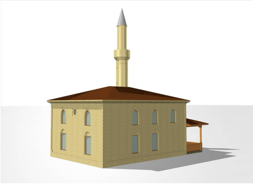
Resim 4.145. Habib Ağa Camii, restitüsyon modeli (1860'lı yıllardaki olası durumu) (M.E.Yılmaz, 2006)
