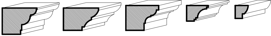
Şekil 6.5. Hacıoğlu Pazarcığı'nda görülen kesme taş saçak silme profilleri
