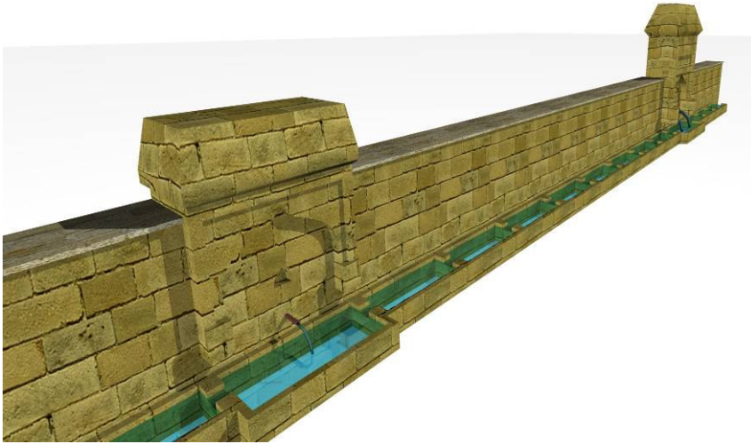
Resim 4.158. Kavarna Çeşmeleri, rölöve modeli (M.E.Yılmaz, 2006)
