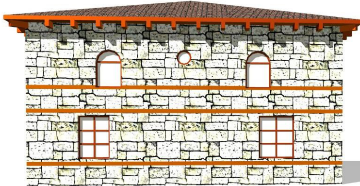
Resim 4.64. İsmail Efendi Camii, restitüsyon modeli (1862'deki olası durumu) (M.E.Yılmaz, 2006)
