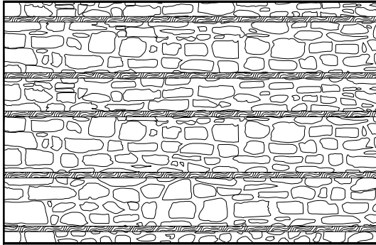
Şekil 6.1. Hacıoğlu Pazarcığı'nda görülen ahşap hatıllı moloz taş duvar örgü
