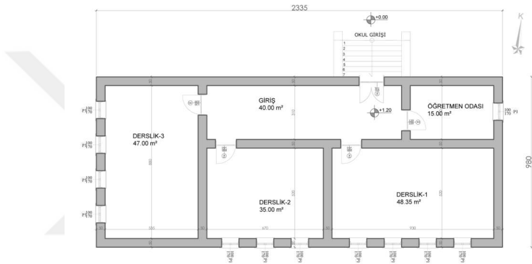
Şekil 6.11.1.7. Alanköy Köyü Okulu Zemin Kat Planı (Yılmaz Özev, 2024)
