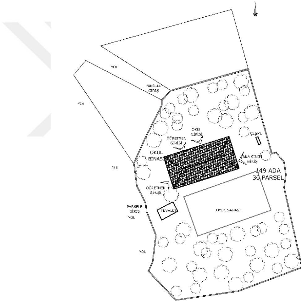
Şekil 6.2.2.3. Bayındır Köyü Okulu Vaziyet Planı (Yılmaz Özev, 2024)
