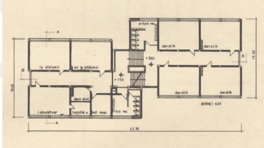
Şekil 6.1.8.15. Ortaokul/ Lise Tip Proje 1. Kat Planı (Okan, 1976)
