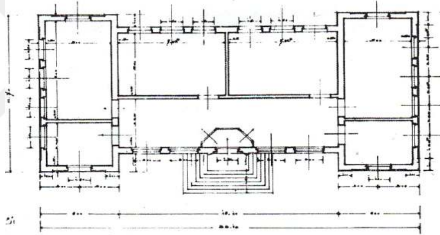
Şekil 5.5. Edirne Karaağaç Mektebi Planı (Yavuz, 1981)
