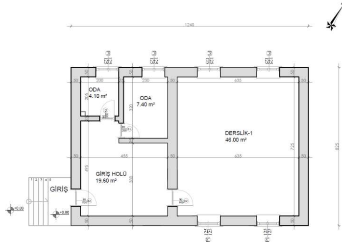
Şekil 6.2.14.5. Kuruçay Köyü Okulu Zemin Kat Planı (Yılmaz Özev, 2024)
