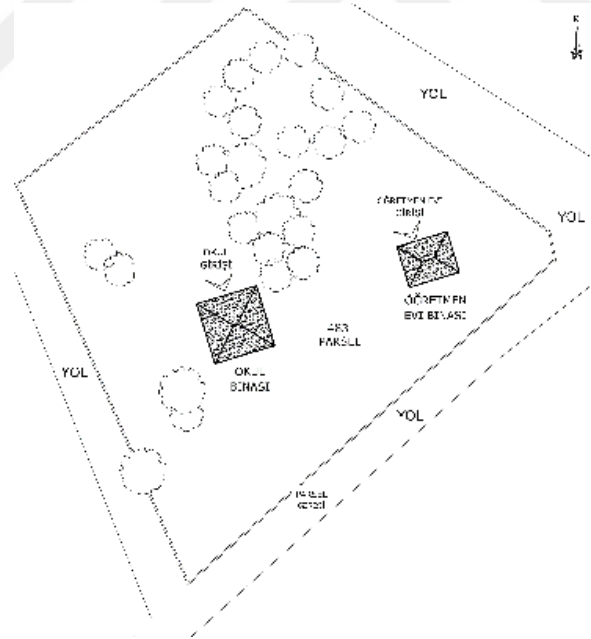
Şekil 6.11.3.3. Bayırbaşı Köyü Okulu Vaziyet Planı (Yılmaz Özev, 2024)
