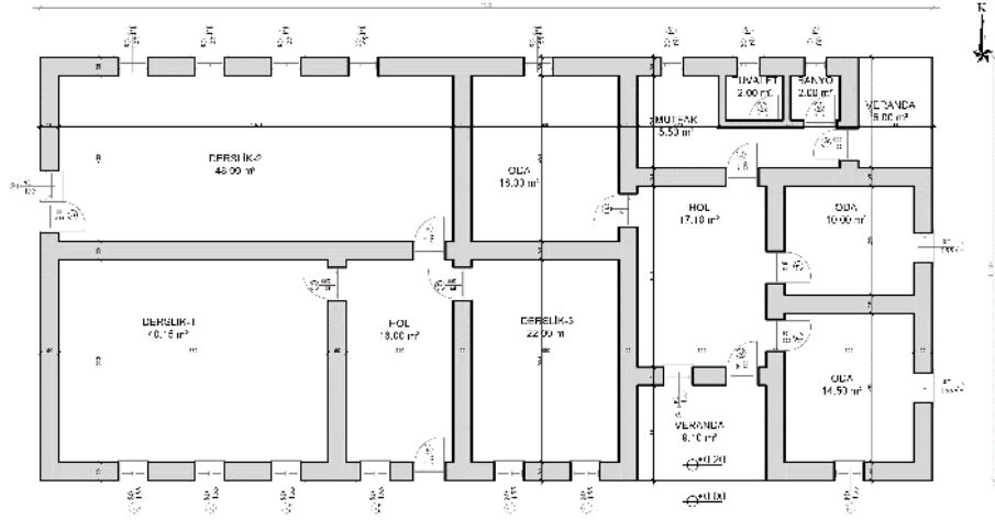
Şekil 6.6.2.12. Çebiş Köyü İkinci Okulu Zemin Kat Planı (Yılmaz Özev, 2024)
