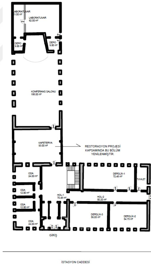
Şekil 6.1.6.8. Kız Sanat Enstitüsü Zemin Kat Planı (Yılmaz Özev, 2022)
