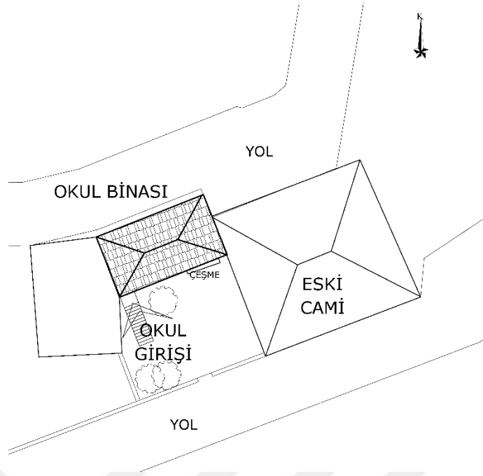
Şekil 6.2.9.2. Halıcılar Köyü Vaziyet Planı (Yılmaz Özev, 2024)
