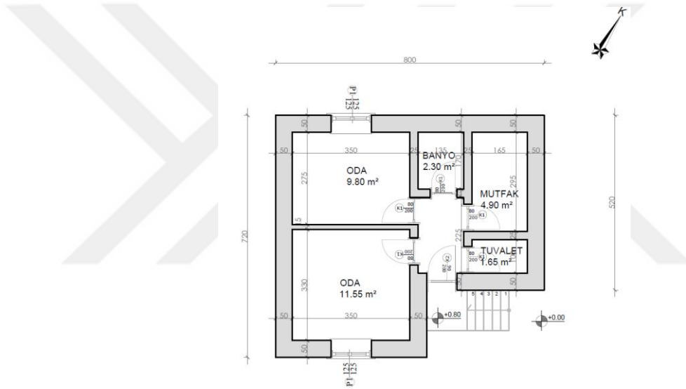
Şekil 6.2.14.15. Kuruçay Köyü Okulu Öğretmen Evi Zemin Kat Planı (Yılmaz Özev, 2024)
