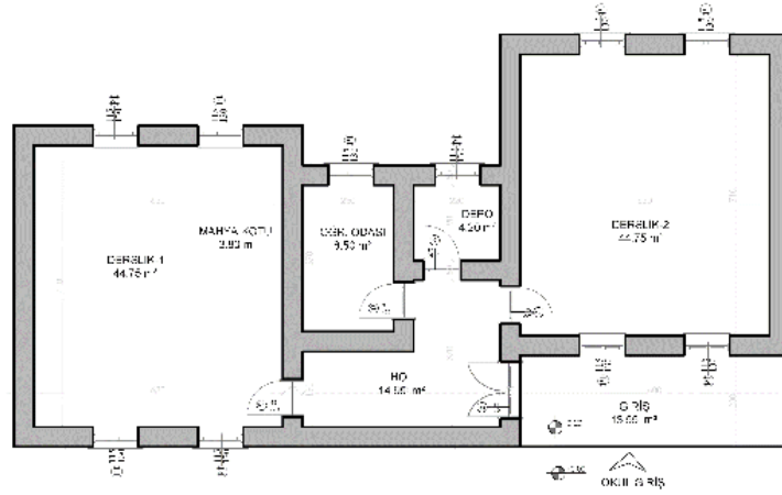
Şekil 6.11.2.5. Yeşilova Bayındır Köyü Okulu Zemin Kat Planı (Yılmaz Özev, 2024)
