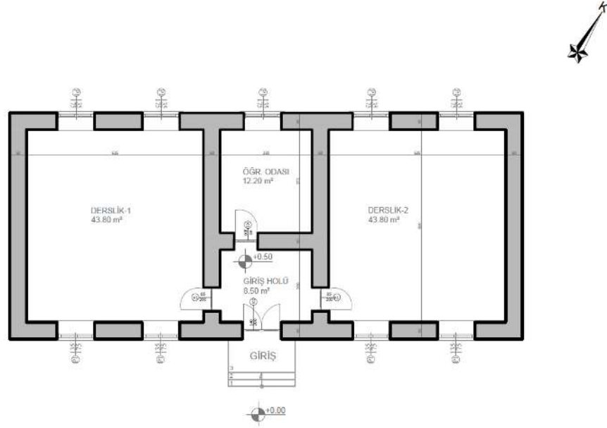
Şekil 6.2.7.4. Cimbilli Köy Okulu Zemin Kat Planı (Yılmaz Özev, 2024)
