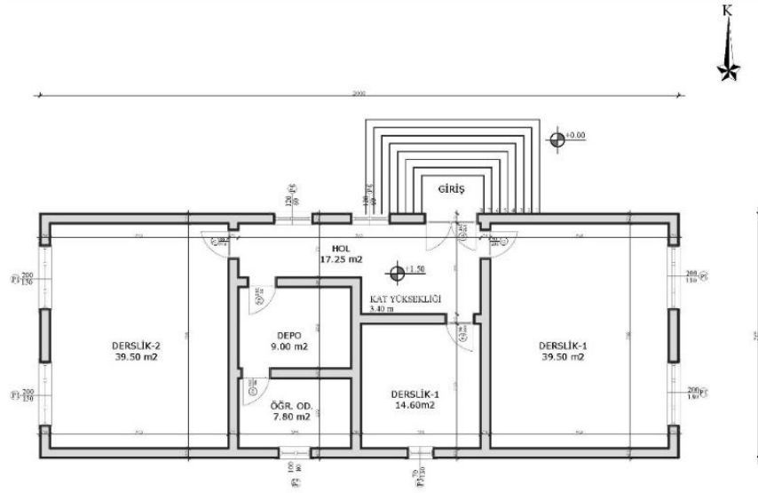
Şekil 6.11.7.4. Karaköy Köyü Okulu Zemin Kat Planı (Yılmaz Özev, 2024)
