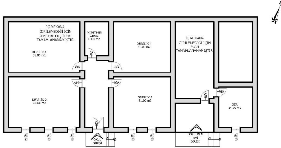
Şekil 6.3.2.4. Yazır Köyü Okulu Zemin Kat Planı (Yılmaz Özev, 2024)
