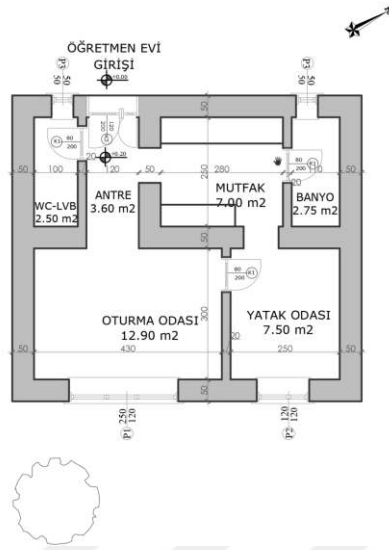
Şekil 6.2.3.9. Bereket Köyü Okulu Öğretmen Evi Zemin Kat Planı (Yılmaz Özev, 2024)
