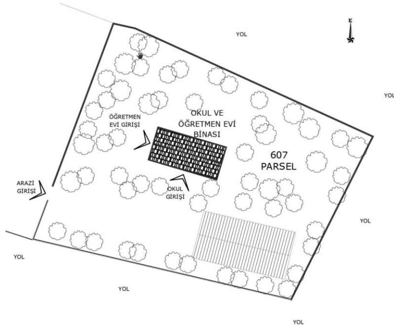
Şekil 6.2.4.3. Beşkavak Köyü Okulu Vaziyet Planı (Yılmaz Özev, 2024)
