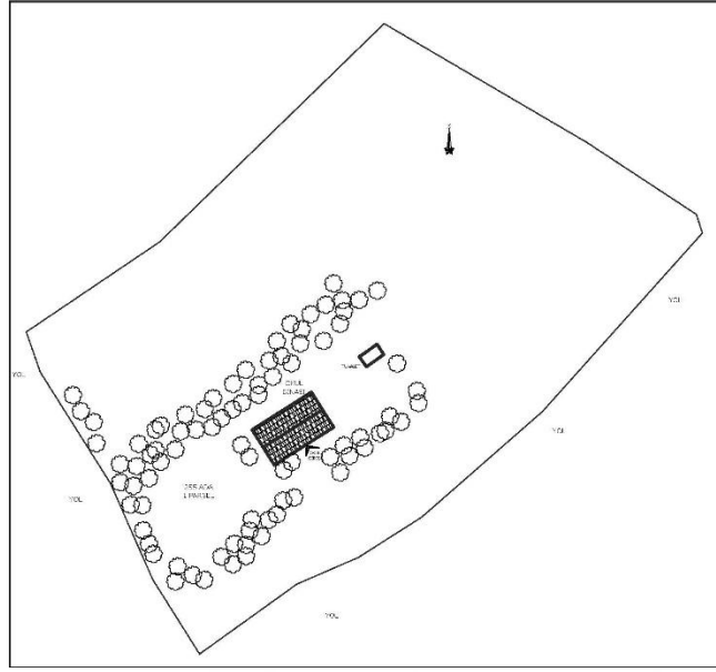
Şekil 6.5.2.3. Büyükalın Köyü Okulu Vaziyet Planı (Yılmaz Özev, 2024)
