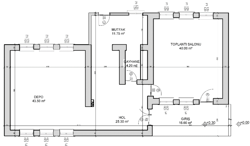
Şekil 6.6.2.8. Çebiş Köyü Birinci Okul Tadilat Sonrası Zemin Kat Planı (Yılmaz Özev, 2024)
