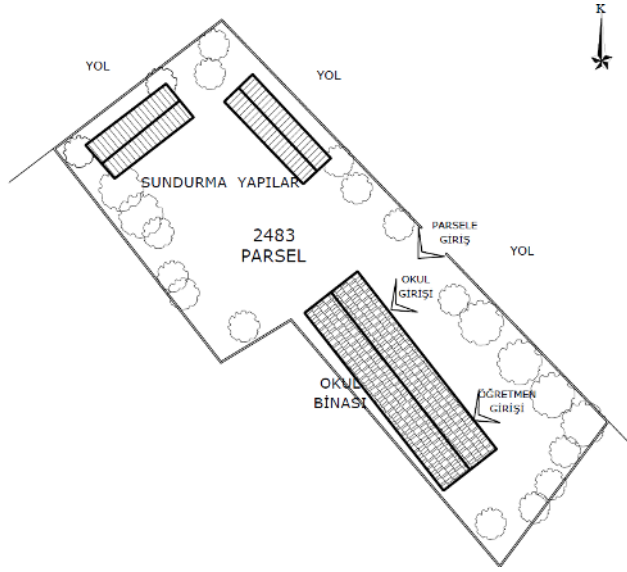
Şekil 6.11.6.3. Işıklar Köyü Okulu Vaziyet Planı (Yılmaz Özev, 2024)
