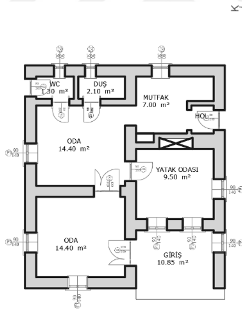
Şekil 6.9.2.28. Elmacık Köyü Okulu Öğretmen Evi Zemin Kat Planı (Yılmaz Özev, 2022)
