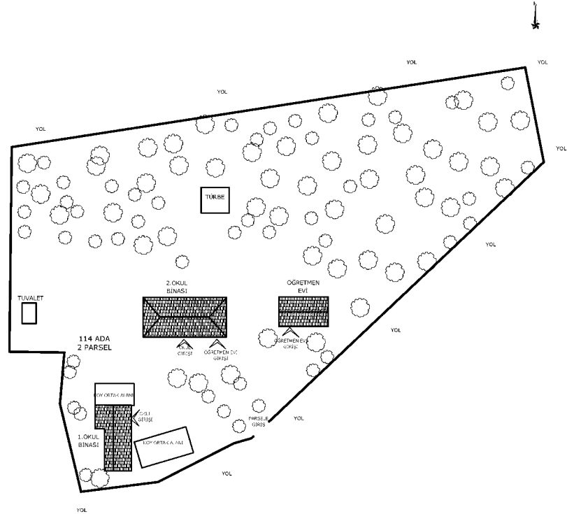
Şekil 6.6.2.3. Çebiş Köyü Okulları Vaziyet Planı (Yılmaz Özev, 2024)
