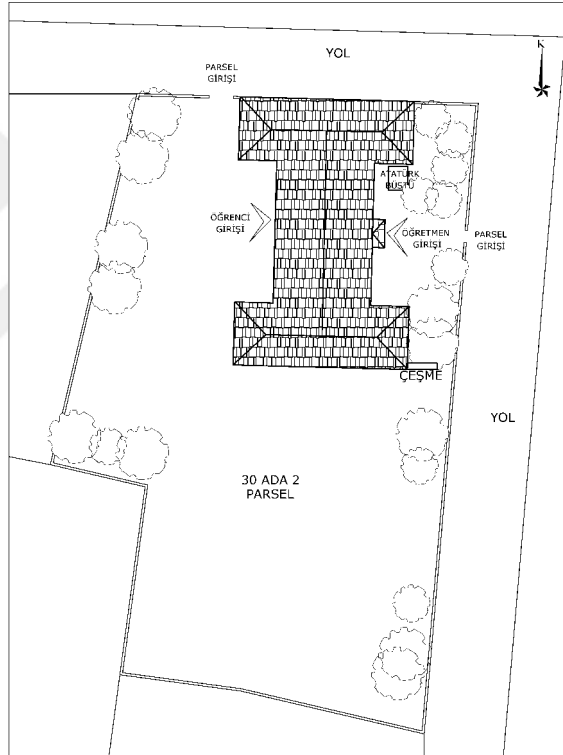
Şekil 6.10.1.3. Namık Kemal Okulu Vaziyet Planı (Yılmaz Özev, 2024)
