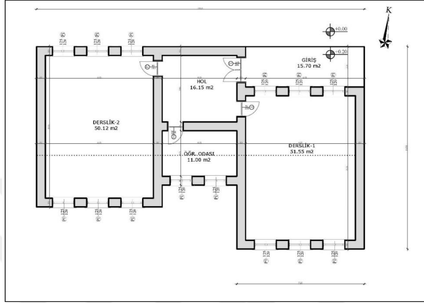
Şekil 6.5.1.4. Kayacık Köyü Okulu Zemin Kat Planı (Yılmaz Özev, 2024)
