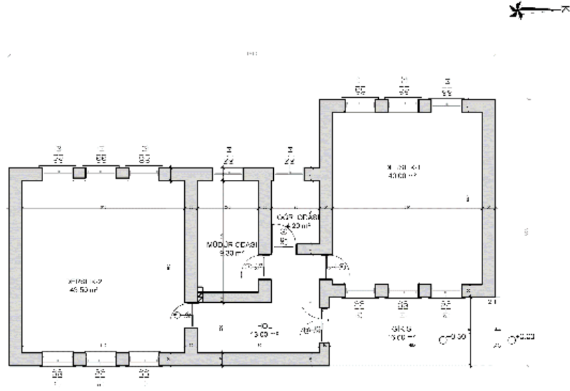
Şekil 6.6.2.7. Çebiş Köyü Birinci Okul Tadilat Öncesi Orijinal Zemin Kat Planı (Yılmaz Özev, 2024)
