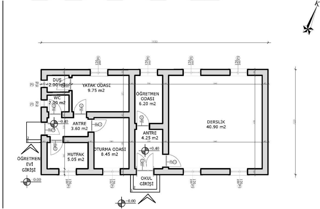
Şekil 6.3.1.4. Çamlıdere Köyü Zemin Kat Planı (Yılmaz Özev, 2024)
