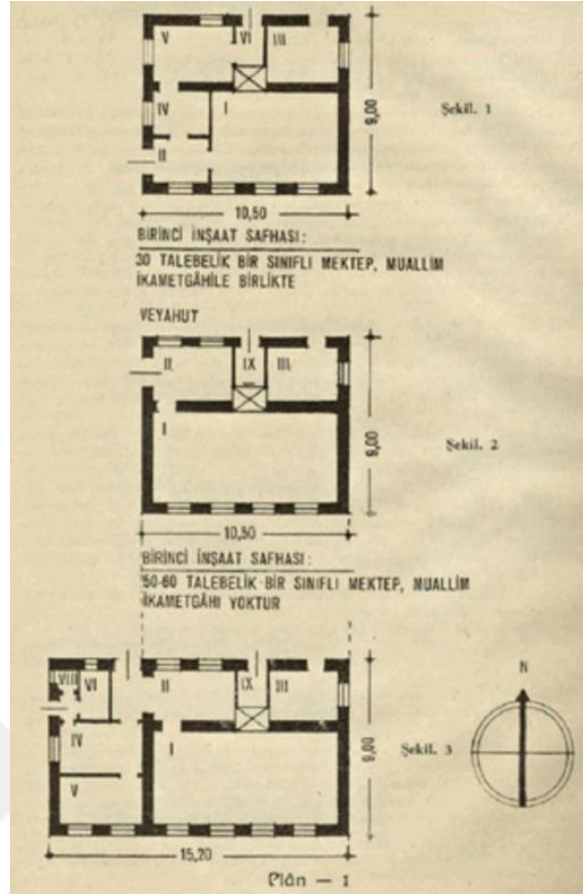
Şekil 5.11. G. Schütte Lihotzky tarafından köylerde inşa edilmesi planlanan farklı büyüklüklerdeki tek derslikli plan örnekleri (Lihotzky, 1939)
