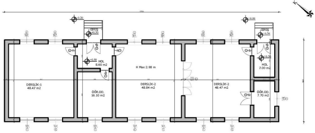
Şekil 6.11.6.4. Işıklar Köyü Okulu Zemin Kat Planı (Yılmaz Özev, 2024)
