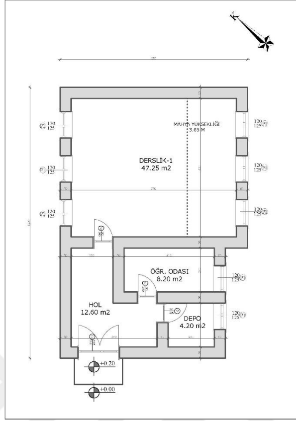
Şekil 6.11.4.4. Çardak Köyü Okulu Zemin Kat Planı (Yılmaz Özev, 2024)
