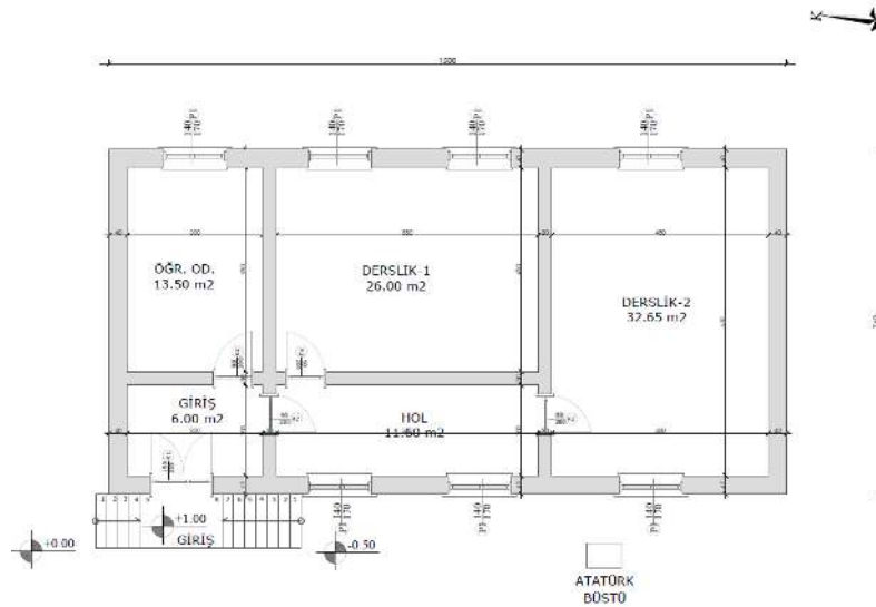
Şekil 6.7.1.4. Kuşdili Köyü Okulu Zemin Kat Planı (Yılmaz Özev, 2024)
