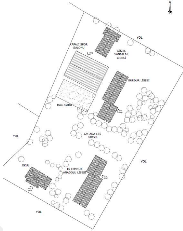
Şekil 6.1.8.12. Burdur Lisesi Vaziyet Planı (Yılmaz Özev, 2025)
