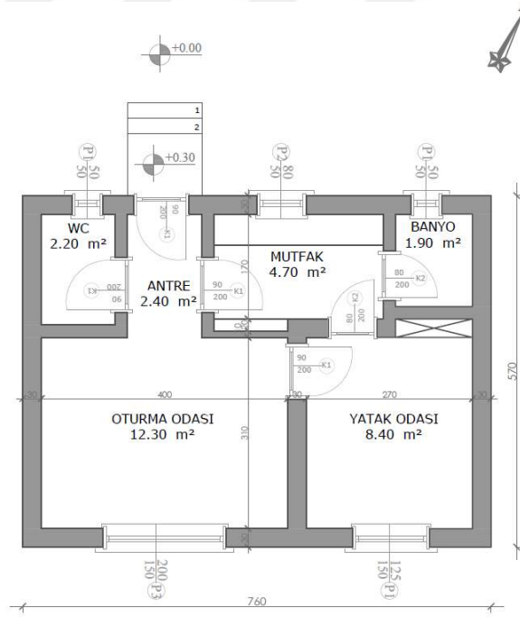
Şekil 6.2.12.15. Karakent Köyü Okulu Öğretmen Evi Zemin Kat Planı (Yılmaz Özev, 2024)
