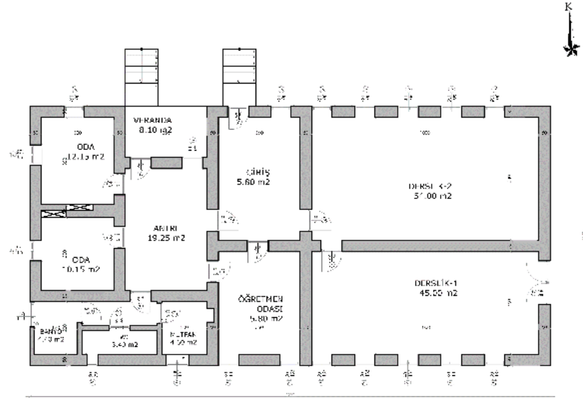
Şekil 6.2.6.4. Bozlar Köyü Zemin Kat Planı (Yılmaz Özev, 2024)
