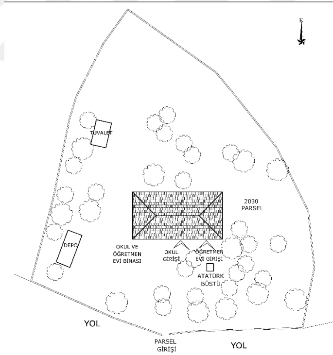
Şekil 6.2.8.3. Günelan Köyü Okulu Vaziyet Planı (Yılmaz Özev, 2024)
