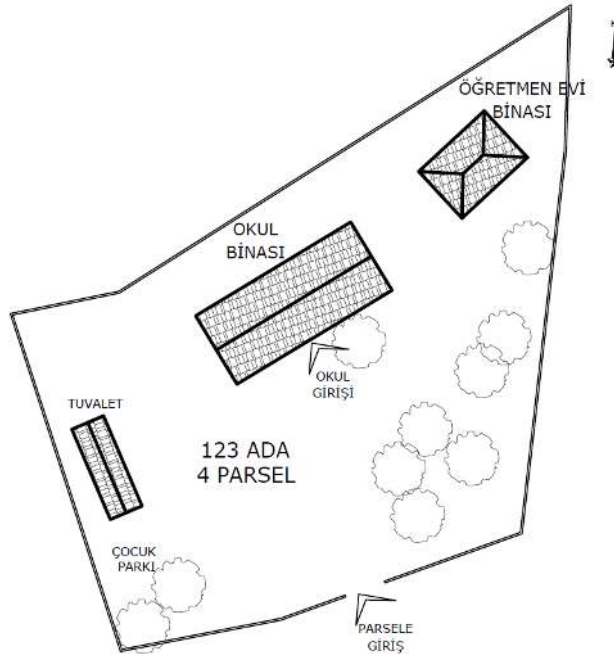
Şekil 6.2.7.3. Cimbilli Köyü Okulu Vaziyet Planı (Yılmaz Özev, 2024)
