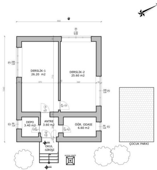
Şekil 6.2.3.4. Bereket Köyü Okulu Zemin Kat Planı (Yılmaz Özev, 2024)
