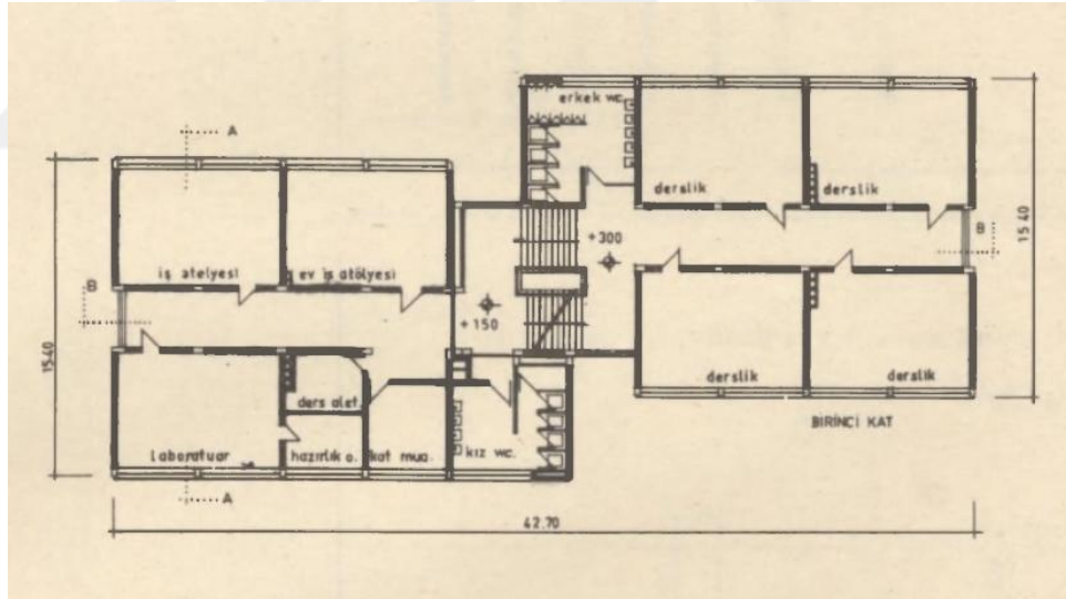
Şekil 5.14. Ortaokul/ Lise Tip Proje 1. Kat Planı (Okan, 1976)
