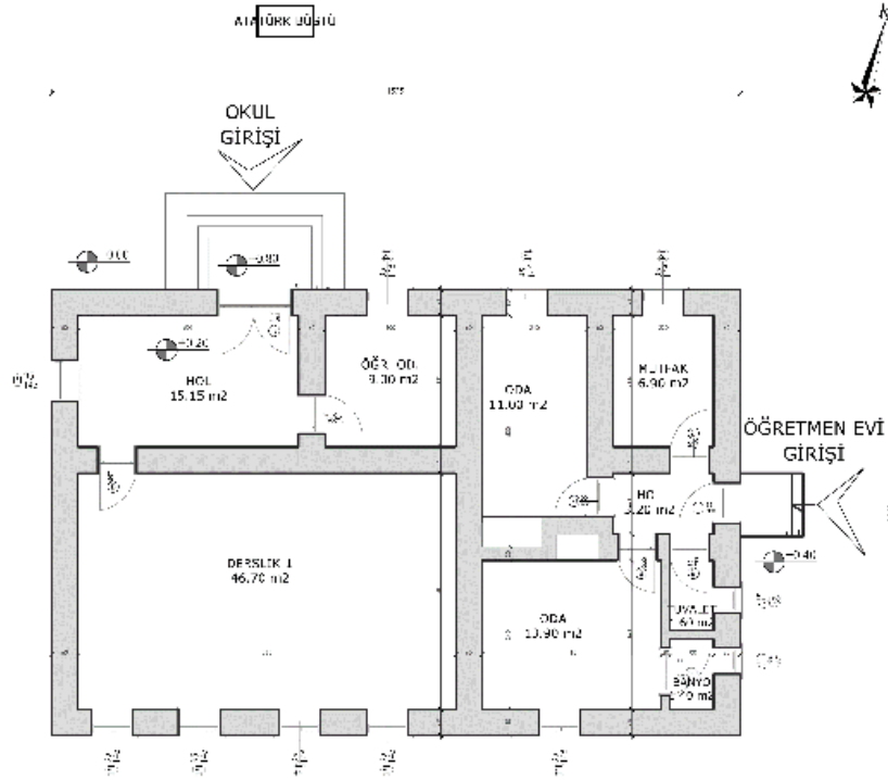
Şekil 6.2.11.6. Karacaören Köyü Okulu Zemin Kat Planı (Yılmaz Özev, 2024)
