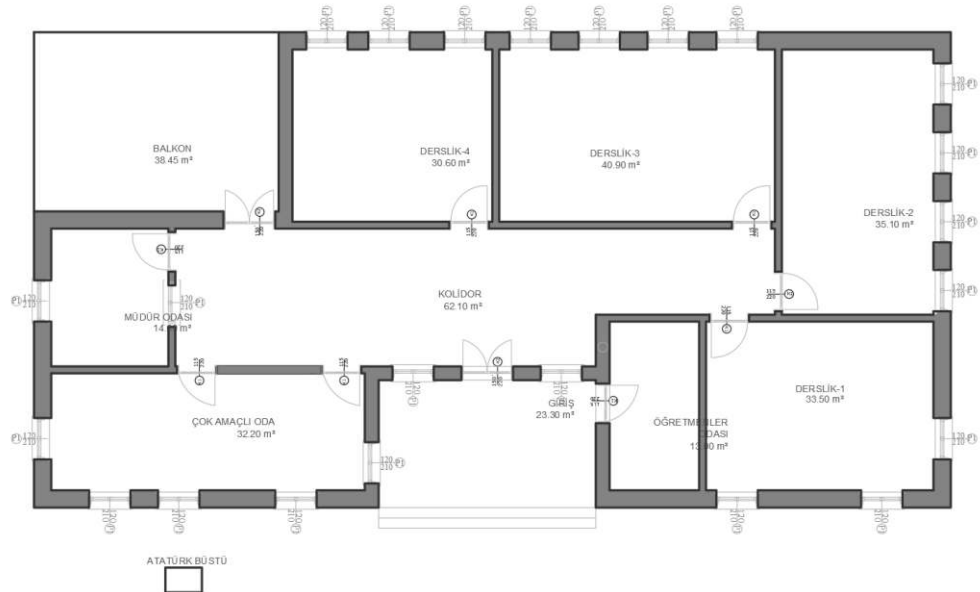
Şekil 6.2.13.4. Kayaaltı Köyü Okulu Zemin Kat Planı (Yılmaz Özev, 2024)
