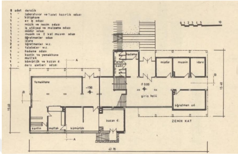
Şekil 5.13. Ortaokul/ Lise Tip Proje Zemin Kat Planı (Okan, 1976)
