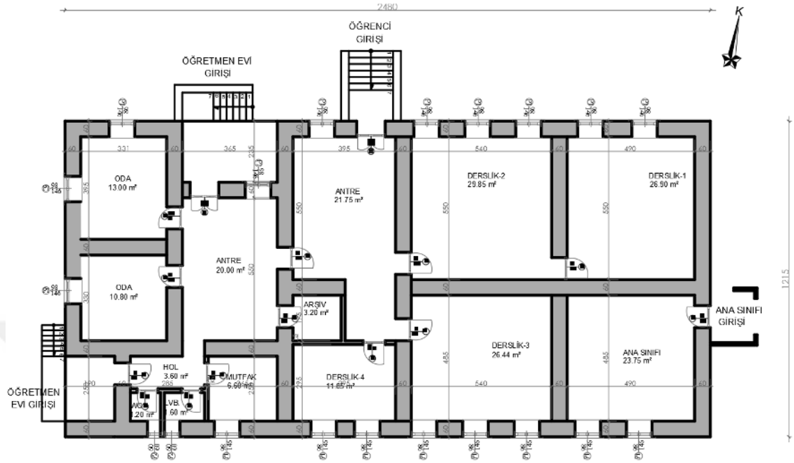
Şekil 6.2.2.4. Bayındır Köyü Okulu Zemin Kat Planı (Yılmaz Özev, 2024)
