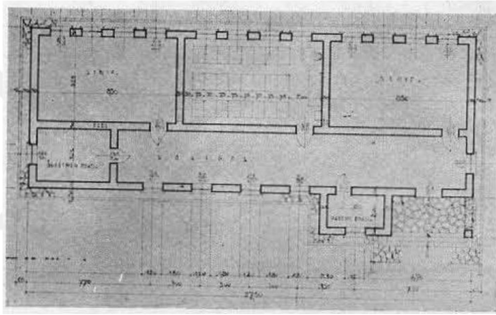
Şekil 5.16. Behçet Ünsal'ın çizimi olan köy mektebi planı (Ünsal, 1940)
