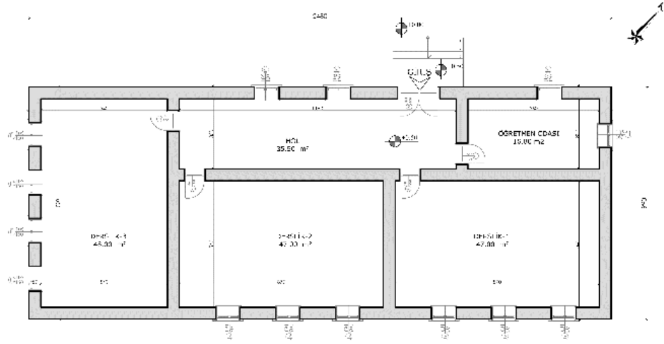
Şekil 6.2.15.4. Yarıköy Köyü Okulu Zemin Kat Planı (Yılmaz Özev, 2024)
