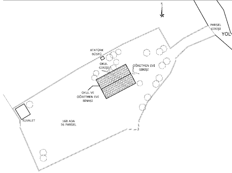
Şekil 6.2.11.3. Karacaören Köyü Okulu Vaziyet Planı (Yılmaz Özev, 2024)
