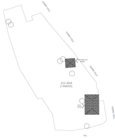
Şekil 6.9.2.3. Elmacık Köyü Okulu Vaziyet Planı (Yılmaz Özev, 2024)
