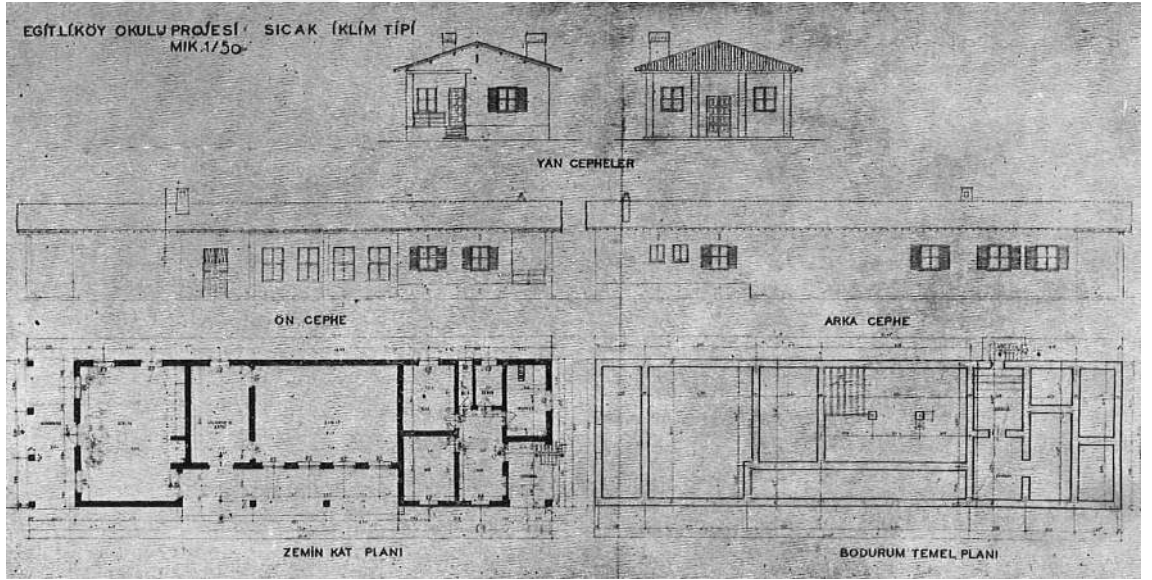
Şekil 5.10. Sıcak İklim Bölgesi Okul Projesi (Sayar, 1941)
