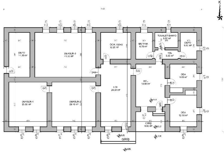
Şekil 6.2.8.4. Günelan Köyü Okulu Zemin Kat Planı (Yılmaz Özev, 2024)
