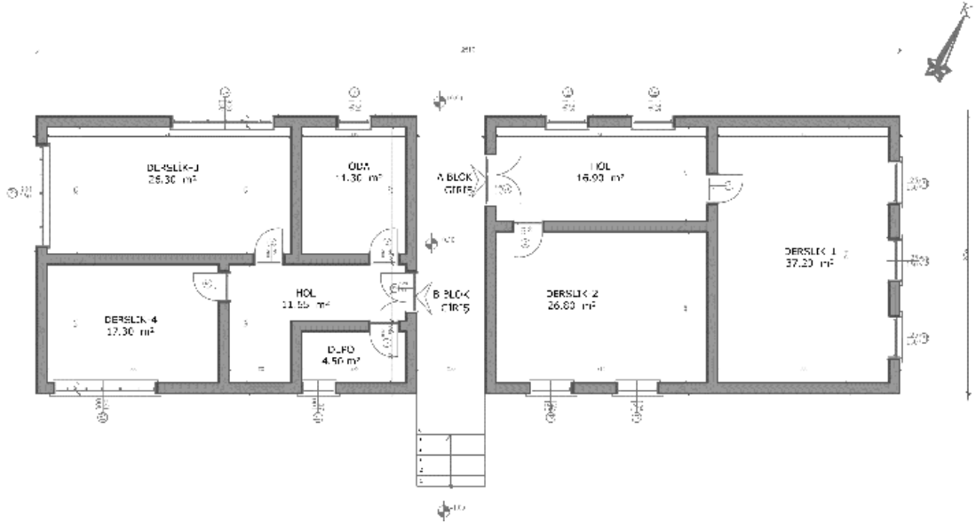
Şekil 6.2.12.4. Karakent Köyü Okulu Zemin Kat Planı (Yılmaz Özev, 2024)
