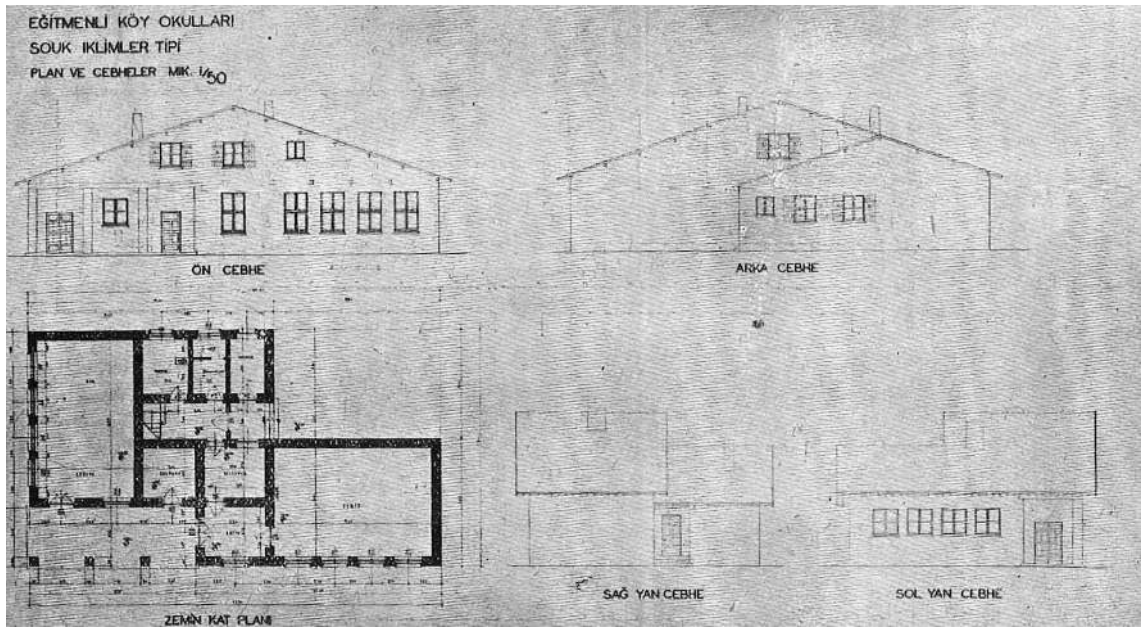
Şekil 5.8. Soğuk İklim Bölgesi Okul Projesi (Sayar, 1941)
