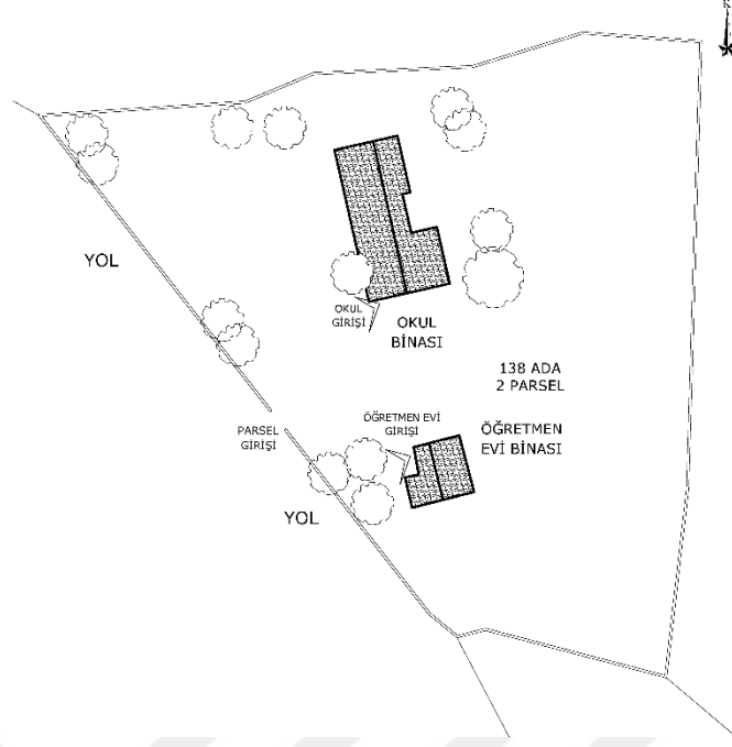
Şekil 6.11.2.3. Yeşilova Bayındır Köyü Okulu Vaziyet Planı (Yılmaz Özev, 2024)
