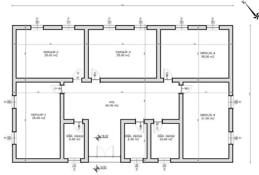
Şekil 6.10.3.26. Hasanpaşa Köyü Üçüncü Okulu Zemin Kat Planı (Yılmaz Özev, 2024)
