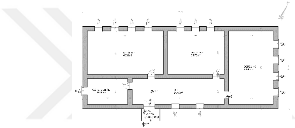
Şekil 6.2.16.5. Yaylabeli Köyü Okulu Zemin Kat Planı (Yılmaz Özev, 2024)
