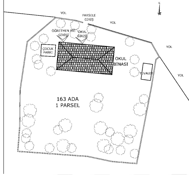
Şekil 6.2.6.3. Bozlar Köyü Vaziyet Planı (Yılmaz Özev, 2024)
