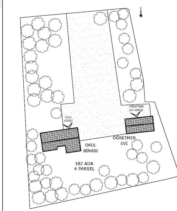
Şekil 6.5.1.3. Kayacık Köyü Okulu Vaziyet Planı (Yılmaz Öz, 2024)
