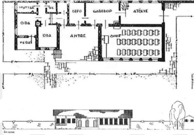
Şekil 5.4. Soğuk İklim Bölgesi Proje Örneği-1 (Mutlu ve Yapanar, 1941)
