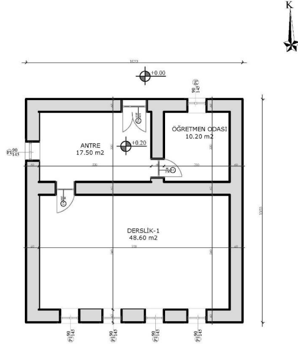
Şekil 6.3.3.4. Yumrutaş Çamova Köyü Okulu Zemin Kat Planı (Yılmaz Özev, 2024)
