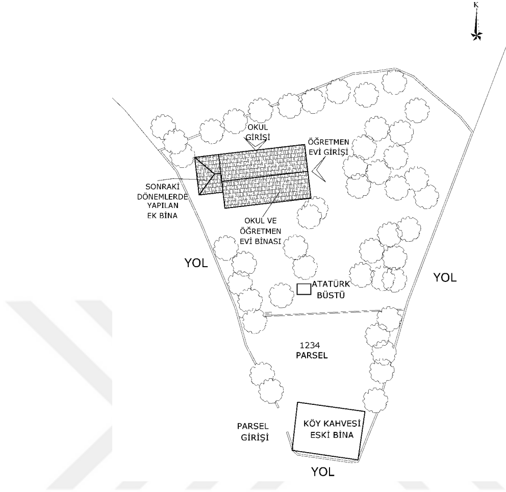
Şekil 6.10.2.3. Ece Köyü Okulu Vaziyet Planı (Yılmaz Özev, 2024)
