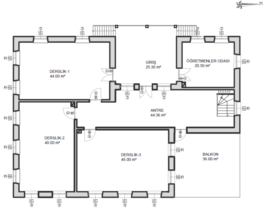
Şekil 6.9.2.7. Elmacık Köyü Okulu Zemin Kat Planı (Yılmaz Öz, 2022)
