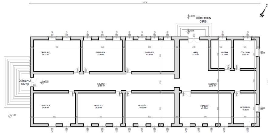
Şekil 6.8.1.5. Devrim Okulu Zemin Kat Planı (Yılmaz Özev, 2024)
