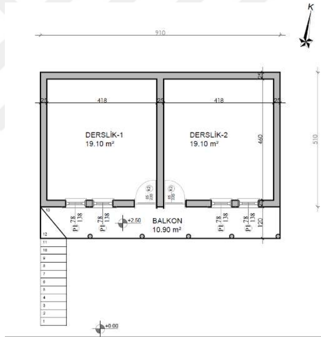
Şekil 6.2.9.5. Halıcılar Köyü Okulu 1. Kat Planı (Yılmaz Özev, 2024)
