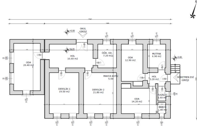
Şekil 6.10.2.5. Ece Köyü Okulu Zemin Kat Planı (Yılmaz Özev, 2024)
