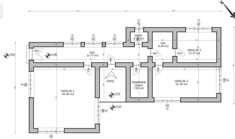
Şekil 6.10.3.13. Hasanpaşa Köyü İkinci Okulu Zemin Kat Planı (Yılmaz Özev, 2024)
