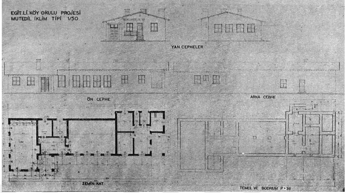
Şekil 5.9. Mutedil İklim Bölgesi Okul Projesi (Sayar, 1941)
