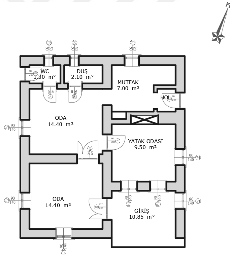
Şekil 6.2.15.13. Yarıköy Köyü Okulu Öğretmen Evi Zemin Kat Planı (Yılmaz Özev Arşivi, 2024)
