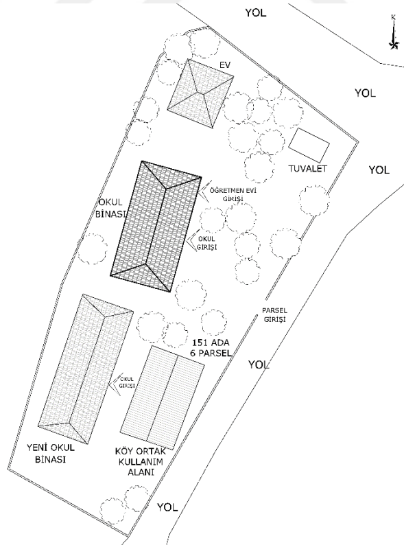
Şekil 6.11.8.3. Yukarı Kırılı Köyü Okulu Vaziyet Planı (Yılmaz Özev, 2024)
