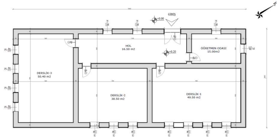
Şekil 6.10.3.4. Hasanpaşa Köyü Birinci Okulu Zemin Kat Planı (Yılmaz Özev, 2024)
