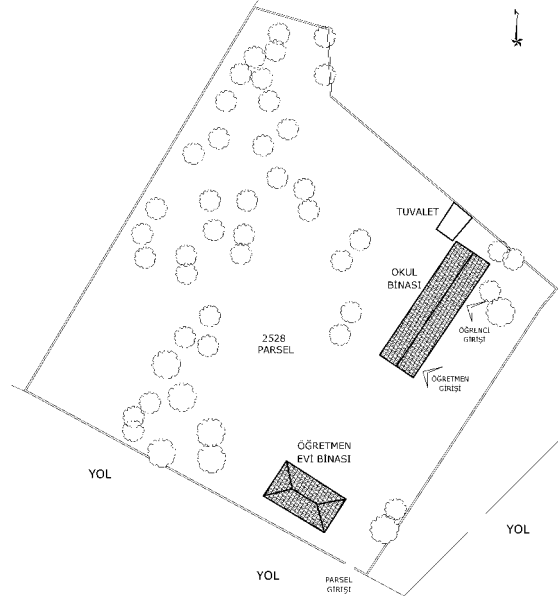
Şekil 6.11.5.3. Gençali Köyü Okulu Vaziyet Planı (Yılmaz Özev, 2024)
