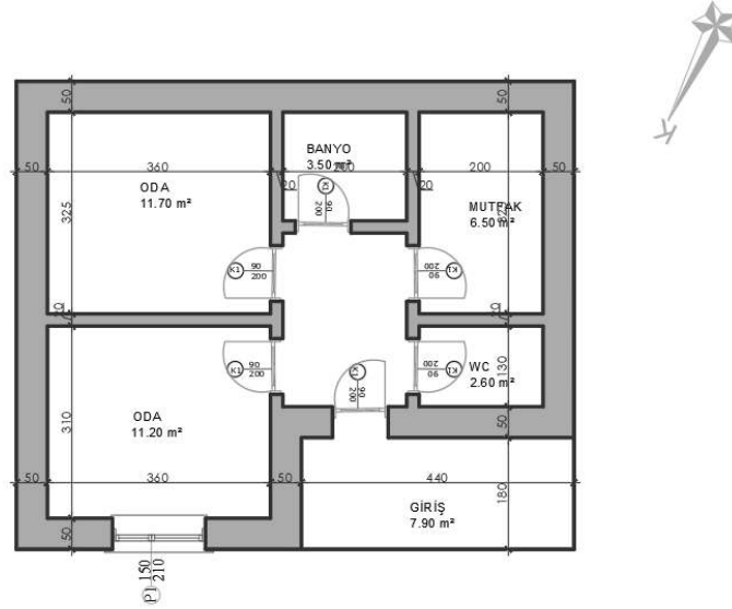
Şekil 6.11.1.13. Alanköy Köyü Okulu Öğretmen Evi Zemin Kat Planı (Yılmaz Özev, 2024)
