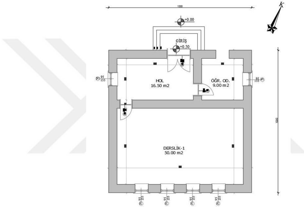
Şekil 6.11.3.5. Yeşilova Bayırbaşı Köyü Okulu Zemin Kat Planı (Yılmaz Özev, 2024)
