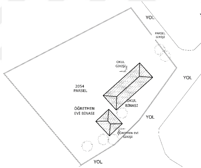
Şekil 6.2.15.3. Yarıköy Köyü Okulu Vaziyet Planı (Yılmaz Özev, 2024)
