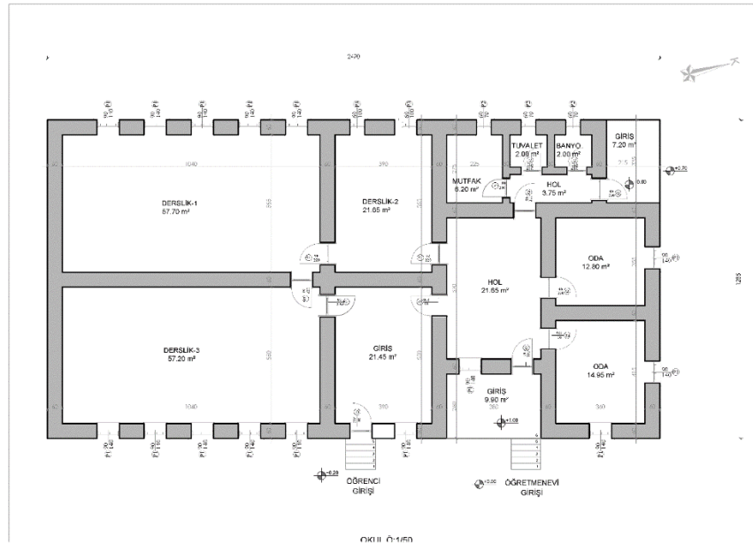
Şekil 6.11.8.6. Yukarı Kırılı Köyü Okulu Zemin Kat Planı (Yılmaz Özev, 2024)
