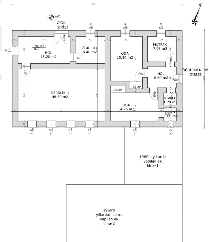
Şekil 6.10.4.5. Sazak Köyü Okulu Zemin Kat Planı (Yılmaz Özev, 2024)
