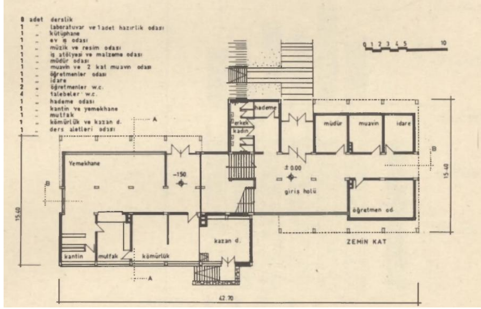
Şekil 6.1.8.14. Ortaokul/ Lise Tip Proje Zemin Kat Planı (Okan, 1976)
