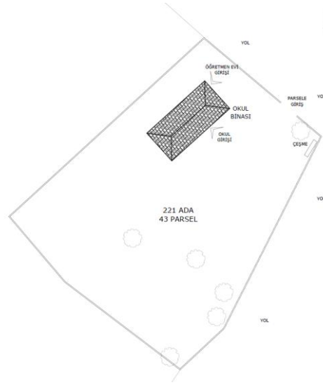
Şekil 6.2.1.3. Başmakçı Köyü Vaziyet Planı (Yılmaz Özev, 2024)
