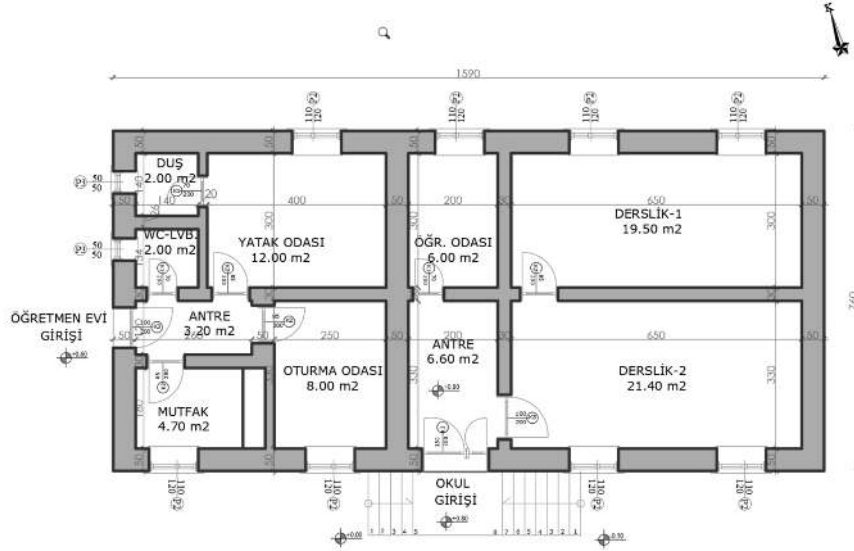
Şekil 6.2.4.7. Beşkavak Köyü Okulu Zemin Kat Planı (Yılmaz Özev, 2024)
