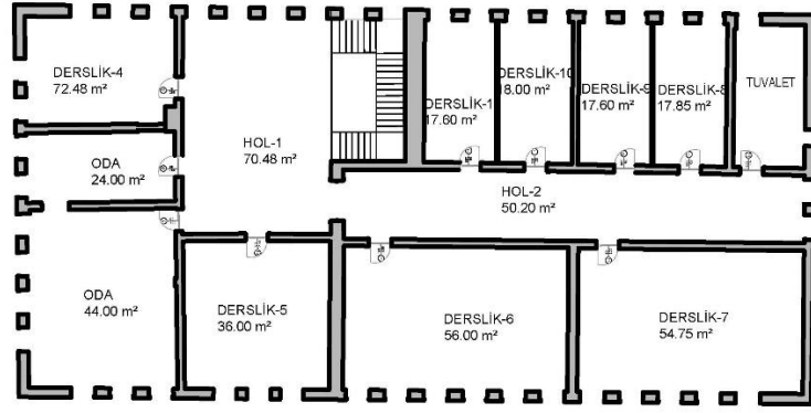
Şekil 6.1.6.9. Kız Sanat Enstitüsü 1. Kat Rölöve Planı (Yılmaz Özev, 2022)
