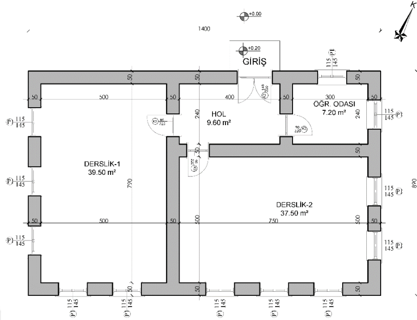
Şekil 6.2.5.4. Boğaziçi Köyü Okulu Zemin Kat Planı (Yılmaz Özev, 2024)
