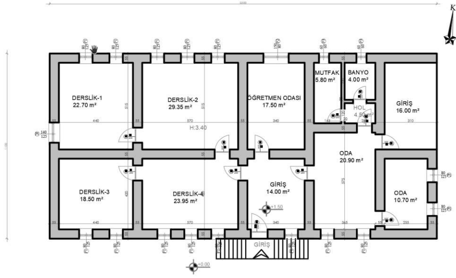
Şekil 6.2.1.6. Başmakçı Köyü Okulu Zemin Kat Planı (Yılmaz Özev, 2024)
