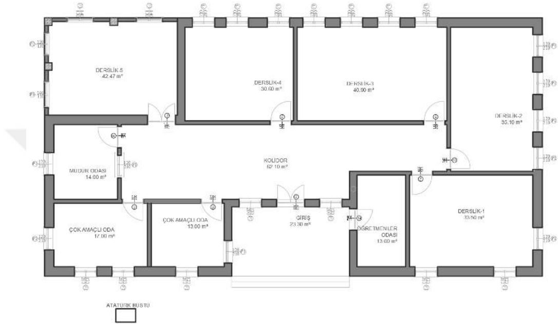
Şekil 6.2.13.5. Kayaaltı Köyü Okulu Tadilatlı Zemin Kat Planı (Yılmaz Özev, 2024)
