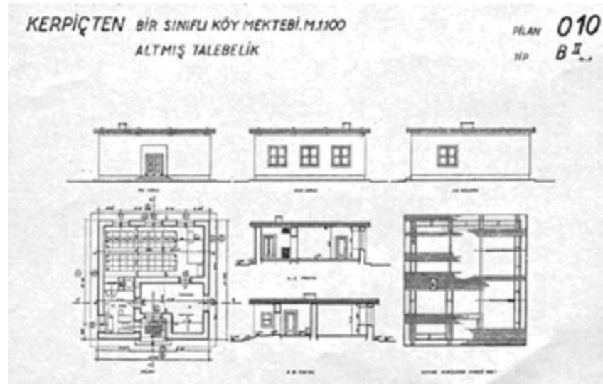
Şekil 5.12. İnşaat Bürosu tarafından tasarlanan, kerpiç malzeme ile yapılması öngörülen bir sınıflı 60 öğrencili köy okulu (İlkmektep Planları Albümü, 1933)
