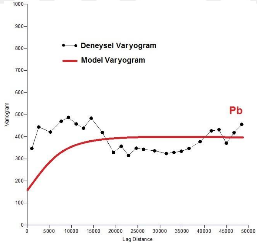
Şekil 6.8. Bölgedeki Pb cevherleşmesine ait deneyel ve model varyogramı
