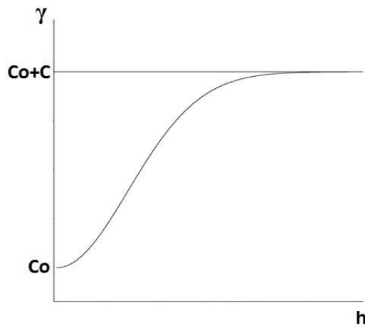
Şekil 6.2. Gauss modeli
