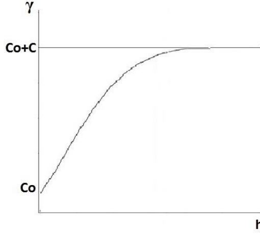
Şekil 6.3. Üssel model
