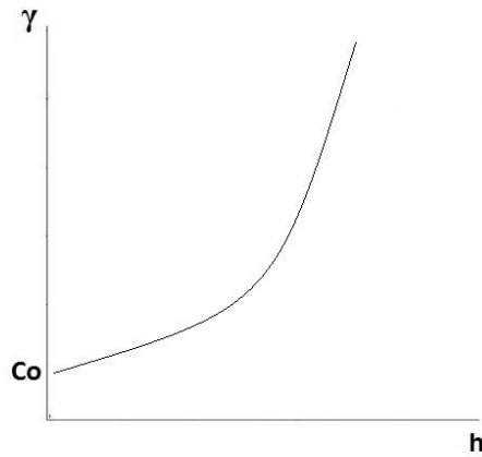
Şekil 6.6. Logaritmik model
