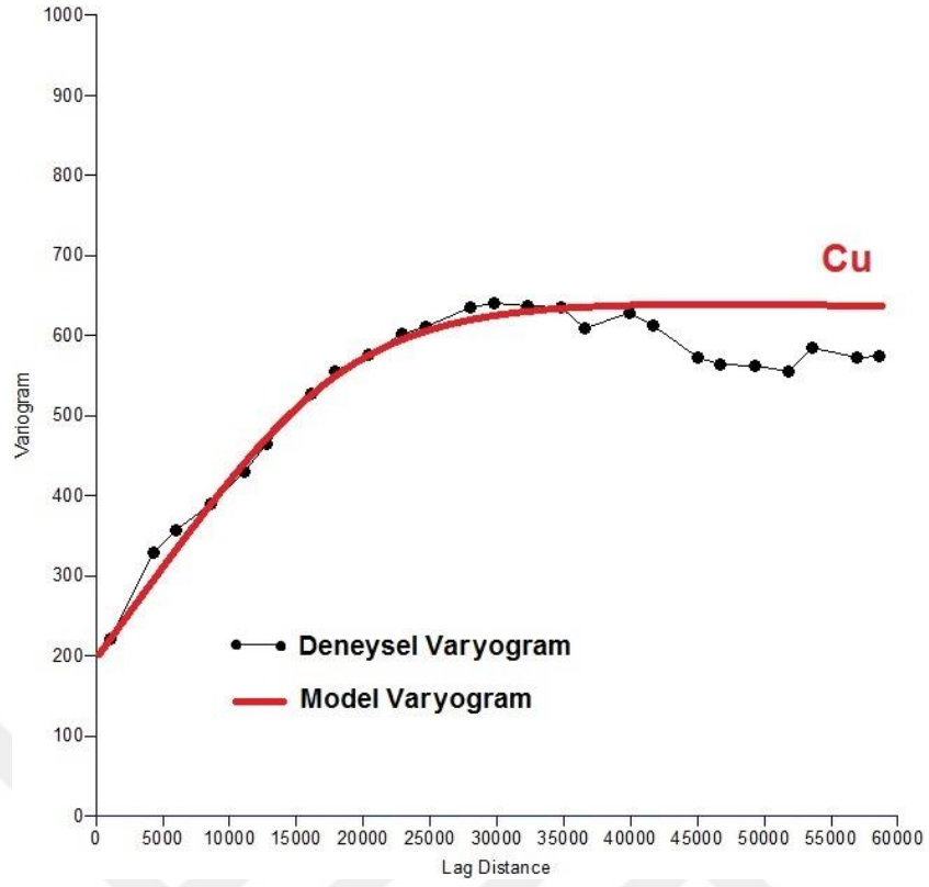
Şekil 6.7. Bölgedeki Cu cevherleşmesine ait deneyel ve model varyogramı
