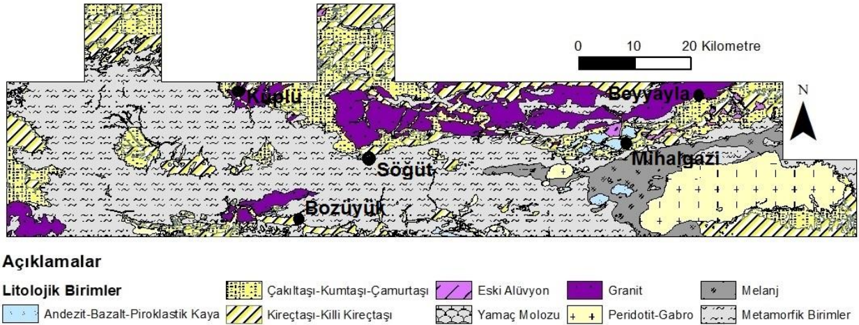
Şekil 3.1: Çalışma sahasının jeolojik haritası (MTA 1/25000'lik jeolojik harita paftalarından değiştirilerek ve sadeleştirilerek hazırlanmıştır).
