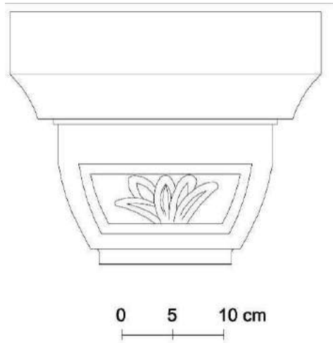
Çizim 55. Başlığın Güney Yüzü (Çizen: YPD, Genim-2016)
