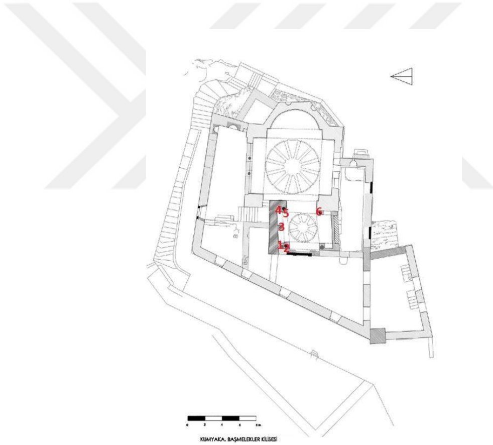
Çizim 29. Sütun Kaidelerinin Yapı Topluluğundaki Yerleri (Çizen: YPD, Genim'den Değiştirilerek-2017)
