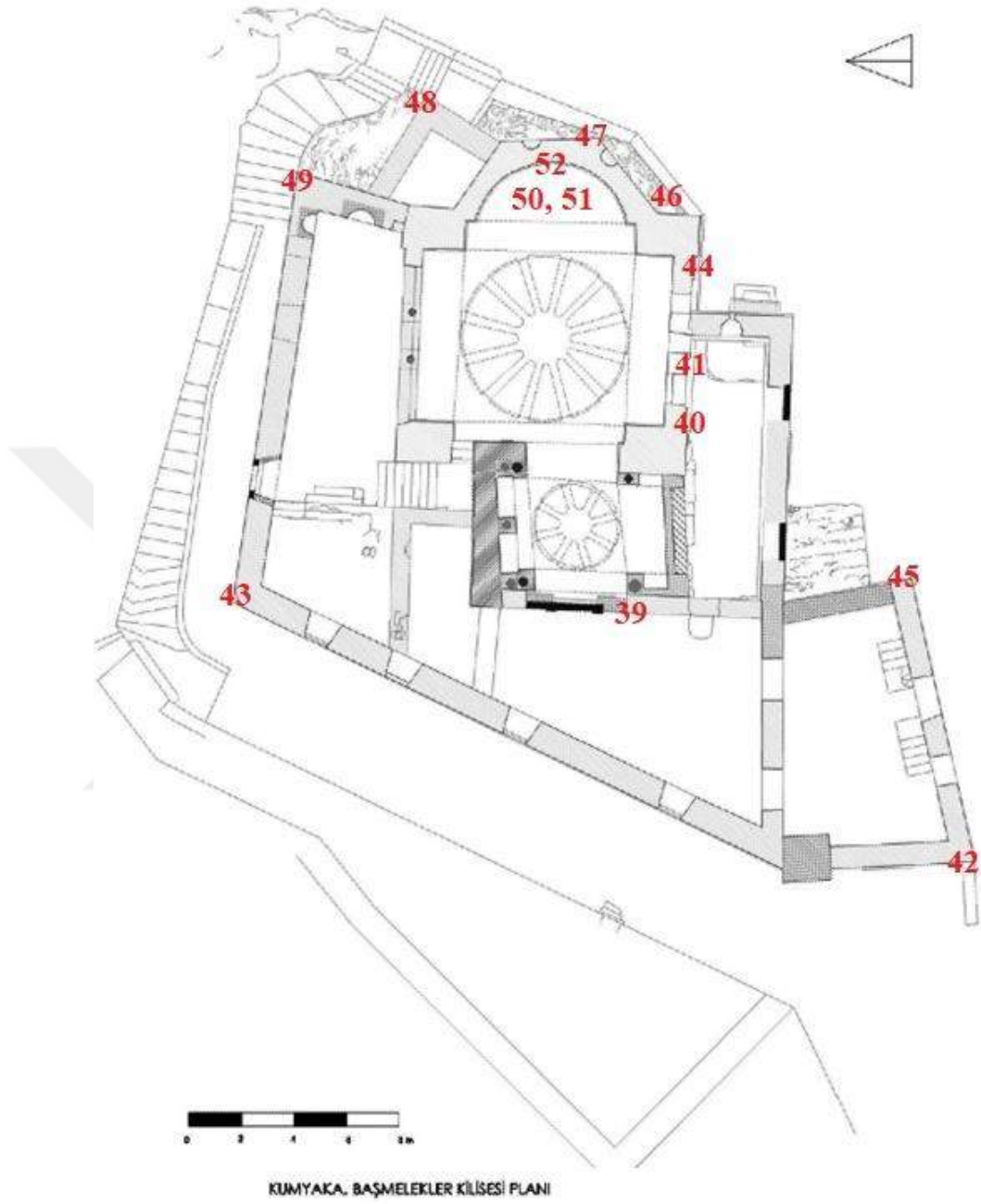
Çizim 34. Templon Payeleri, Altar Kaidesi, Altar Ayağı ve Kathedra'nın Yapı Topluluğundaki Yerleri (Çizen: YPD, Genim'den Değiştirilerek-2017)
