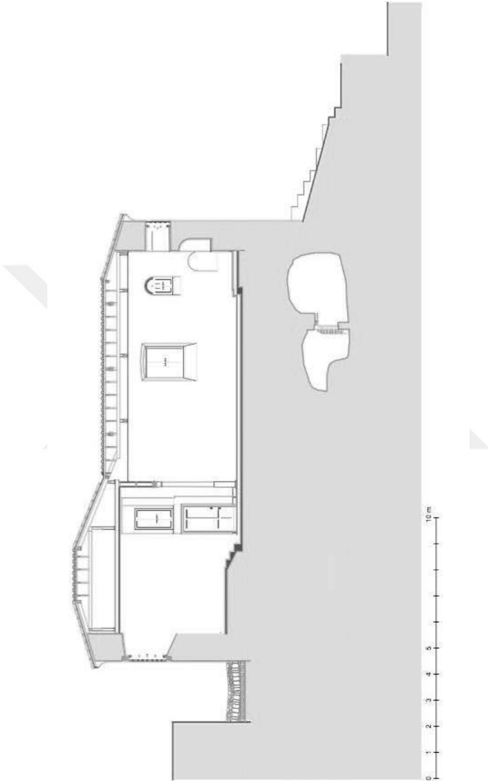
Çizim 121. Restitüsyon Önerisi XVI, C Mekanı (Aziz Haralambos Şapeli), E ve F Mekanları (Kayaya Oyulmuş Mekanlar) Batı Doğu Kesiti (Çizen: YPD, Genim'den Değiştirilerek D. Gür- 2017)
