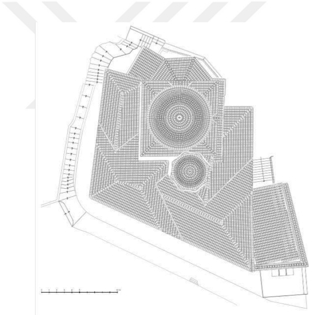
Çizim 129. Restitüsyon Önerisi XXIV, Örtü Sistemi (Çizen: YPD, Genim'den Değiştirilerek D. Gür- 2017)
