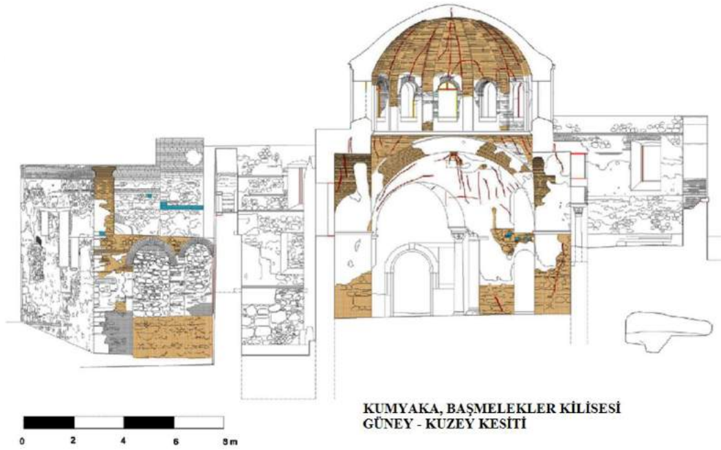
Çizim 21. Kumyaka, Başmelekler Kilisesi, Güney – Kuzey Kesiti (Çizen: YPD, Genim-2016)
