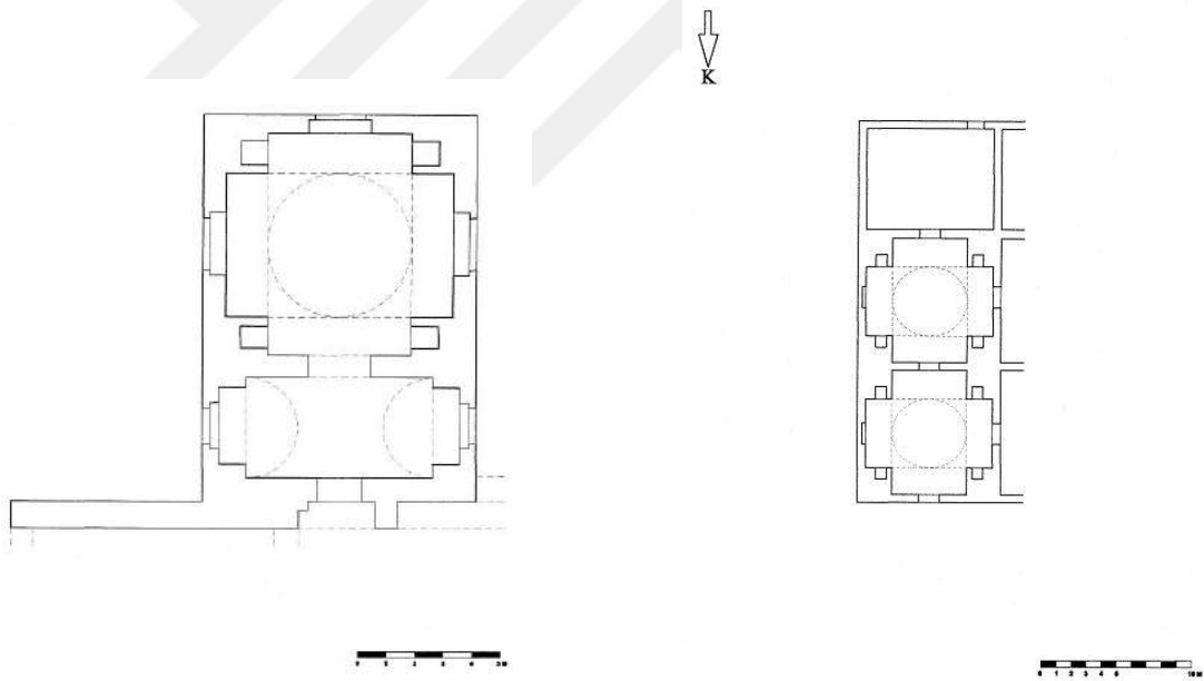
Çizim 85. Side Mabretler Bazilikasının Güneyindeki Martyrion (Eyice, 1960)
