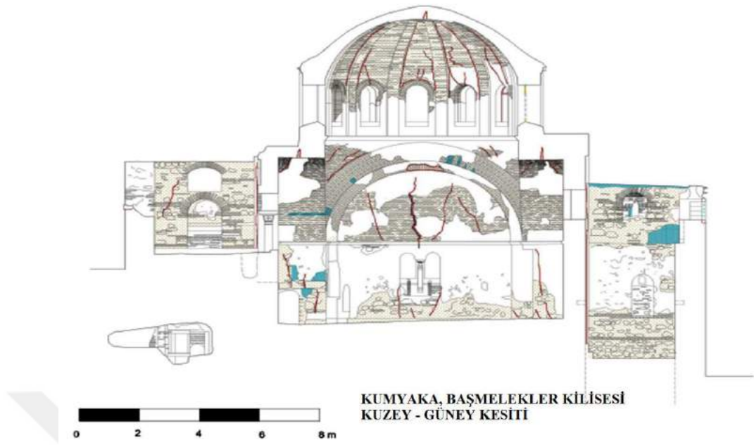
Çizim 20. Kumyaka, Başmelekler Kilisesi, Kuzey – Güney Kesiti (Çizen: YPD, Genim-2016)
