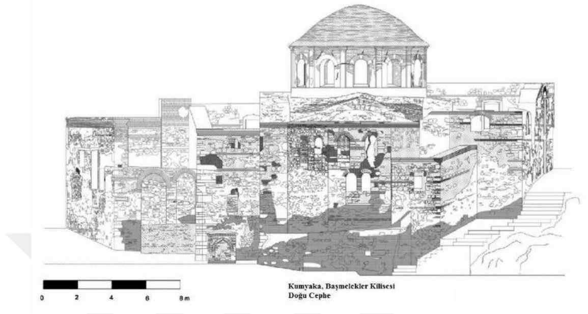
Çizim 22. Doğu Cephe (Çizen: YPD, Genim-2016)
