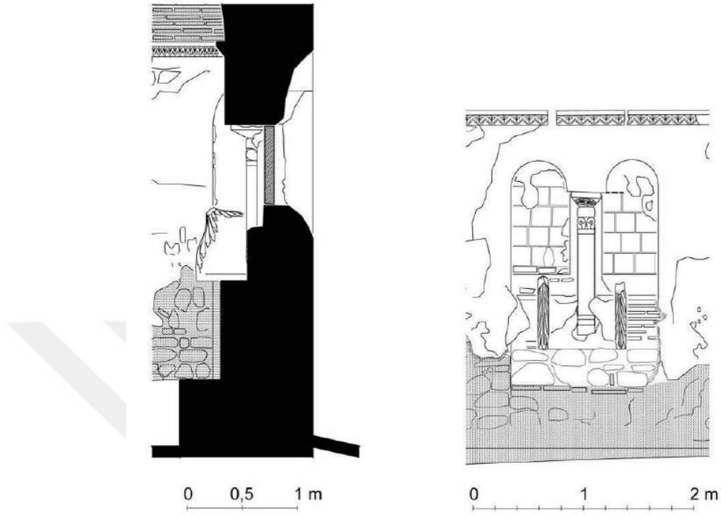
Çizim 49. İkiz Pencere Sütunu, Kesit ve Görünüş (Çizen: YPD, Genim-2016)
