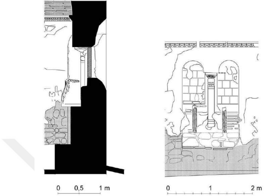
Çizim 49/79. Kat.No.20/52, Çift Pencere Sütunu ve Kathedra, Kesit ve Görünüş (Çizen: YPD, Genim-2016)
