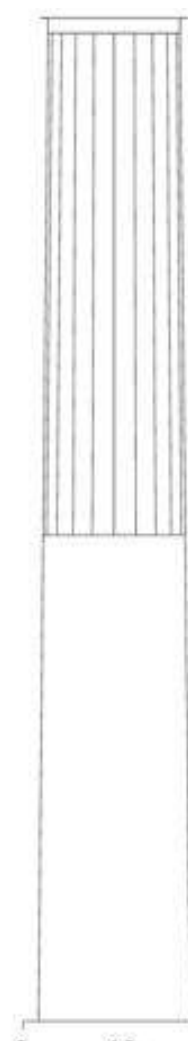
Çizim 39. Kaidenin Kuzey Yüzü (Çizen: YPD, Genim-2016)
