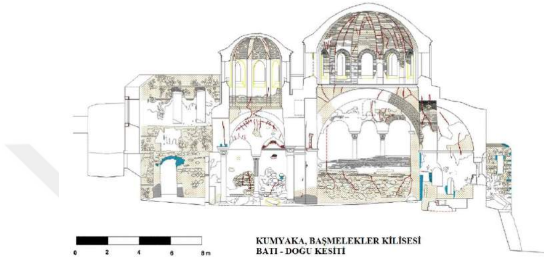
Çizim 18. Kumyaka, Başmelekler Kilisesi, Batı – Doğu Kesiti (Çizen: YPD, Genim-2016)
