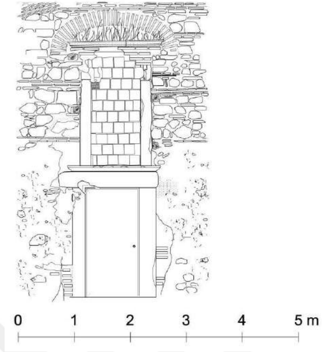
Çizim 69. Söve (Çizen: YPD, Genim-2016)
