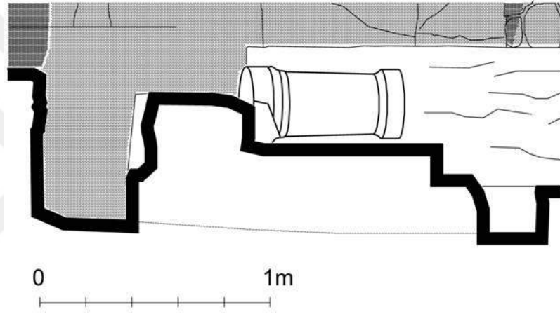
Çizim 77. Altar Ayağı, Kesit (Çizen: YPD, Genim-2016)
