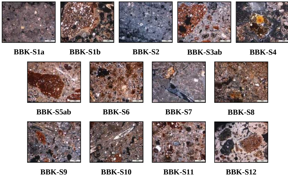
Şekil 7. Başmelekler Kilisesi taş, tuğla, harç ve sıva örneklerinin ince kesit mikrofotografaları
