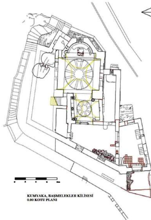
Çizim 6. Başmelekler Kilisesi, 0.00 Kotu Planı (Çizen: YPD, Genim-2016)
