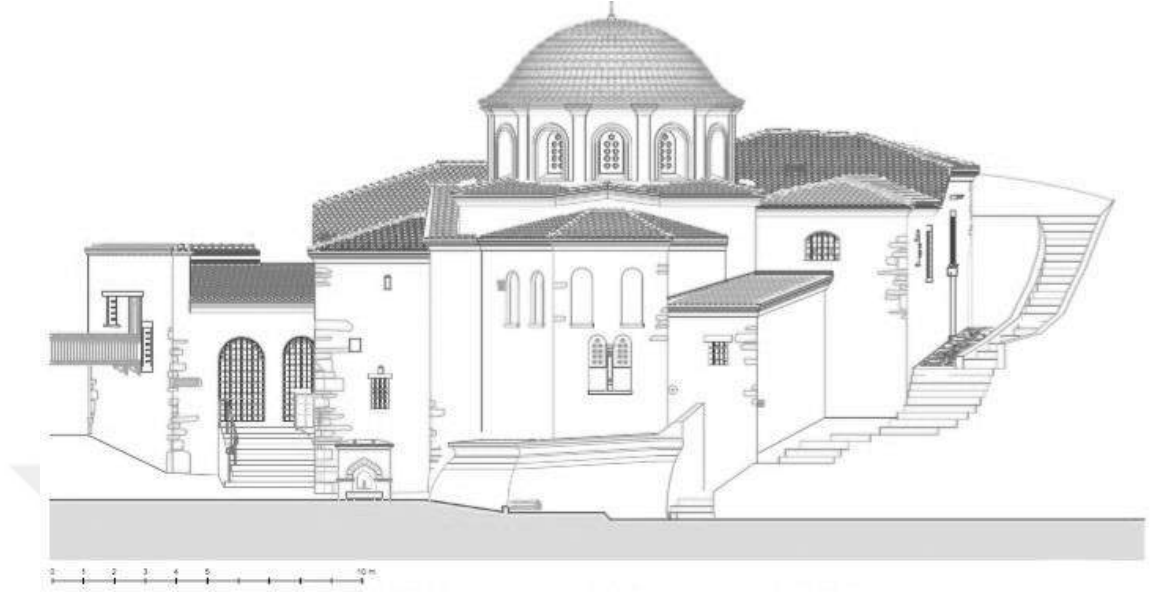
Çizim 127. Restitüsyon Önerisi XXII, Doğu Cephe (Çizen: YPD, Genim'den Değiştirilerek D. Gür- 2017)
