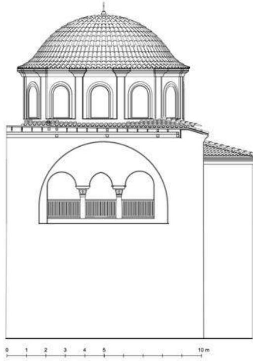
Çizim 104. Restitüsyon Önerisi IV, Kuzey Cephe (Çizen: YPD, Genim'den Değiştirilerek D. Gür- 2017)
