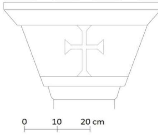
Çizim 58. Kat.No.27, Başlığın Batı Yüzü (Çizen: YPD, Genim-2016)
