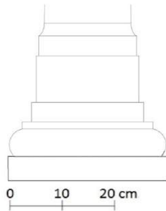
Çizim 39. Kaidenin Kuzey Yüzü (Çizen: YPD, Genim-2016)
