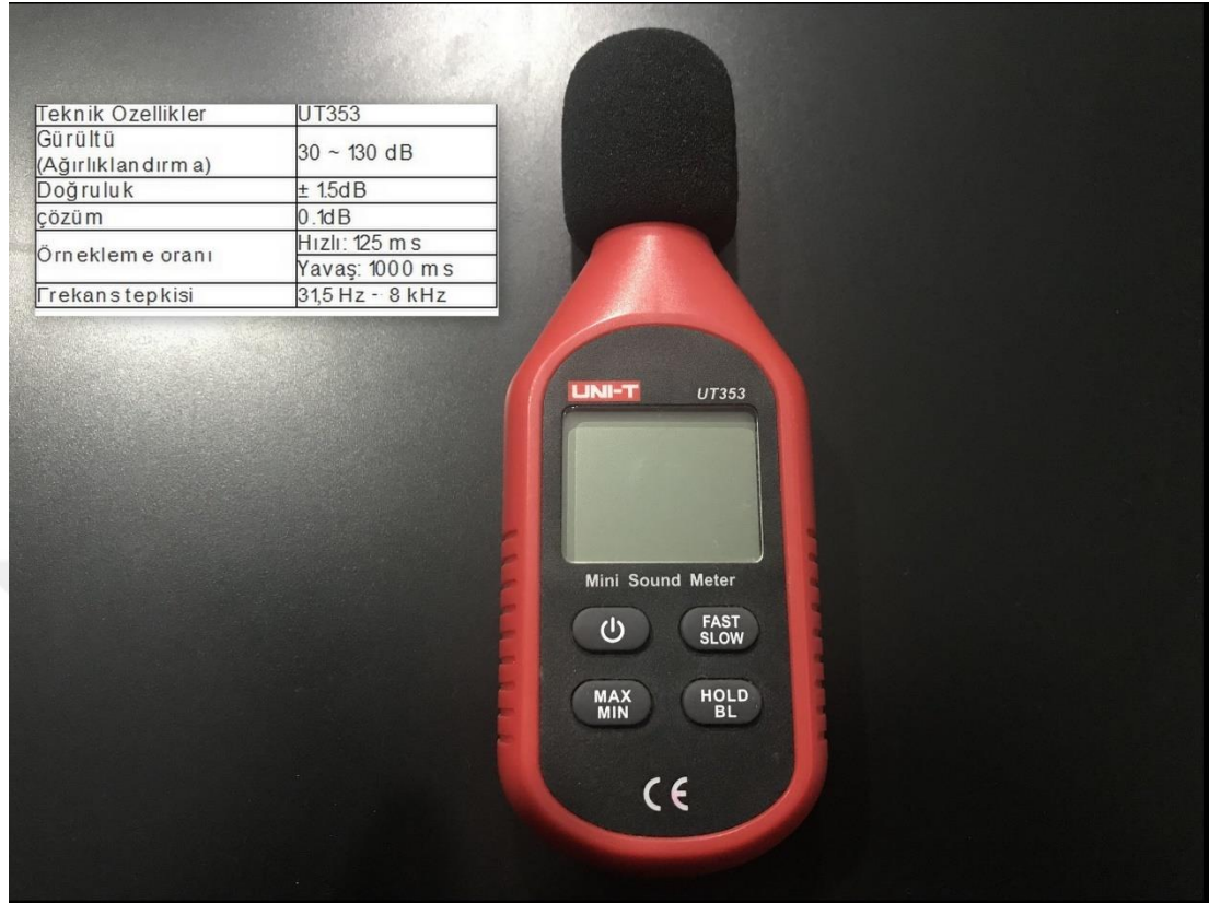
Şekil 4.192: UNI-T UT353 gürültü ölçüm cihazı
