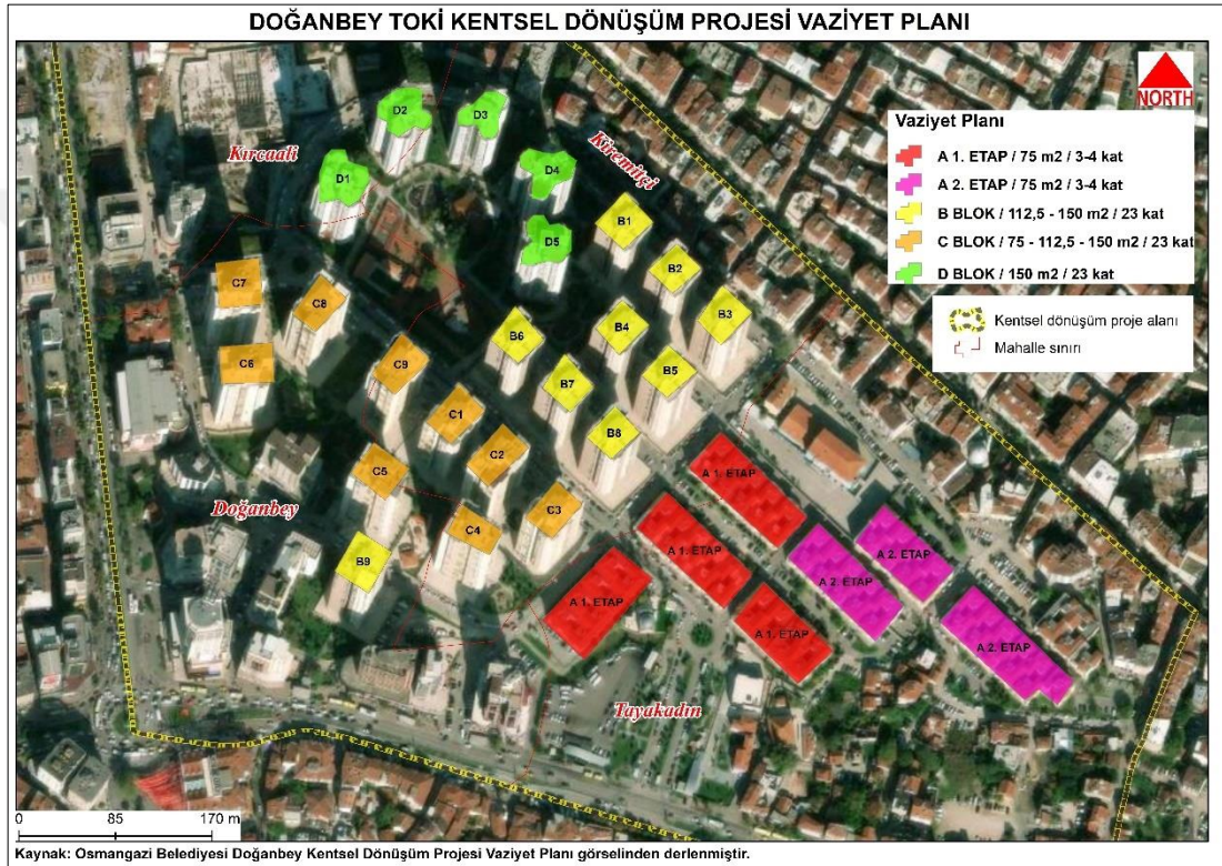
Şekil 4.119: Doğanbey TOKİ kentsel dönüşüm projesi vaziyet planı
