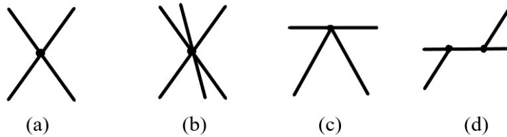
Şekil 2.4. Doğrunun izdüşümü
