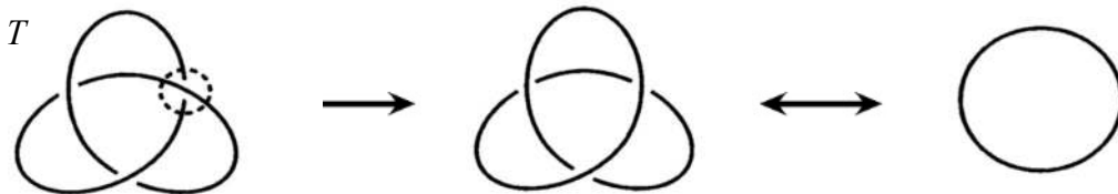
Şekil 2.15. u(T) = 1
