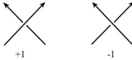
Şekil 2.6. Kavşakların çaprazlanması
