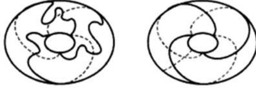
Şekil 2.8. (2,3) –torus düğümü
