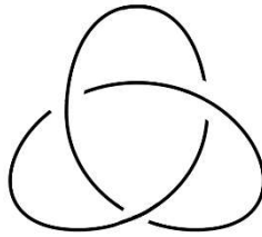
Şekil 2.1. Trefoil
