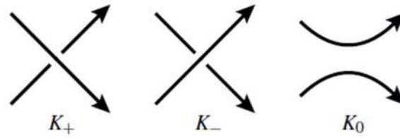
Şekil 3.1. Giriftlik diyagramları
