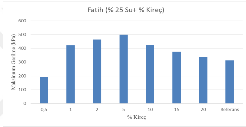
Şekil 6.5. Fatih zeminleri serbest basınç deneyi sonuçları-1
