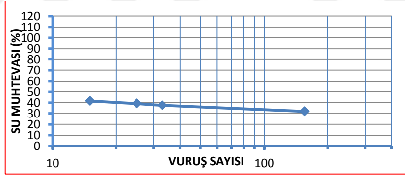
Şekil 5.7. Osmangazi mahallesi zemin numunesi likit limit deneyi grafiği
