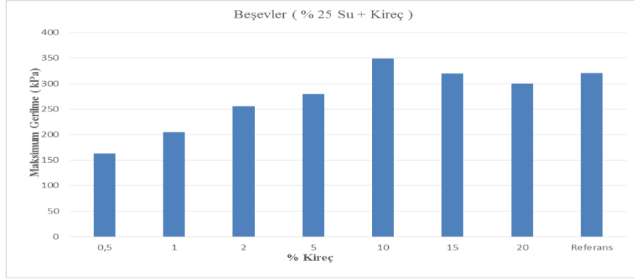
Şekil 6.1. Beşevler zeminleri serbest basınç deneyi sonuçları-1
