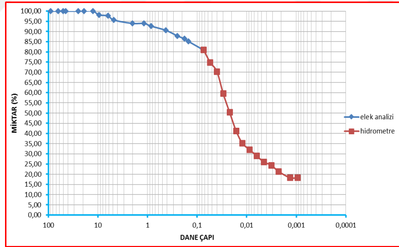
Şekil 5.10. Fabrikalar Bölgesi zemin numunesi granülometri eğrisi
