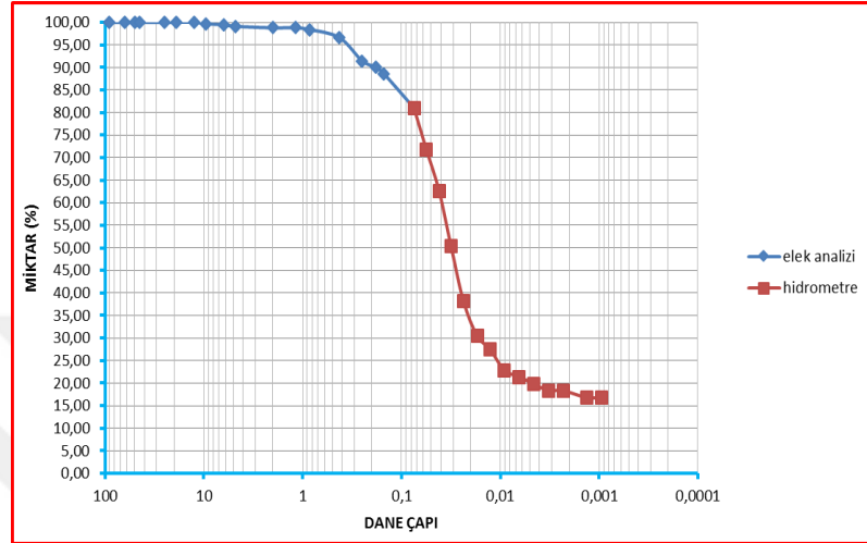
Şekil 5.9. Beşevler mahallesi zemin numunesi granülometri eğrisi
