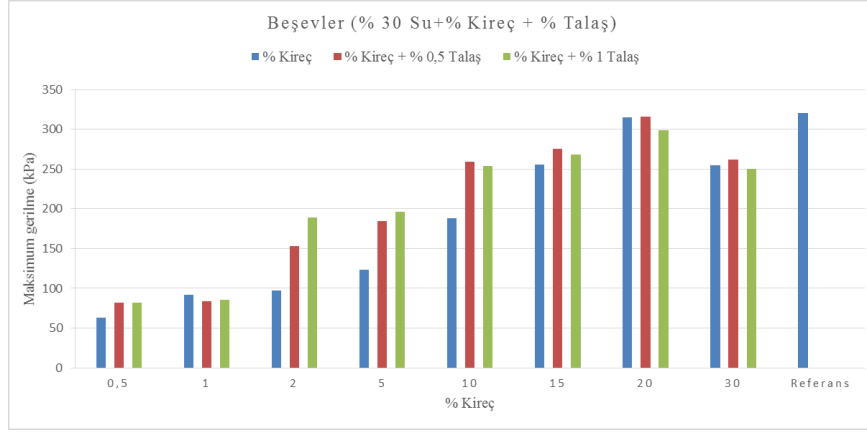
Şekil 6.4. Beşevler zeminleri serbest basınç deneyi sonuçları-4
