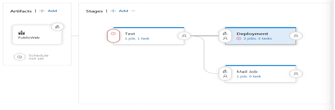
Şekil 5.6. Pipeline Diagram
