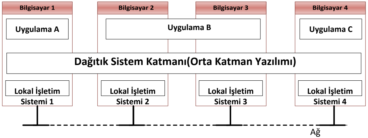
Şekil 1.1. Dağıtık sistem mimarisi [1]
