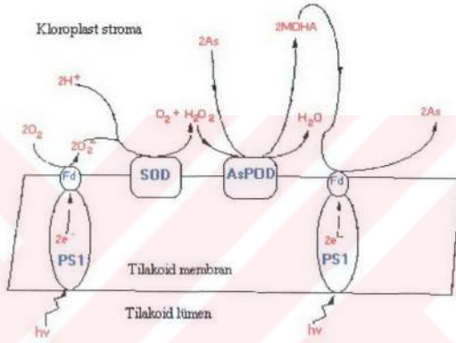
Şekil 1: Tilakoid membranlardaki mehler- peroksidaz reaksiyon dizisi (PS I: Fotosistem I, Fd: Ferrodoksin, As: Askorbik asit, MDHA: Monodehidro askorbat)
