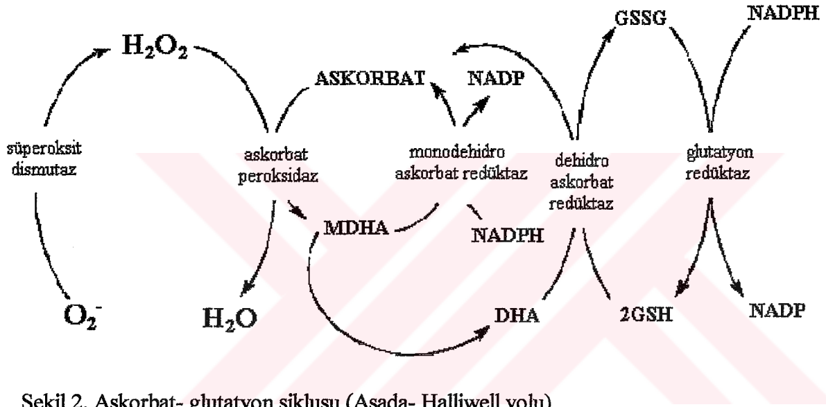
Şekil 2. Askorbat- glutatyon siklusu (Asada- Halliwell yolu)
