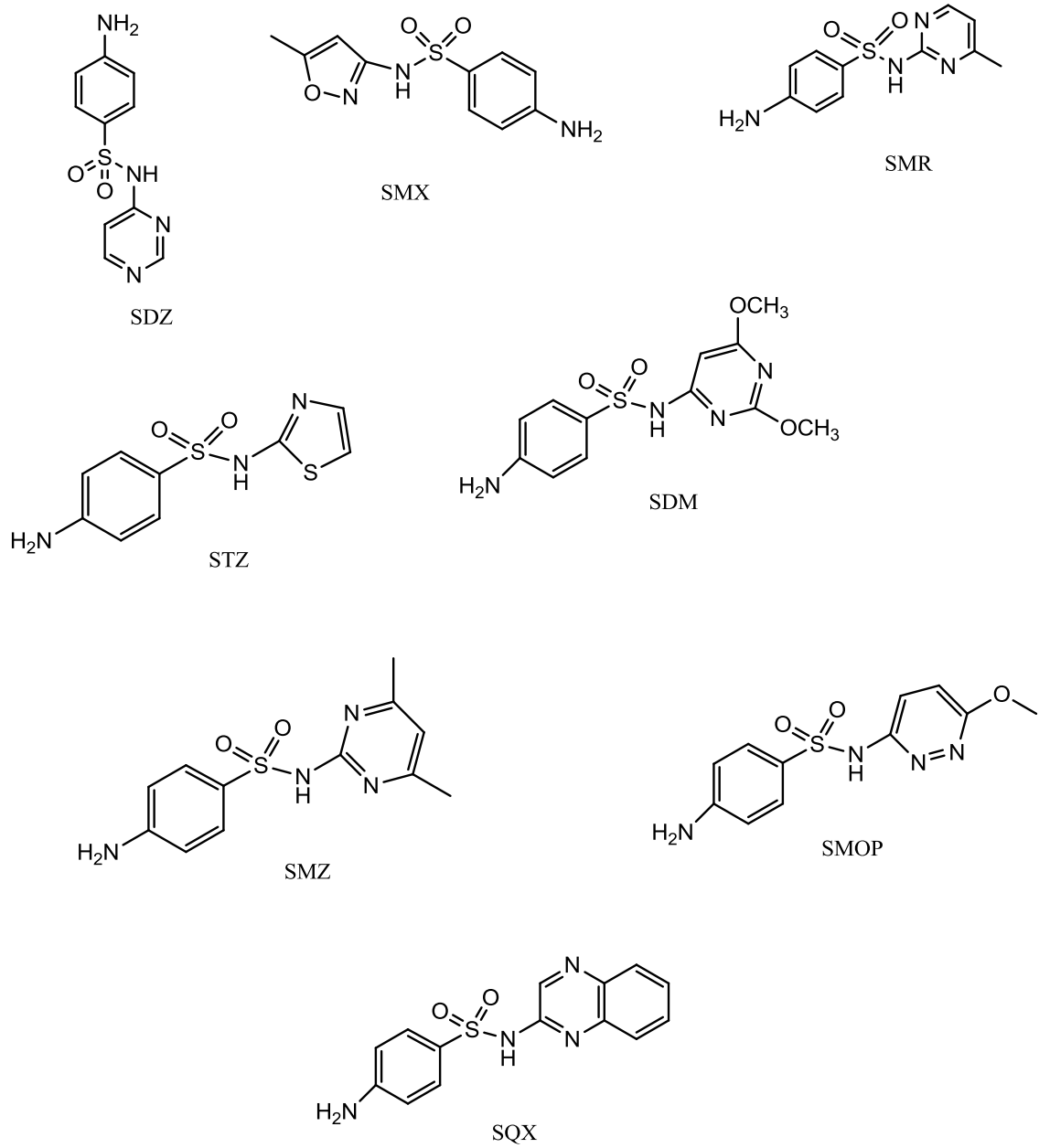
Şekil 3.1. Sülfonamidlerin Yapısı
