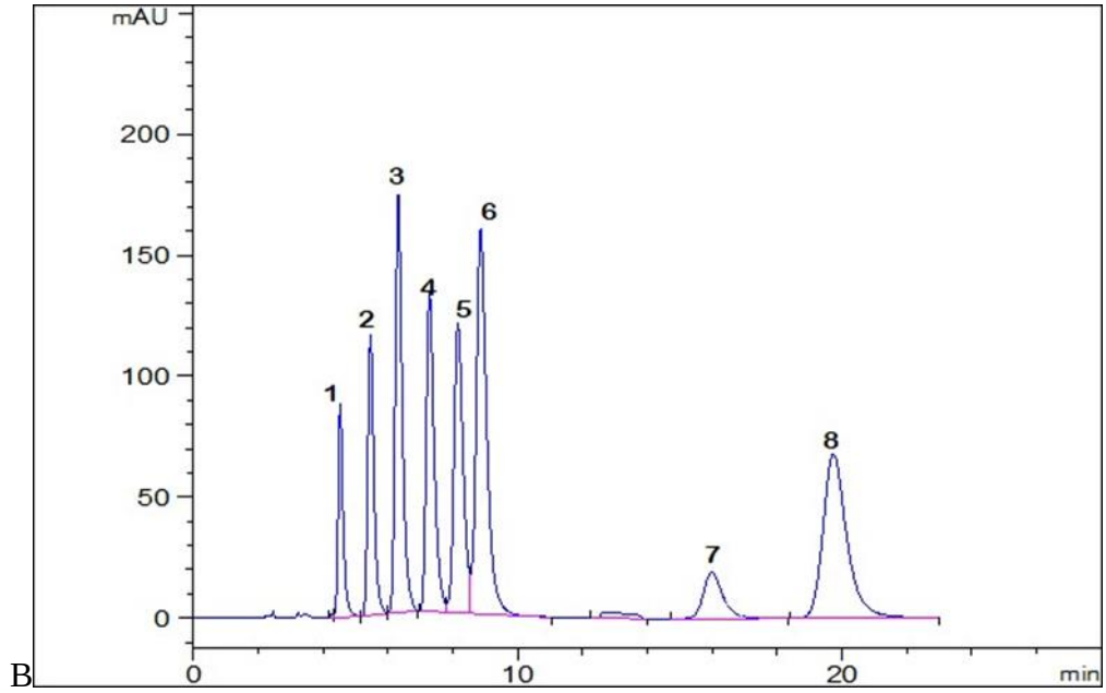
Şekil 4.1. Sekiz sülfonamidin ayrılması için optimum (A) gradyan ve (B) izokratik koşullar. Kromatografik Koşullar: (A) ACN/tampon (pH 6.5, 40 mM \text{KH}_2\text{PO}_4/\text{K}_2\text{HPO}_4 , 10/90 (h/h)); 0–14 dak, 40/60; 14–20 dak., akış hızı: 1 mL/dak; 0–14 dak, 1–1.5 mL/dak; 14–20 dak; sıcaklık: 15 °C; enjeksiyon hacmi: 10 mL/100 ppm; dalga boyu: 250 nm. (B) ACN/tampon (pH 6.5, 40 mM \text{KH}_2\text{PO}_4/\text{K}_2\text{HPO}_4 , 10/90 (h/h)), akış hızı: 1.5 mL/dak, sıcaklık: 15 °C, enjeksiyon hacmi: 10 \mu\text{L} /100 ppm, dalga boyu: 250 nm. Analitler: SDZ, SMX, SMR, STZ, SMZ, SMOP, SDM ve SQX'tir.
