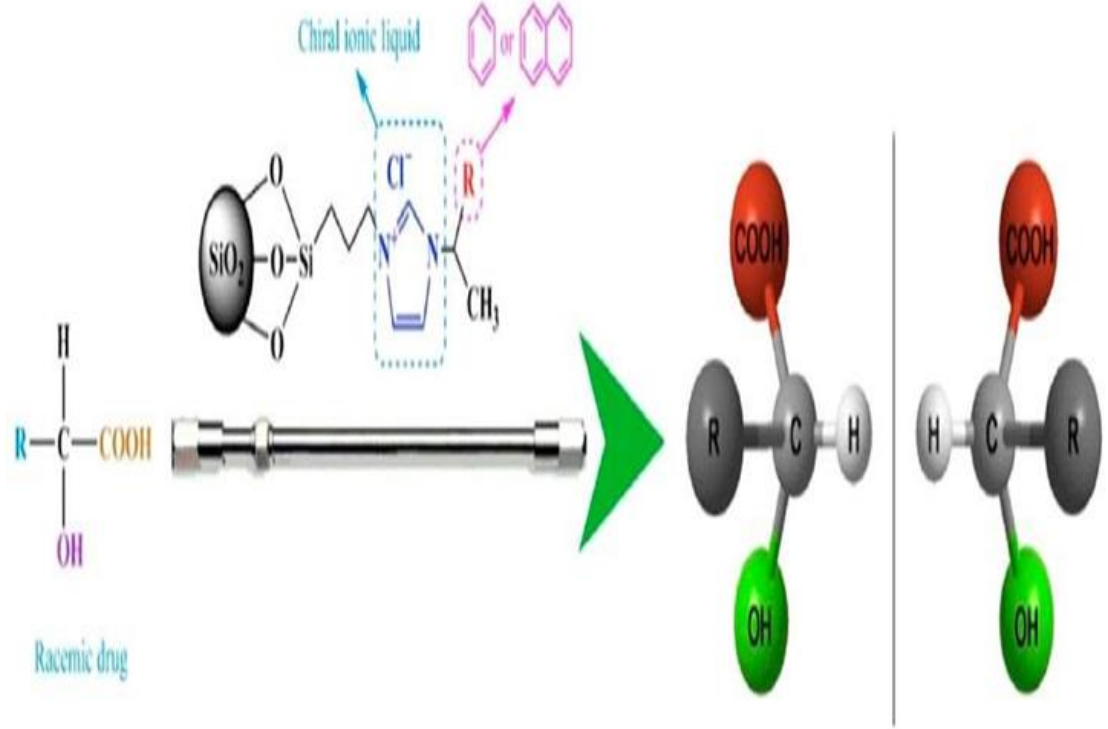
Şekil 2.3. HPLC için kiral imidazolium sabit fazları.(Rusli, 2022, akt. Wang vd. 2016, s.70) kaynaklı izni ile yeniden basılmıştır.
