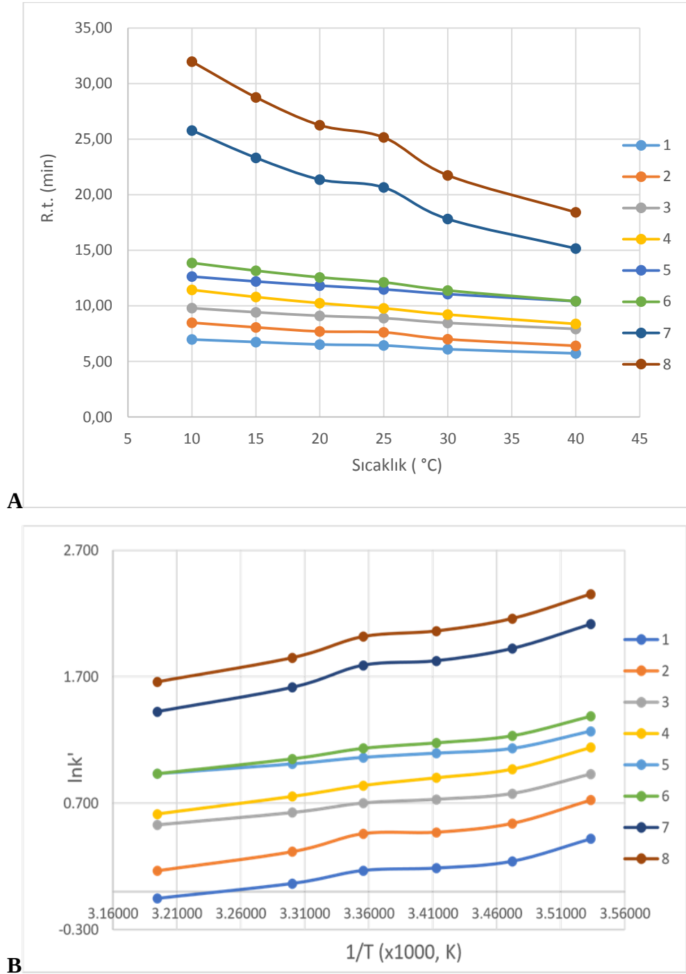
Şekil 4.6. Sıcaklığın, sülfonamidlerin C12-diol karma mod kolonu üzerindeki (A) alıkonma süresi (R.T.) ve (B) \ln k' ile 1/T (Van't Hoff denklemi) arasındaki ilişki üzerine etkisi. Analitler: (1) (SDZ), (2) (SMX), (3) (SMR), (4) (STZ), (5) (SMZ), (6) (SMOP), (7) (SDM), (8) (SQX). k' : kapasite faktörü
