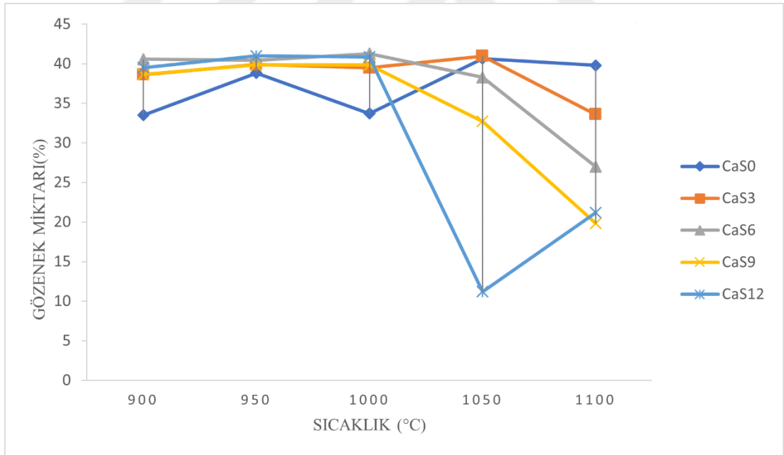
Şekil 6.10. Artan \text{CaF}_2 kompozisyonuna sahip numunelerin artan sinterleme sıcaklıklarına bağlı olarak gözenek miktarlarında meydana gelen değişim.
