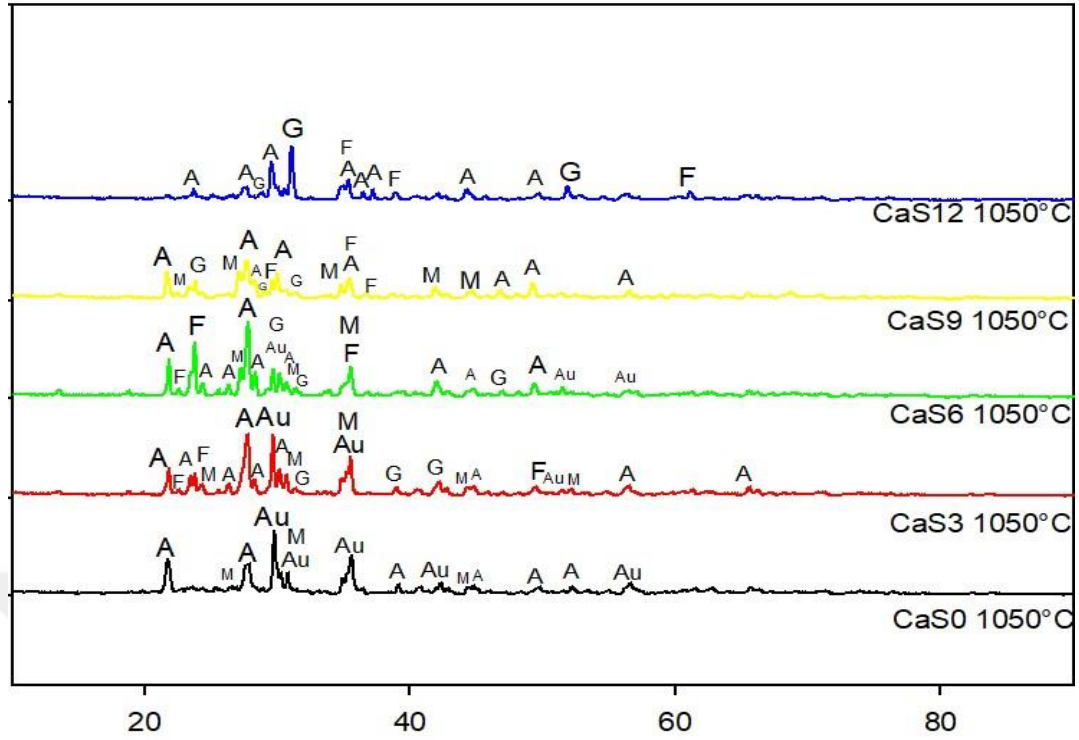
Şekil 6.21. Ağırlıkça beş farklı oranda (%0, %3, %6, %9, %12) \text{CaF}_2 içeren 1050 °C’de sinterlenmiş numunelerin XRD grafiği.
