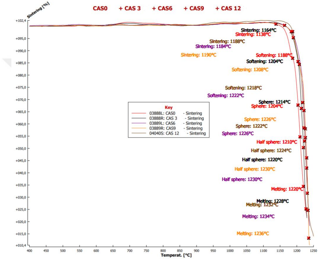
Şekil 6.6. Artan \text{CaF}_2 kompozisyonuna sahip numunelere uygulanan ısı mikroskop analiz sonuçlarının grafiksel gösterimi.
