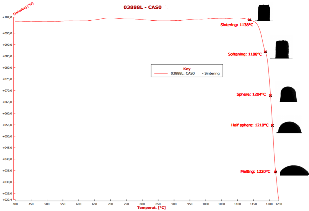
Şekil 6.1. CaS0 kodlu numunenin ısı mikroskop analiz sonuçlarının grafiksel gösterimi.
