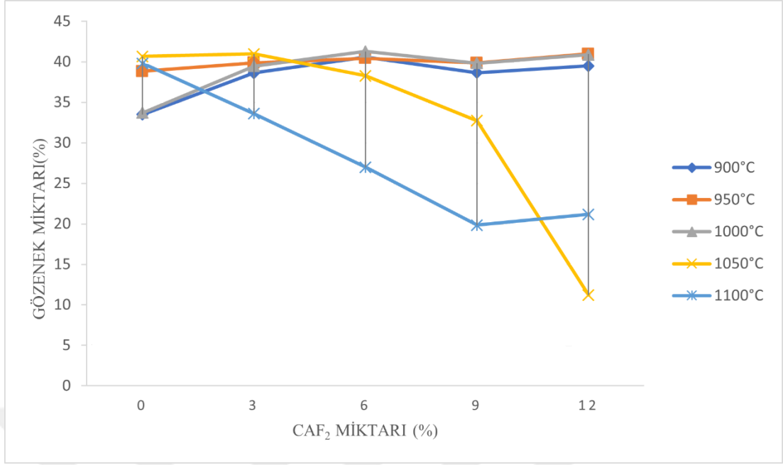
Şekil 6.9. 5 farklı sıcaklıkta sinterlenmiş numunelerin artan \text{CaF}_2 kompozisyonuna bağlı olarak gözenek miktarlarında meydana gelen değişim.
