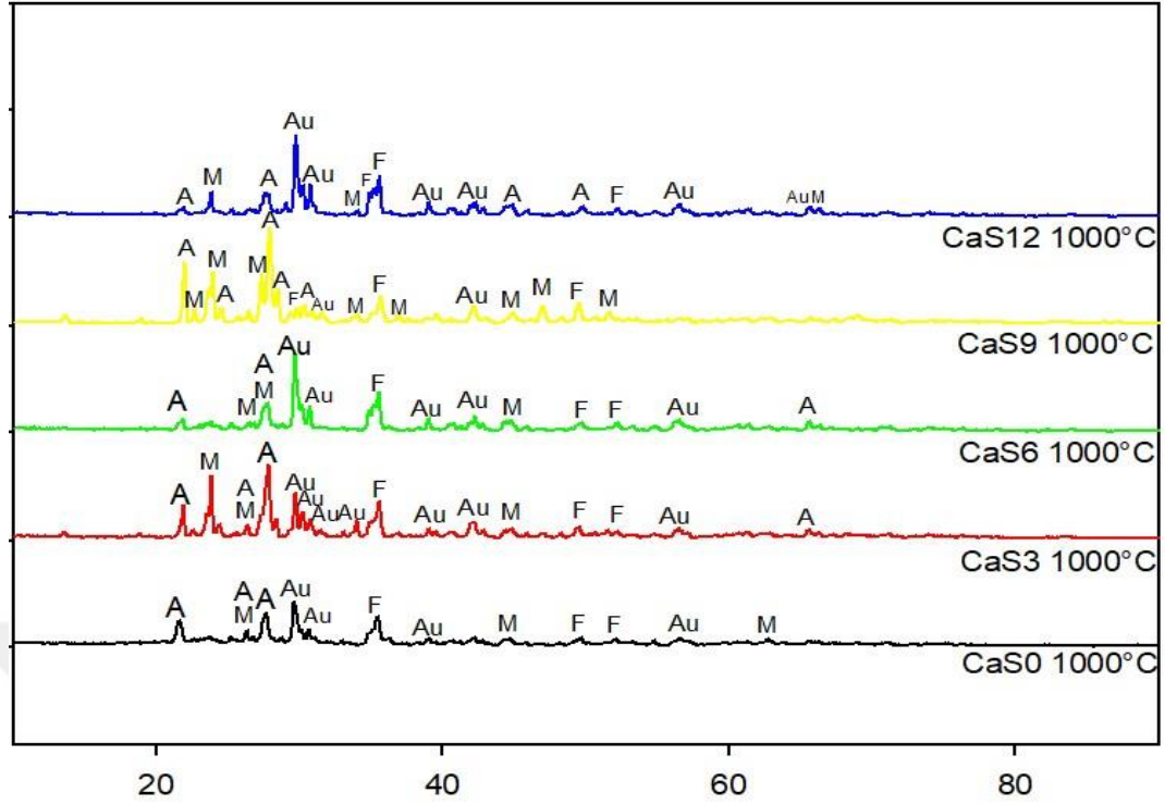
Şekil 6.20. Ağırlıkça beş farklı oranda ( %0, %3, %6, %9, %12) \text{CaF}_2 içeren 1000 °C’de sinterlenmiş numunelerin XRD grafiği.
