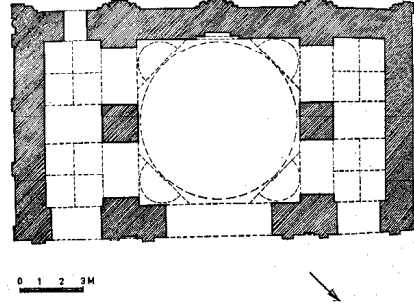
Şekil 1.3. Talhatan Baba Camii planı [55]
