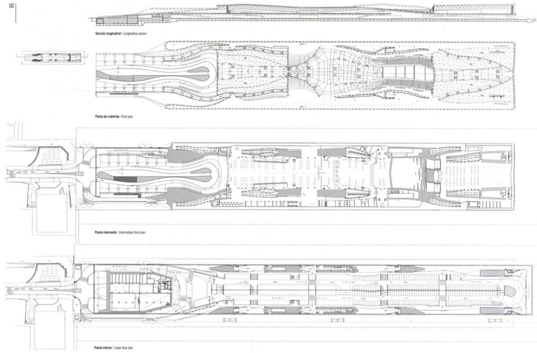
Şekil 4.10. Yokohama Terminali kesit ve kat planları [FOA, 2003]
