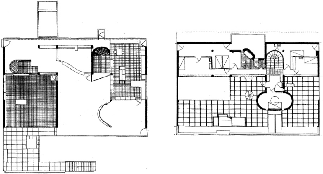
Şekil 2.16. Corbusier, Stein Villası, zemin ve birinci kat planları [Rowe,1977]
