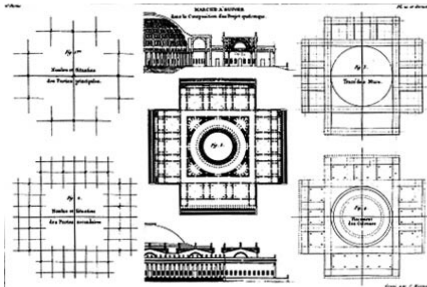
Şekil 2.6. Herhangibi bir projenin oluşturulmasında izlenen yol, J. N. L. Durand, Marche à suivre dans la composition d'un Project quelconque , Précis, 1813 [Madrazo, 1984].
