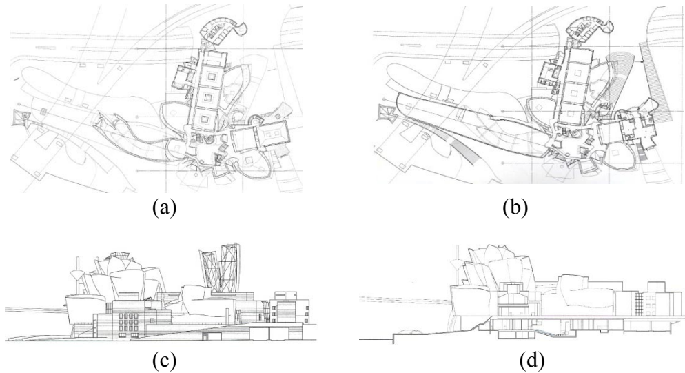
Şekil 4.14. Guggenheim Müzesi çizimleri
