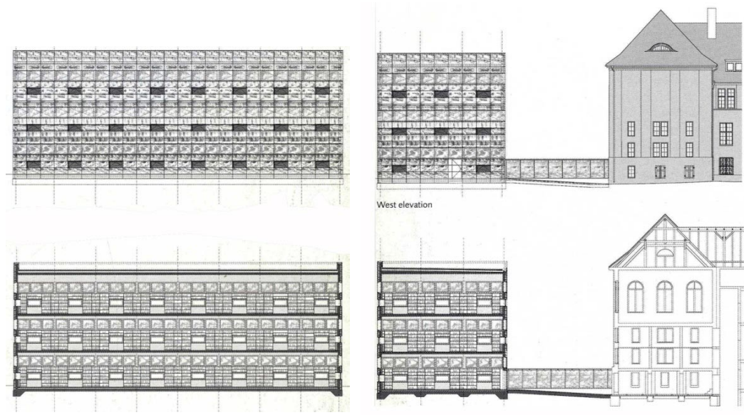
Şekil 4.18. Eberswalde kütüphanesi çizimleri
