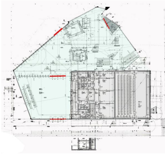
Şekil 4.4. UFA sineması, kristal ve düzlemsel bölüm ayrışması.
