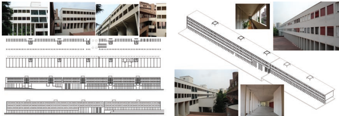
(a) (b) Resim 2.12. Gallarate Projesi, a. Görünüş ve planlar [Yılman, 2010] b. Görünüş ve cephe çizimleri [Yılman, 2010]
