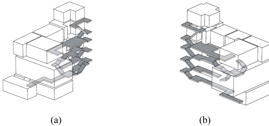
Şekil 2.13. Loos Müller Evi sirkülasyon ve hacim ilişkisi [Besser, Liebscher, 2010] a. Düşey sirkülasyon b. Düşey sirkülasyon
