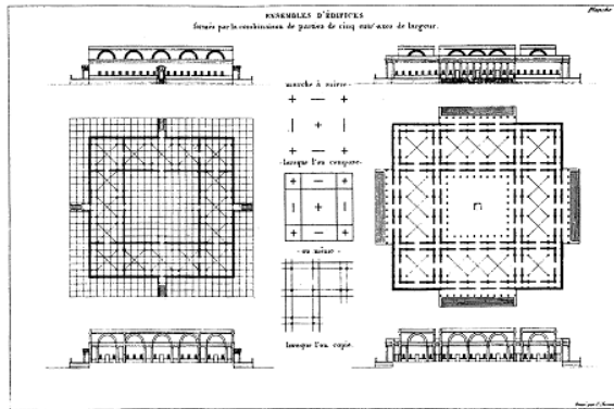
Şekil 2.9. Yapı Kompleksleri, J. N. L. Durand, Ensembles d'édifices , Partie Graphique, 1821 [Madrado, 1984].
