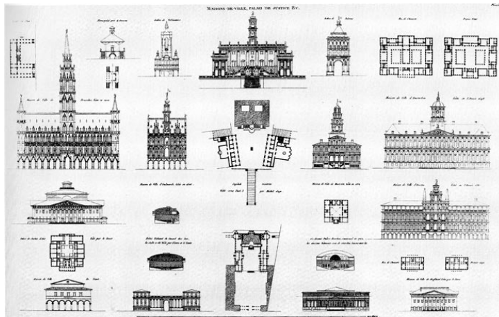
Şekil 2.3. Fonksiyonel yapılar, J. N. L. Durand, Recueil et Parallèle des édifices , 1801 [Durand, 1801].
