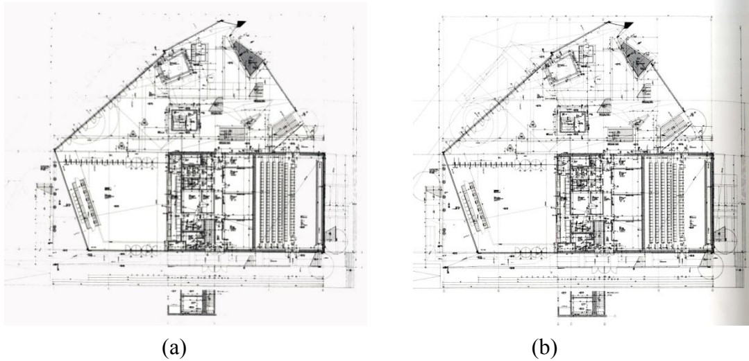
Şekil 4.5. UFA Sineması Planları
