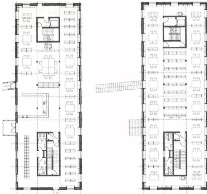
Şekil 4.16. Eberswalde Kütüphanesi, zemin kat ve birinci kat planları [Mack, 2000]
