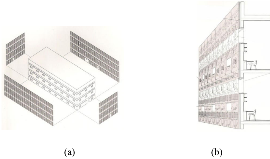
Şekil 4.17. Eberswalde Kütüphanesi, Kaplamanın strüktürel özellikleri ve biçim dili a. Yüzey konstrüksiyonu ve biçime eklenmesi [Moussavi, Kubo, 2008] b. Yüzey konstrüksiyon sistemi [Moussavi, Kubo, 2008]
