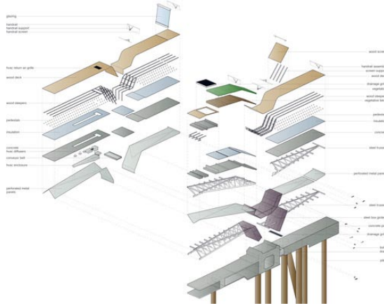
Şekil 4.11. Yokohama terminali zeminin katlanması ve onun strüktürel niteliği
