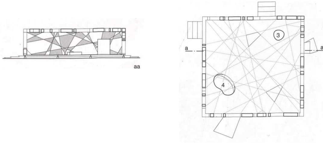
Şekil 4.27. Serpentine Galerisi kesit ve plan çizimleri [El Croquis, 2005]
