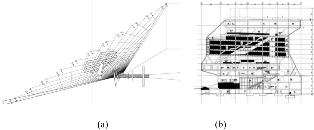
Şekil 4.24. Seattle Kütüphanesi yapısal ifadeler a. Yüzey konstrüksiyonu [Koolhaas, 2010] b. Kesit [Gargiani, 2008]
