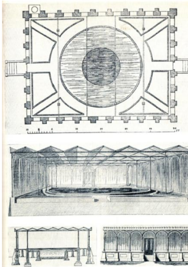
Şekil 2.10. Chatsworth'te yapılan nilüfer evinin planı, iç mekân perspektifi, kesiti ve cephesi [Chadwick, 1961]
