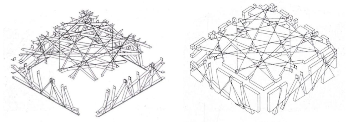
Şekil 4.29. Serpentine Galerisi Strüktürel Model ve kaplama Modeli
