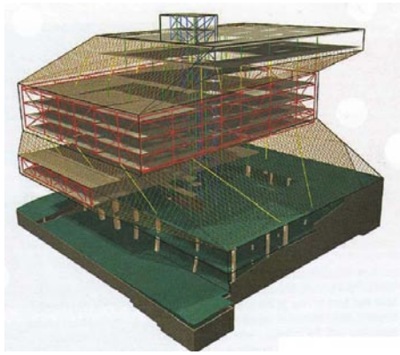
Resim 4.41. Seattle Kütüphanesi konstrüksiyon sistemi, güçlendirilmiş konsol döşemeler ve yüzeye yük aktarımı [Koolhaas, 2011]
