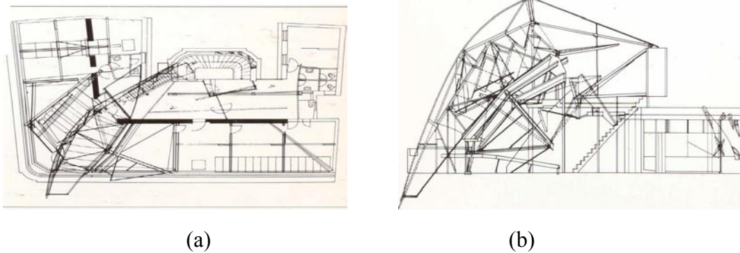
Şekil 4.2. Coop Himmelblau'nun çatısı a. Çatı planı [Papadakis, 1989] b. Çatı kesiti [Papadakis, 1989]
