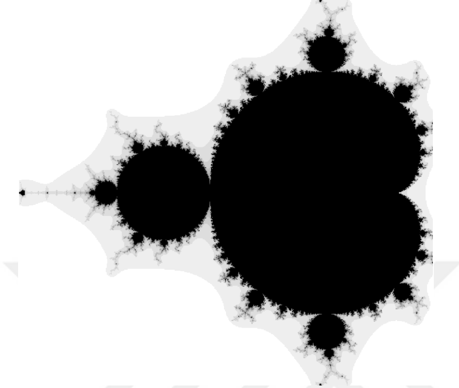
Şekil 14. Mandelbrot Set
