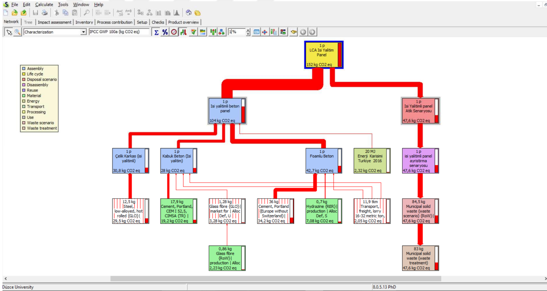
Şekil 5.2. Isı yalitimlı panelin küresel ısınma etki ağacı (kg CO 2 eq).
