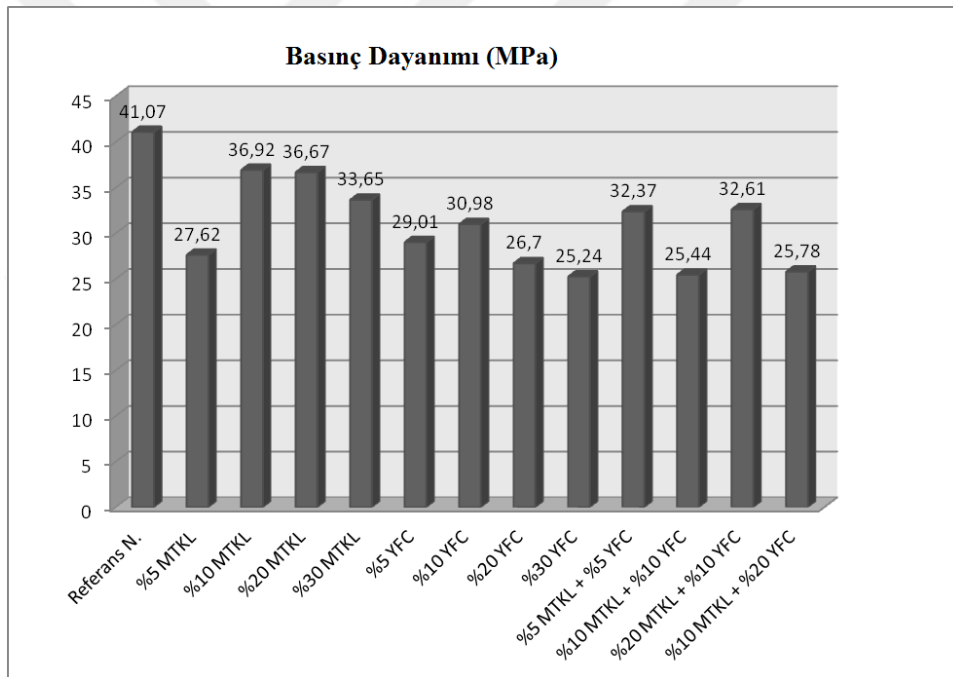
Şekil 6.2. Katkılı betonların basınç dayanımları [173].
