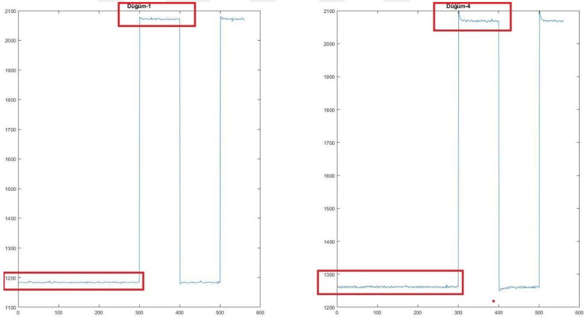
Şekil 5.4 5 Kbps Veri Hızı İçin Düğüm-1 ve Düğüm-4 CAN-L Sinyal Sapması
