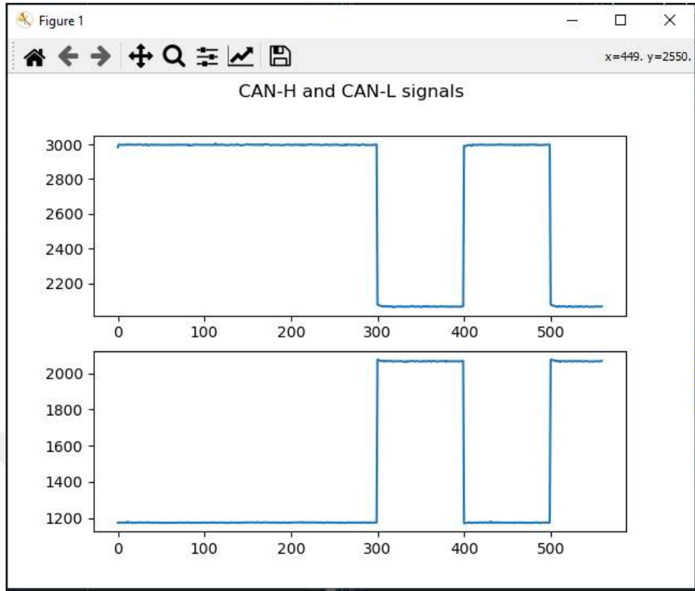
Şekil 4.45 CAN Düğümünden Python ile Alınan Veri Örneği
