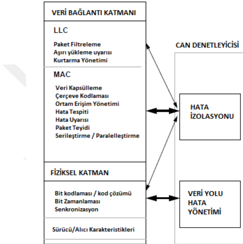
Şekil 3.2. CAN OSI modeline göre katmanları [1]
