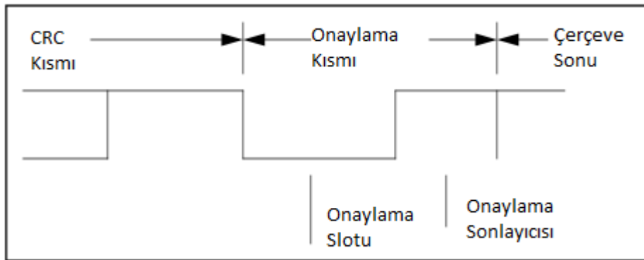
Şekil 3.13 CAN Çerçevesi Onaylama (ACK) Kısım [1]
