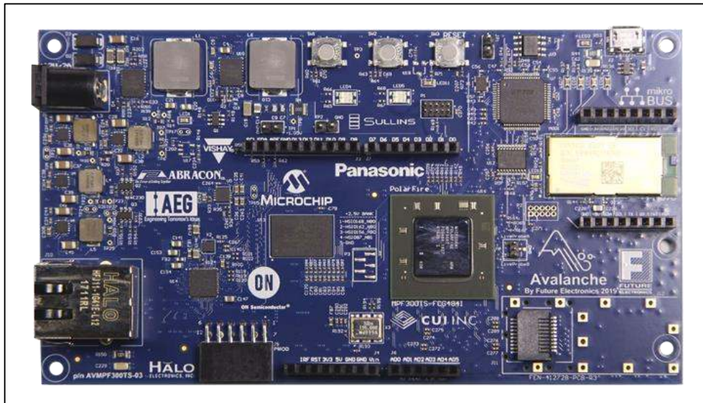
Şekil 4.2 Avalanche Geliştirme Kartı [34]
