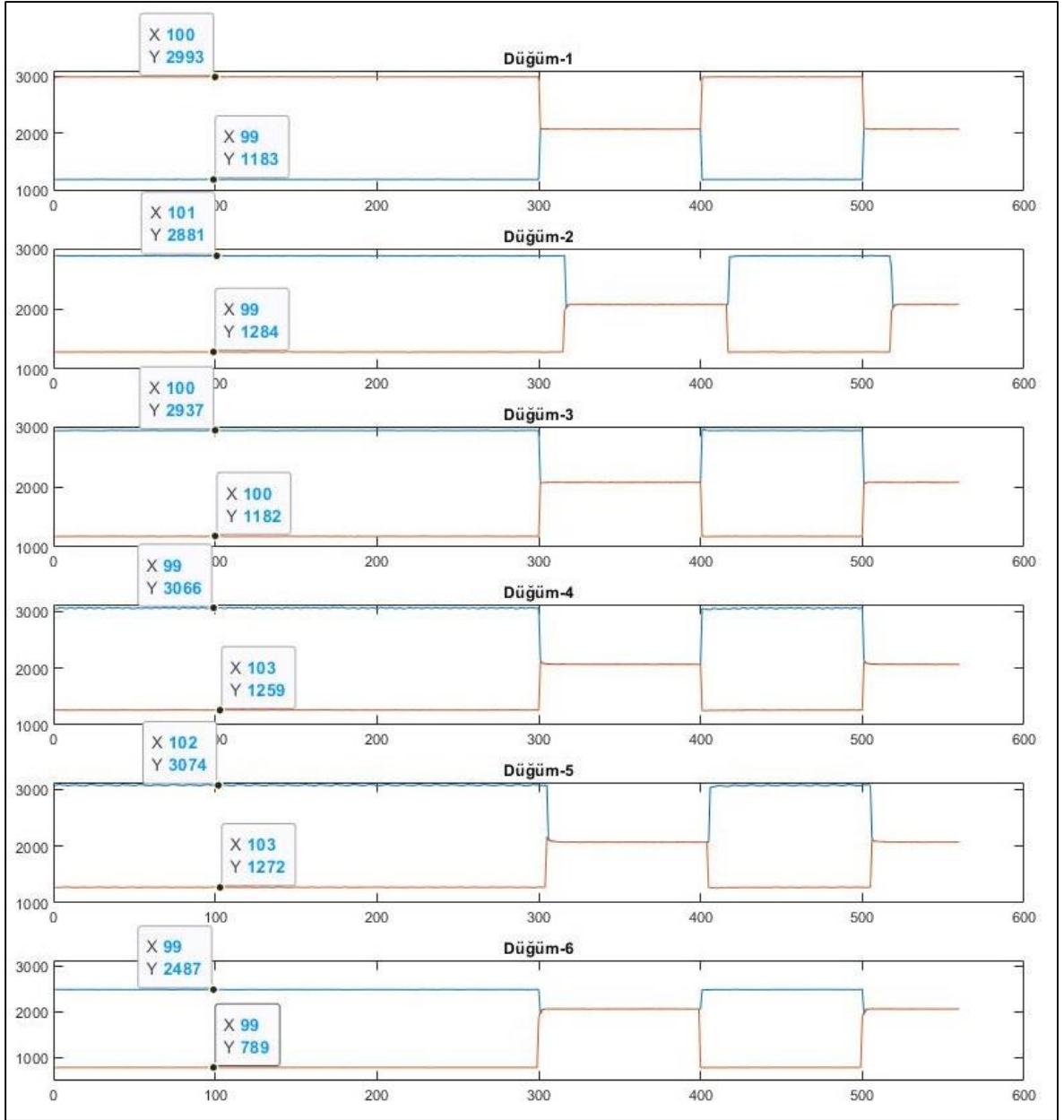
 ekil 5.2 CAN D ğ mleri Sinyal Maksimum ve Minimum Değerleri
