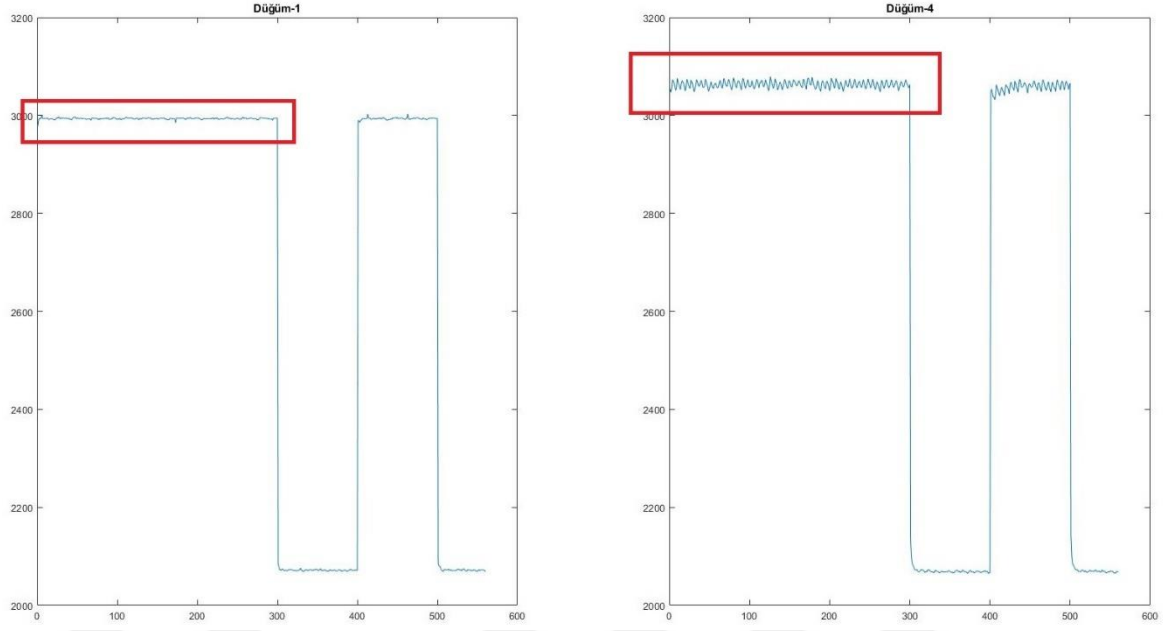
Şekil 5.3 5 Kbps Veri Hızı İçin Düğüm-1 ve Düğüm-4 CAN-H Sinyal Sapması
