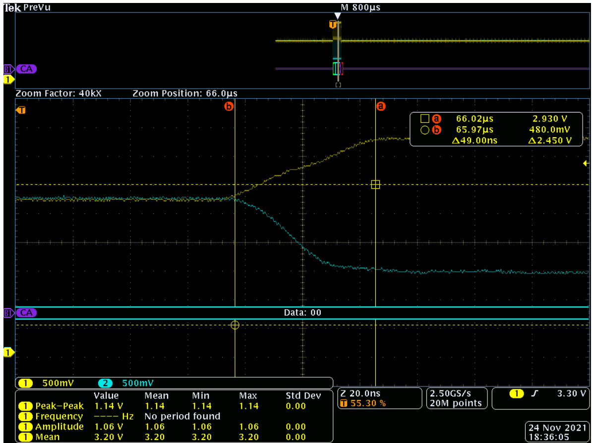
Şekil 4.12 SVN65HVD CAN Alıcı-Verici Sinyal Kalkış İniş Süresi
