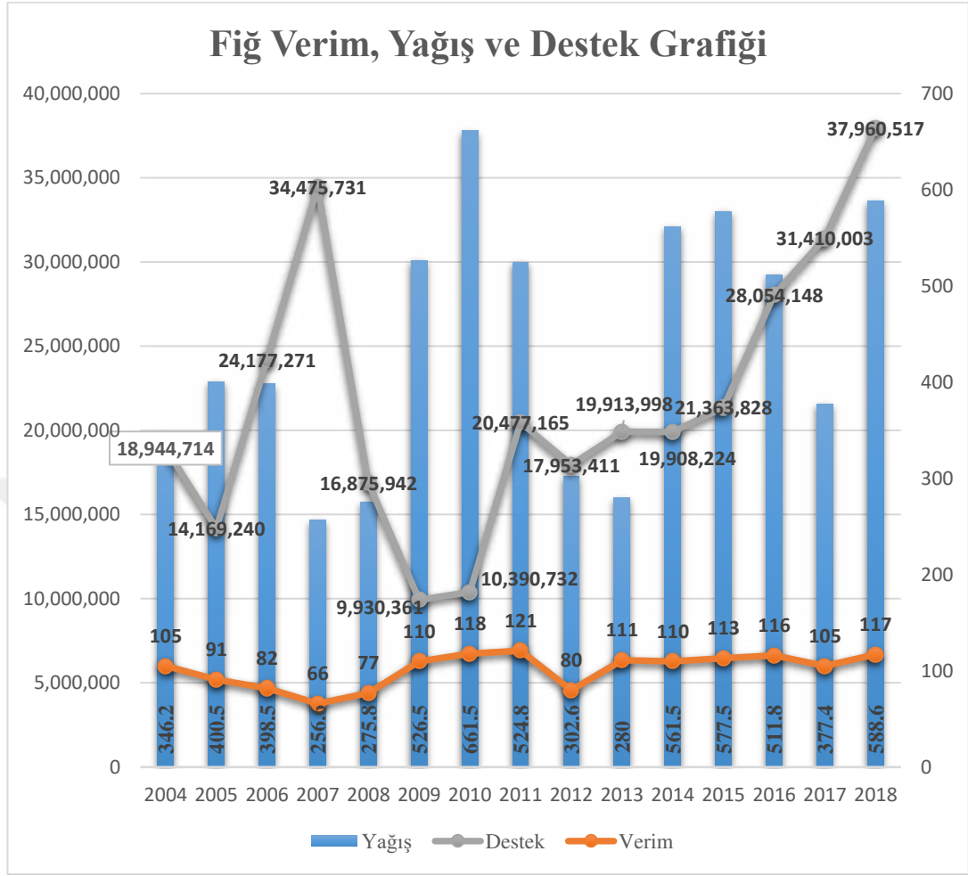
Şekil 10.2: Çankırı fiğ yağış, verim ve destekleme grafiği
