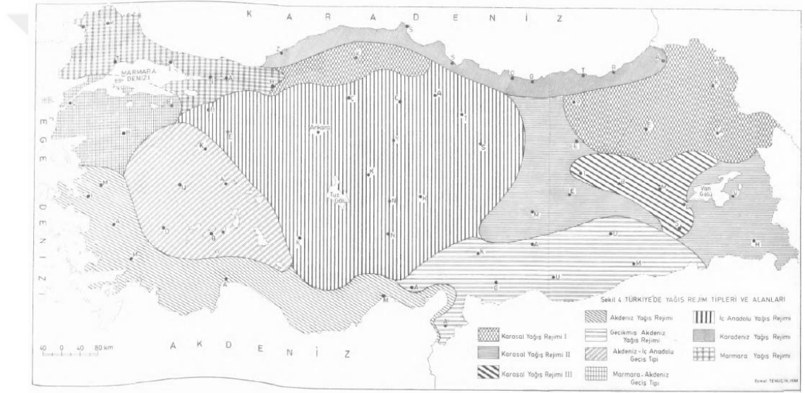
Şekil 2.11: Türkiye yağış rejimi tipleri ve alanları
