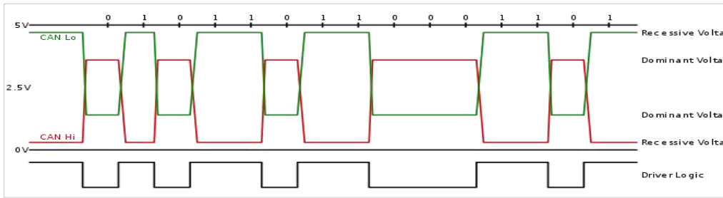
Şekil 6 Düşük Hızlı CAN Sinyali. ISO 11898-3
