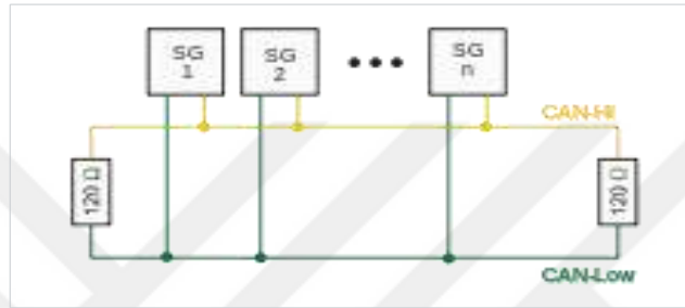
Şekil 10 Sonlandırıcı dirençli CAN bus elektriksel bağlantı örnek topolojisi
