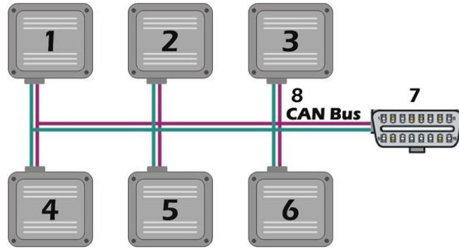
Şekil 2 CAN sisteminin basitleştirilmiş şematik diyagramını ve CAN veri yoluna bağlanabilecek olası ünitelerin / cihazların (ECU-Electronic Kontrol Üniteleri), bazılarını göstermektedir.
