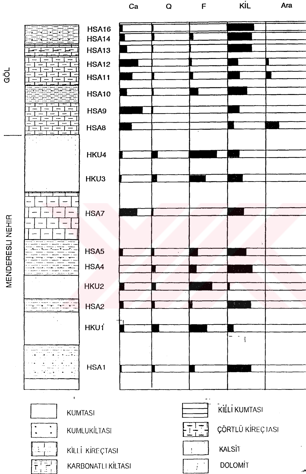
Şekil 4.25. Hacısam Kesitinde belirlenen minerallerin XRD-TK dikey dağılımları
