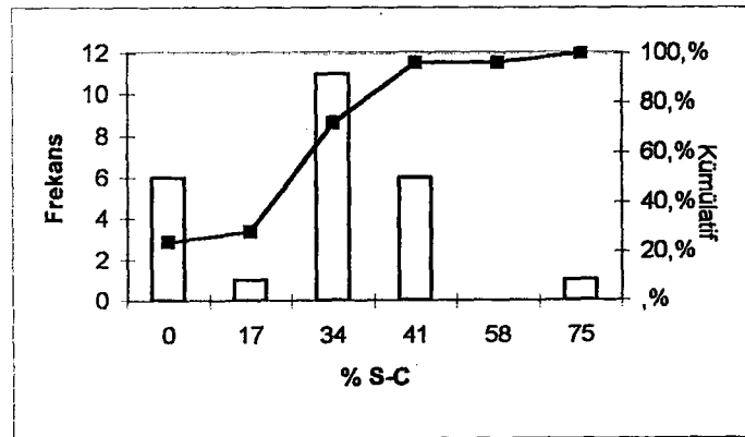
Şekil 6.3. örneklerin XRD-KF sıklık dağılımları
