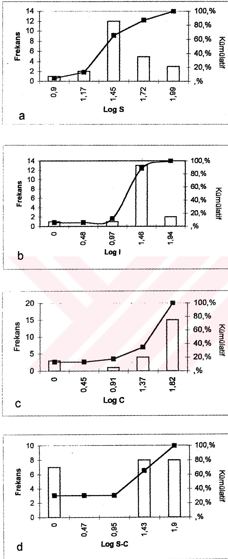
Şekil 6.4. Örneklerin XRD-KF logaritmik dağılımları
