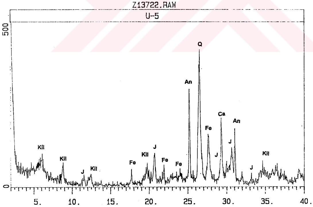
Şekil 4.18 Anhidritli kilitaşı örneğinin X ışınları kırınım profili F:Feldispat J:Jips Ca:Kalsit An:anhidrit Q:Kuvars Örnek No:U5
