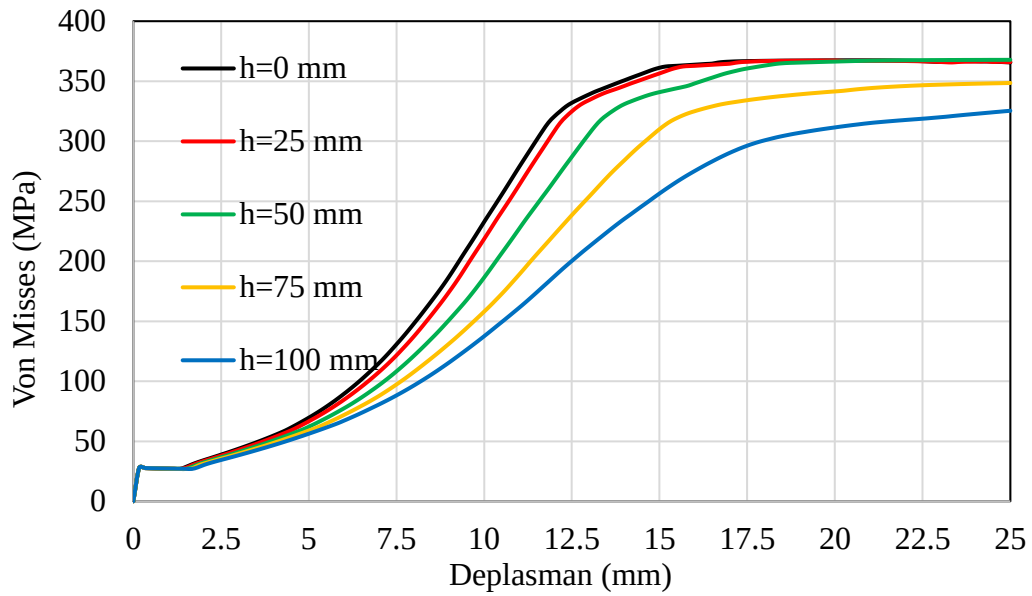
Şekil 6.93. Kolon taban levhasının üst kısmında kullanılan somunlarda gerilme-deplasman parametrelerinin kıyaslanmasıyla elde edilen analiz sonuçları (model 3)
