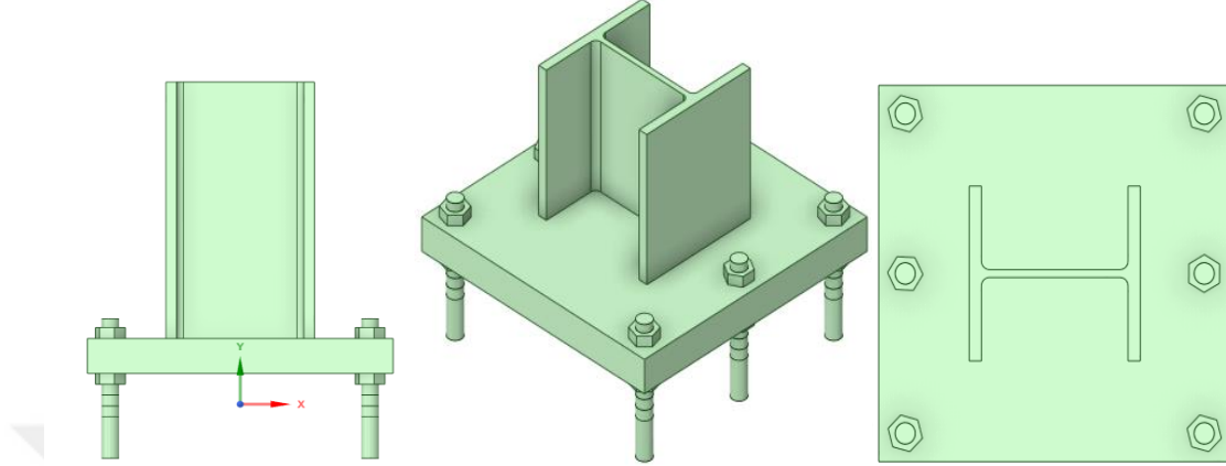
Şekil 5.3. Çelik kolon ayak-temel birleşimine ait 6 adet ankraj bulonlu model-3
