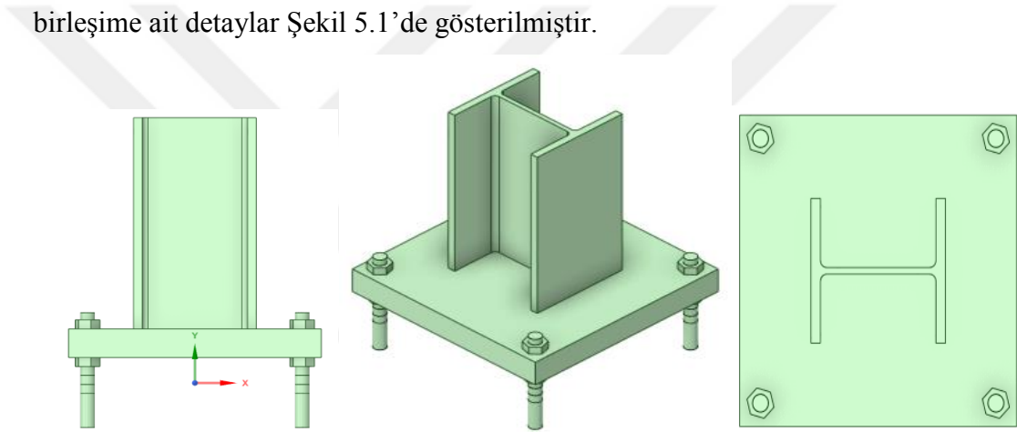
Şekil 5.1. Çelik kolon ayak-temel birleşimine ait 4 adet ankraj bulonlu model-1
