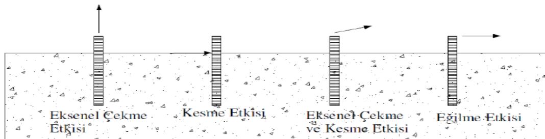
Şekil 3.6. Ankrajlarda Oluşan Farklı Yüklemeler [25]
