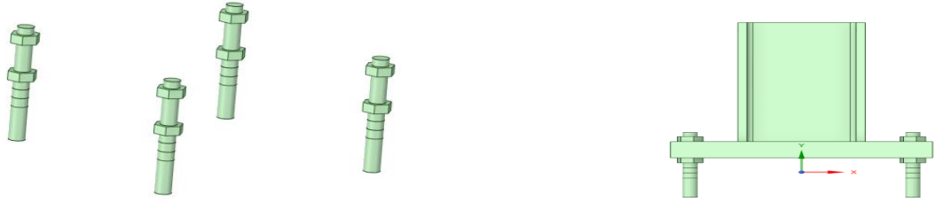
Şekil 5.10. Bulonların görünümüne ait kesit görünüşü (model-1)
