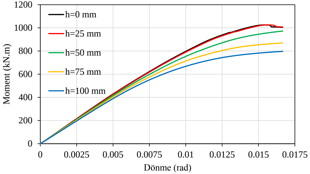
Şekil 6.90. Moment-dönme parametrelerinin kıyaslanmasıyla elde edilen analiz sonuçları (model 3)
