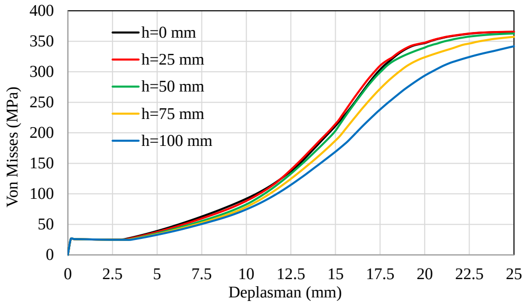
Şekil 6.88. Kolon taban levhasının üst kısmında kullanılan somunlarda gerilme-deplasman parametrelerinin kıyaslanmasıyla elde edilen analiz sonuçları (model 2)
