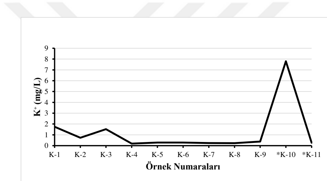
Şekil 4.25. İnceleme alanındaki suların K + iyon konsantrasyonları
