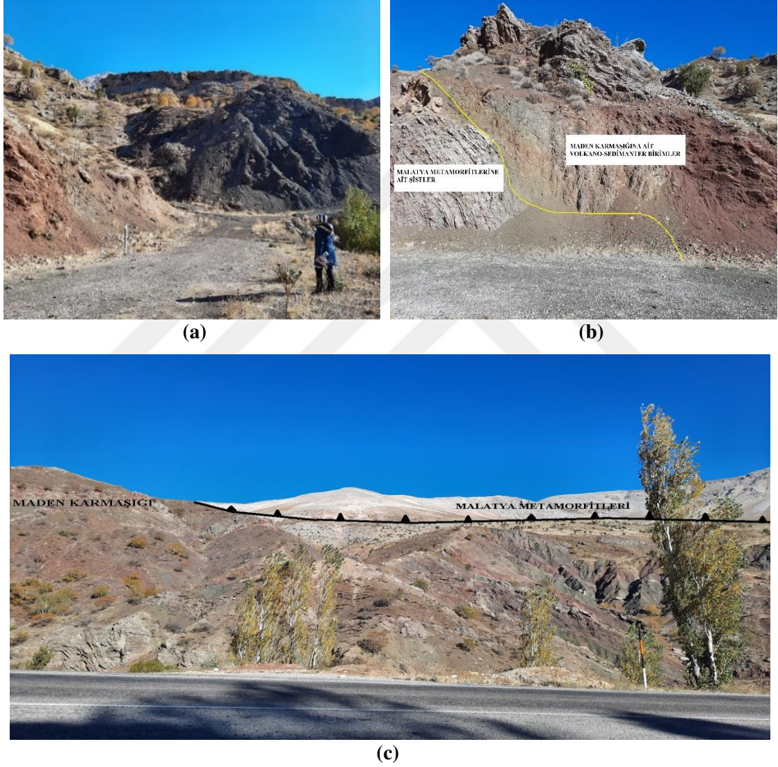
Şekil 3.5. (a) Maden Karmaşığı'na ait volkano-sedimanter birimler (37S436715D-4204621K), (b) Maden Karmaşığı ile Malatya Metamorfitleeri arasındaki stratigrafik ilişki (37S436715D-4204621K), (c) Maden Karmaşığı ile Malatya Metamorfitleeri arasındaki tektonik ilişki (37S436288D-4204473K, rakım 1207)
