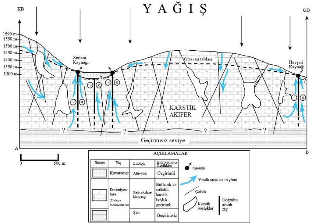
Şekil 4.5. Zerban Kaynağı ile Havşarı Kaynağı'nın oluşumunu gösteren şematik hidrojeoloji kesiti (kesit izi jeolojik haritası üzerinde gösterilmiştir).
