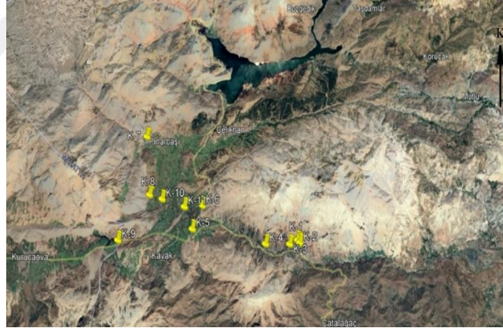
Şekil 2.1. Su örnekleme lokasyonları (Ölçeksiz)
