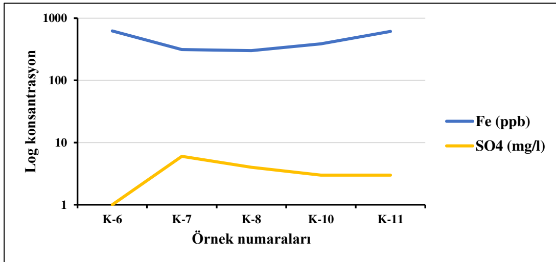
Şekil 4.35. İncelenen sularda Fe ve SO_4^{2-} konsantrasyonları arasındaki ilişki
