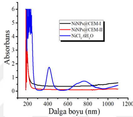
Şekil 4.2. \text{NaBH}_4 'ün katalitik metanolizinden elde edilen \text{NiNPs}@ \text{CEM-n} ve saf \text{NiCl}_2 \cdot 6\text{H}_2\text{O} tuzunun UV-vis spektrumları
