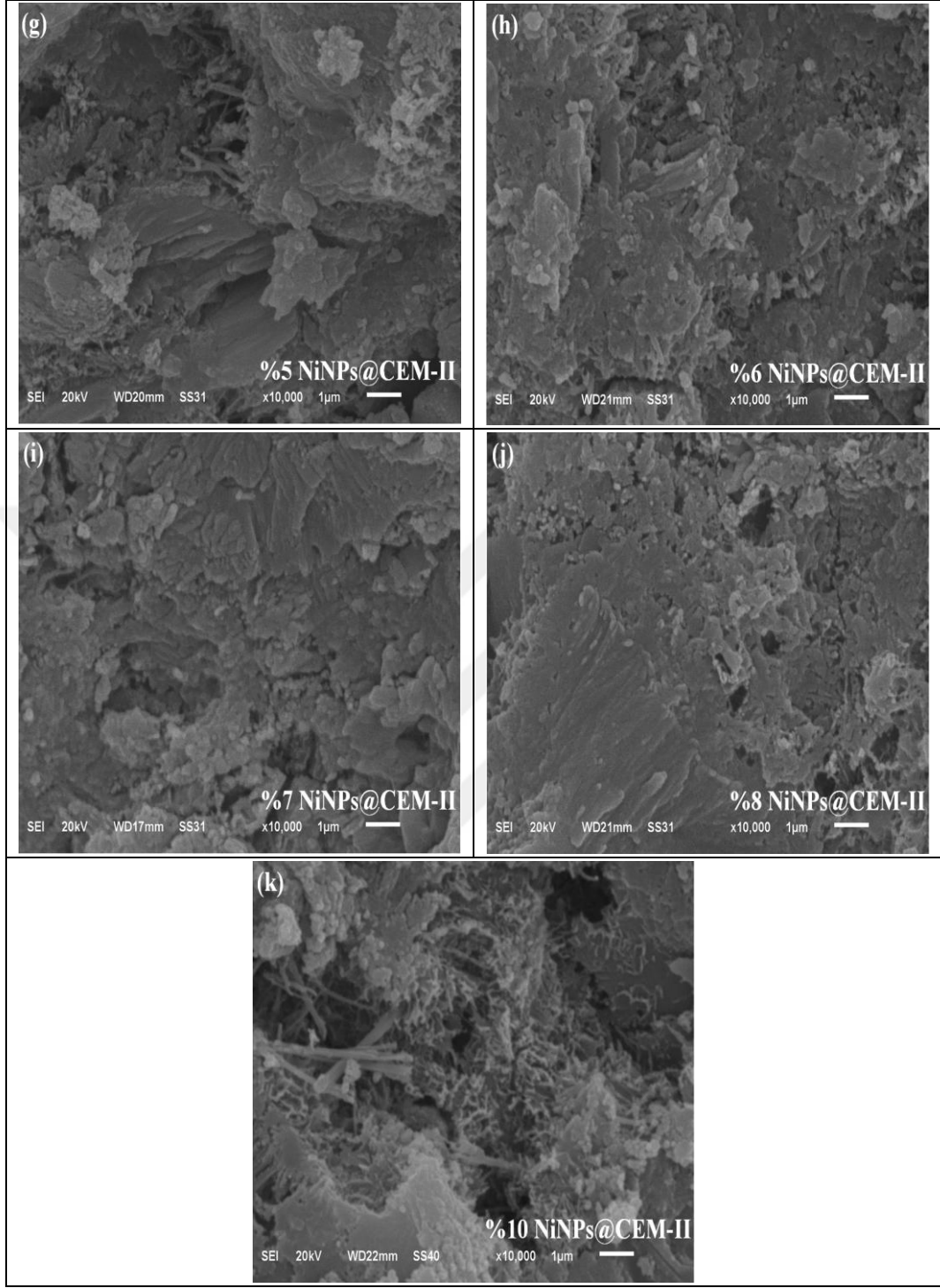
Şekil 4.21. (a) (a) Kontrol CEM-II numunesi (%100 çimento), (b) NaBH 4 -CEM-II (metalsız), (c) %1,0, (d) %2,0, (e) %3,0, (f) %4,0, (g) %5,0, (h) %6,0, (i) %7,0, (j) %8,0 ve (k) %10 NiNPs@CEM-II'i içeren kırık beton numunelerinin x10,0 K büyütmede 1 μm ölçekli SEM mikrografları
