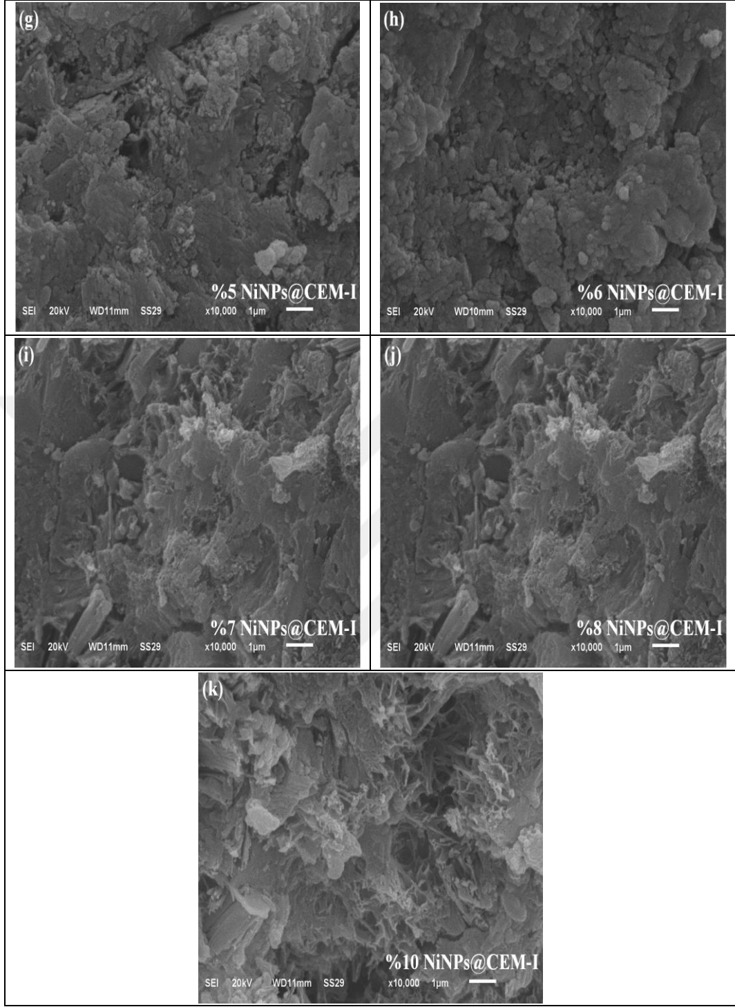
Şekil 4.20. (a) Kontrol CEM-I numunesi (%100 çimento), (b) NaBH 4 -CEM-I (metalsız), (c) %1,0, (d) %2,0, (e) %3,0, (f) %4,0, (g) %5,0, (h) %6,0, (i) %7,0, (j) %8,0 ve (k) %10 NiNPs@CEM-I'ı içeren kırık beton numunelerinin x 10,0 K büyütmede 1 µm ölçekli SEM mikrografları
