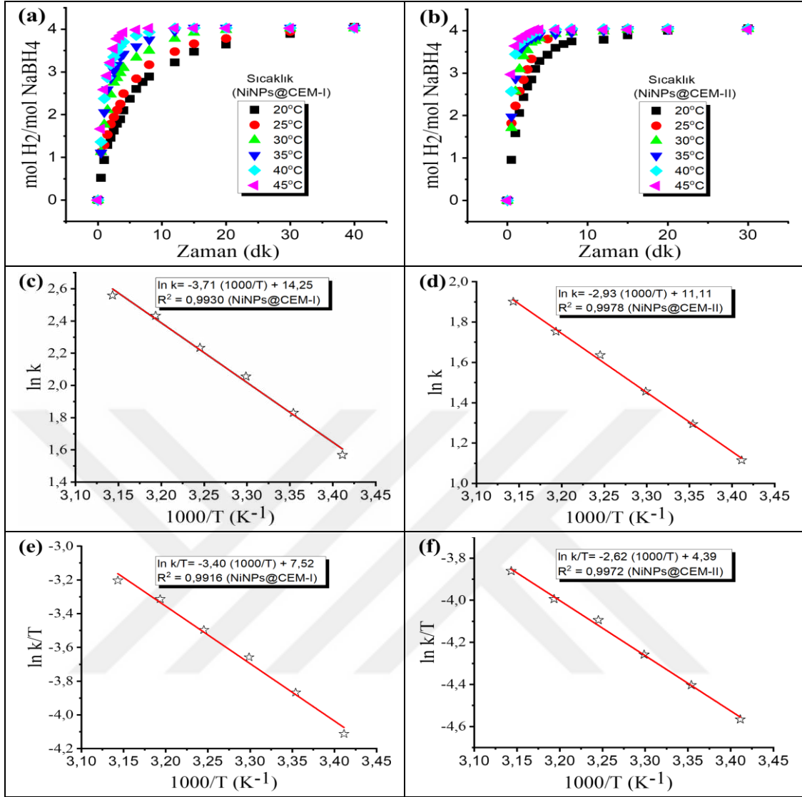
Şekil 4.13. Farklı sıcaklıklarda (20-45°C) (a) NiNPs@CEM-I ve (b) NiNPs@CEM-II tarafından katalizlenen NaBH_4 'ün metanolizi için zamana karşı mol H_2 /mol NaBH_4 grafiği, (c) NiNPs@CEM-I ve (d) NiNPs@CEM-II için Arrhenius eğrisi, (e) NiNPs@CEM-I ve (f) NiNPs@CEM-II için Eyring eğrisi.
