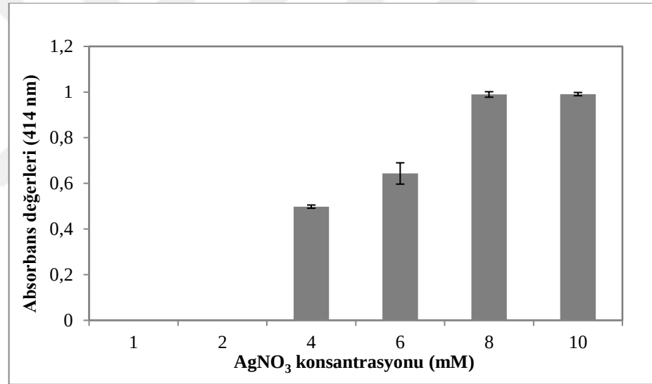
Şekil 4.9. Farklı konsantrasyonlarda (1,2,4,6,8,10 mM) \text{AgNO}_3 eklenen örneklerin 414 nm’de 48.saat sonunda ölçülen absorbans değerlerinin grafiği.
