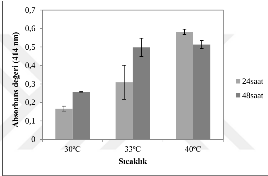
Şekil 4.3. Aynı konsantrasyonda AgNP içeren süpernatantların farklı sıcaklıklarda (30, 33 ve 40°C) 24 ve 48 saat sonundaki absorbens değerlerinin grafiği (Absorbans değerleri 1/10 oranında seyreltilmiş örneklerde okunmuştur).
