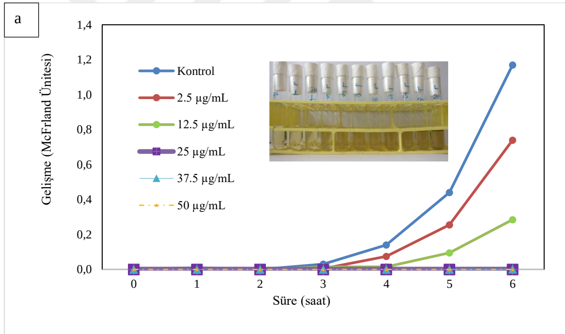
Şekil 4.13. Bazı patojen bakterilerin farklı konsantrasyonlarda (0-50 \mu\text{g/mL} ) 6 saatlik gelişme grafiği a) L. monocytogenes b) P. aeruginosa c) S. Typhimurium .
