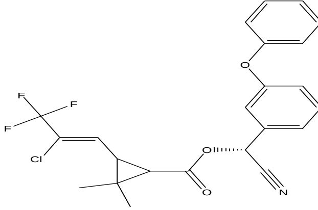
Şekil 2.5. Lambda-cyhalothrin'in moleküler yapısı
