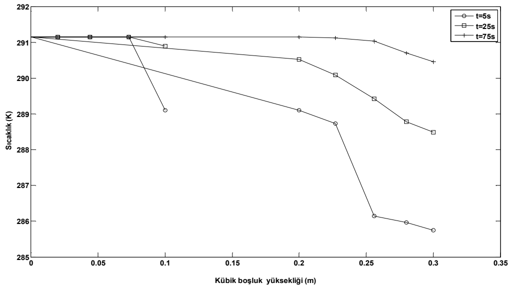
Şekil 4.18. x/X=0 da sıcaklık değerlerinin kübik boşluk yüksekliğince değişimi
