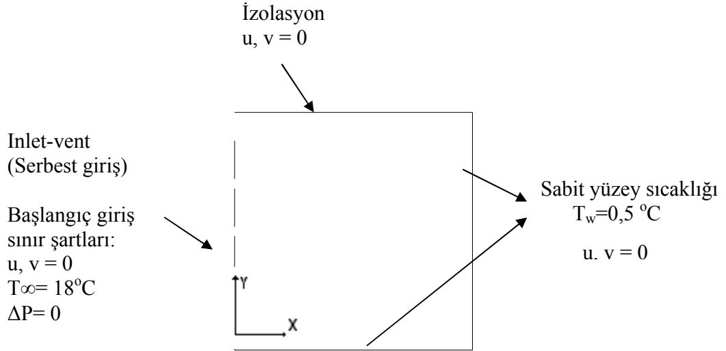
Şekil 3.39. Sayısal çözüm için uygulanan sınır ve başlangıç şartları
