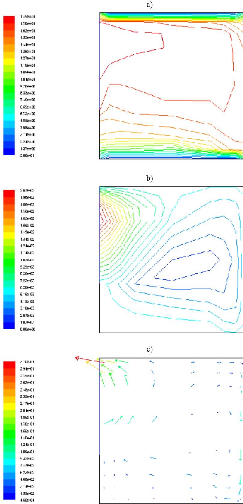
Şekil 4.181. t=250 . s için kübik boşluk içerisindeki eşdeğer eğrilerin dağılımı a) sıcaklık, b) akım fonksiyonu, c) hız vektörleri
