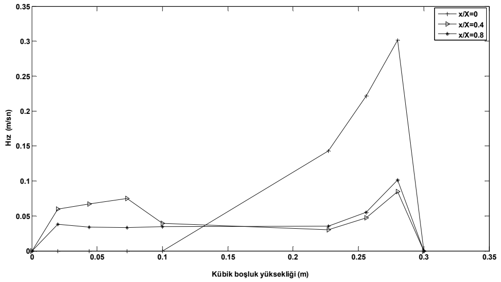
Şekil 4.151. t=130 s için kübik boşluk içerisindeki bileşke hız değerlerinin kübik boşluk yüksekliğince değişimi
