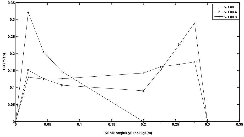
Şekil 4.131. t=100 s için kübik boşluk içerisindeki bileşke hız değerlerinin kübik boşluk yüksekliğince değişimi
