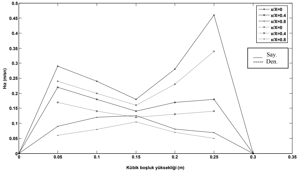
Şekil 3.61. t=65 s için kübik boşluk içerisindeki deneysel ve sayısal bileşke hız değerlerinin kübik boşluk yüksekliğince değişimi
