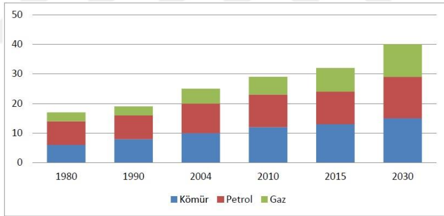
řekil 2.3. D nya'da Yakıt T rlerine G re Karbondioksit Salınımı (Milyon Ton)
