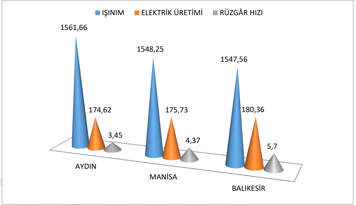
Şekil 4.1. Aydın, Manisa ve Balıkesir illeri için sabit açı değerlerinde gelen yıllık ışıınım ( \text{kW/m}^2 ), üretilen elektrik ( \text{kW/m}^2 ) ve yıllık ortalama hız ( \text{m/s} ) değerleri
