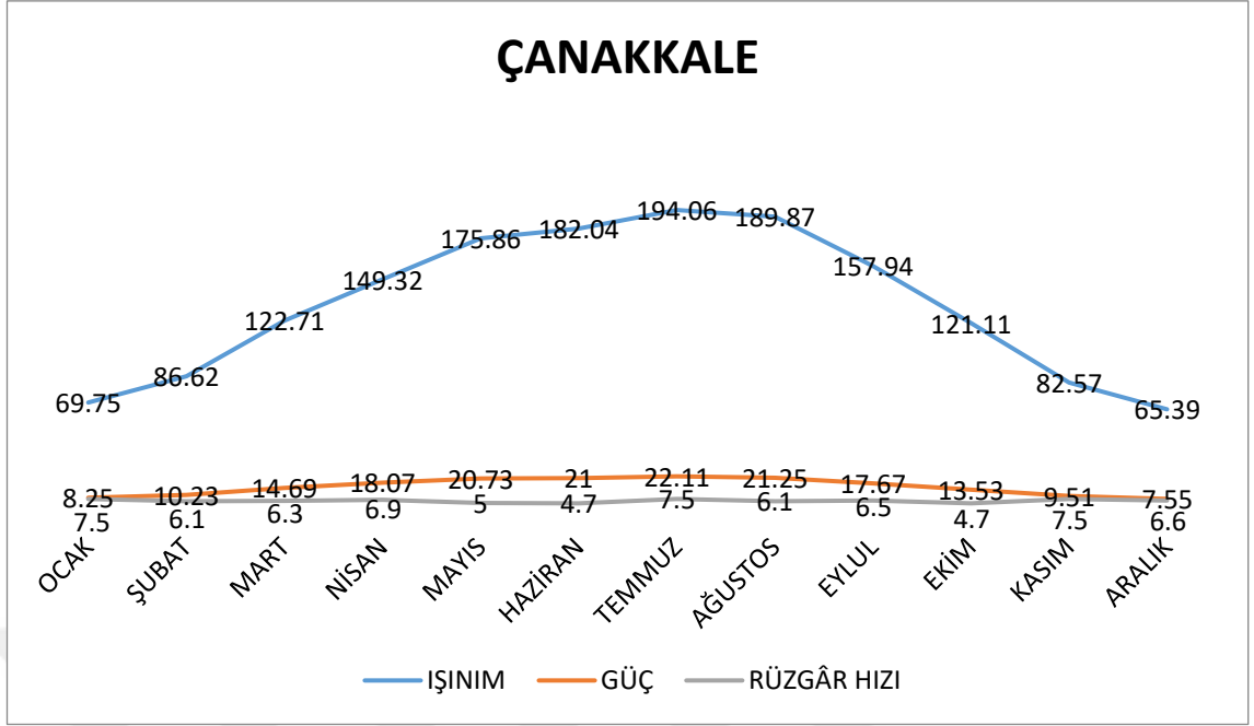
Şekil 4.6. Çanakkale ili için sabit açı değerlerinde gelen aylık ışıınım ( \text{kW/m}^2 ), üretilen elektrik ( \text{kW/m}^2 ) ve aylık ortalama hız ( \text{m/s} ) değerleri
