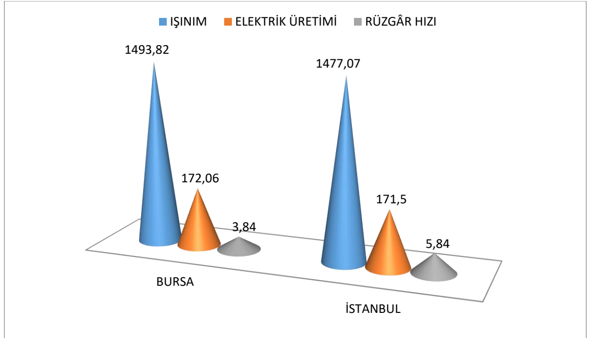
Şekil 4.4. Bursa ve İstanbul illeri için sabit açı değerlerinde gelen yıllık ışıınım ( \text{kW/m}^2 ), üretilen elektrik ( \text{kW/m}^2 ) ve yıllık ortalama hız (m/s) değerleri
