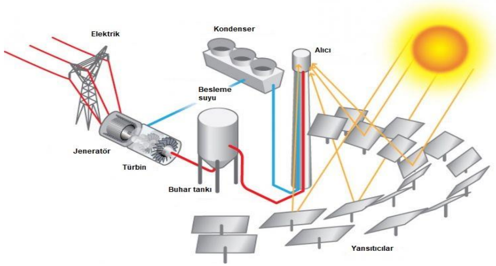
Şekil2.3. Merkezi alıcı sistemli güç santrali (www.yegm.gov.tr)
