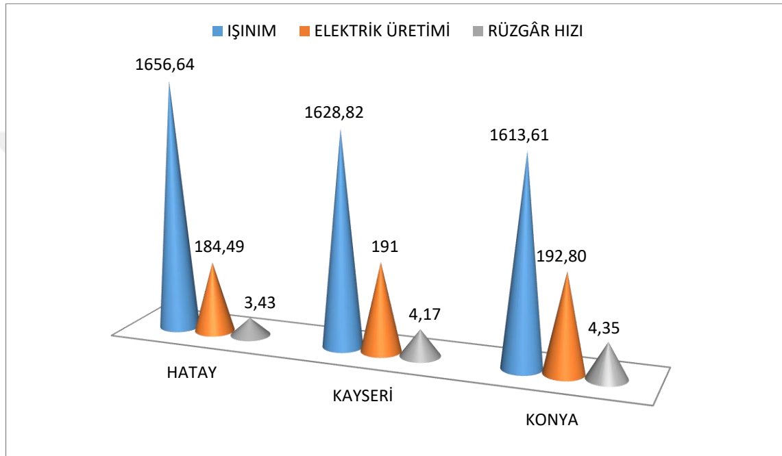
Şekil 4.2. Hatay, Kayseri ve Konya illeri için sabit aç değelerinde gelen yıllık ışıını ( \text{kW/m}^2 ), üretilen elektrik ( \text{kW/m}^2 ), ve yıllık ortalama hız ( \text{m/s} ) değeleri
