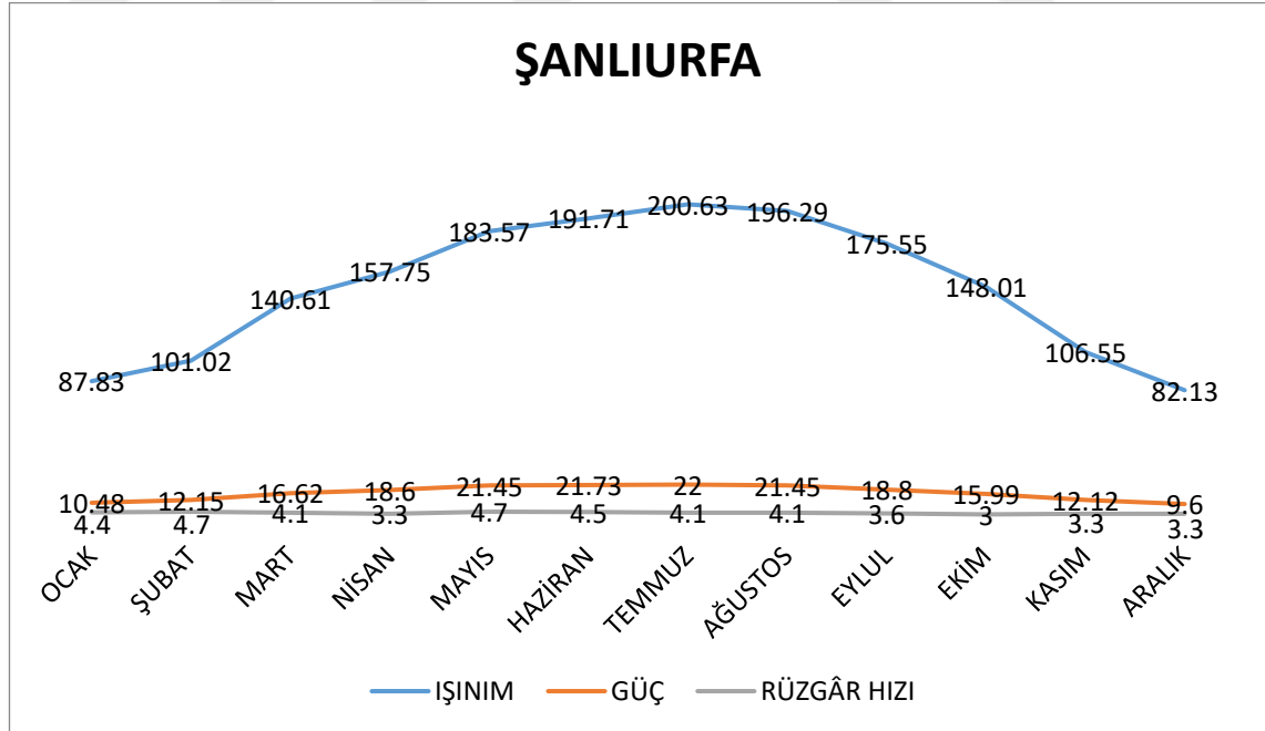
Şekil 4.5. Şanlıurfa ili için sabit aç değerlerinde gelen aylık ışıınım (kW/m 2 ), üretilen elektrik (kW/m 2 ) ve aylık ortalama hız (m/s) değerleri
