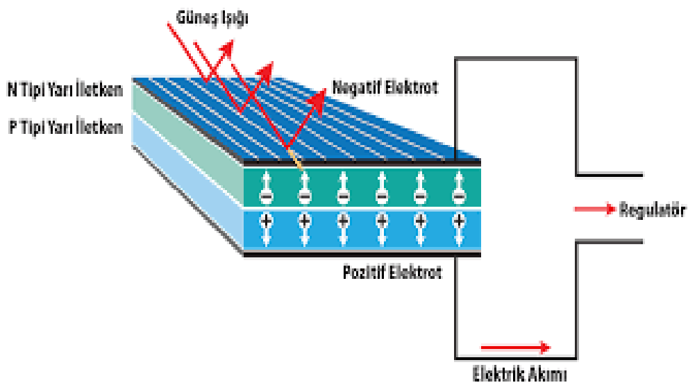
řekil2.7. Güneř pillerinin yapısı (www.antalyaenerji.com)
