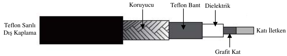
Şekil 3.7. 003A20 Model kablo iç yapısı
