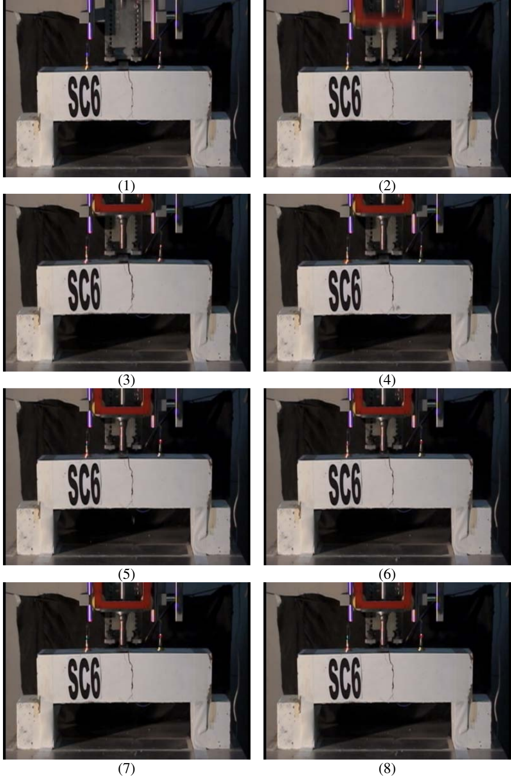
Resim 5.24. SC6 Deney elemanı göçme durumu
