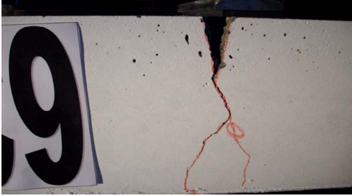
Resim 5.34. SC9 Elemanının göçme durumu
