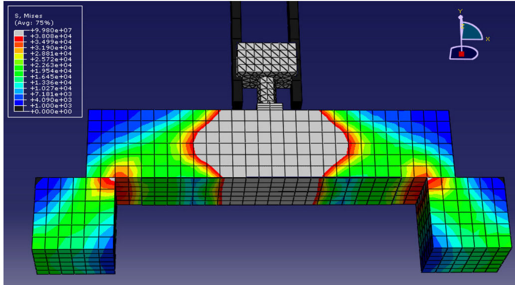
Şekil 6.20. 600 mm için Abaqus gerilme dağılımı
