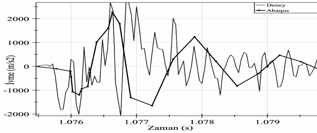
Şekil 6.47. SC9 Deney ile Abaqus ilk çarpma anı ivme değerleri karşılaştırılması
