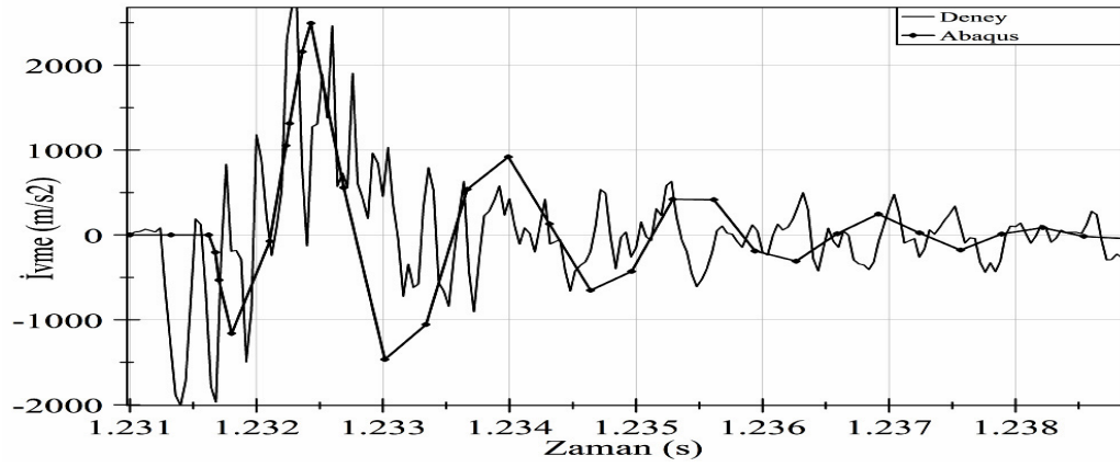
Şekil 6.37. SC7 Deney ile Abaqus ilk çarpma anı ivme değerleri karşılaştırılması
