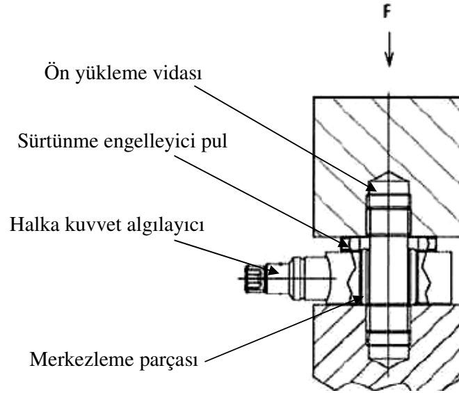
Şekil 3.6. Halka kuvvet algılayıcısı montaj şekli
