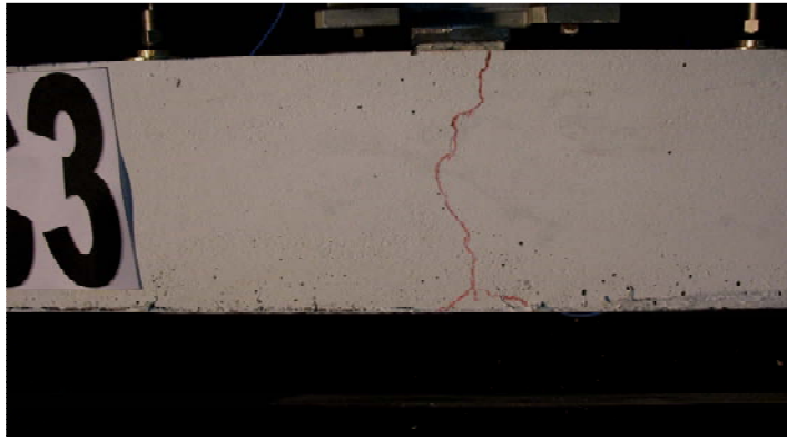
Resim 5.9. SC3 Elemanında oluşan ilk hasar
