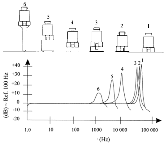
Şekil 3.5. İvmeölçerlerin montaj şekilleri ve yüksek frekansa etkileri 1. Vida ile 2. Yapıştırıcı ile 3. Montaj pedi ile 4. Düz mıknatıs ile 5. Çift taraflı mıknatıs ile 6. El çubuğu ile(Manual)
