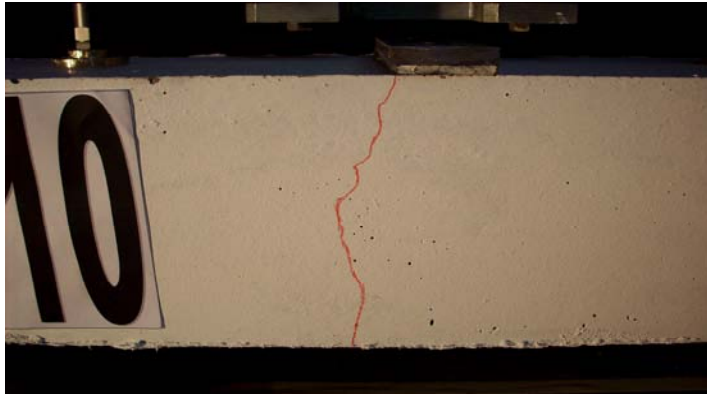
Resim 5.37. SC10 Elemanında oluşan ilk hasar
