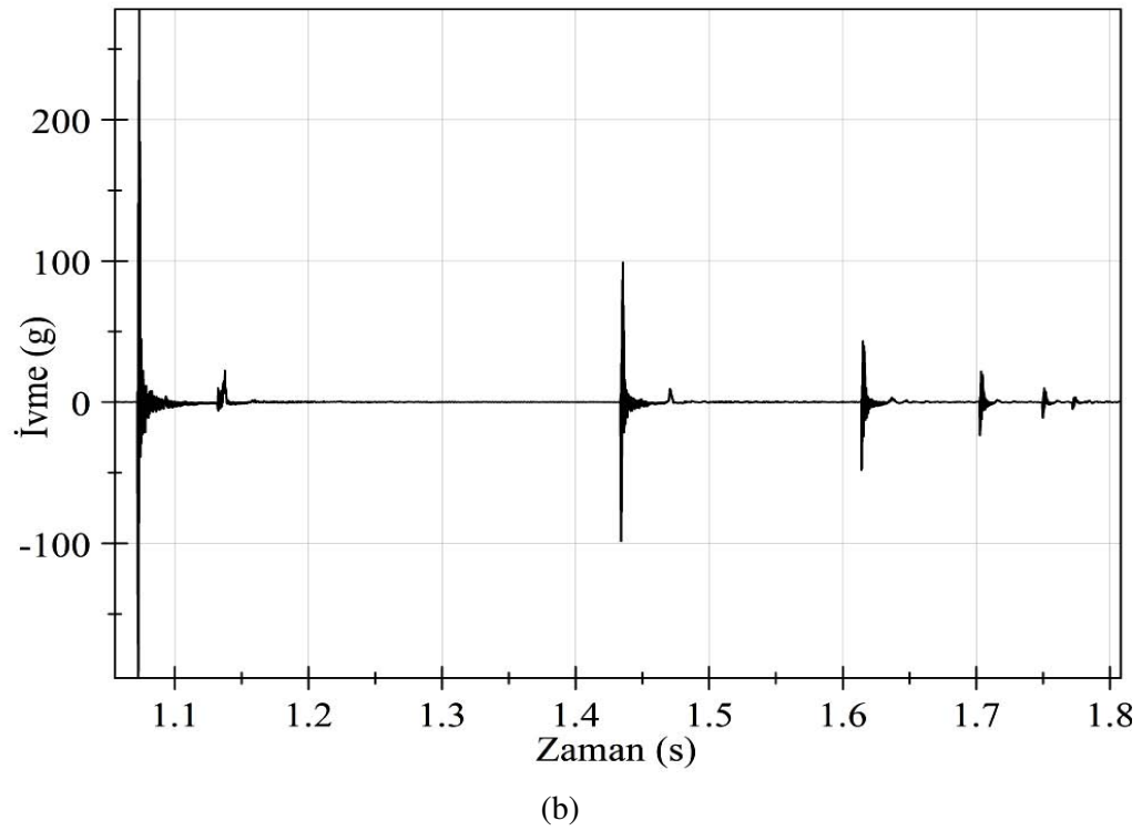
Şekil 5.1. SC1 Deney elemanının 1. düşme(hasarsız) ivme-zaman grafikleri a) Sol ivmeölçer b) Sağ ivmeölçer
