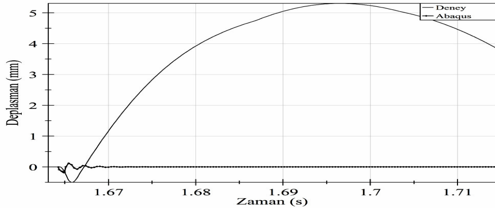
Şekil 6.14. SC2 Deney ile Abaqus ilk çarpma anı deplasman değerleri karşılaştırılması
