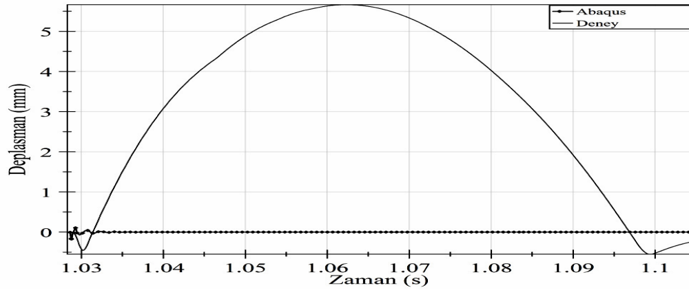
Şekil 6.19. SC3 Deney ile Abaqus ilk çarpma anı deplasman değerleri karşılaştırılması
