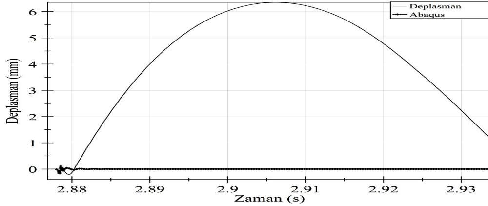
Şekil 6.54. SC10 Deney ile Abaqus ilk çarpma anı deplasman değerleri karşılaştırılması
