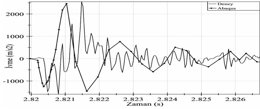
Şekil 6.22. SC4 Deney ile Abaqus ilk çarpma anı ivme değerleri karşılaştırılması
