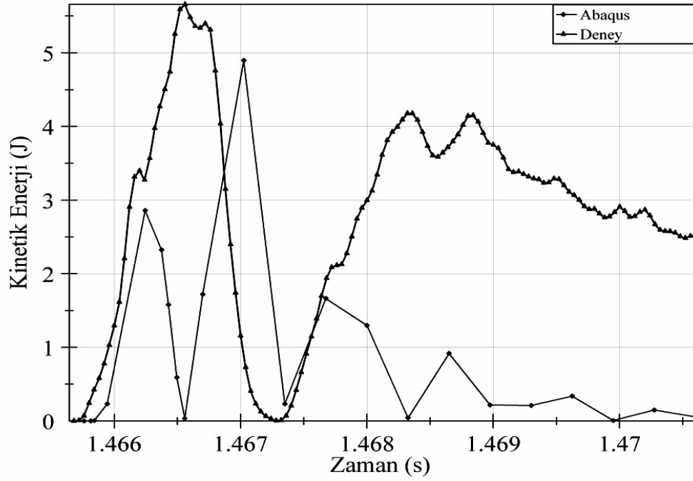
Şekil 6.63. Normal dayanımlı beton, 700 mm yükseklik için kinetik enerji değerleri karşılaştırması
