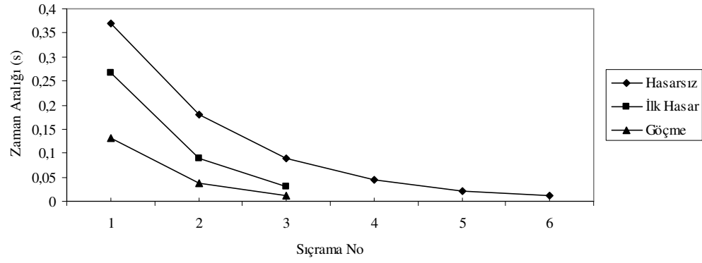
Şekil 5.53. SC2 Deney elemanı sıçrama-zaman aralığı ilişkisi
