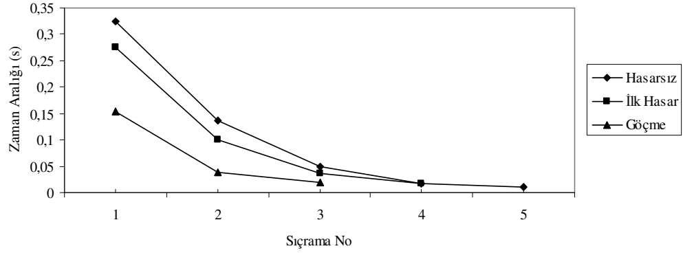
Şekil 5.57. SC6 Deney elemanı sıçrama-zaman aralığı ilişkisi
