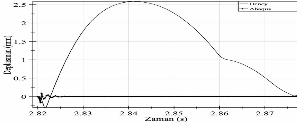
Şekil 6.24. SC4 Deney ile Abaqus ilk çarpma anı deplasman değerleri karşılaştırılması
