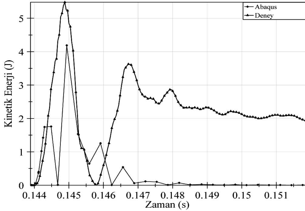
Şekil 6.62. Yüksek dayanımlı beton, 650 mm yükseklik için kinetik enerji değerleri karşılaştırması
