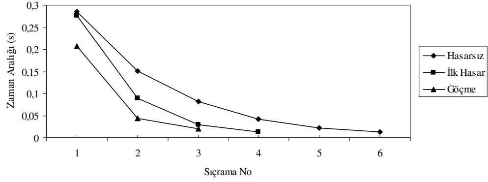
Şekil 5.55. SC4 Deney elemanı sıçrama-zaman aralığı ilişkisi
