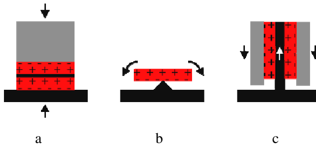
Şekil 3.3. Piezoelektrik algılayıcılarda piezo malzeme şekilleri a. Basınç b. Eğilme c. Kayma
