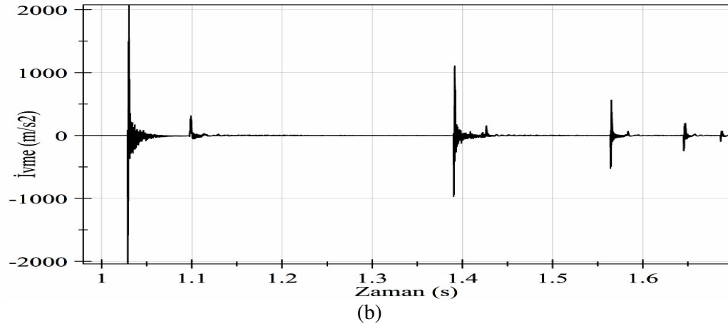
Şekil 6.16. İvme değerleri a) Abaqus analizi b) Deney sonucu
