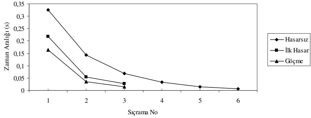
Şekil 5.52. SC1 Deney elemanı sıçrama-zaman aralığı ilişkisi
