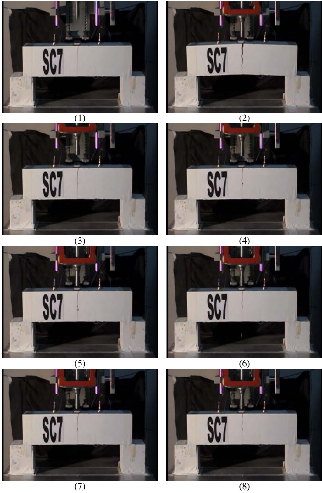
Resim 5.28. SC7 Deney elemanı göçme durumu
