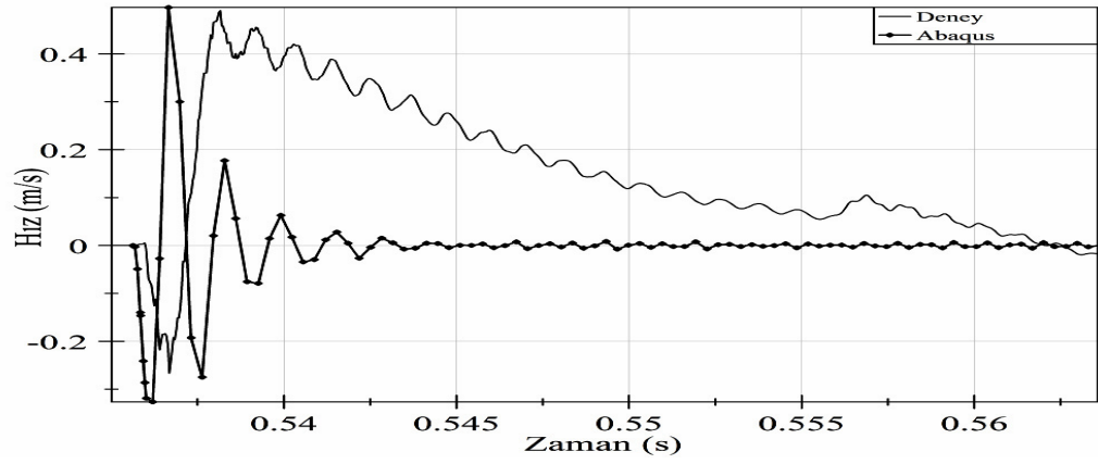
Şekil 6.43. SC8 Deney ile Abaqus ilk çarpma anı hız değerleri karşılaştırılması
