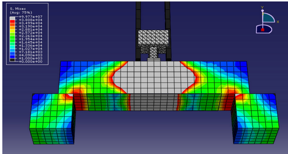
Şekil 6.45. 600 mm için Abaqus gerilme dağılımı
