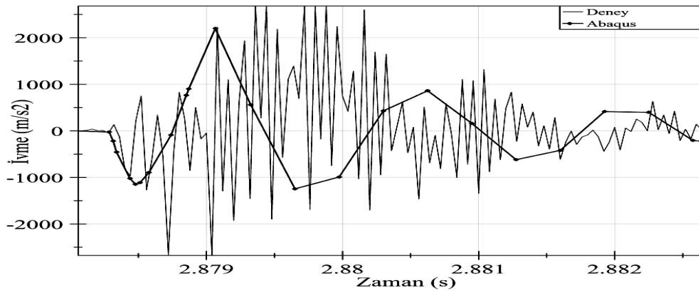
Şekil 6.52. SC10 Deney ile Abaqus ilk çarpma anı ivme değerleri karşılaştırılması
