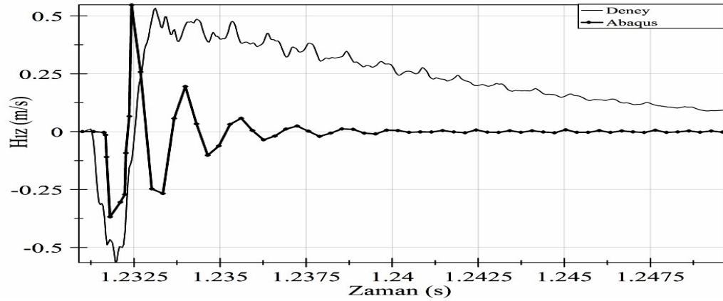
Şekil 6.38. SC7 Deney ile Abaqus ilk çarpma anı hız değerleri karşılaştırılması
