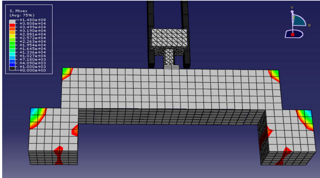
Şekil 6.40. 650 mm için Abaqus gerilme dağılımı
