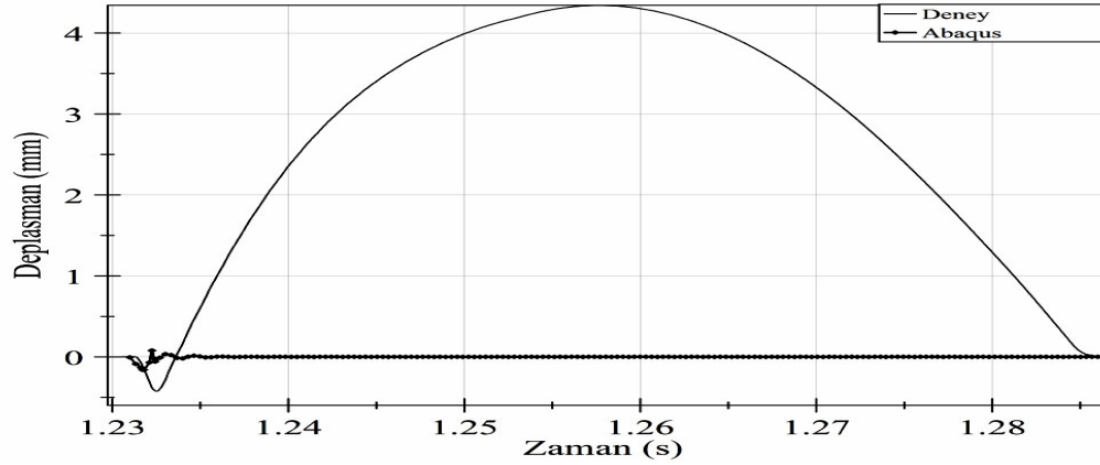
Şekil 6.39. SC7 Deney ile Abaqus ilk çarpma anı deplasman değerleri karşılaştırılması
