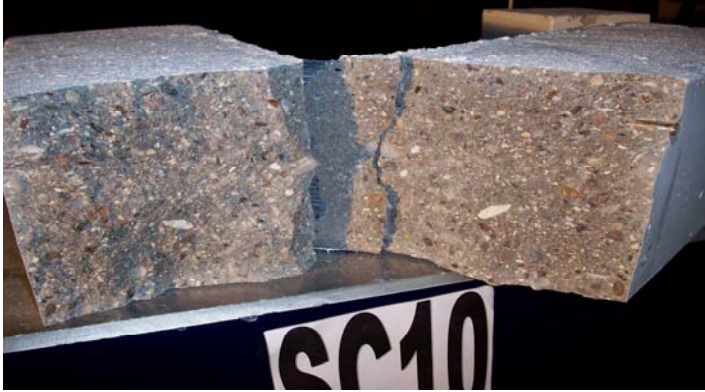
Resim 5.39. SC10 Elemanının agrega-matris görünümü
