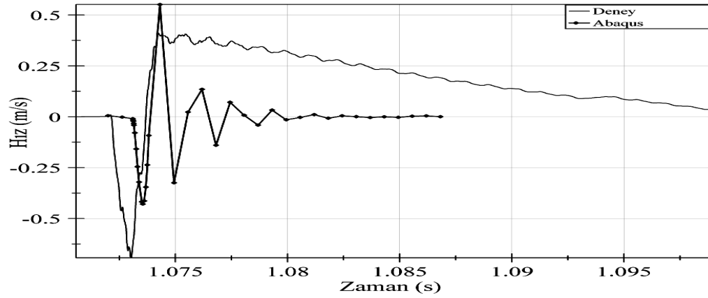
Şekil 6.8. SC1 Deney ile Abaqus ilk çarpma anı hız değerleri karşılaştırılması
