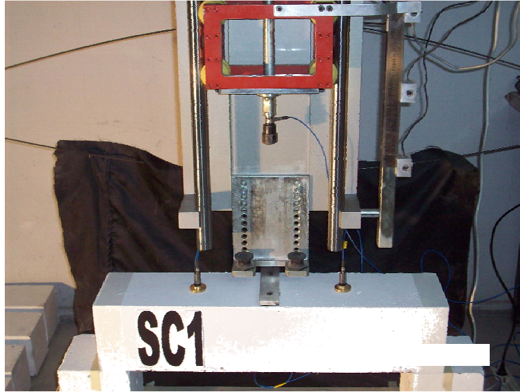
Resim 4.8. Deney elemanı
