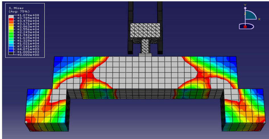
Şekil 6.30. 750 mm için Abaqus gerilme dağılımı
