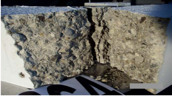
Resim 5.15. SC4 Elemanının agrega-matris görünümü
