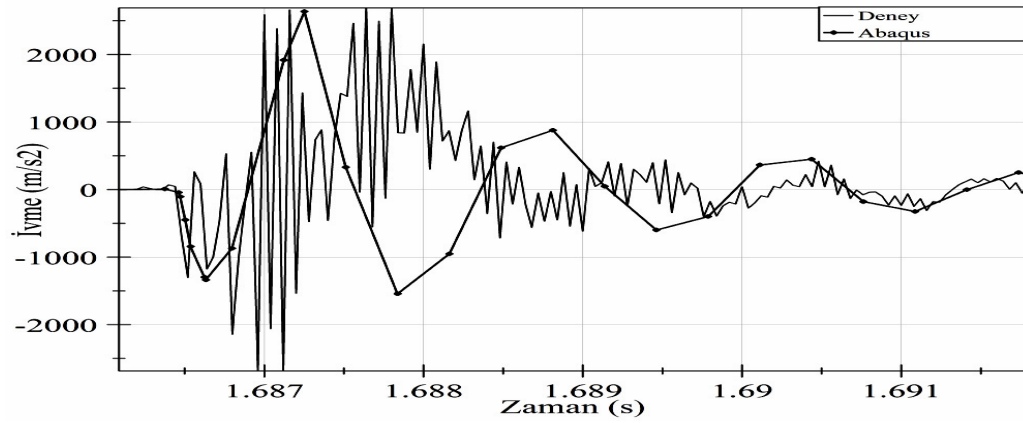
Şekil 6.32. SC6 Deney ile Abaqus ilk çarpma anı ivme değerleri karşılaştırılması
