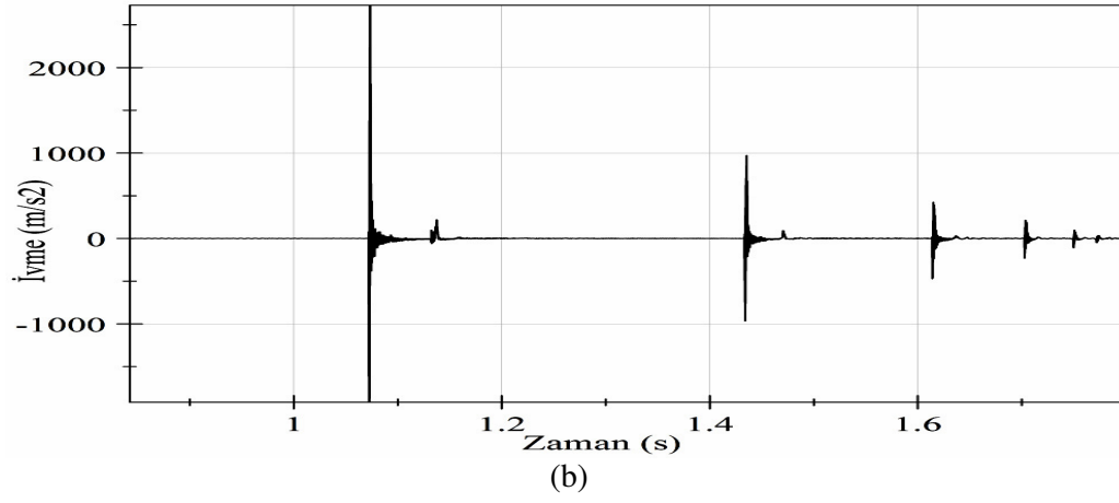
Şekil 6.6. İvme değerleri a) Abaqus analizi b) Deney sonucu
