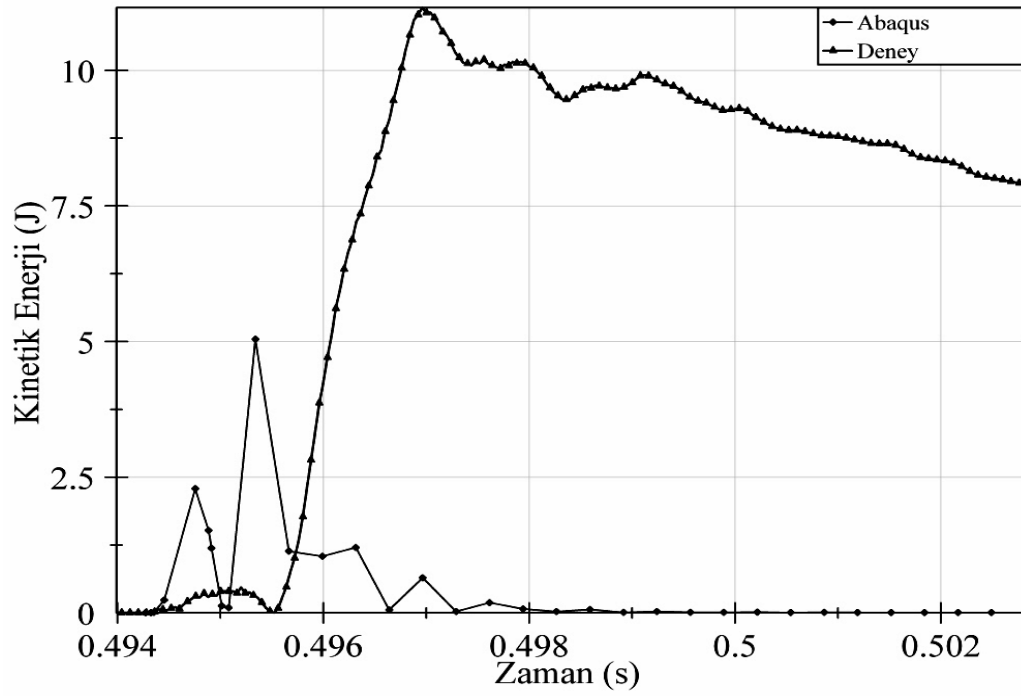
Şekil 6.64. Yüksek dayanımlı beton, 700 mm yükseklik için kinetik enerji değerleri karşılaştırması
