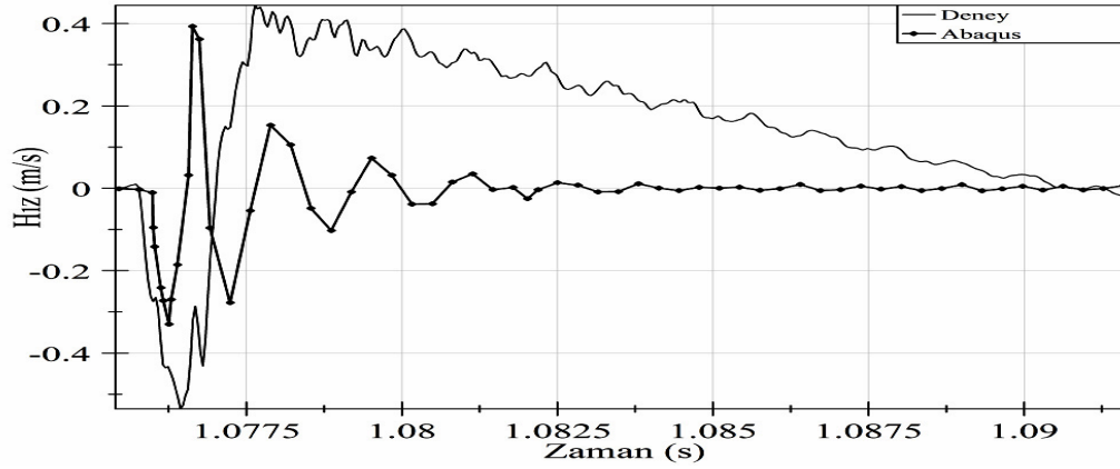
Şekil 6.48. SC9 Deney ile Abaqus ilk çarpma anı hız değerleri karşılaştırılması
