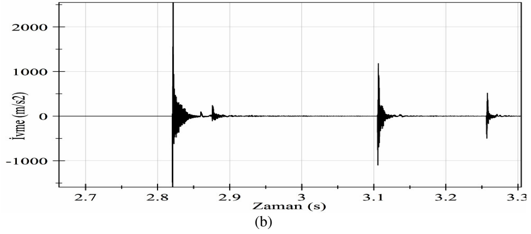
Şekil 6.21. İvme değerleri a) Abaqus analizi b) Deney sonucu
