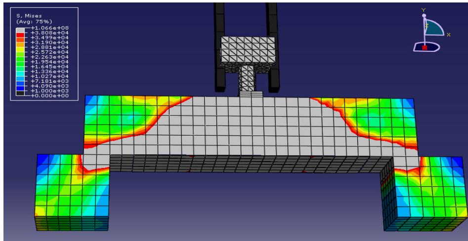
Şekil 6.15. 650 mm için Abaqus gerilme dağılımı
