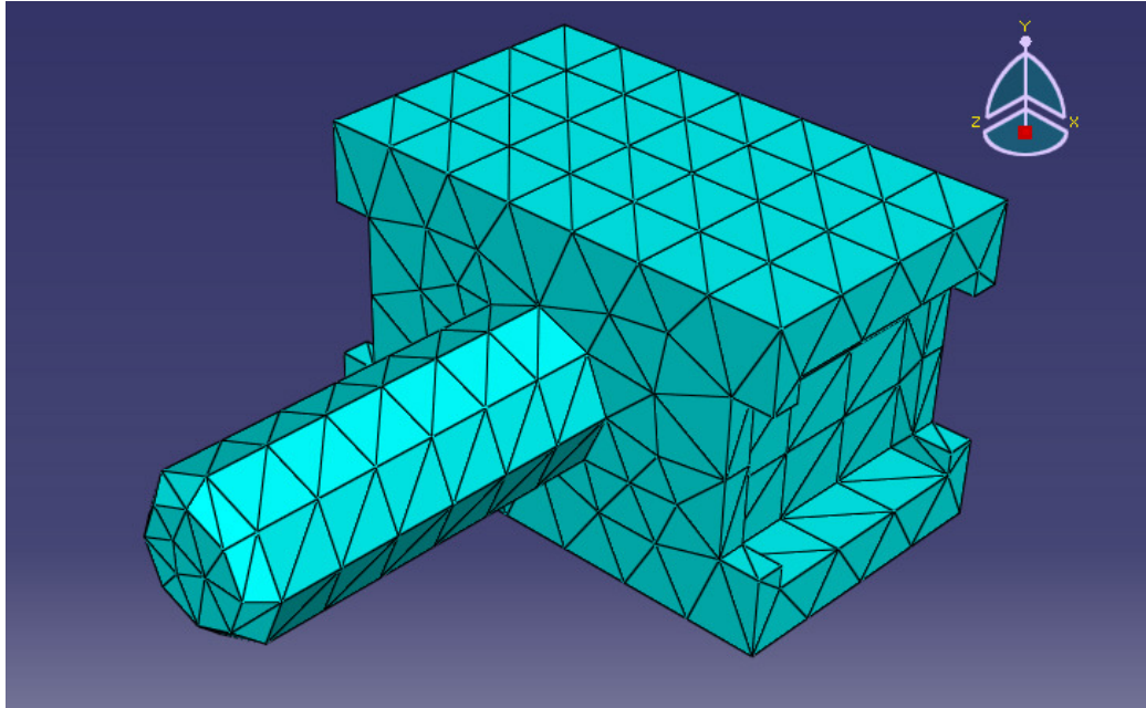
Şekil 6.4. Çekiç modelinin sonlu elemanlara bölünmesi
