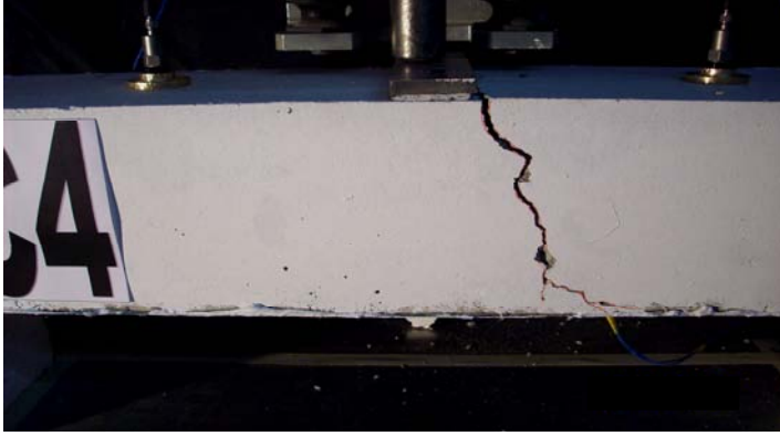
Resim 5.14. SC4 Elemanının göçme durumu
