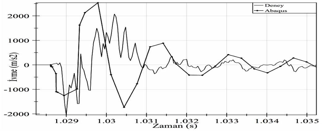
Şekil 6.17. SC3 Deney ile Abaqus ilk çarpma anı ivme değerleri karşılaştırılması
