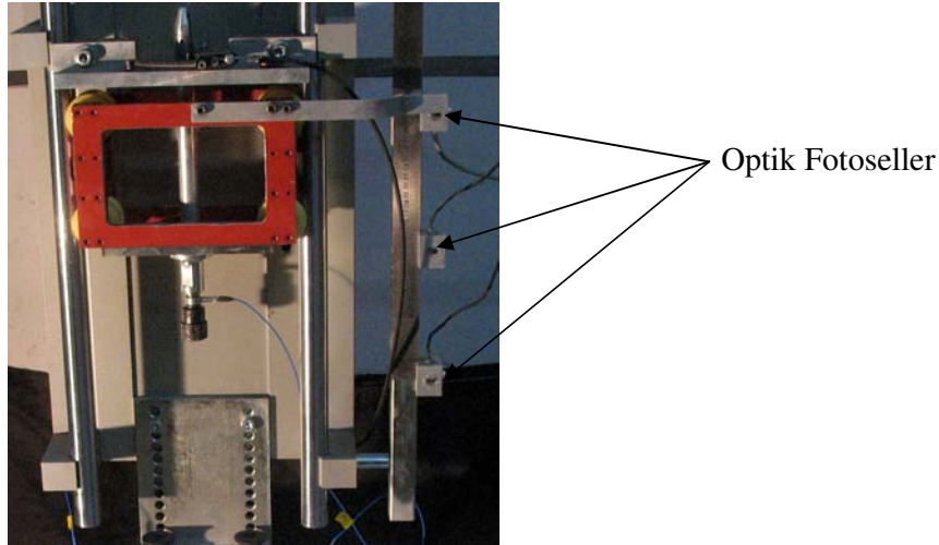
Resim 3.8. Optik fotoseller ve yerleşimi
