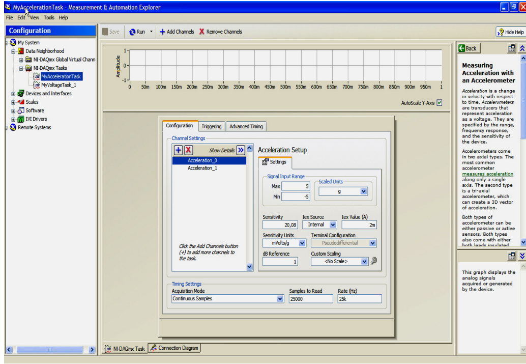
Resim 4.7. National Instruments firması tarafından hazırlanan Measurement & Automation programı
