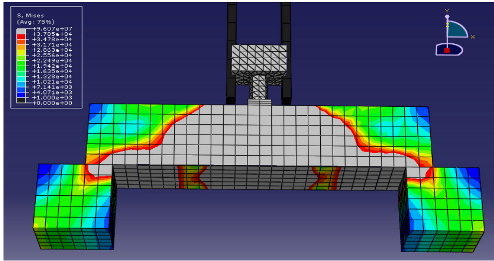
Şekil 6.35. 700 mm için Abaqus gerilme dağılımı
