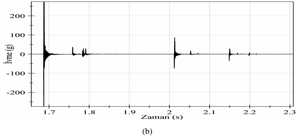
Şekil 6.31. İvme değerleri a) Abaqus analizi b) Deney sonucu
