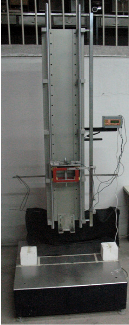
Resim 3.1. Deney düzeneđi
