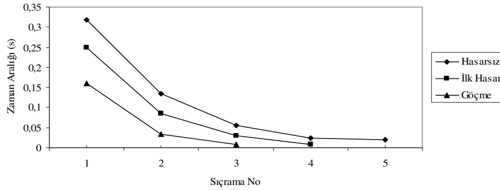
Şekil 5.61. SC10 Deney elemanı sıçrama-zaman aralığı ilişkisi
