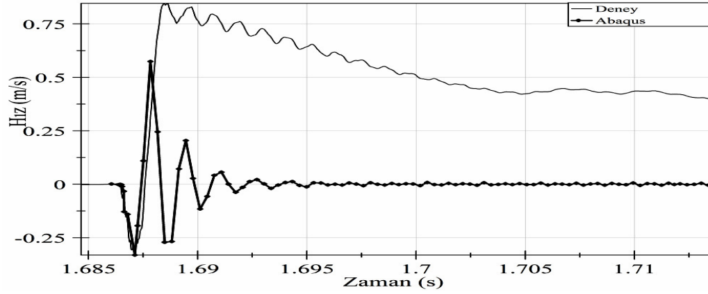
Şekil 6.33. SC6 Deney ile Abaqus ilk çarpma anı hız değerleri karşılaştırılması
