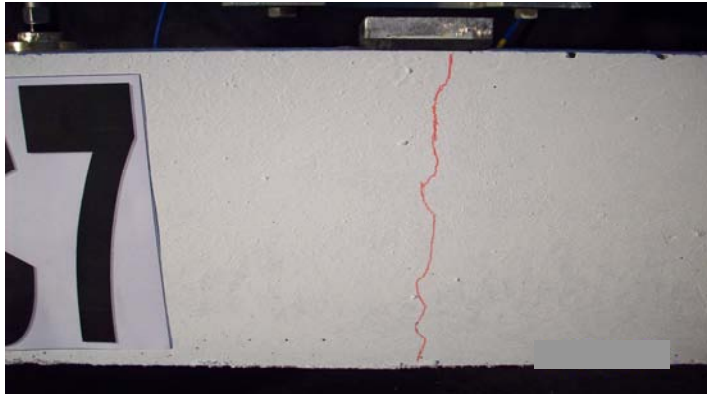
Resim 5.25. SC7 Elemanında oluşan ilk hasar
