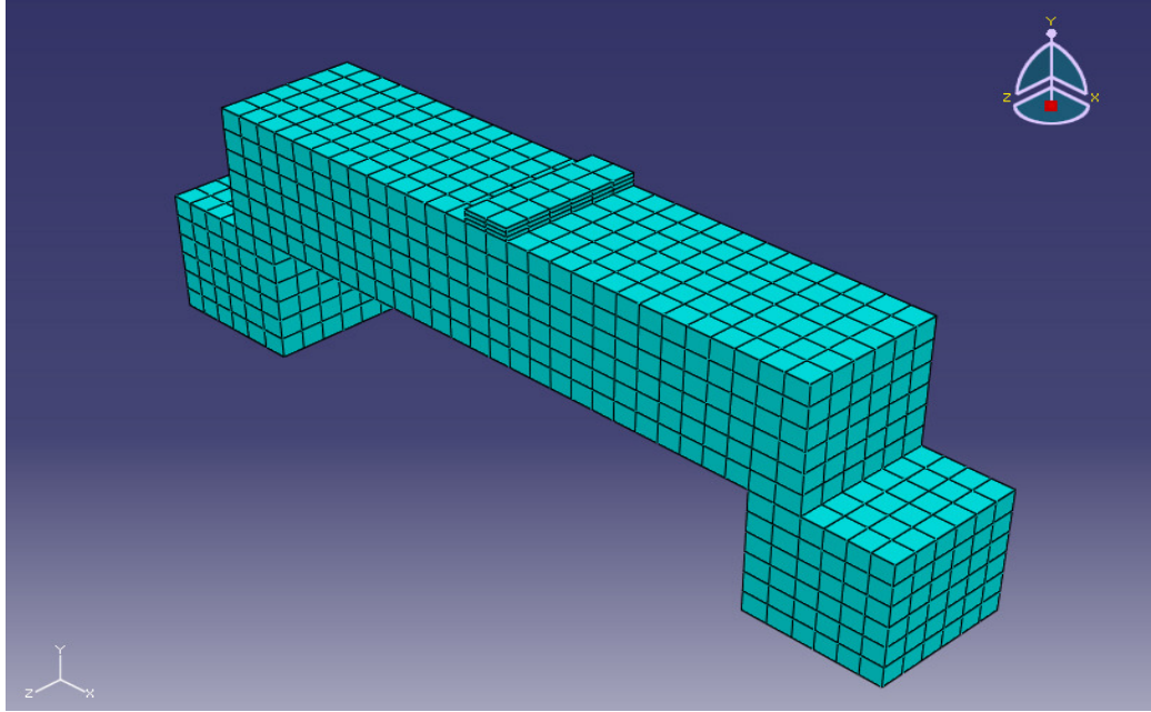
Şekil 6.3. Deney elemanı modelinin sonlu elemanlara bölünmesi
