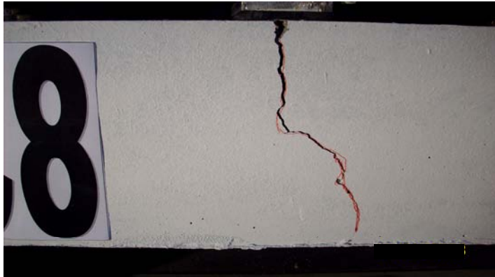
Resim 5.29. SC8 Elemanında oluşan ilk hasar
