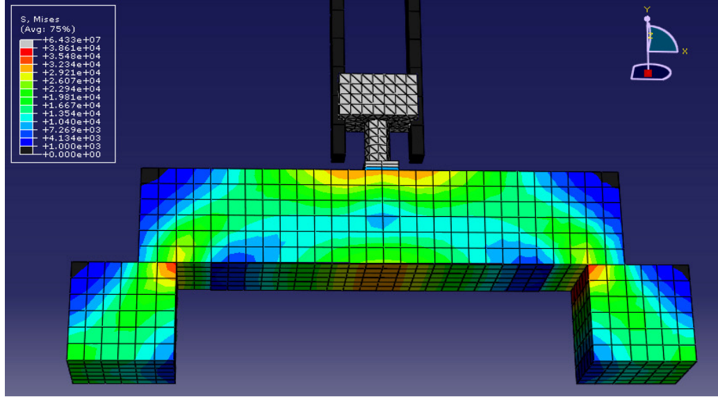
Şekil 6.10. 700 mm için Abaqus gerilme dağılımı
