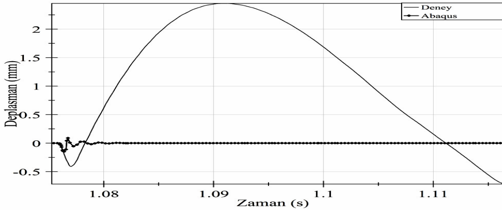
Şekil 6.49. SC9 Deney ile Abaqus ilk çarpma anı deplasman değerleri karşılaştırılması
