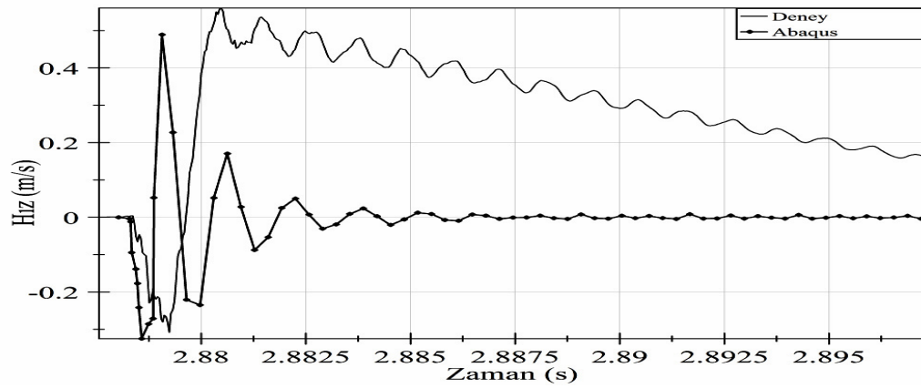
Şekil 6.53. SC10 Deney ile Abaqus ilk çarpma anı hız değerleri karşılaştırılması
