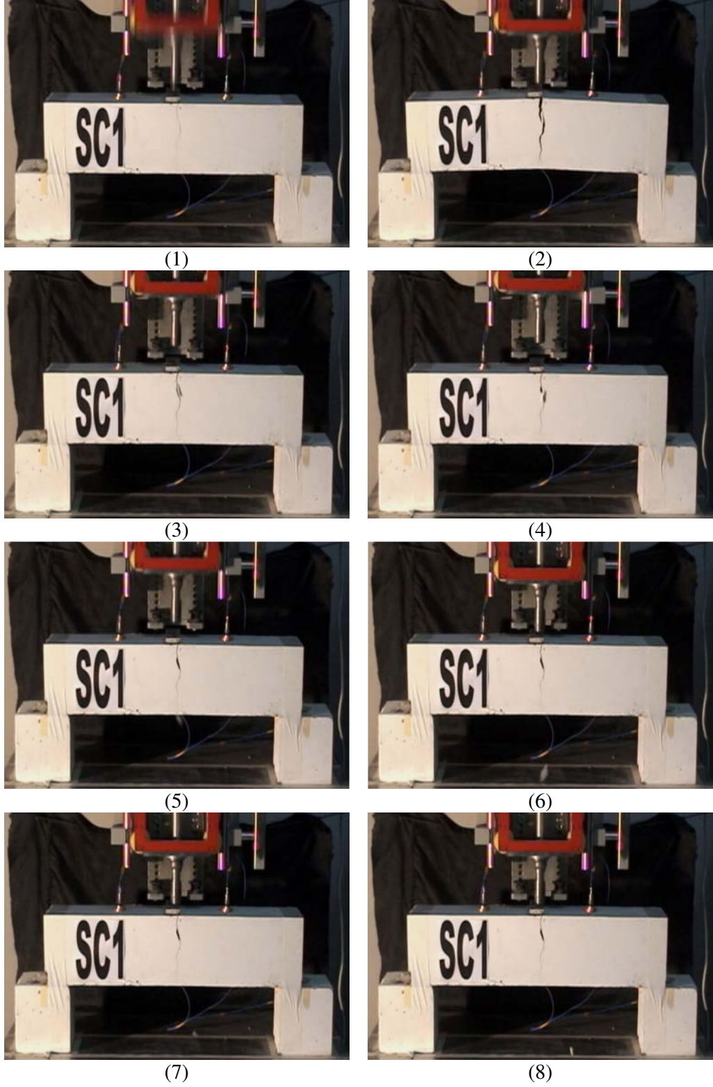
Resim 5.4. SC1 Deney elemanı göçme durumu
