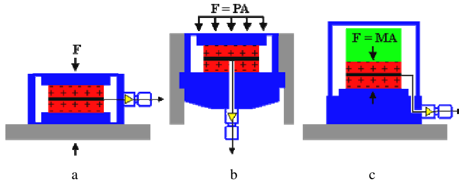
Şekil 3.4. Piezoelektrik algılayıcılar a. Kuvvet b. Basınç c. İvme algılayıcıları
