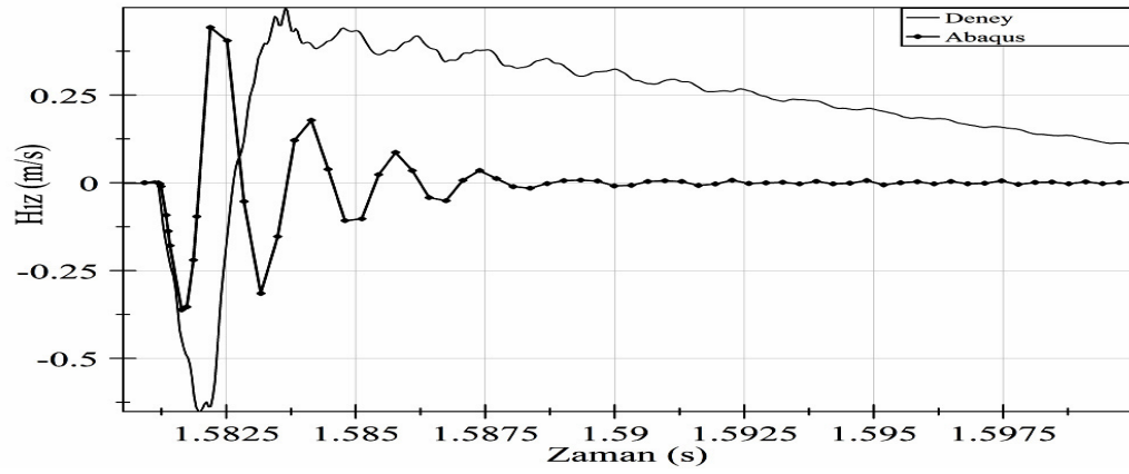
Şekil 6.28. SC5 Deney ile Abaqus ilk çarpma anı hız değerleri karşılaştırılması
