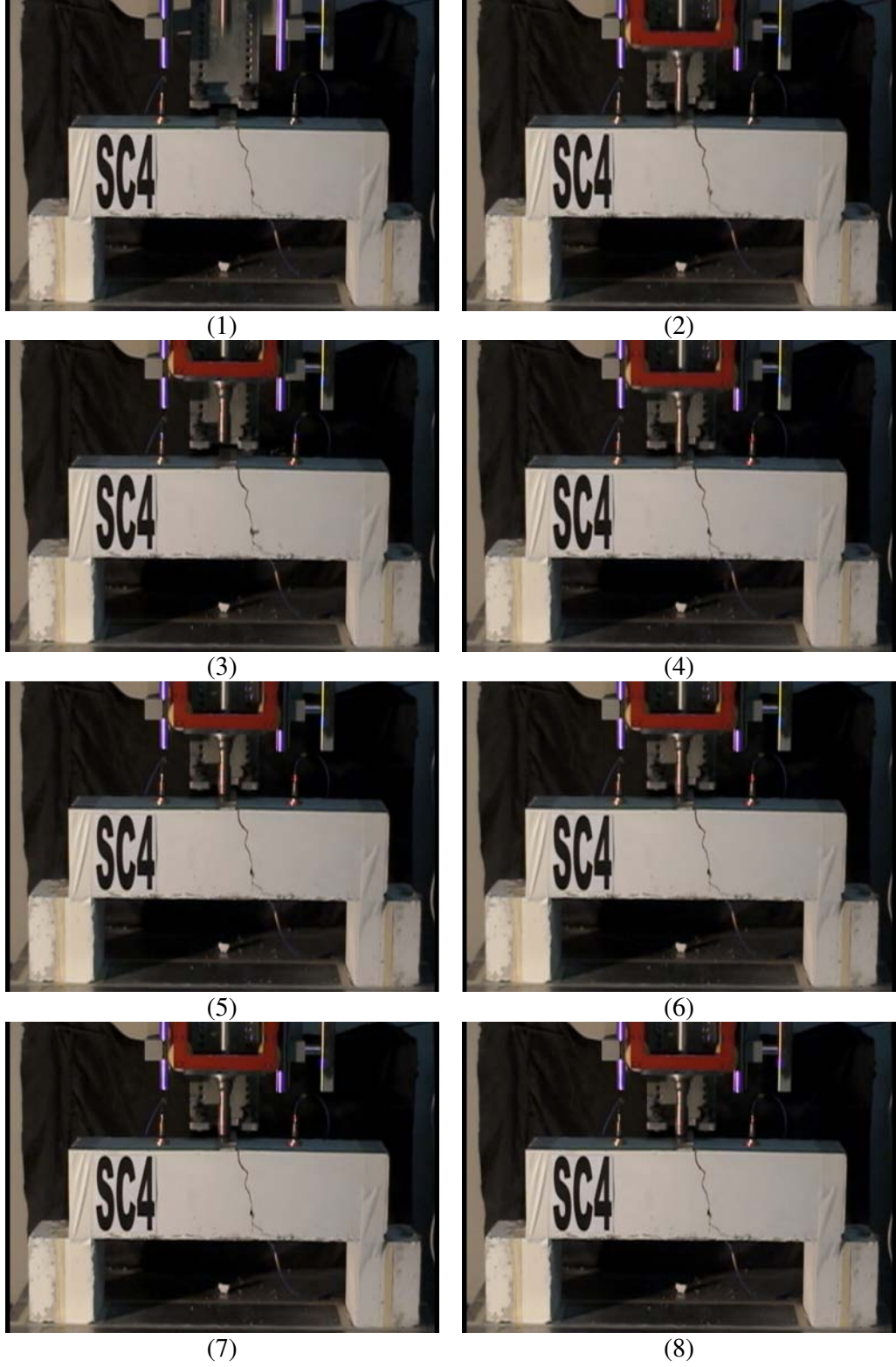
Resim 5.16. SC4 Deney elemanı göçme durumu
