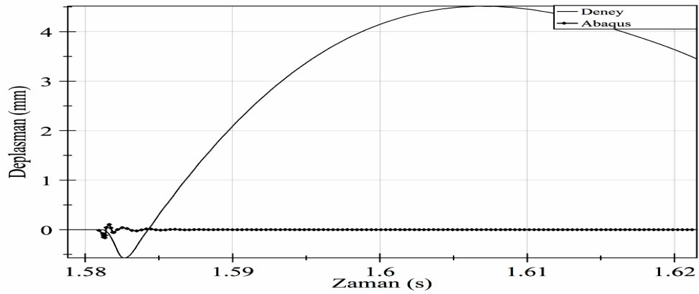
Şekil 6.29. SC5 Deney ile Abaqus ilk çarpma anı deplasman değerleri karşılaştırılması
