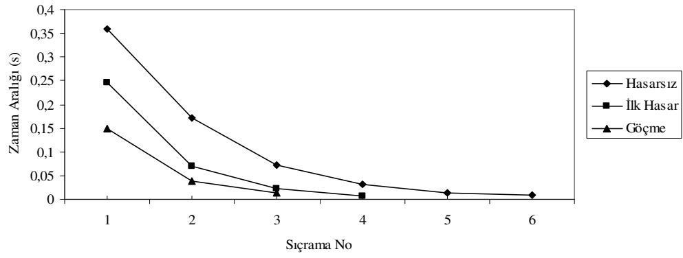
Şekil 5.59. SC8 Deney elemanı sıçrama-zaman aralığı ilişkisi
