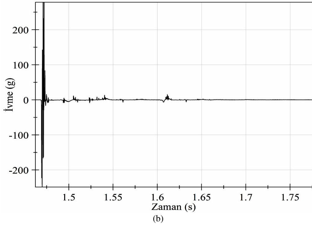
Şekil 5.3. SC1 Deney elemanın 19. düşme(göçme) ivme-zaman grafikleri a) Sol ivmeölçer b) Sağ ivmeölçer
