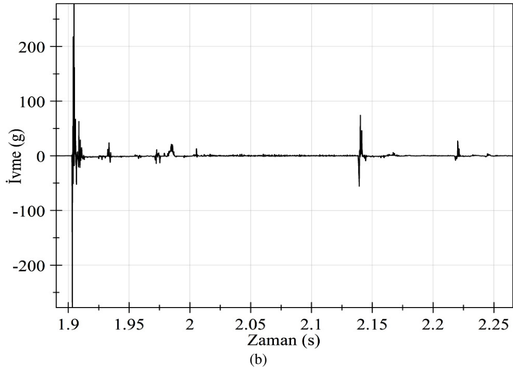
Şekil 5.2. SC1 Deney elemanın 6. düşme(ilk hasar) ivme-zaman grafikleri a) Sol ivmeölçer b) Sağ ivmeölçer
