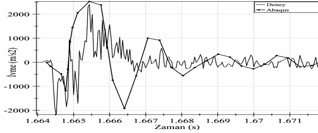
Şekil 6.12. SC2 Deney ile Abaqus ilk çarpma anı ivme değerleri karşılaştırılması
