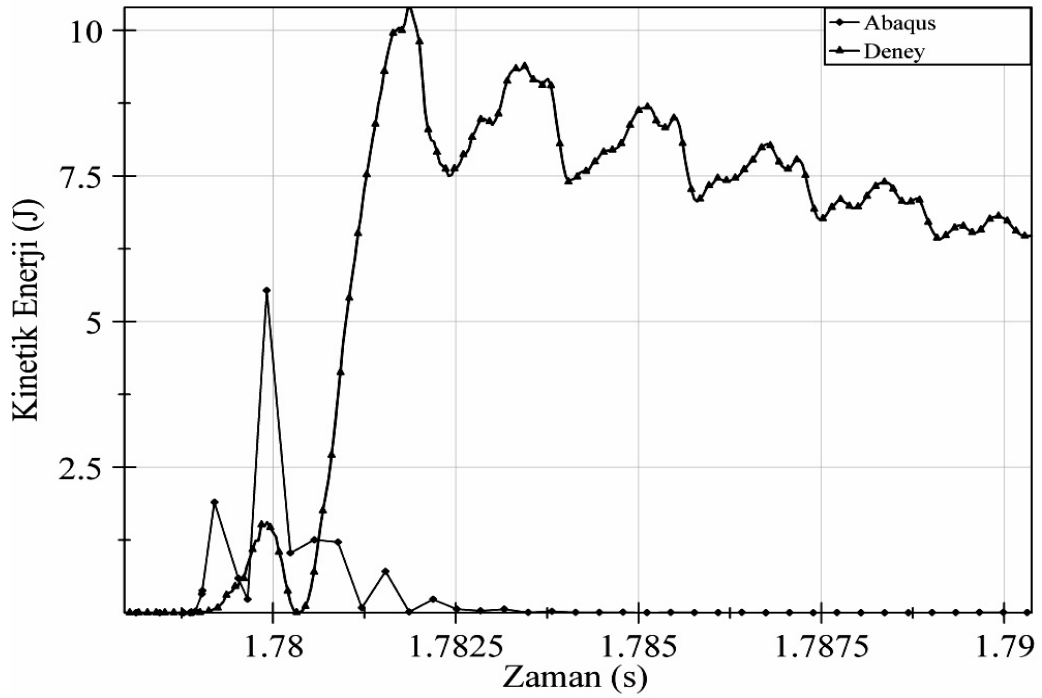
Şekil 6.66. Yüksek dayanımlı beton, 750 mm yükseklik için kinetik enerji değerleri karşılaştırması
