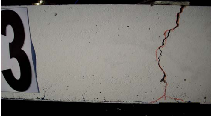
Resim 5.10. SC3 Elemanının göçme durumu
