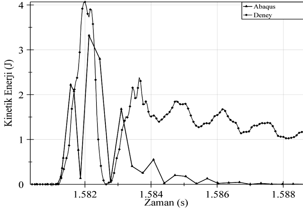
Şekil 6.57. Normal dayanımlı beton, 550 mm yükseklik için kinetik enerji değerleri karşılaştırması
