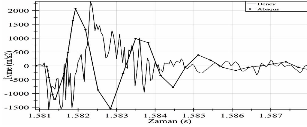
Şekil 6.27. SC5 Deney ile Abaqus ilk çarpma anı ivme değerleri karşılaştırılması
