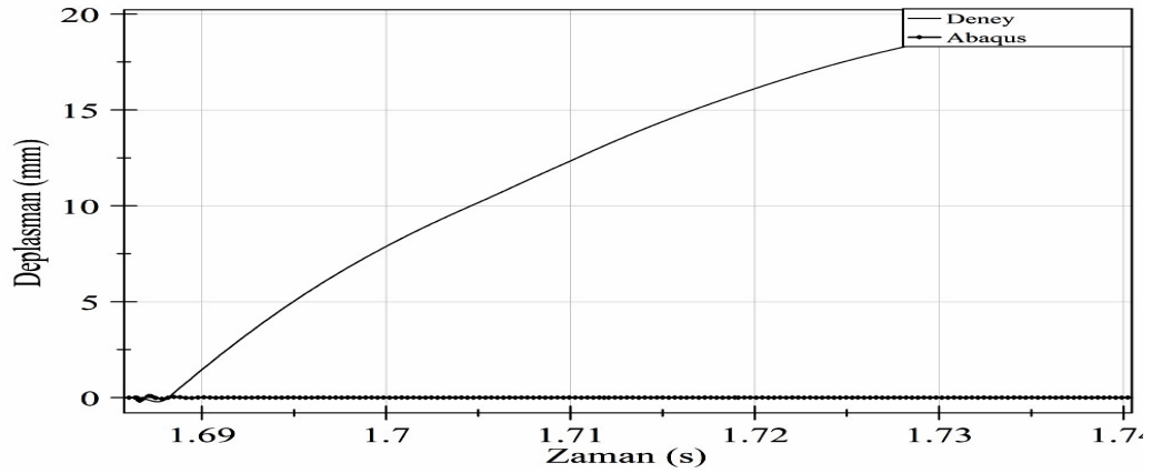
Şekil 6.34. SC6 Deney ile Abaqus ilk çarpma anı deplasman değerleri karşılaştırılması
