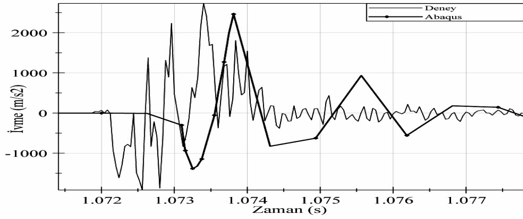
Şekil 6.7. SC1 Deney ile Abaqus ilk çarpma anı ivme değerleri karşılaştırılması
