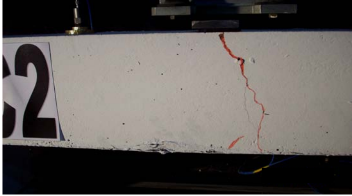
Resim 5.5. SC2 Elemanında oluşan ilk hasar
