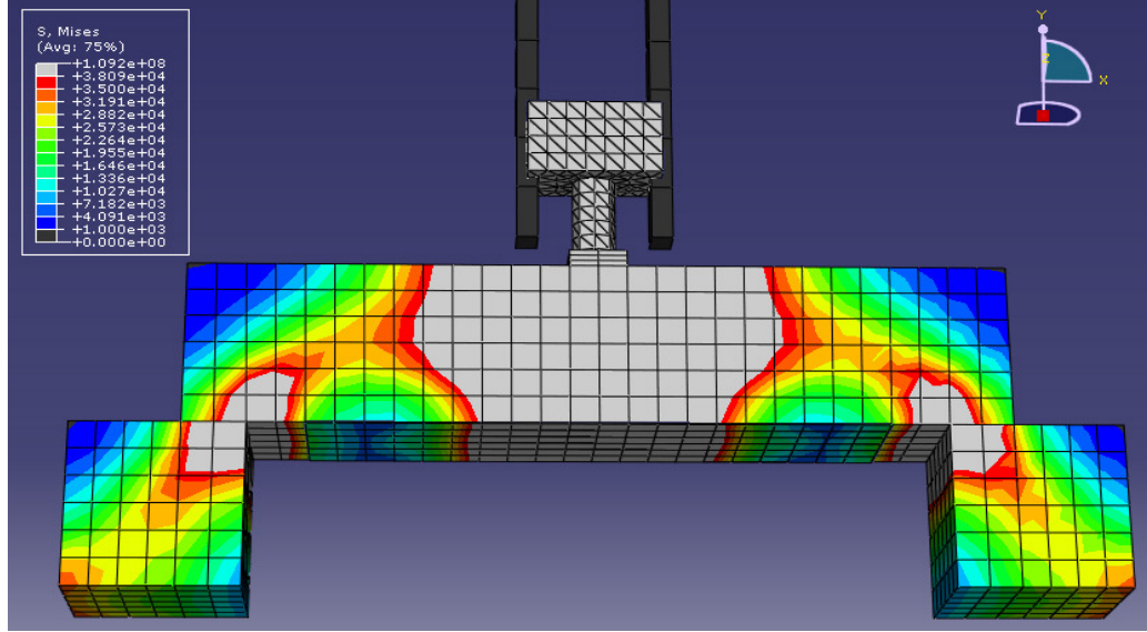
Şekil 6.5. 750 mm için Abaqus gerilme dağılımı
