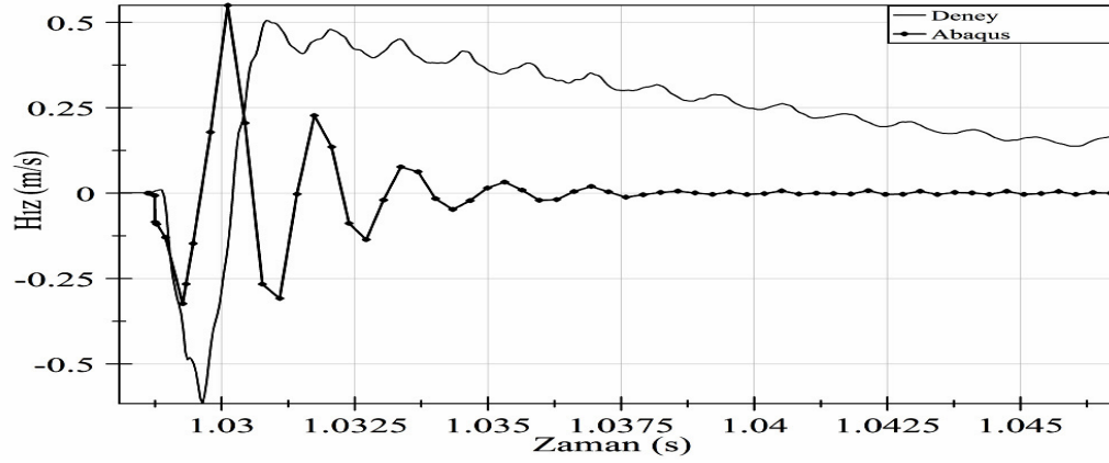
Şekil 6.18. SC3 Deney ile Abaqus ilk çarpma anı hız değerleri karşılaştırılması
