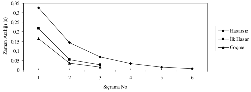
Şekil 5.56. SC5 Deney elemanı sıçrama-zaman aralığı ilişkisi
