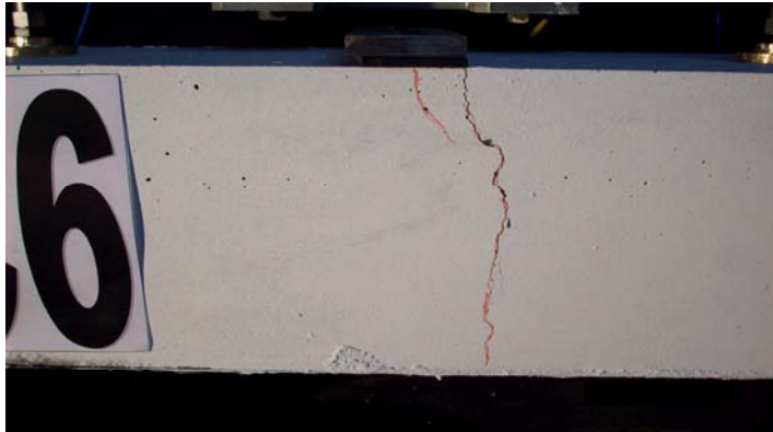
Resim 5.21. SC6 Elemanında oluşan ilk hasar
