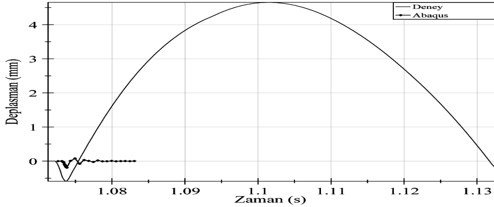
Şekil 6.9. SC1 Deney ile Abaqus ilk çarpma anı deplasman değerleri karşılaştırılması
