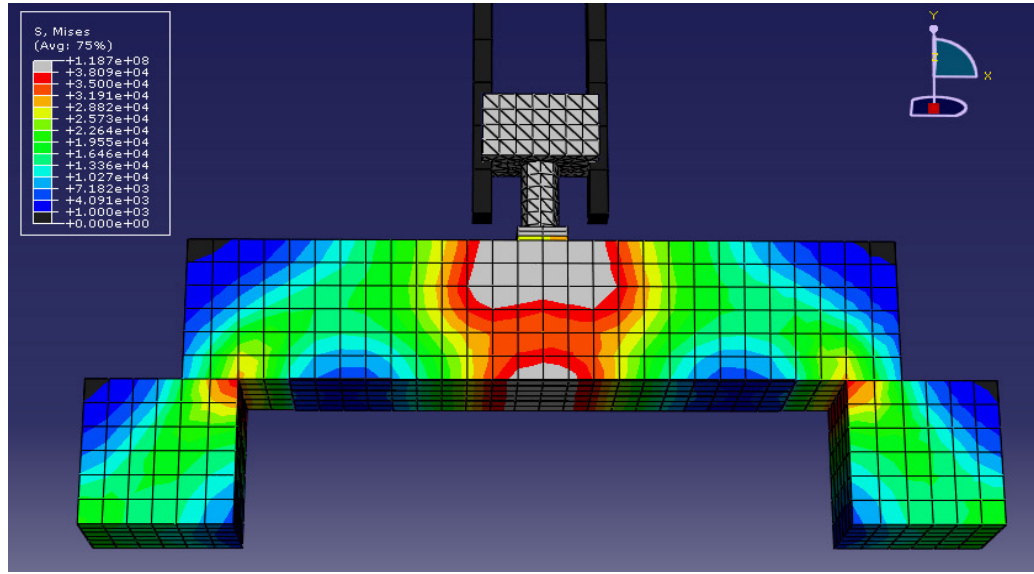
Şekil 6.50. 550 mm için Abaqus gerilme dağılımı
