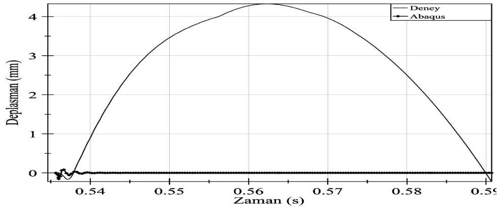
Şekil 6.44. SC8 Deney ile Abaqus ilk çarpma anı deplasman değerleri karşılaştırılması
