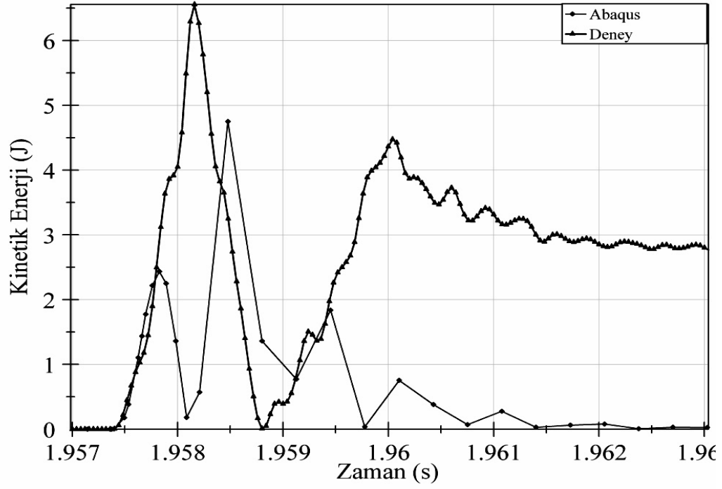
Şekil 6.59. Normal dayanımlı beton, 600 mm yükseklik için kinetik enerji değerleri karşılaştırması
