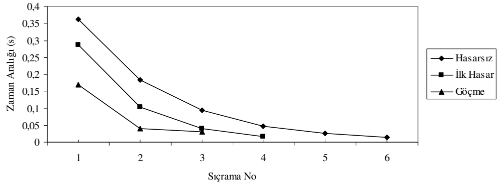
Şekil 5.58. SC7 Deney elemanı sıçrama-zaman aralığı ilişkisi
