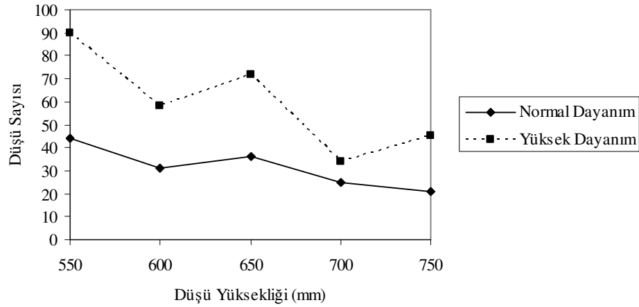
Şekil 5.51. Düşme sayısı, düşme yüksekliği ve beton dayanımının karşılaştırması
