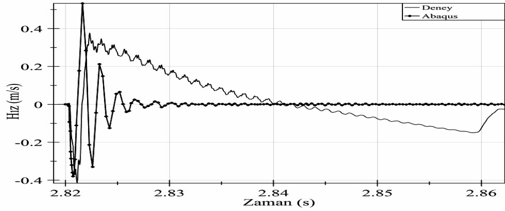
Şekil 6.23. SC4 Deney ile Abaqus ilk çarpma anı hız değerleri karşılaştırılması
