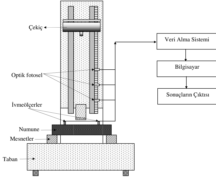
Şekil 3.1. Ağırlık düşürücü deney düzeneğinin tasarım şeması
