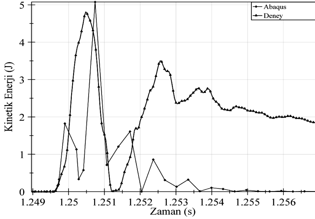
Şekil 6.61. Normal dayanımlı beton, 650 mm yükseklik için kinetik enerji değerleri karşılaştırması
