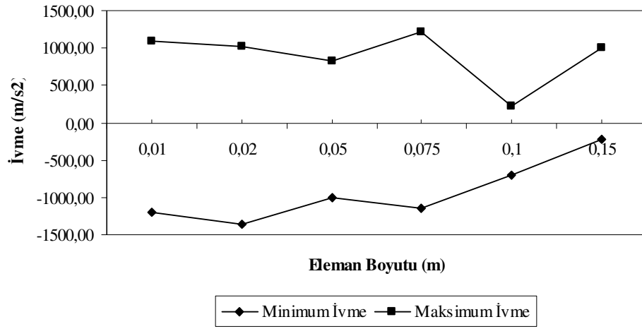
Şekil 6.2. Sonlu eleman boyutlarına göre ivme değerlerindeki değişim
