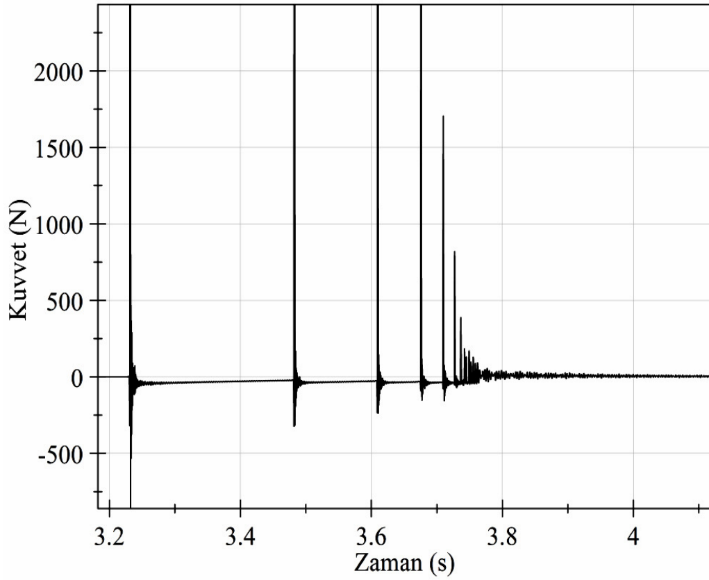
Şekil 5.6. Kuvvetölçerden elde edilen değerler
