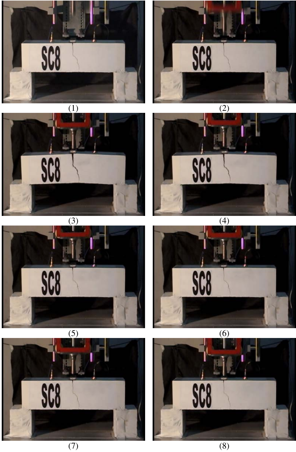
Resim 5.32. SC8 Deney elemanı göçme durumu
