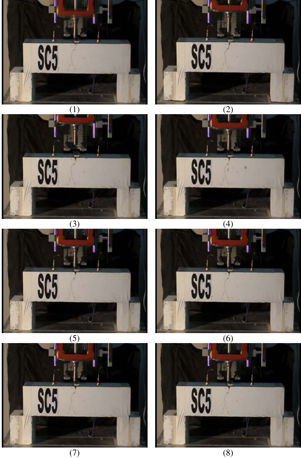
Resim 5.20. SC5 Deney elemanı göçme durumu
