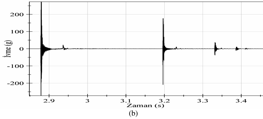
Şekil 6.51. İvme değerleri a) Abaqus analizi b) Deney sonucu
