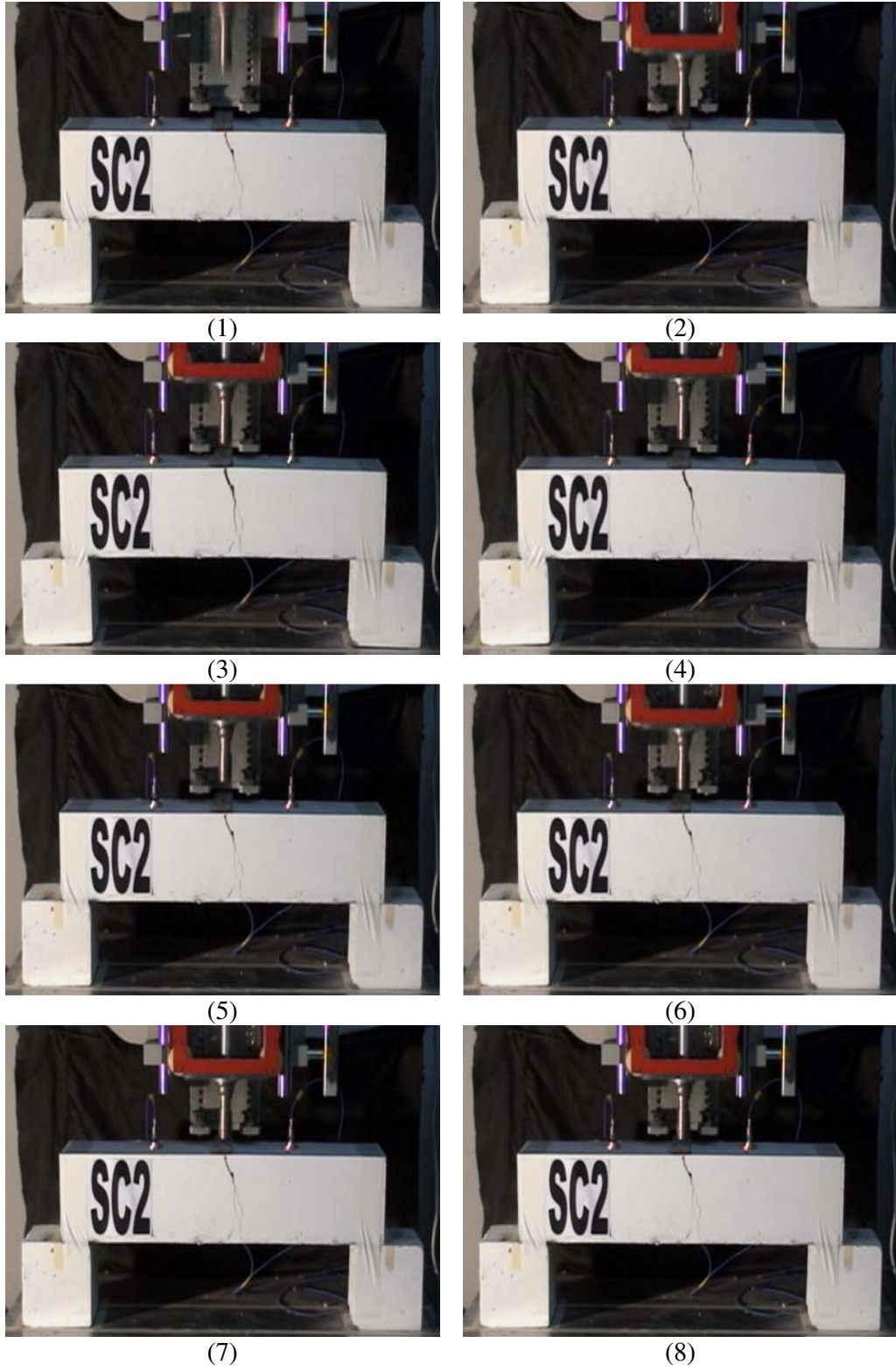
Resim 5.8. SC2 Deney elemanı göçme durumu
