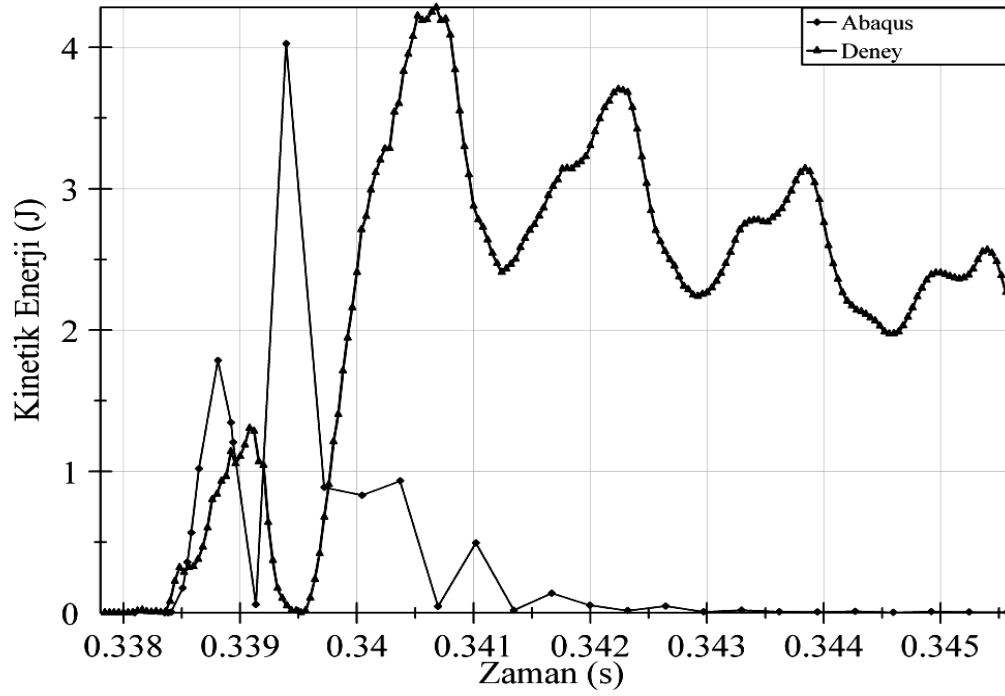
Şekil 6.58. Yüksek dayanımlı beton, 550 mm yükseklik için kinetik enerji değerleri karşılaştırması
