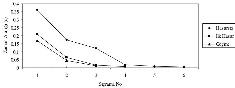
Şekil 5.54. SC3 Deney elemanı sıçrama-zaman aralığı ilişkisi
