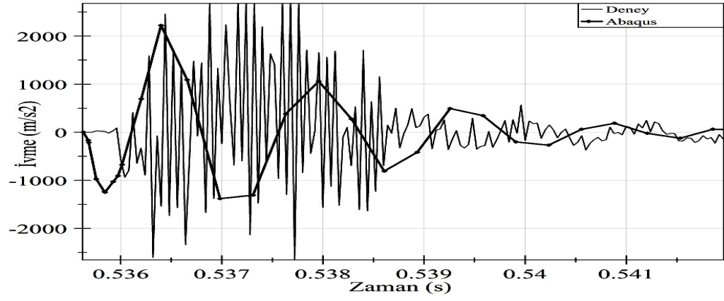
Şekil 6.42. SC8 Deney ile Abaqus ilk çarpma anı ivme değerleri karşılaştırılması
