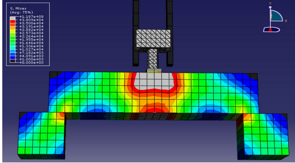
Şekil 6.25. 550 mm için Abaqus gerilme dağılımı
