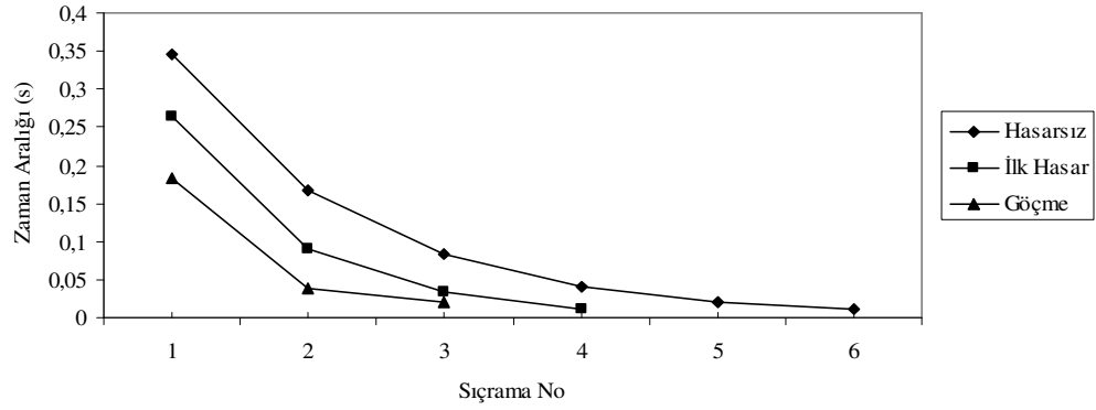
Şekil 5.60. SC9 Deney elemanı sıçrama-zaman aralığı ilişkisi
