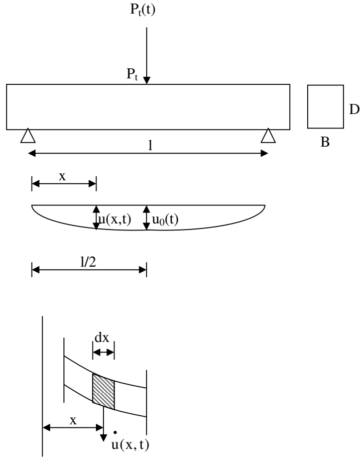
Şekil 6.55. Kabul edilen kiriş deplasmanı
