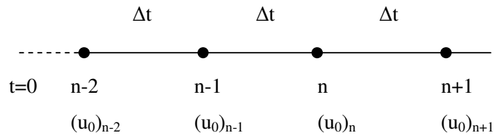
Şekil 6.56. Sonlu farklar yöntemi şekilsel gösterimi
