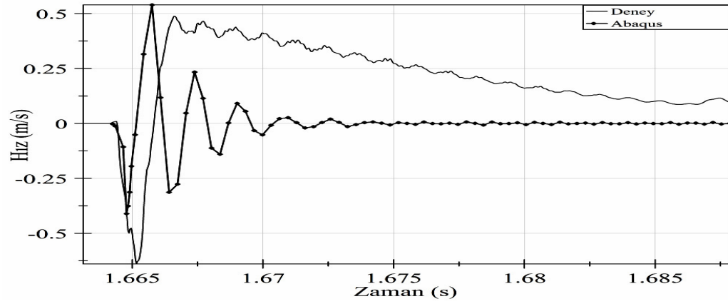
Şekil 6.13. SC2 Deney ile Abaqus ilk çarpma anı hız değerleri karşılaştırılması
