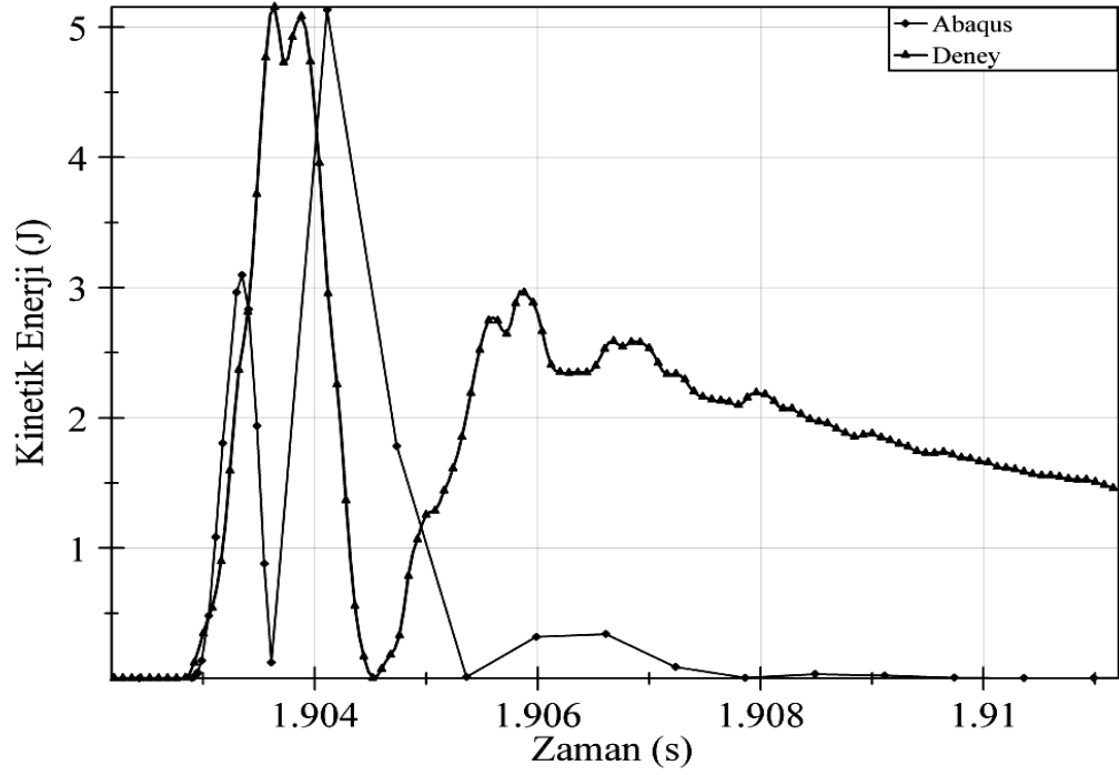
Şekil 6.65. Normal dayanımlı beton, 750 mm yükseklik için kinetik enerji değerleri karşılaştırması
