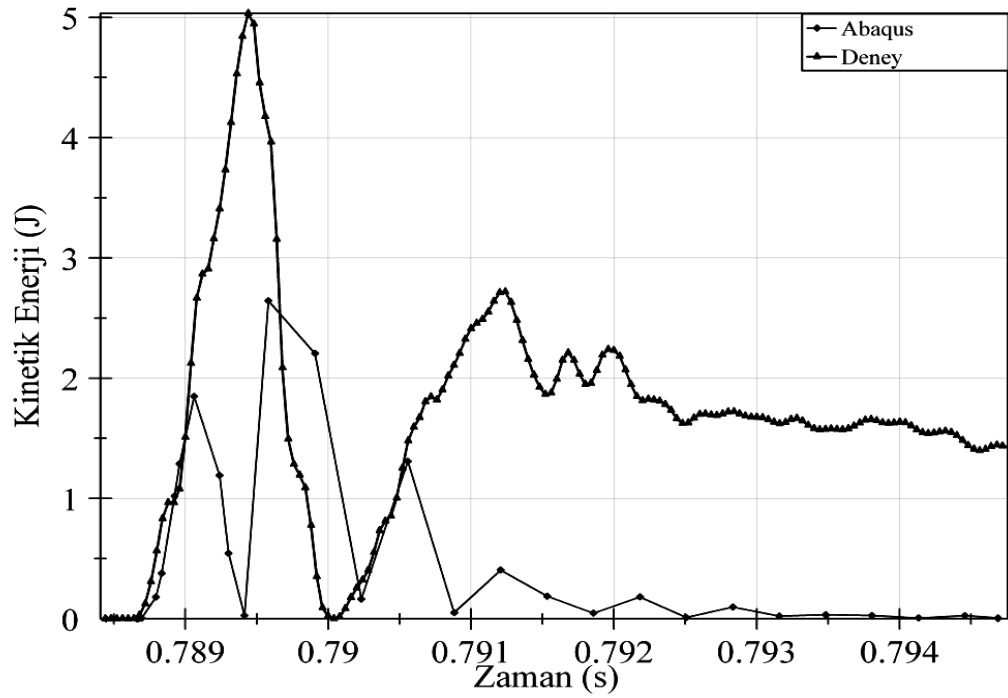
Şekil 6.60. Yüksek dayanımlı beton, 600 mm yükseklik için kinetik enerji değerleri karşılaştırması
