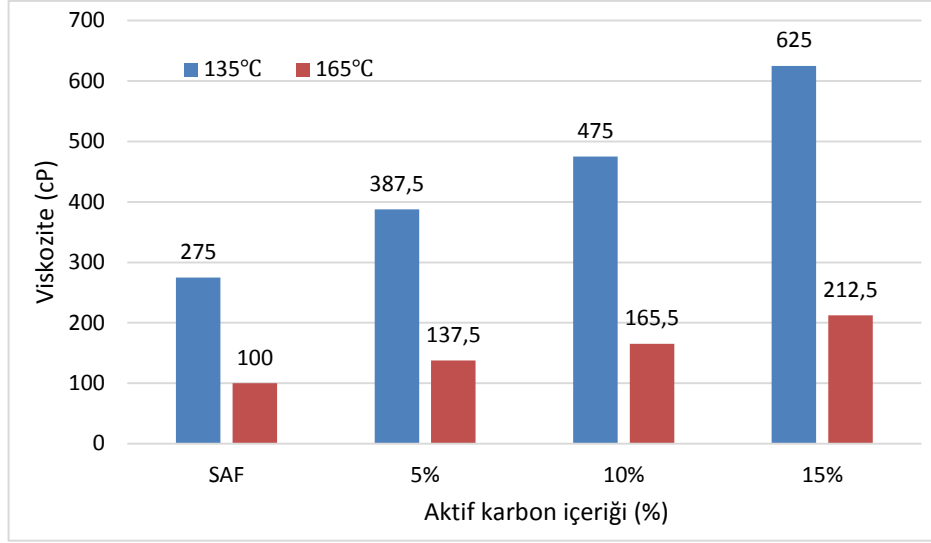
Şekil 4.11. Saf ve modifiye bitümlerin viskozite değerleri
