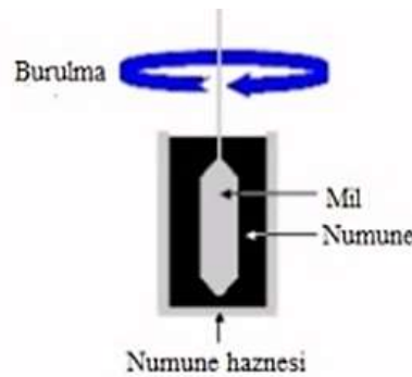
Şekil 3.5. Dönel viskozimetre deney şeması
