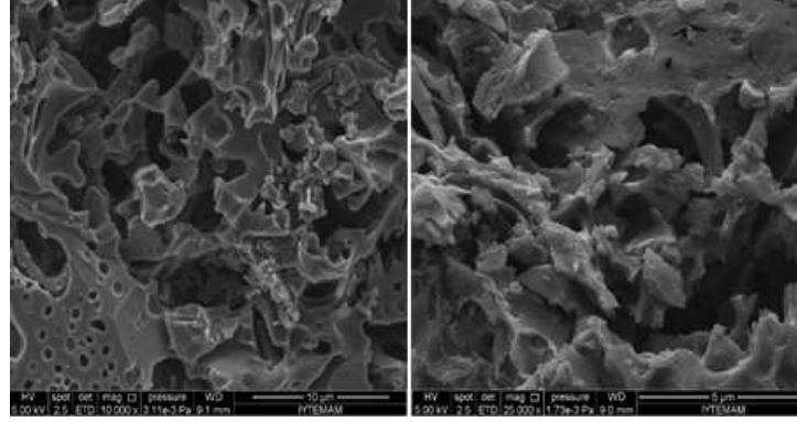
Şekil 4.5. Elde edilen aktif karbonun SEM görüntüleri (Piroliz şartları : S/C=2 , Piroliz sıcaklığı: 600°C, Piroliz süresi : 120 dakika, Asit ile stabilizasyon : 2N HCl, Sıvı/Katı oranı = 10, Oda sıcaklığı, Kurutma sıcaklığı: 100°C).
