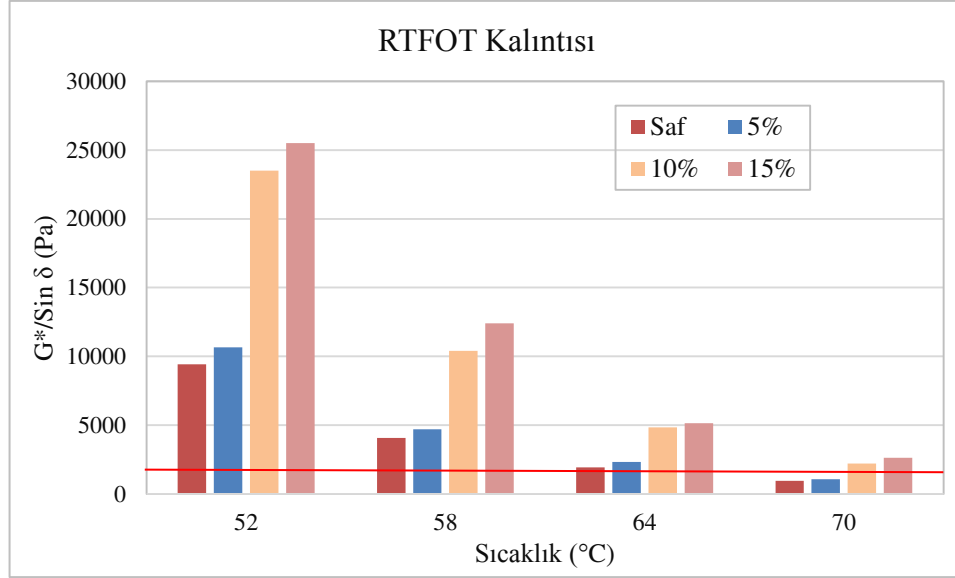
Şekil 4.17. RTFOT sonrası bağlayıcıların G^*/\sin \delta değerlerinin sıcaklıkla değişimi
