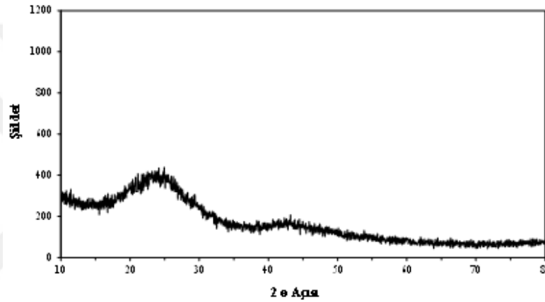
Şekil 4.6. Elde edilen aktif karbonun X ışını difraktogramı (XRD) (Piroliz şartları : S/C=2 , Piroliz sıcaklığı: 600°C, Piroliz süresi : 120 dakika, Asit ile stabilizasyon : 2N HCl, Sıvı/Katı oranı = 10, Oda sıcaklığı, Kurutma sıcaklığı: 100°C).
