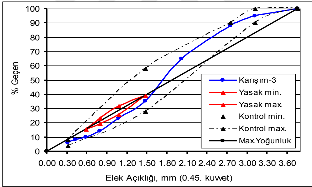
Şekil 4.21. Çalışmada kullanılan agreg gradasyonu
