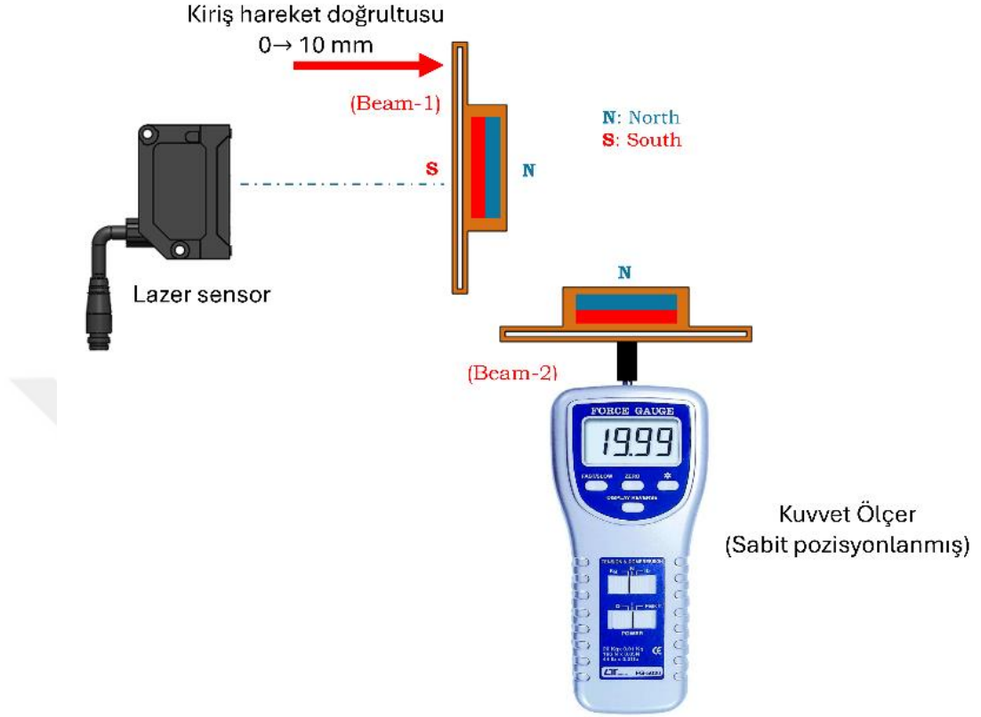
Şekil 5.7. Deneyisel kuvvet ölçümü için kullanılan düzeneğin şematik görünüşü.
