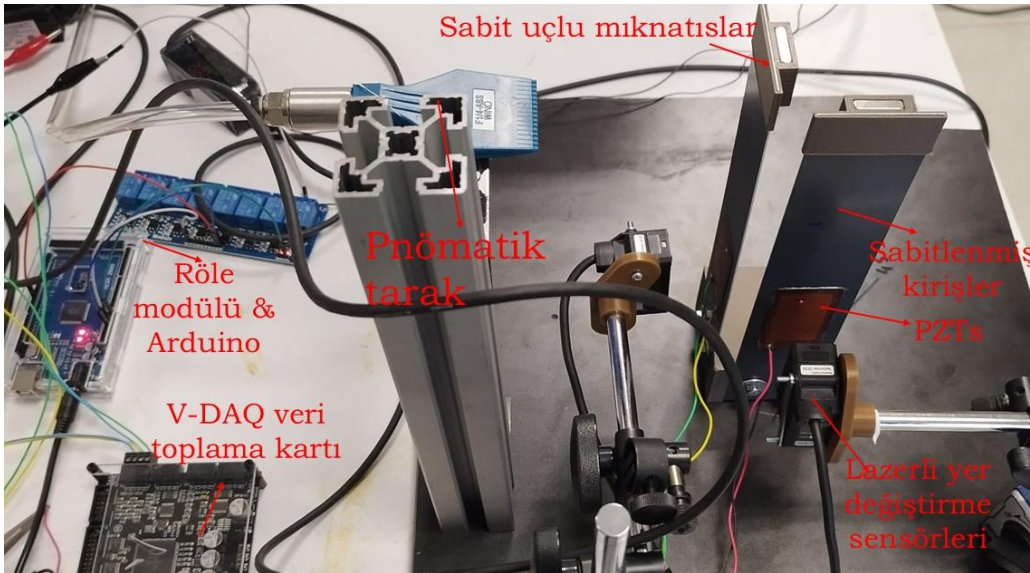
Şekil 4.4. Önerilen sistemin deneySEL düzenneđi.
