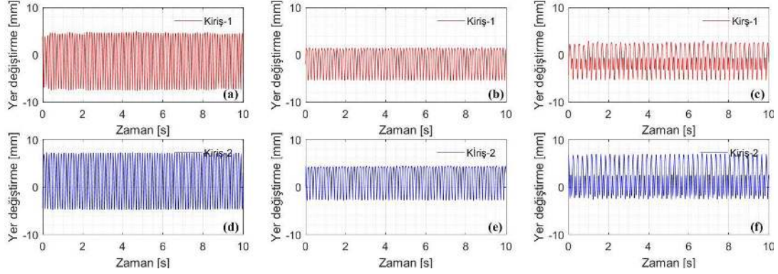
Şekil 6.8. Farklı rotor devir hızlarında kirişlerin yer değiştirme davranışı. (a) Beam-1: \omega = 500 rpm (b) Beam-1: \omega = 400 rpm (c) Beam-1: \omega = 300 rpm (d) Beam-2: \omega = 500 rpm (e) Beam-2: \omega = 400 rpm (f) Beam-2: \omega = 300 rpm.
