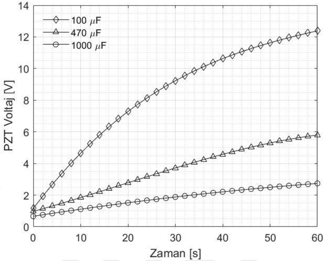
Şekil 6.11. Farklı kapasitör tiplerinin şarj hızları.
