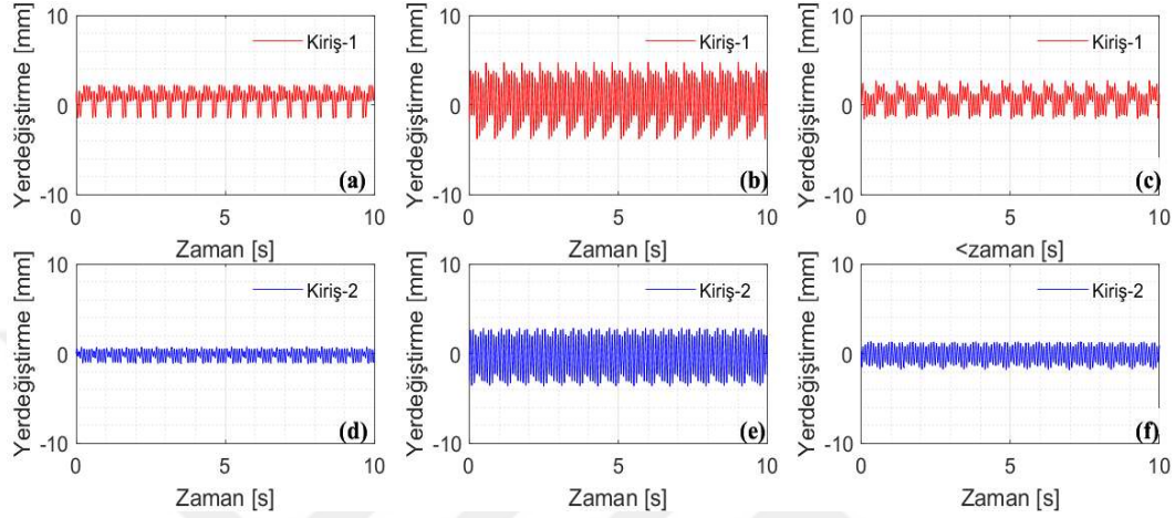
Şekil 6.4. Sistemin Yer Değiştirme Sonuçları: (a) Beam-1: T_p = 0.3 s, T_s = 0.2 s (b) Beam-1: T_p = 0.3 s, T_s = 0.3 s (c) Beam-1: T_p = 0.3 s, T_s = 0.4 s (d) Beam-2: T_p = 0.3 s, T_s = 0.2 s (e) Beam-2: T_p = 0.3 s, T_s = 0.3 s (f) Beam-2: T_p = 0.3 s, T_s = 0.4 s.
