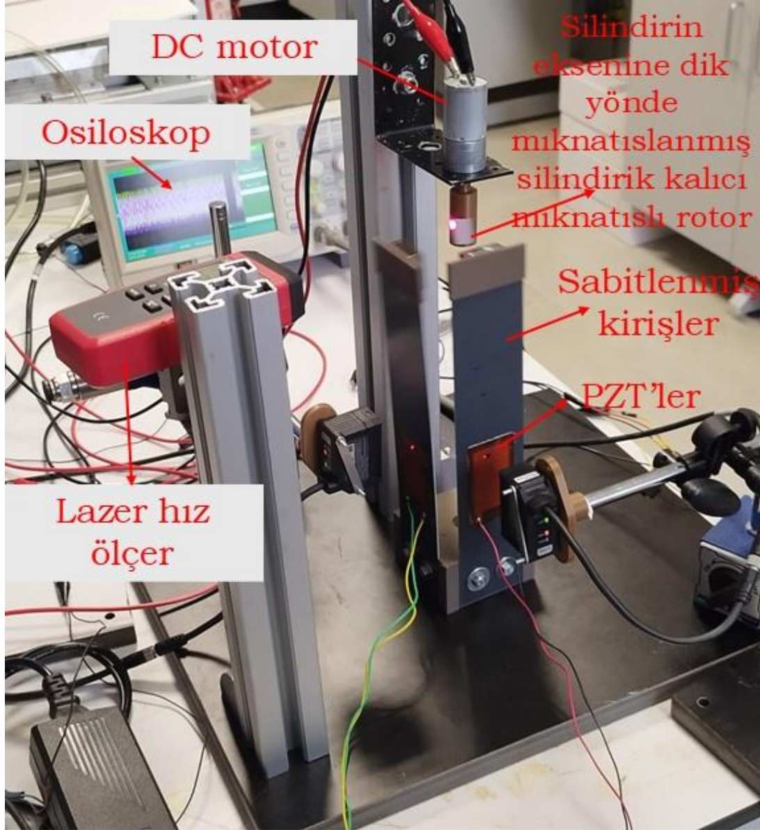
řekil 4.6. Dōnen manyetik uyarımlı deneysel dūzenek.
