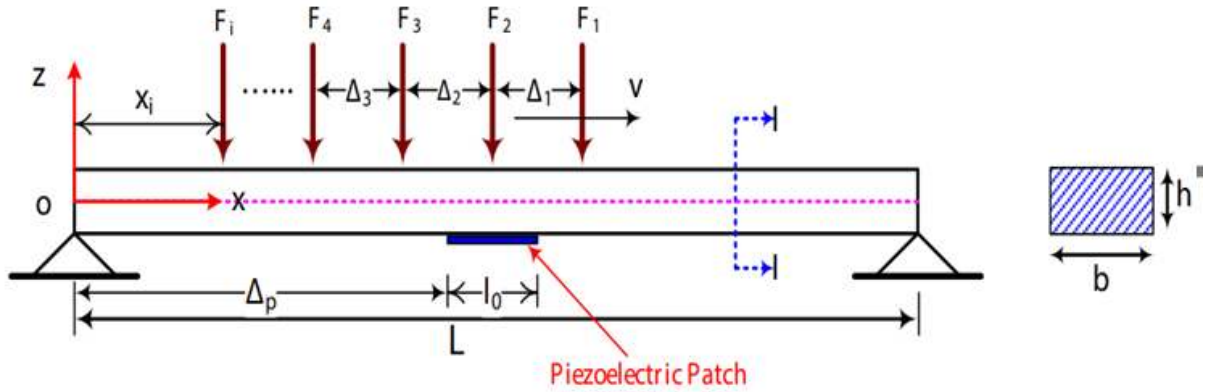
Şekil 2.2. Kiriş üzerine uygulanan dik yöndeki kuvvetler sayesinde gerçekleştirilen enerji hasadı
