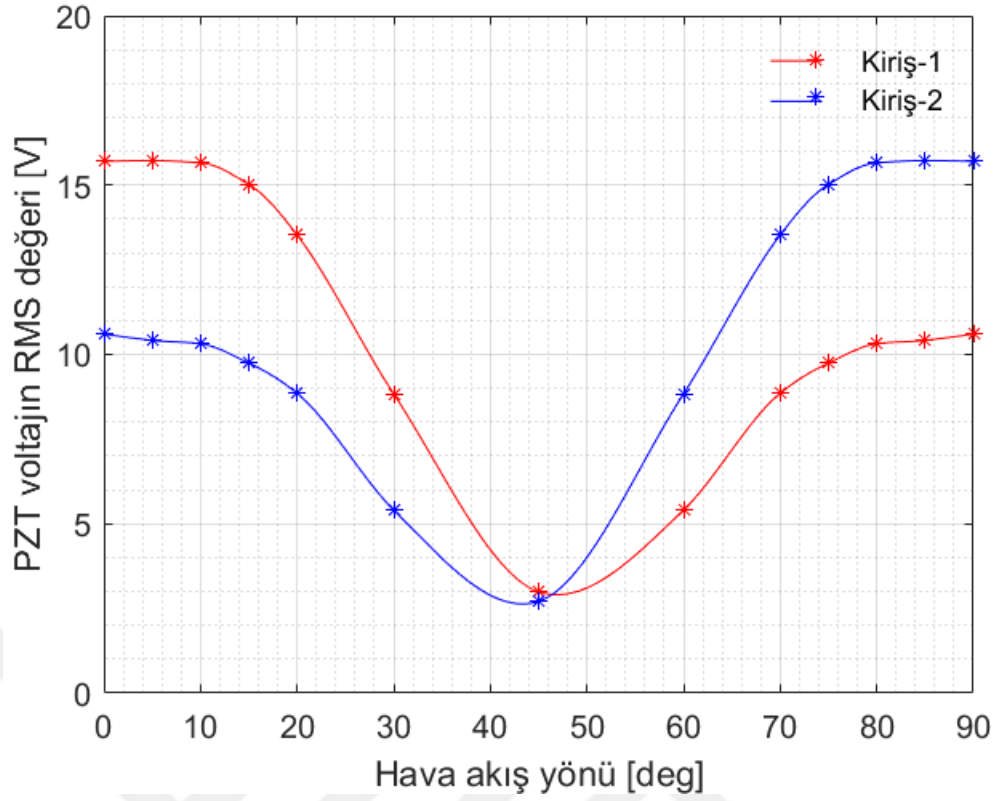
Şekil 6.6. Hava üfleme yönüne göre kirişler tarafından elde edilen RMS gerilim değerlerindeki değişim.
