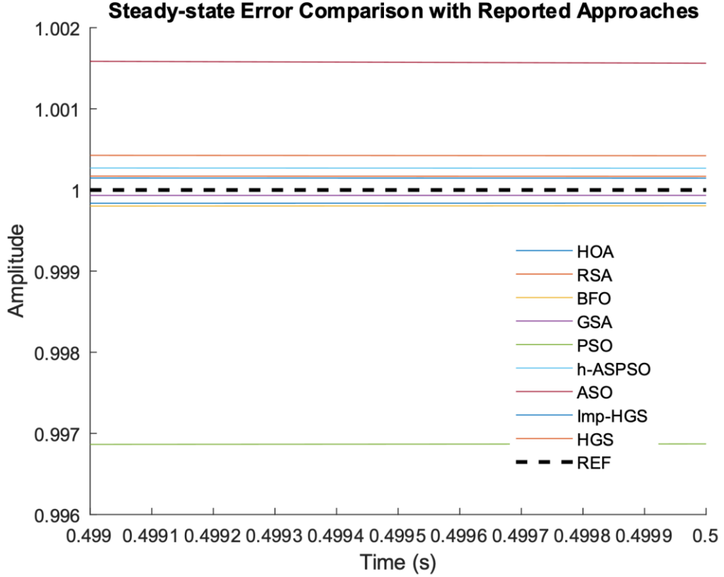
Şekil 6.6. HOA, RSA, BFO, GSA, PSO, h-ASPSO, ASO, Imp-HGS ve HGS uygulamalarından elde edilen karşılaştırmalı sabit durum hata değerleri
