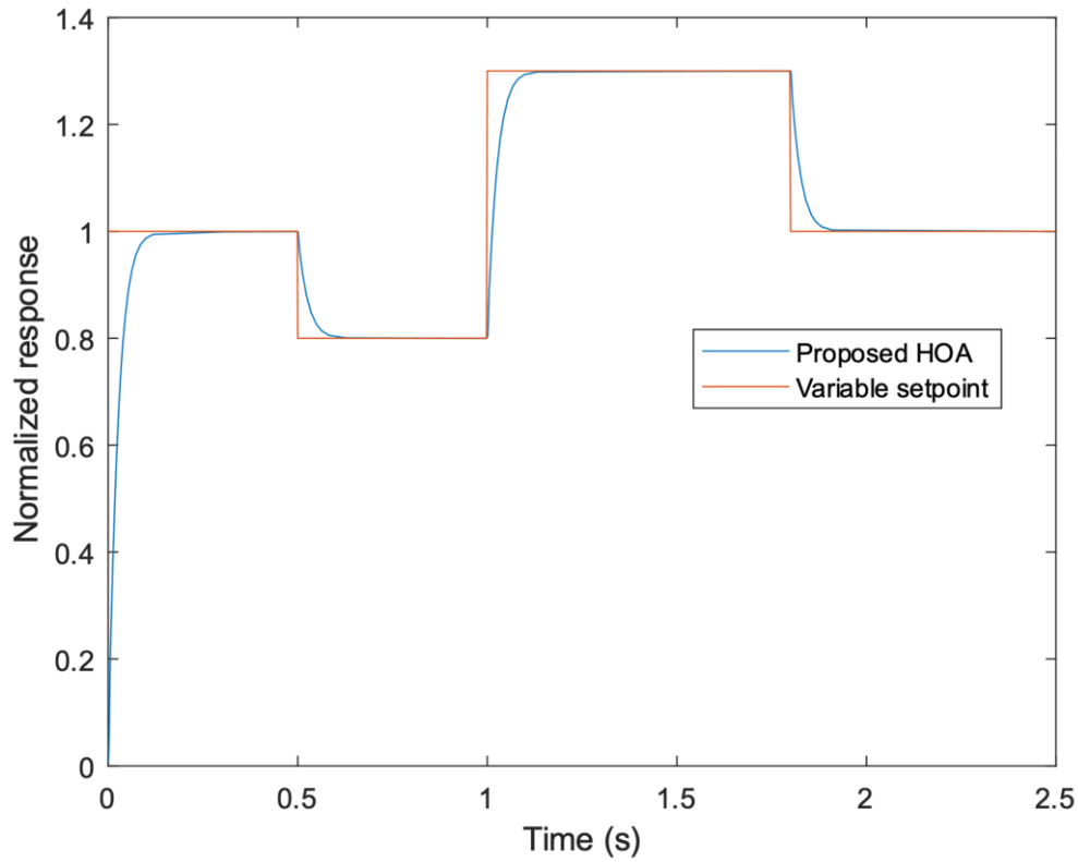
Şekil 6.7. Değişken giriş koşulları için HOA tabanlı yaklaşımın performans değerlendirmesi
