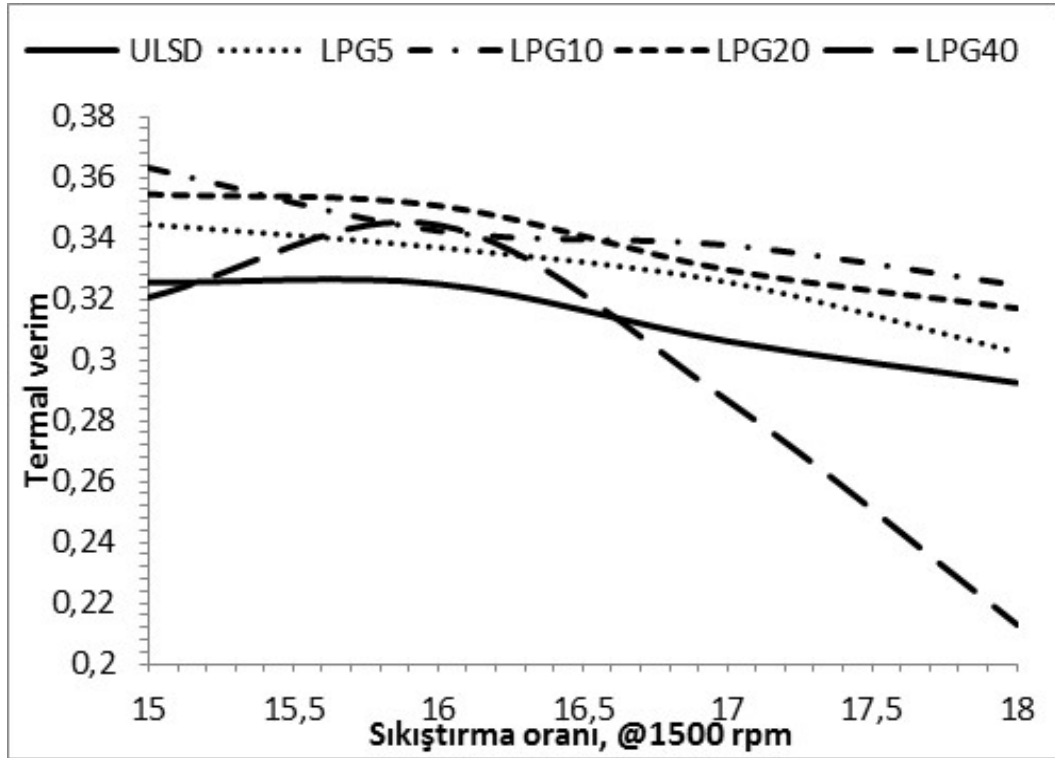
Şekil 5.9. Farklı sıkıştırma oranlarında termal verimlilik değışimi
