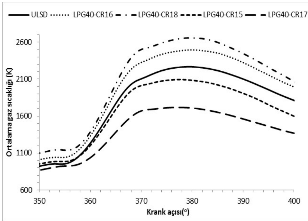
Şekil 5.13. Farklı krank açılarında Ortalama gaz sıcaklığı (K)
