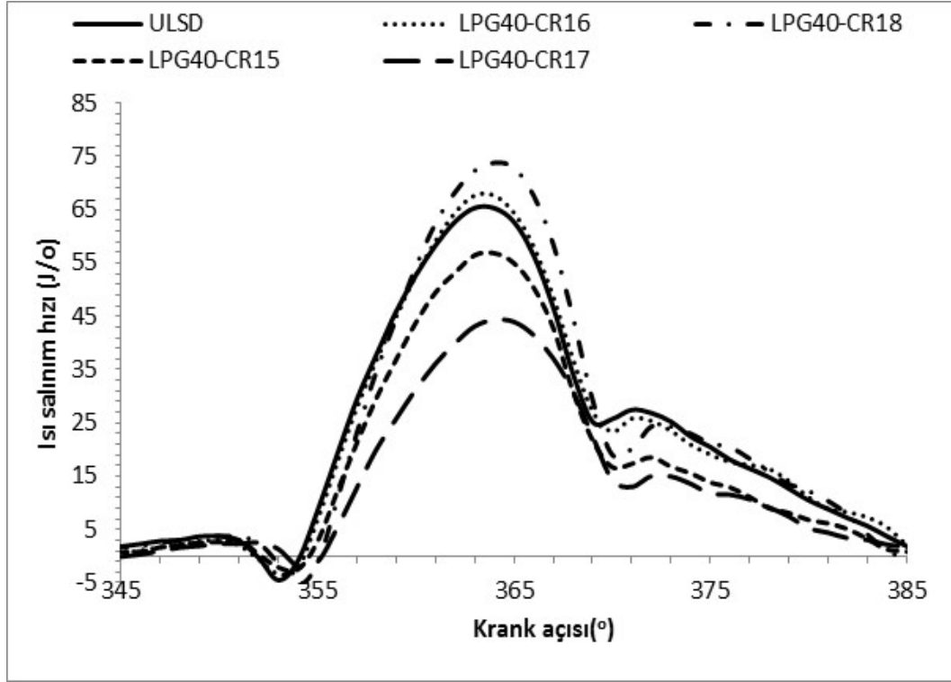
Şekil 5.12. Farklı krank açılarındaki Isı salınım hızı (j/o)
