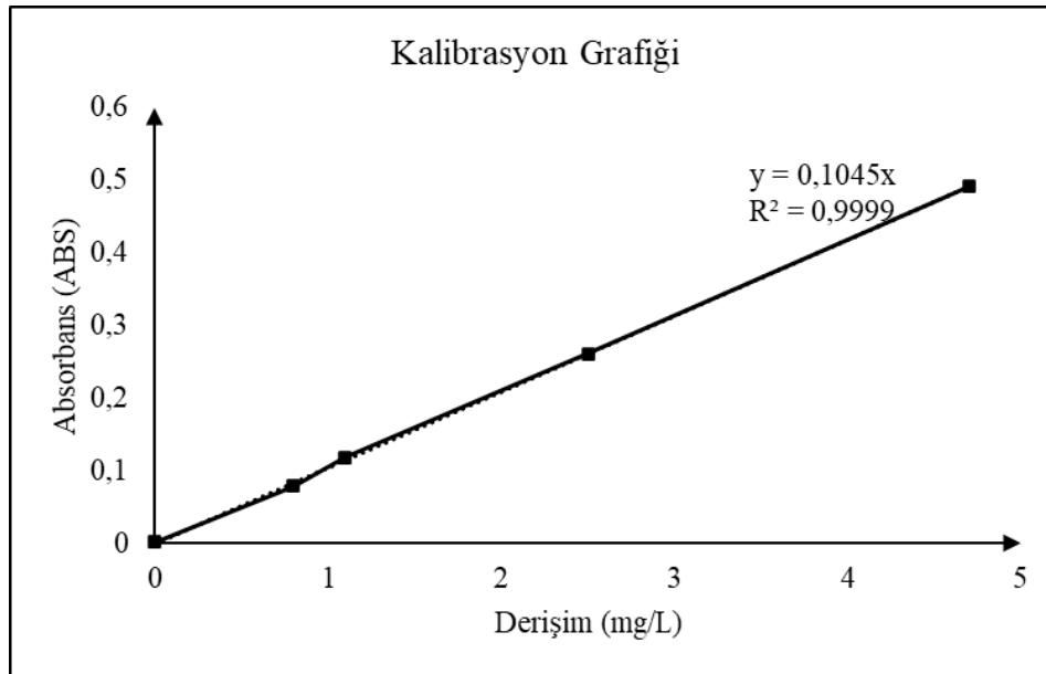
Şekil 6. 5. Kalibrasyon grafiği
