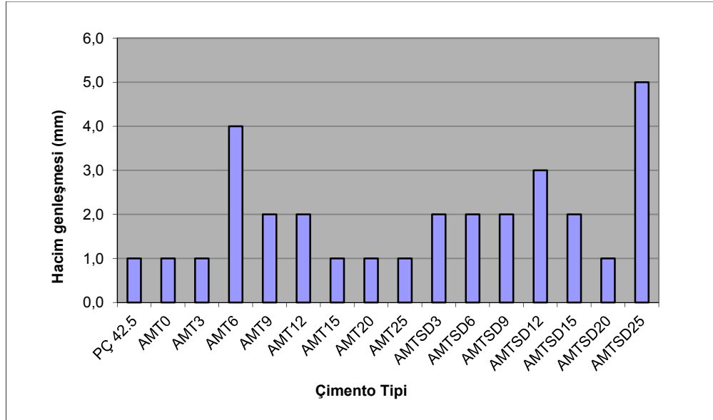
Şekil 4.6. Çimento tipi ile hacim genleşmesi ilişkisi
