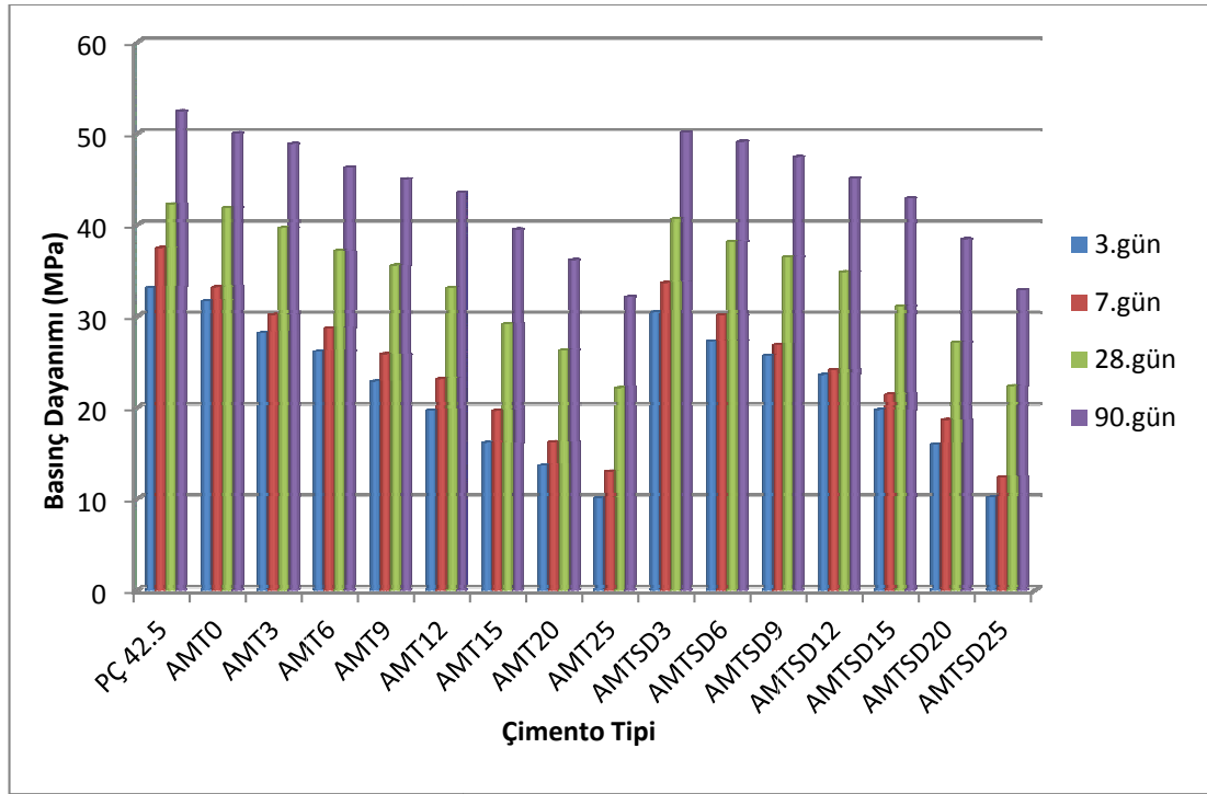
Şekil 4.12. Harçlarda çimento tipi ile basınç dayanımı ilişkisi
