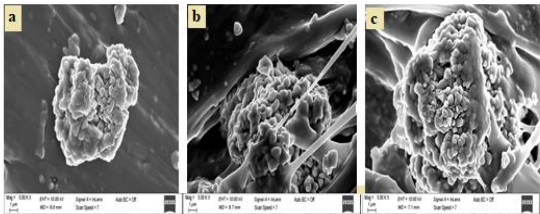
Şekil 3.4: Ölçek 5,00 KX, 1µm boyutlu soldan sağa sırasıyla a)%36,45, b)%39,06, c)%43,88 çinko borat katkılı TPU tanecik-polier etkileşimleri.
