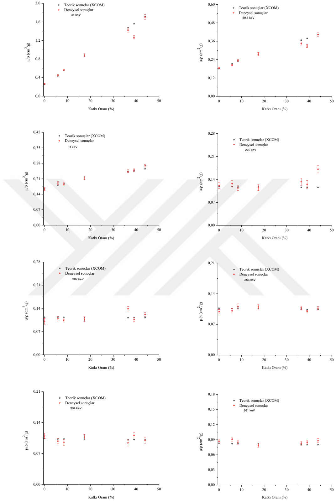
Şekil 3.15: Termoplastik poliüretan (TPU) örneklerinin teorik ve deneysel kütle azaltma katsayılarının 31-1332 keV enerji aralığında karşılaştırılması.
