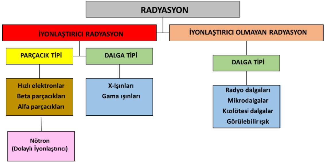
Şekil 1.4: Radyasyonun sınıflandırılması.
