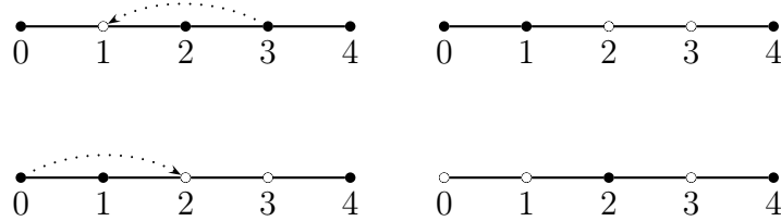
Şekil 3.26: P_5 yol çizgesi üzerinde solo test oyunu
