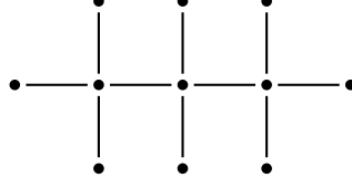
Şekil 2.12: Bir ağaç örneği
