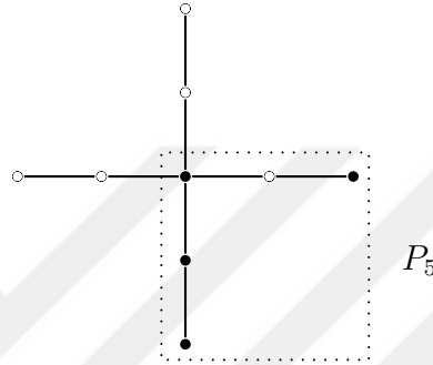
Şekil 3.30: (4, 2) -yıldız çizge
