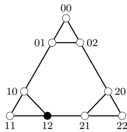
Şekil 4.42: Başlangıç deliği 00 köşesinde iken S(2,3) Sierpinski çizge üzerinde solo test oyunu
