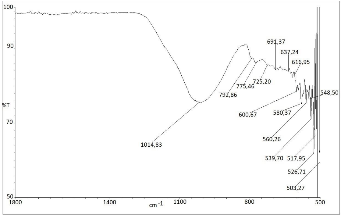
Şekil 3. 53. CZR-21 kodlu seramik örneğe ait FTIR spektrumu.
