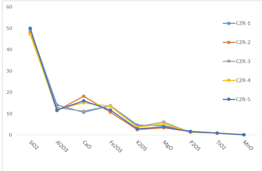
Portatif XRF analizinde tespit edilen oksit iççriklerinin numunelere göre dağılımını gösteren grafik (CZR-1 / CZR-5).
