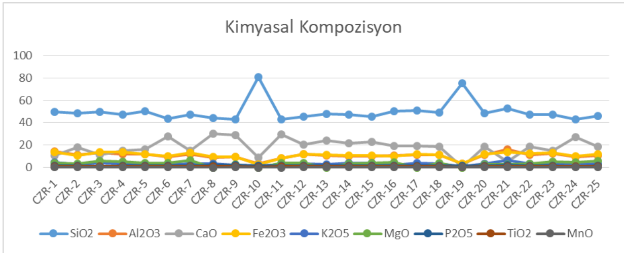
Şekil 3. 1. Numunelere ait p-XRF sonuçlarını gösteren grafik.
