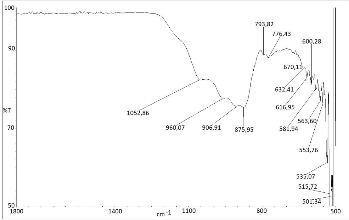
Şekil 3. 55. CZR-23 kodlu seramik örneğe ait FTIR spektrumu.
