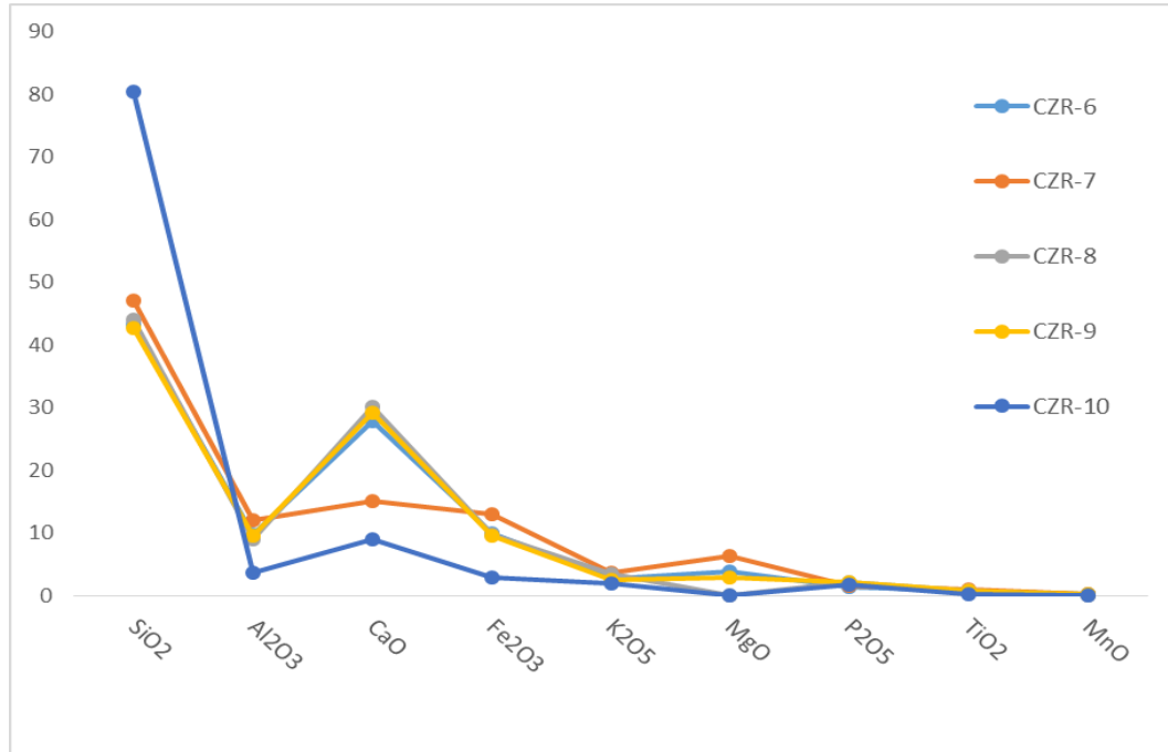
Portatif XRF analizinde tespit edilen oksit iççriklerinin numunelere göre dağılımını gösteren grafik (CZR-6 / CZR-10).
