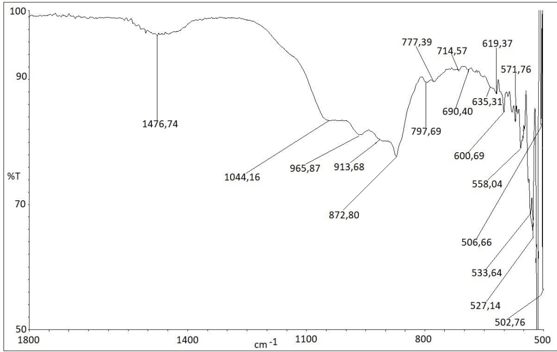
Şekil 3. 57. CZR-25 kodlu seramik örneğe ait FTIR spektrumu.
