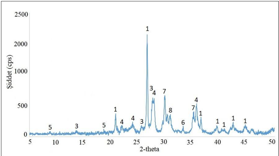
Şekil 3. 6. CZR-4 kodlu örneğe ait XRD paterni.
