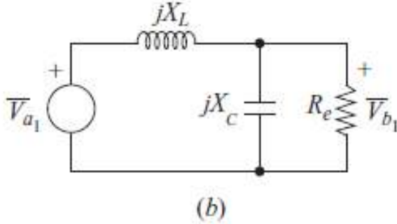
Şekil 3.4. -a) Paralel rezonans dönüştürücü devresi. -b) Paralel rezonans eşdeğer devresi
