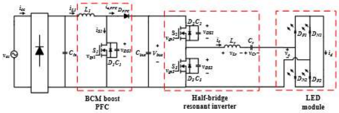
Şekil 2.11. Seri Rezonans dönüştürücülü aktif LED sürücü devresi
