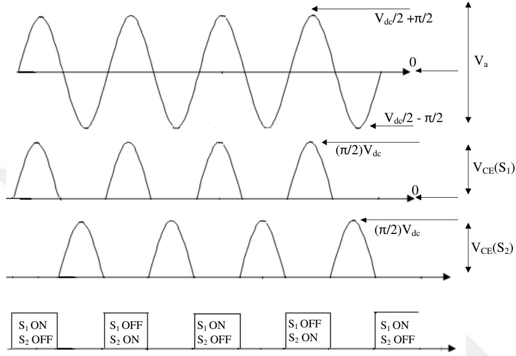
Şekil 3.2. Tasarlanması amaçlanan LED sürücü devresinde, anahtarlama gerilimleri ve anahtarlar üzerindeki gerilim dalga şekilleri
