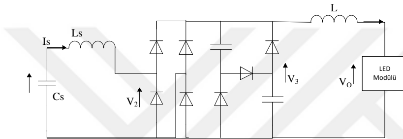
Şekil 2.7. Temel bir pasif LED sürücü devresi
