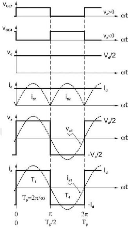
Şekil 3.2. Yarım köprü DC/AC dönüştürücünün temel dalga şekilleri
