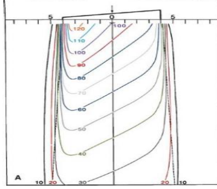
Şekil-2.14. Wedge filtre izodoz dağılımı (Khan, 2010)
