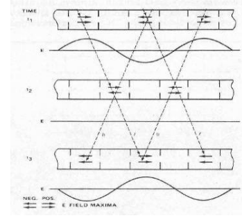
Şekil-2.10. Hızlandırıcı tüp Şekil-2.11. Elektronların hızlandırıcı tüp içerisinde hareketi (Khan, 2010).
