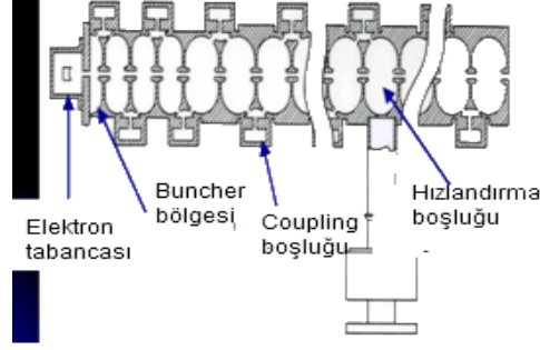
Şekil-2.10. Hızlandırıcı tüp Şekil-2.11. Elektronların hızlandırıcı tüp içerisinde hareketi (Khan, 2010).
