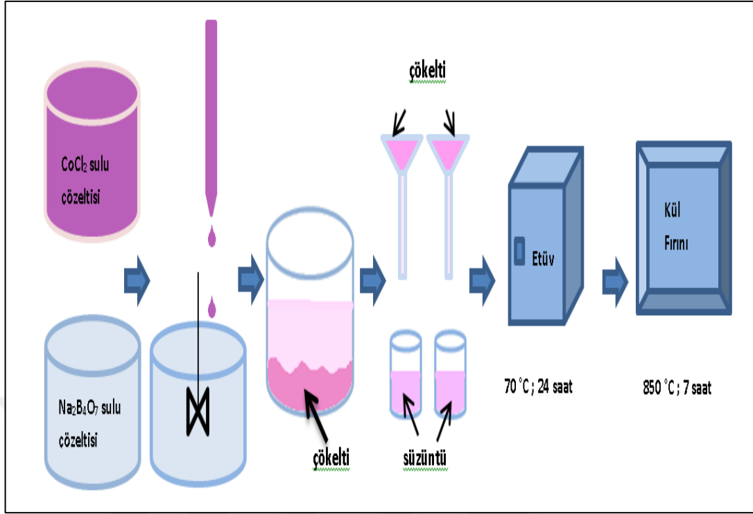
Şekil 4.4. Kobalt borat sentez sürecinin şematik gösterimi
