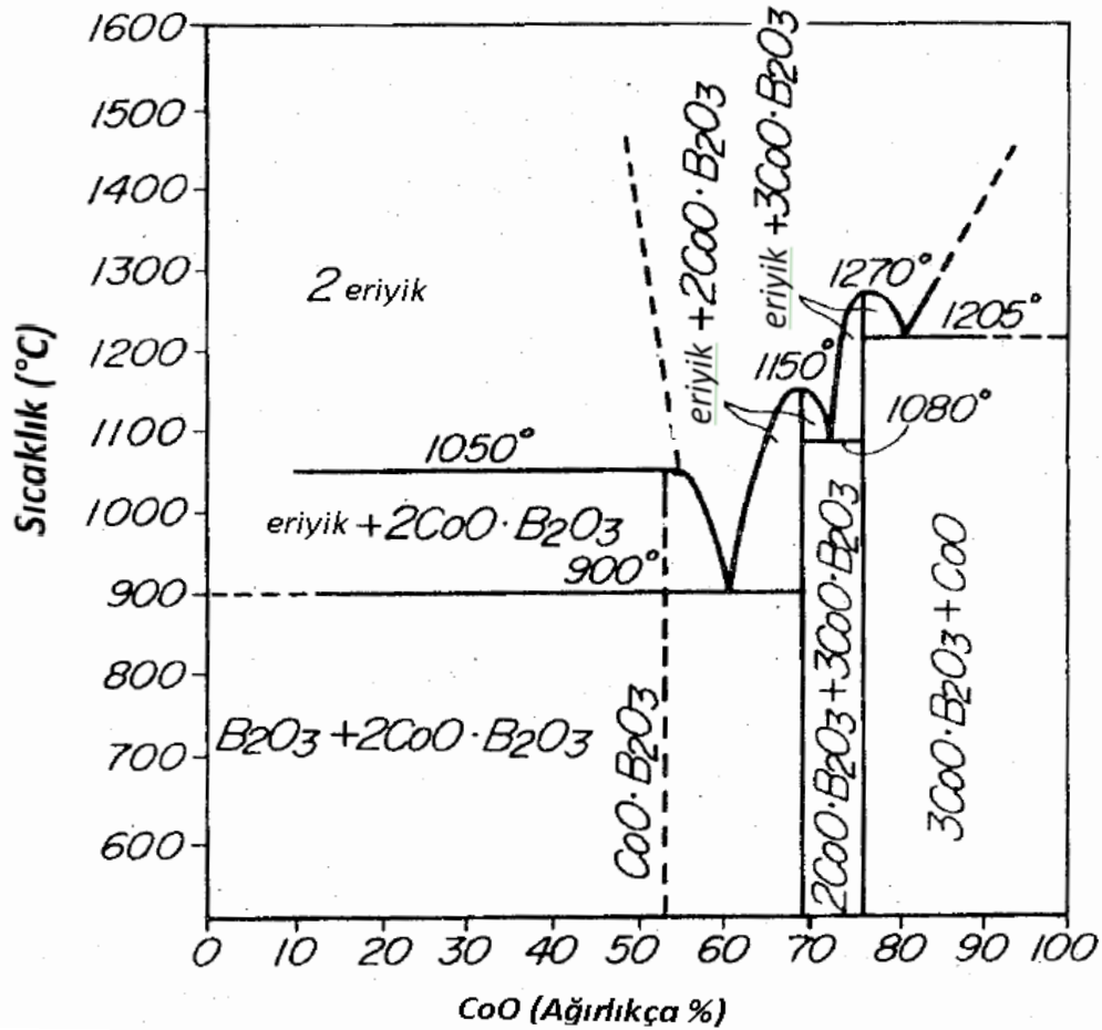
Şekil 3.1. \text{CoO}-\text{B}_2\text{O}_3 sistemi faz diyagramı [87]
