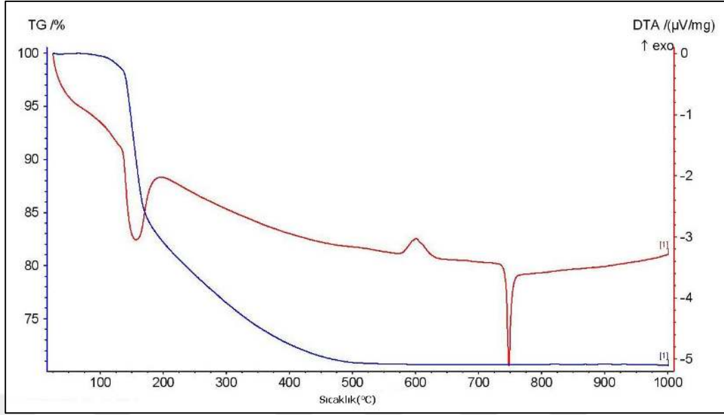
Şekil 4.2. Boraks pentahidrat ( \text{Na}_2\text{B}_4\text{O}_7 \cdot 5\text{H}_2\text{O} ) TG-DTA grafiği [27]
