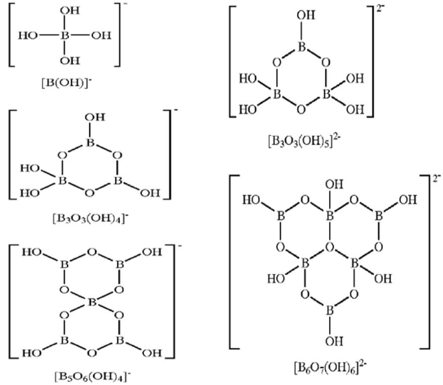
Şekil 2.1. Bazı borat anyonlarının yapısal gösterimi [32]
