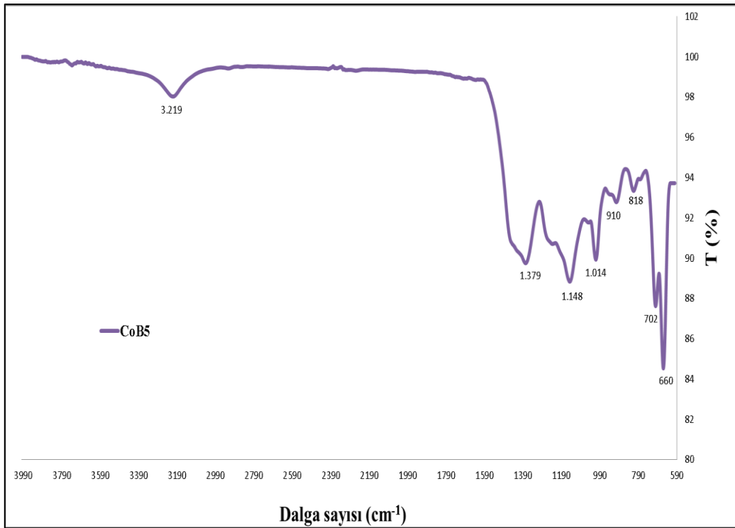
Şekil 5.10. CoB 5 nolu numunenin FTIR spektrumu.
