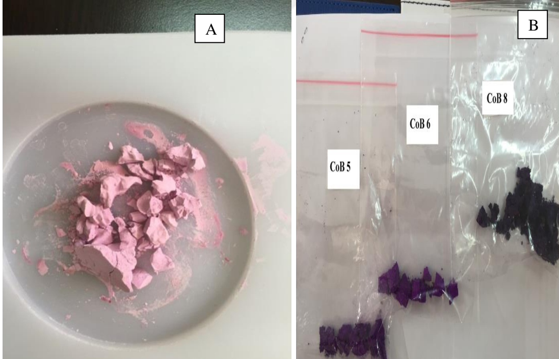
Şekil 4.8. Kobalt borat sentez deney görüntüleri - Kurutma aşaması (A: etüvde kurutma sonrası, B: ısıt işlem sonrası)
