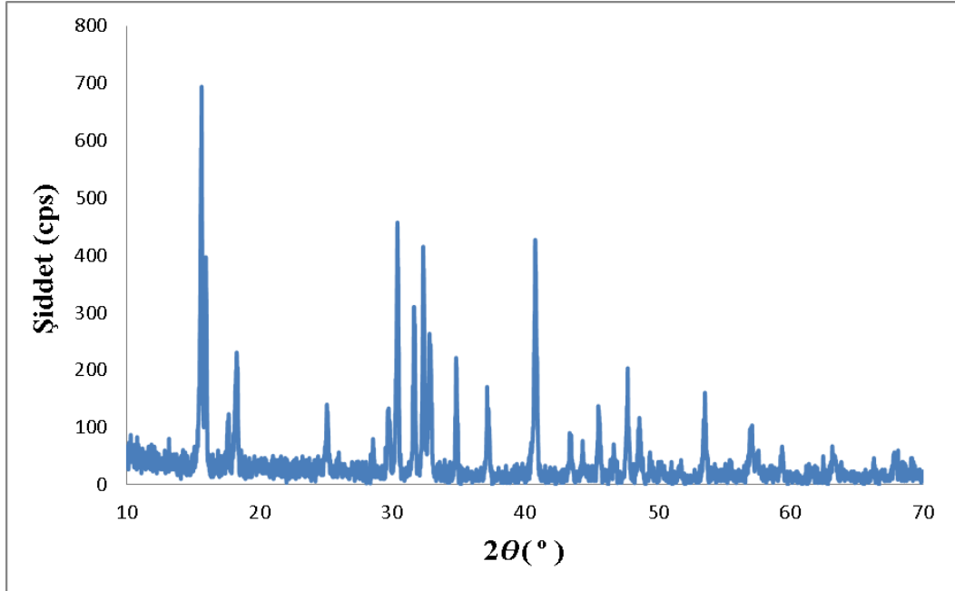
Şekil 4.3. Kobalt II klorür heksahidrat ( \text{CoCl}_2 \cdot 6\text{H}_2\text{O} ) XRD örüntüsü
